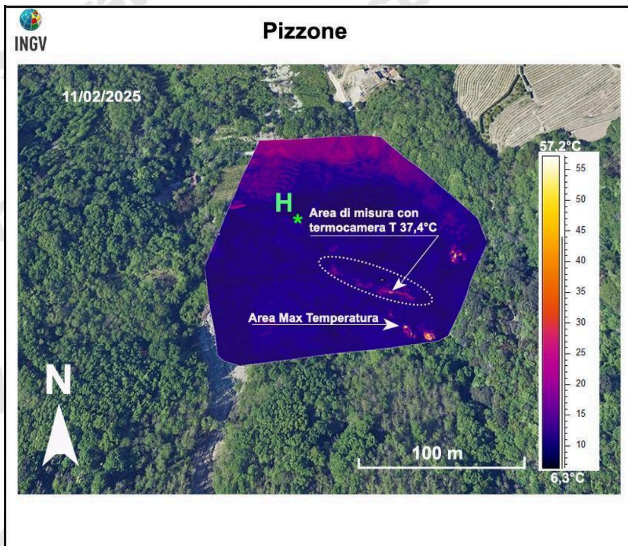
Figura 3.5 – Fotocomposizione di immagini termiche rilevate da drone nel mese di marzo 2025. H indica il sito di decollo e di atterraggio del drone. L'area racchiusa dalla linea tratteggiata è quella dove vengono effettuate le misure termiche mensili nell'area di Pizzone (Fig. 3.1h).
