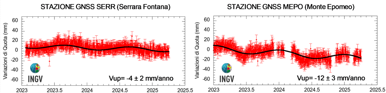
Figura 2.1.2 - Serie temporali delle variazioni giornaliere della componente verticale delle stazioni di SERR e MEPO (Ischia) da gennaio 2023 a marzo 2025.
