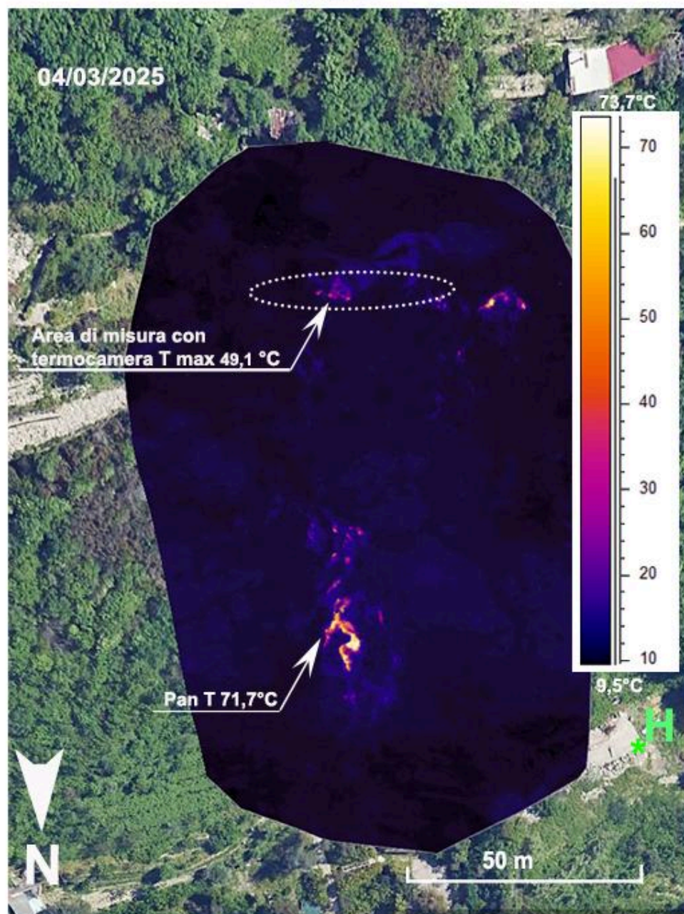
Figura 3.4 – Fotocomposizione di immagini termiche rilevate da drone nel mese di marzo 2025. H indica il sito di decollo e di atterraggio del drone. L'area racchiusa dalla linea tratteggiata è quella dove vengono effettuate le misure termiche mensili nell'area di Pantane (Fig. 3.1a).
