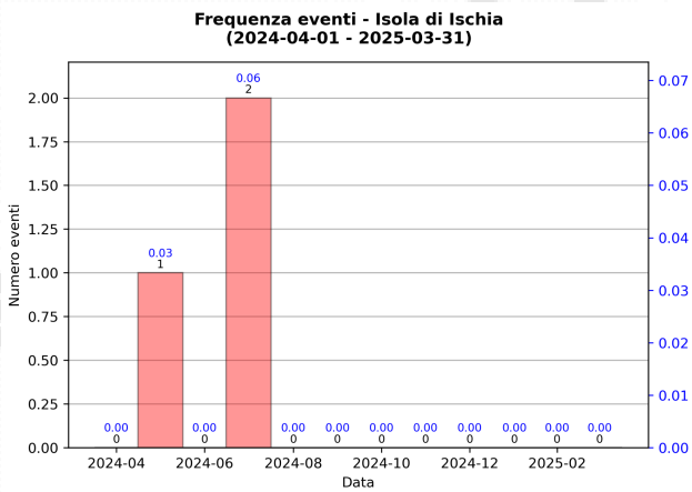
Figura 1.3 – (A sinistra) Numero di eventi registrati ad Ischia nel corso degli ultimi 12 mesi (in totale 3). (A destra) profondità ipocentrali degli eventi registrati ad Ischia nel corso degli ultimi 12 mesi.
