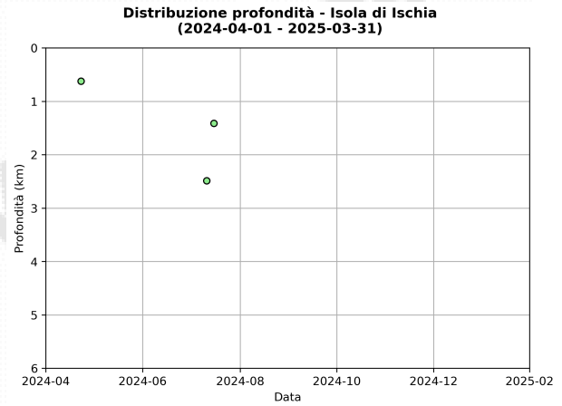
Figura 1.3 – (A sinistra) Numero di eventi registrati ad Ischia nel corso degli ultimi 12 mesi (in totale 3). (A destra) profondità ipocentrali degli eventi registrati ad Ischia nel corso degli ultimi 12 mesi.
