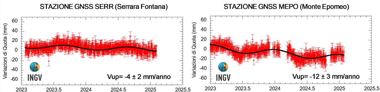
Figura 2.1.2 - Serie temporali delle variazioni giornaliere della componente verticale delle stazioni di SERR e MEPO (Ischia) da gennaio 2023 a gennaio 2025.
