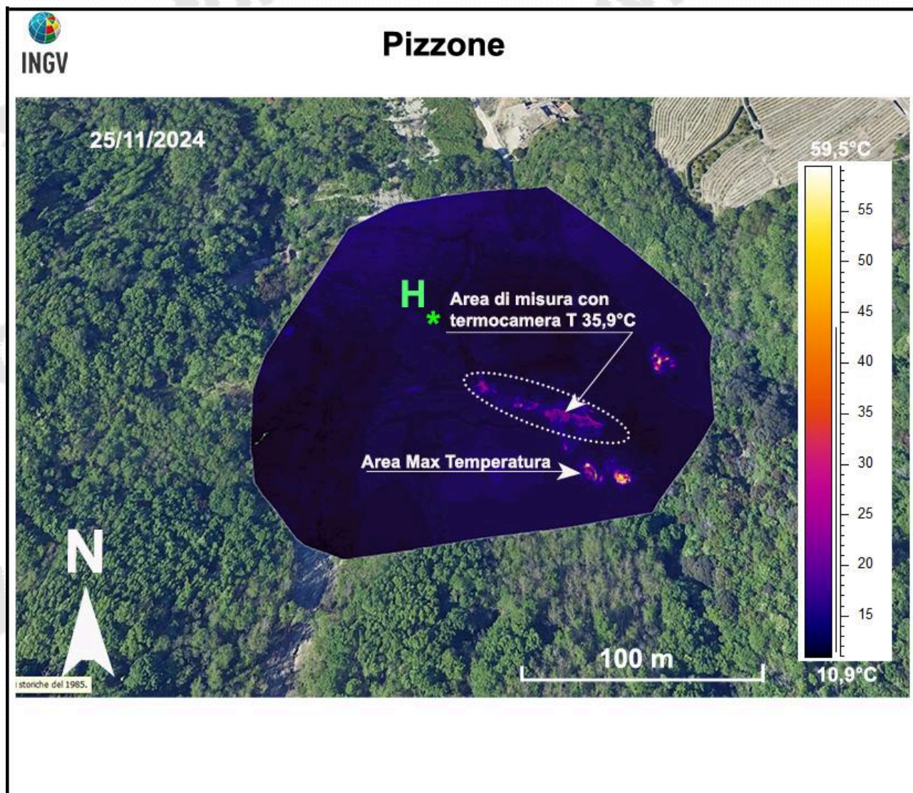
Figura 3.6 – Fotocomposizione di immagini termiche rilevate da drone nel mese di novembre 2024. H indica il sito di decollo e di atterraggio del drone. L'area racchiusa dalla linea tratteggiata è quella dove vengono effettuate le misure termiche mensili nell'area di Pizzone (Fig. 3.1h).
