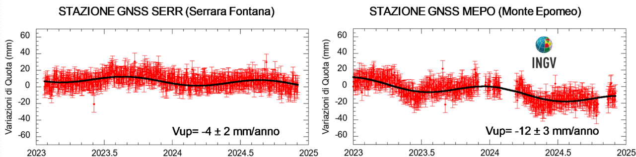
Figura 2.1.2 - Serie temporali delle variazioni giornaliere della componente verticale delle stazioni di SERR e MEPO (Ischia) da gennaio 2023 a novembre 2024.
