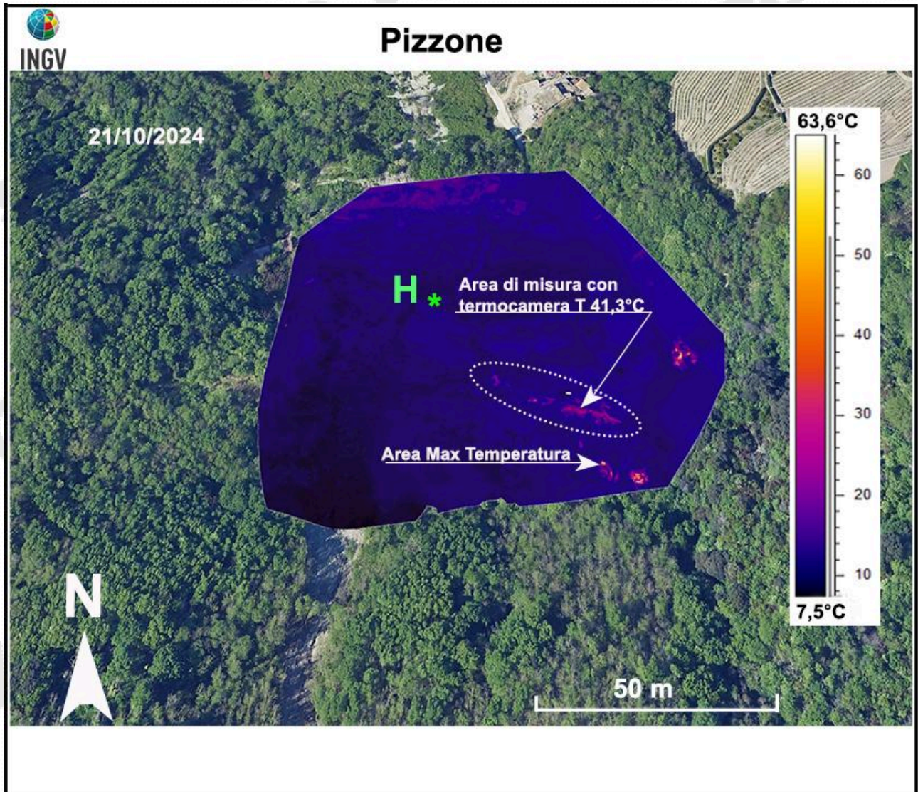
Figura 3.6 – Fotocomposizione di immagini termiche rilevate da drone nel mese di ottobre 2024. H indica il sito di decollo e di atterraggio del drone. L'area racchiusa dalla linea tratteggiata è quella dove vengono effettuate le misure termiche mensili nell'area di Pizzone (Fig. 3.1h).
