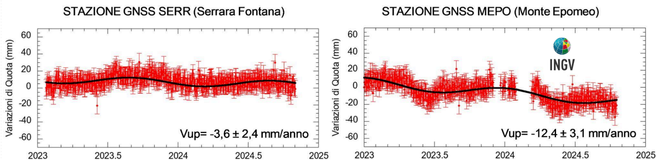
Figura 2.1.2 - Serie temporali delle variazioni giornaliere della componente verticale delle stazioni di SERR e MEPO (Ischia) da gennaio 2023 a ottobre 2024.
