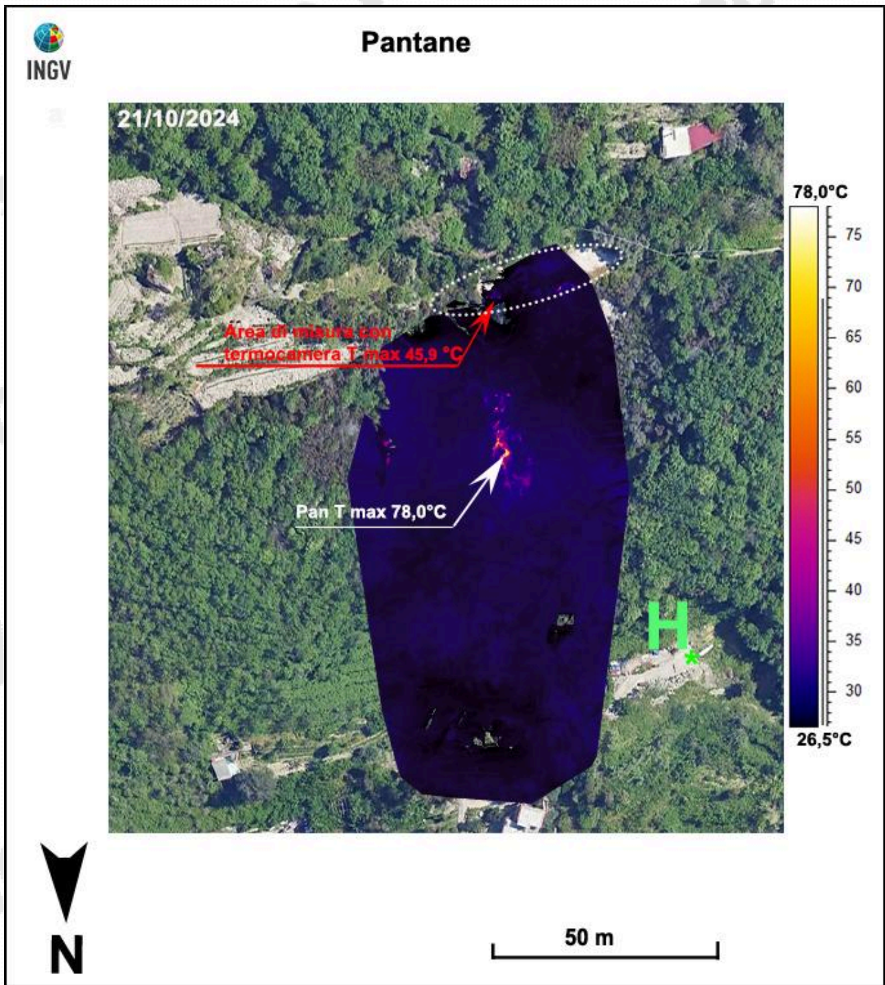
Figura 3.4 – Fotocomposizione di immagini termiche rilevate da drone nel mese di ottobre 2024. H indica il sito di decollo e di atterraggio del drone. L'area racchiusa dalla linea tratteggiata è quella dove vengono effettuate le misure termiche mensili nell'area di Pantane (Fig. 3.1a).
