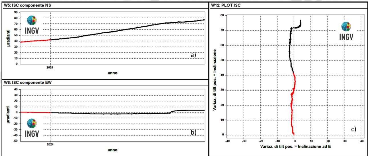
Figura 2.2.2 - Serie temporali e plot del tilt della stazione ISC della rete di Ischia registrati negli ultimi 12 mesi (novembre 2023 - ottobre 2024).
