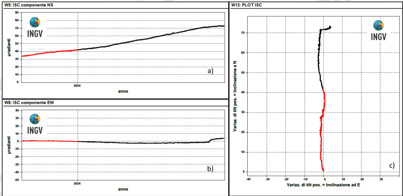
Figura 2.2.2 - Serie temporali e plot del tilt della stazione ISC della rete di Ischia registrati negli ultimi 12 mesi (ottobre 2023 - settembre 2024).
