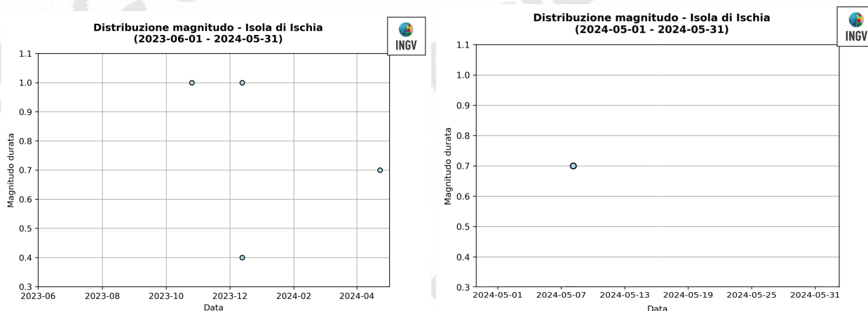
Figura 1.5 – Magnitudo degli eventi registrati ad Ischia nel corso degli ultimi 12 mesi, a sinistra, e nel corso dell'ultimo mese, a destra.
