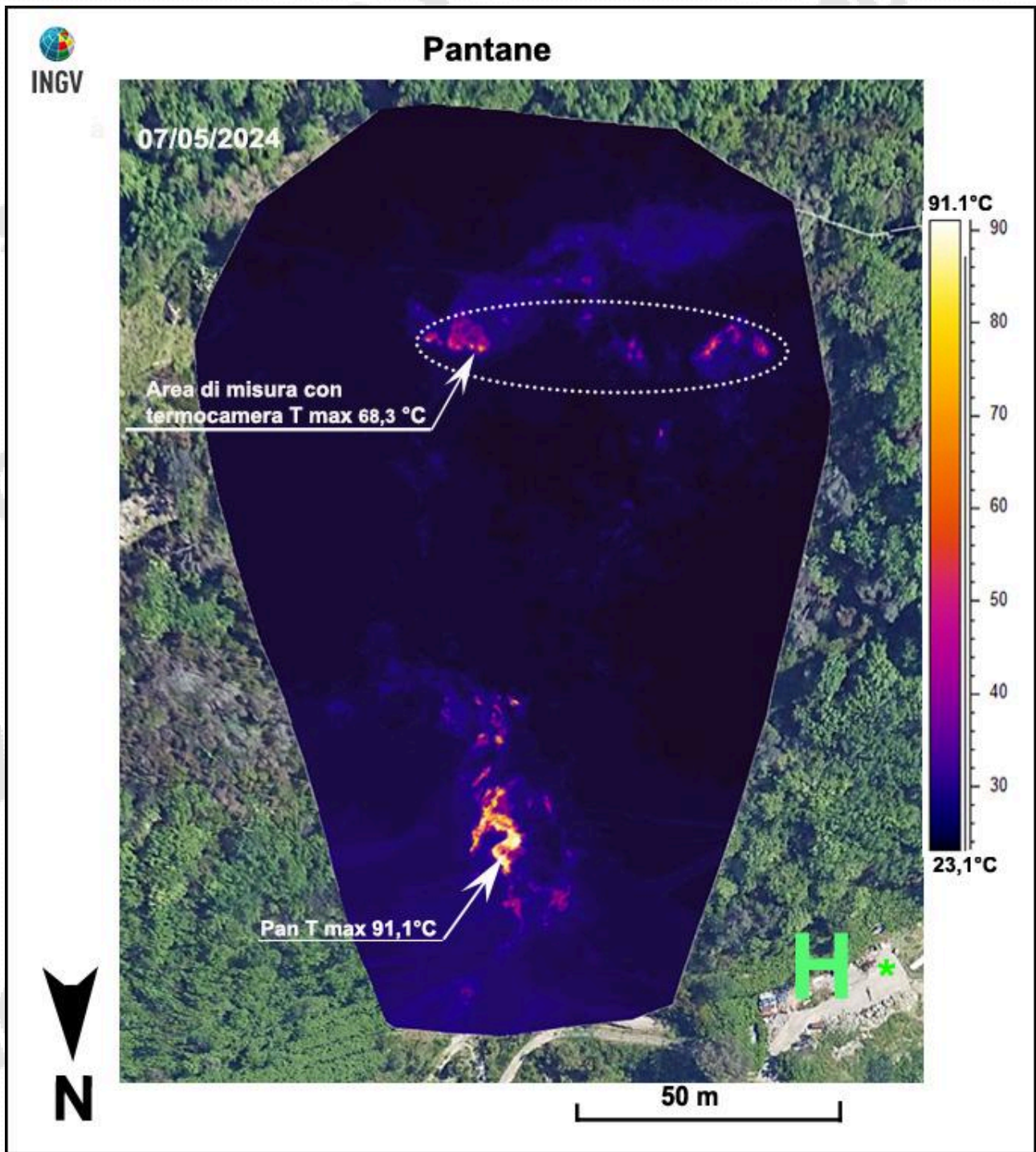
Figura 3.4 – Fotocomposizione di immagini termiche rilevate da drone nel mese di maggio 2024. H indica il sito di decollo e di atterraggio del drone. L'area racchiusa dalla linea tratteggiata è quella dove vengono effettuate le misure termiche mensili nell'area di Pantane (Fig. 3.1a).
