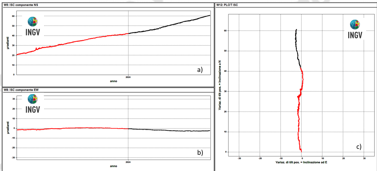
Figura 2.2.2 - Serie temporali e plot del tilt della stazione ISC della rete di Ischia registrati negli ultimi 12 mesi (giugno 2023 - maggio 2024).
