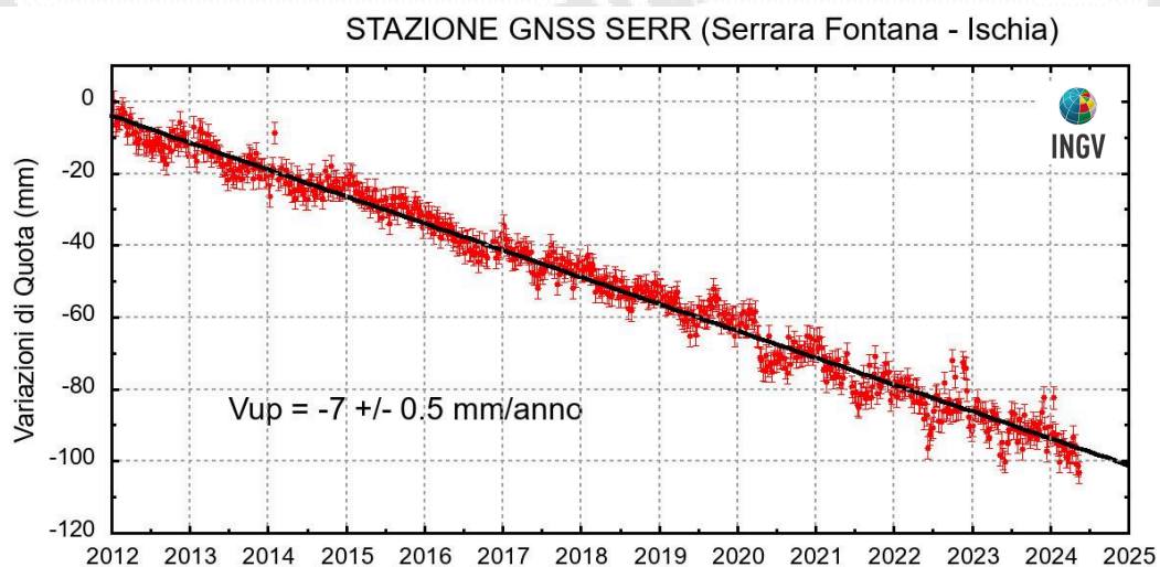
Figura 2.1.2 - Serie temporale delle variazioni settimanali in quota della stazione di SERR (Ischia) da gennaio 2012 a maggio 2024.
