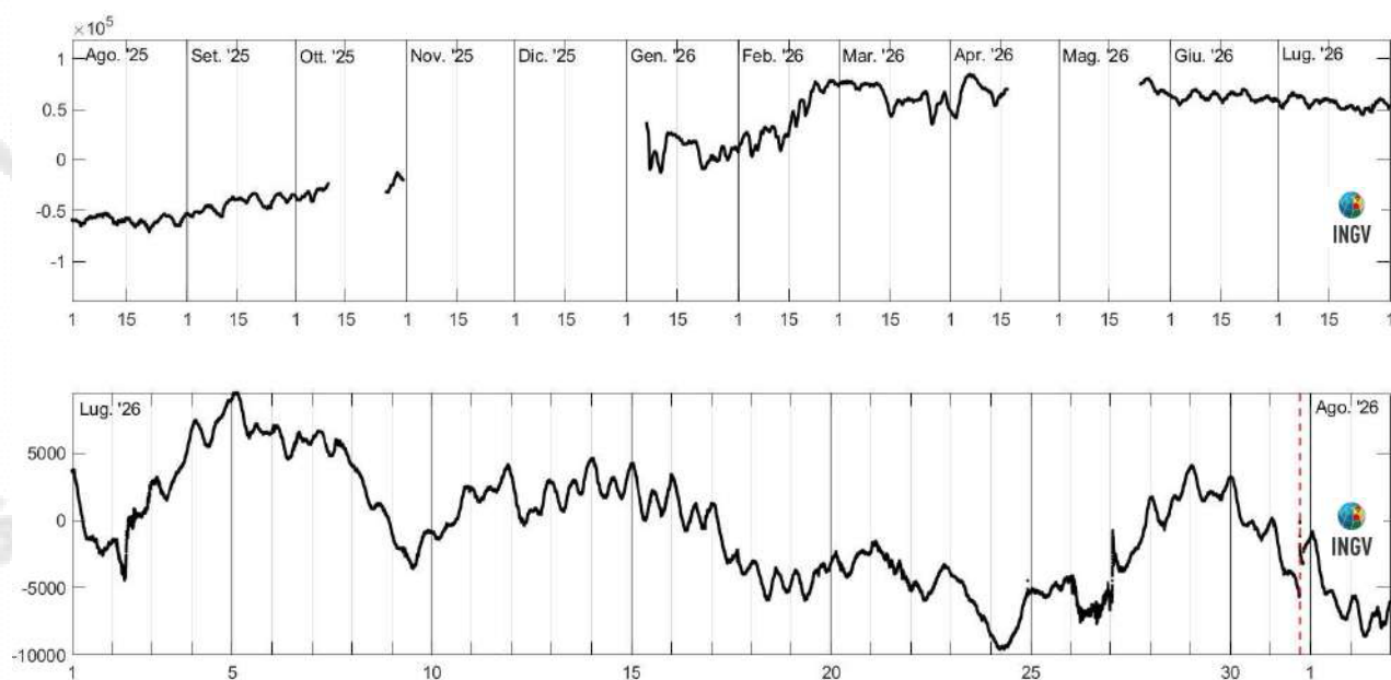
Figura 2.5.2 - Strain registrato dalla stazione dilatometrica di Quarto. In alto è mostrato lo strain registrato nell'ultimo anno, dalle 00:00 UTC del 1/08/2025 alle 24:00 UTC del 31/07/2026. In basso, i dati di strain disponibili nell'ultimo periodo, dalle 00:00 UTC del 01/07/2026 alle 24:00 UTC del 2/08/2026. La linea verticale rossa tratteggiata indica il tempo d'origine del terremoto di magnitudo M_d=4.7 .
