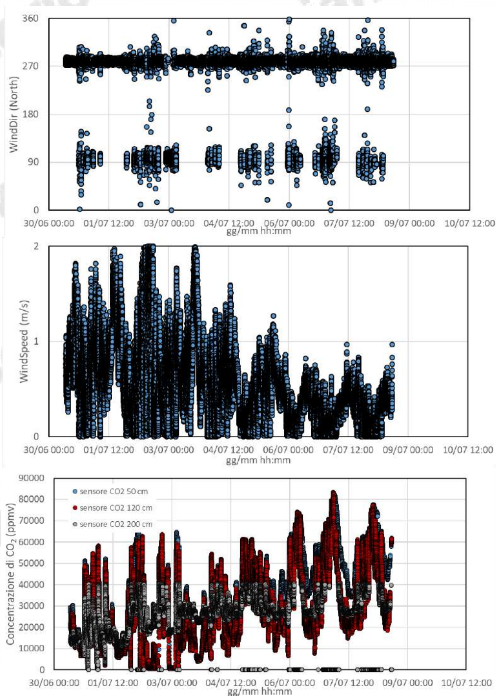
Figura 4.21 - Dati acquisiti dalla stazione installata nella galleria della Linea 2 della Metropolitana di Napoli, tratta Pozzuoli Solfatara - Napoli Campi Flegrei, nel periodo 30 giugno - 7 luglio 2026: a) direzione del vento in gradi da Nord in senso orario; b) intensità del vento in m/s; c) concentrazione di CO 2 in aria, espressa in ppmv, a tre differenti quote dal suolo (50 cm, 120 cm e 200 cm). Nel periodo considerato sono state misurate concentrazioni superiori a circa 8% in volume, corrispondenti a circa 80.000 ppmv. Il sensore di CO 2 posto a più alta quota dal suolo ha mostrato un malfunzionamento a partire dal 5 luglio.
