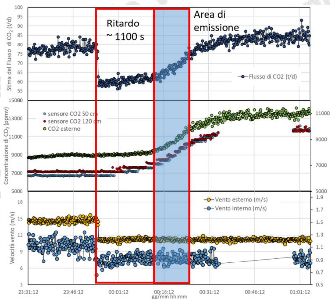
Figura 4.25 - Dati acquisiti dalle stazioni geochimiche posizionate all'interno della galleria e davanti a una delle due turbine utilizzate per l'aerazione forzata della galleria. La variazione di potenza di estrazione delle turbine è stata usata per individuare il settore della galleria caratterizzato dalla maggiore emissione di gas.
