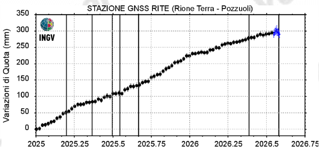
Figura 2.1.3 - Serie temporale delle variazioni in quota della stazione GNSS di RITE dal 01/01/2025 al 02/08/2026. Elaborazione dati con software GNSS Bernese. Le linee nere verticali indicano le date di occorrenza nel periodo degli eventi sismici di M_d \geq 4.0 .
