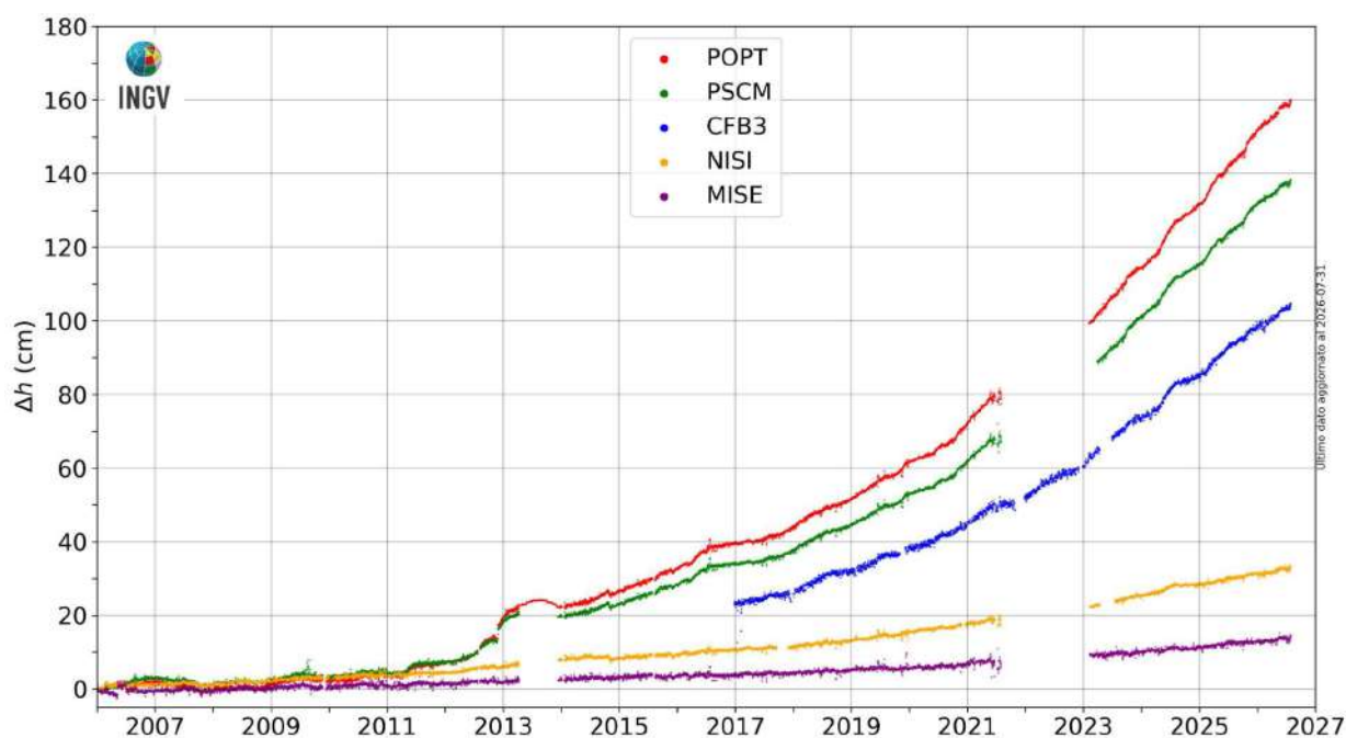
Figura 2.3.4 - Movimenti verticali del suolo nel periodo gennaio 2006 – luglio 2026, ottenuti dall'analisi dei dati acquisiti da tutte le stazioni mareografiche dell'area della caldera Flegrea. Le variazioni, riportate in cm, rappresentano le medie giornaliere e sono tutte riferite alla stazione mareografica di Napoli, molo San Vincenzo (NAMM).
