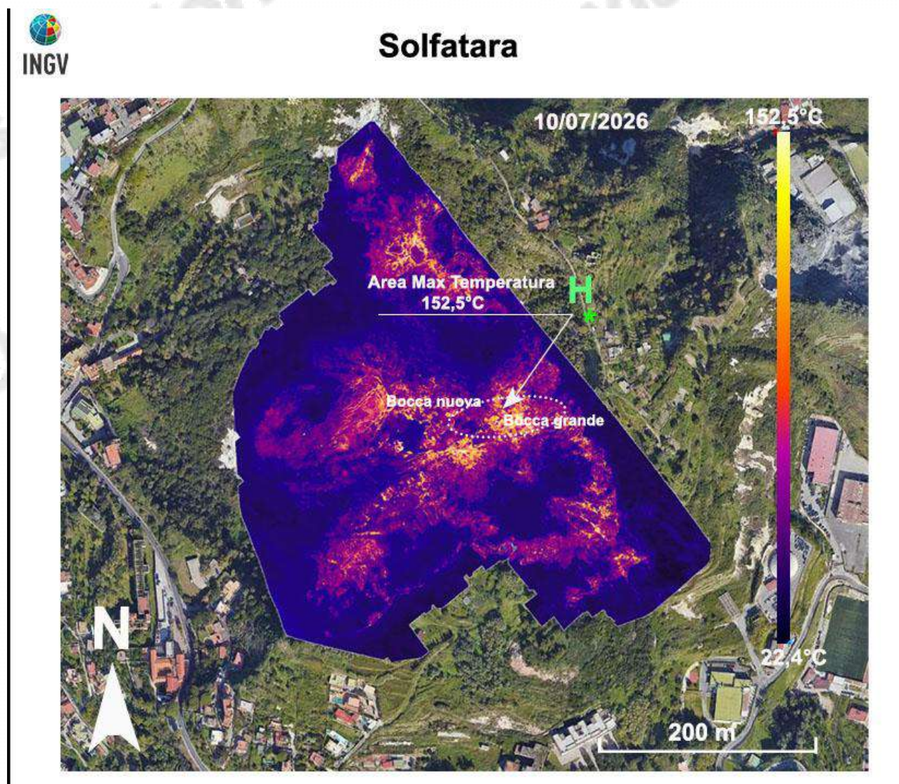
Figura 3.2.4 – Fotocomposizione di immagini termiche rilevate da drone nel mese di luglio 2026 su La Solfatara (Solf in figura 3.2.1.B). H* indica il sito di decollo e di atterraggio del drone corrispondente al punto S1 di Fig.3.2.1.B.
