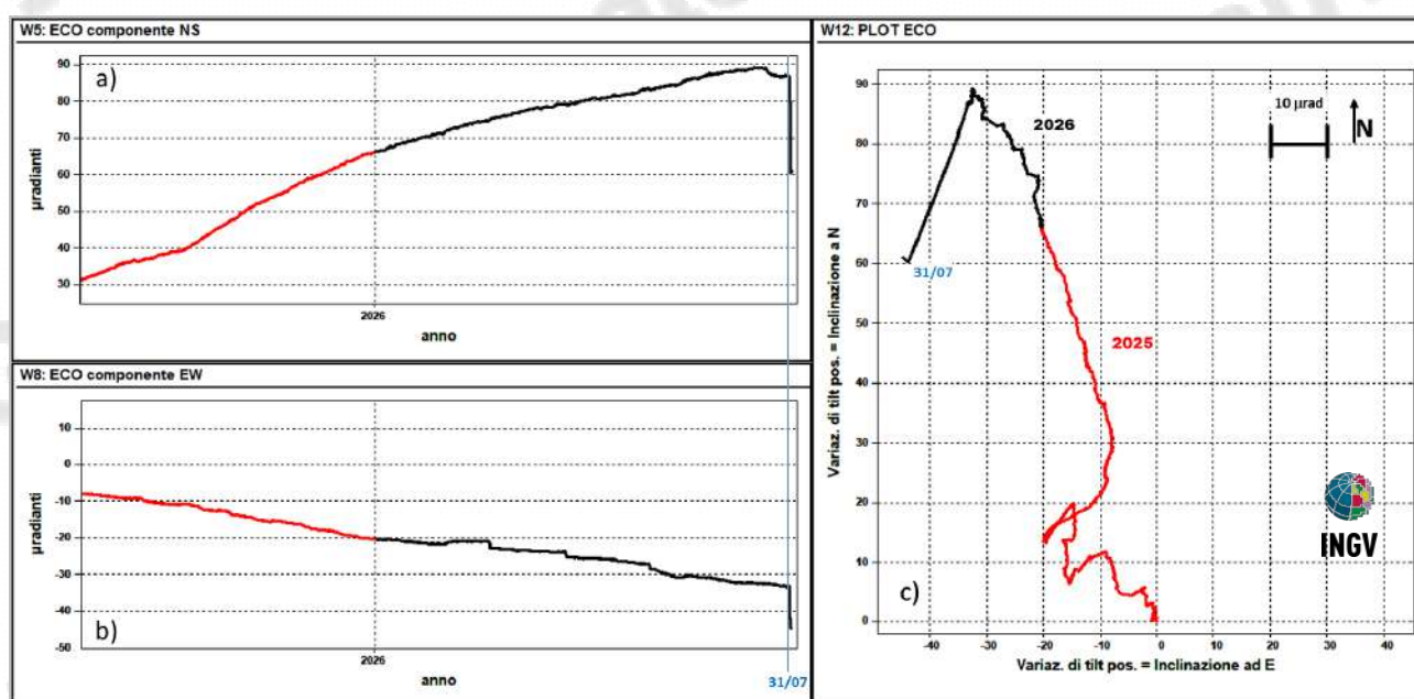
Figura 2.2.3 – Serie temporali e plot (ultimi 12 mesi) del tilt della stazione ECO della rete dei Campi Flegrei.
