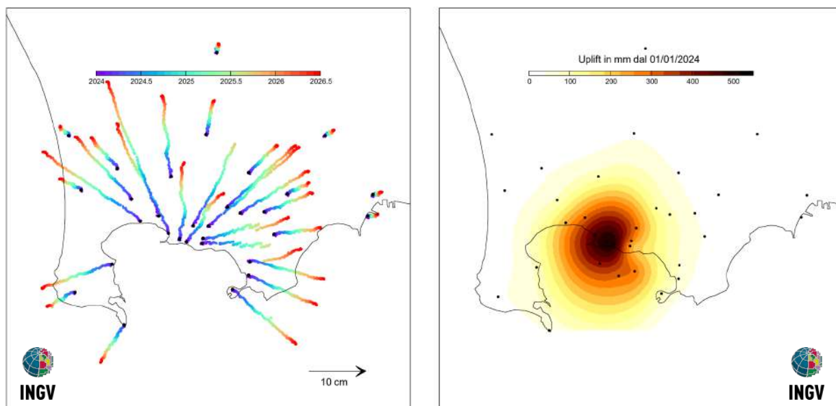
Figura 2.1.7 - Mappa degli spostamenti GNSS orizzontali (a) e verticali (b) registrati nell'area flegrea da gennaio 2024 a luglio 2026.
