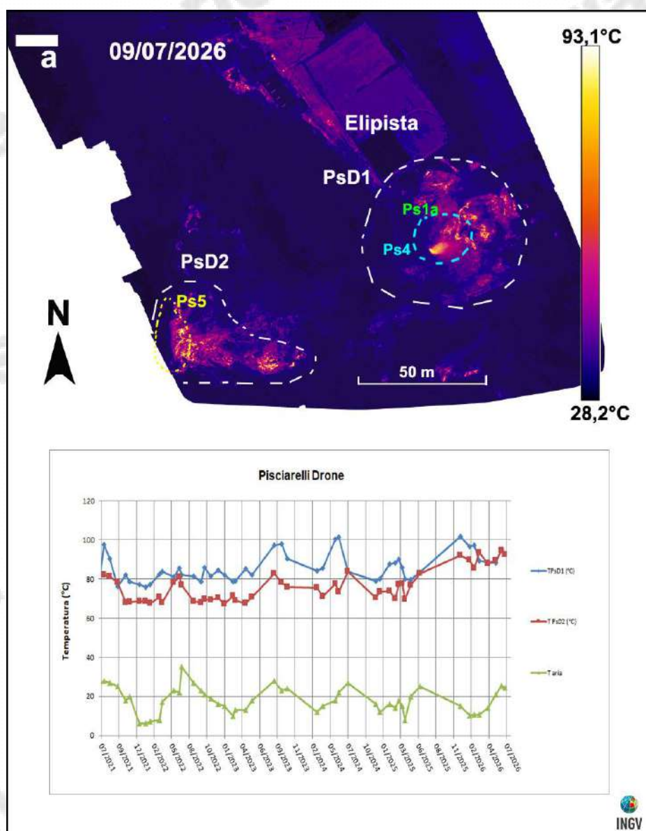
Figura 3.2.2 – Fotocomposizione di immagini termiche rilevate da drone nel mese di luglio 2026 (a) e valori massimi di temperatura ( T ) delle aree a maggiore anomalia termica (PsD1 e PsD2), confrontati con la temperatura dell'aria misurata nel momento del rilievo termico, da luglio 2021 a luglio 2026 (b).
