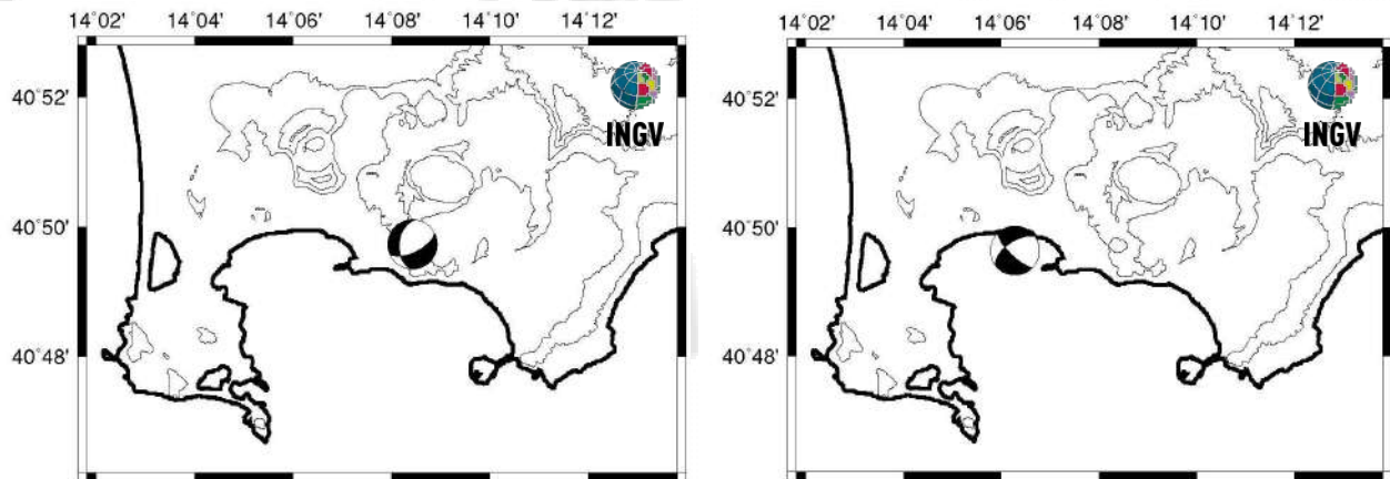
Figura 1.7 - Localizzazione epicentrale e meccanismo focale dell'evento del 31/07/2026 alle ore 17:46 UTC di M_d=4.7\pm0.3 a sinistra, e del 31/07/2026 alle ore 20:00 UTC di M_d=3.8\pm0.3 , a destra.
