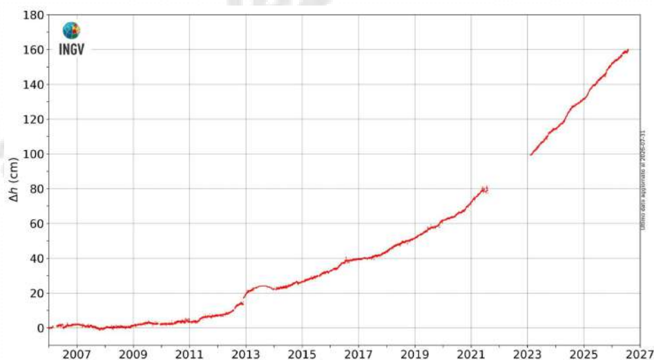
Figura 2.3.3 - Movimenti verticali del suolo nel periodo gennaio 2006 – luglio 2026, ottenuti dall'analisi dei dati acquisiti dalla stazione mareografica di Pozzuoli Porto (POPT) (area centrale della caldera Flegrea). Le variazioni, riportate in cm, rappresentano le medie giornaliere e sono riferite alla stazione mareografica di Napoli, molo San Vincenzo (NAMM).
