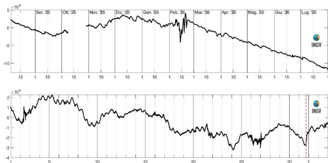
Figura 2.5.3 - In alto: Strain registrato nell'ultimo anno alla stazione di Monterusciello, dalle 00:00 UTC del 01/08/2025 alle 24:00 UTC del giorno 31/07/2026. In basso: Strain registrato nell'ultimo periodo alla stazione di Monterusciello, dalle 00:00 del 1/07/2026 alle 24:00 del 2/08/2026. La linea verticale rossa tratteggiata indica il tempo d'origine del terremoto di magnitudo M_d=4.7 .
