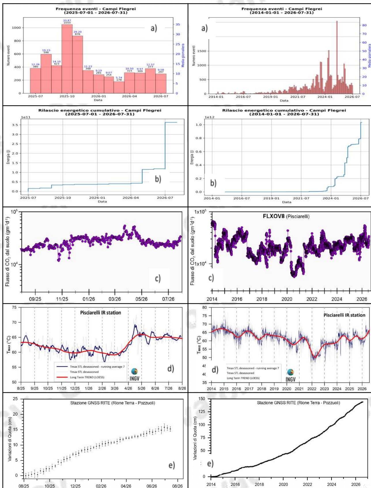
Figura 6.1 – Frequenza di accadimento degli eventi sismici (a), rilascio di energia sismica cumulativa (b), variazioni del flusso di CO 2 alla stazione geochimica di Pisciarelli (c), trend delle temperature massime superficiali destagionalizzate delle telecamera all'infrarosso termico a Pisciarelli (d) e andamento delle deformazioni del suolo alla stazione GNSS di RITE (e), negli ultimi dodici mesi (a sinistra) e dal 2014 (a destra).
