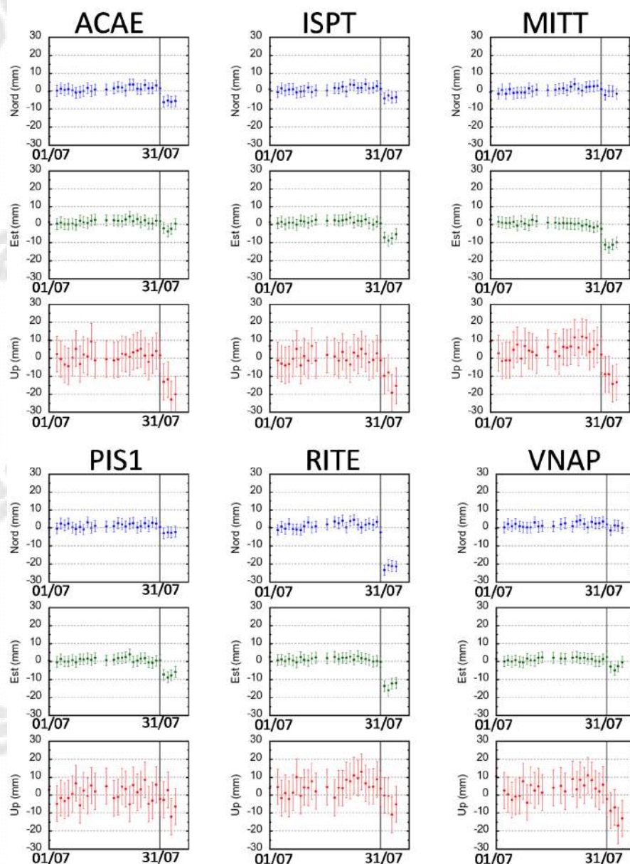
Figura 2.1.5 - Serie temporali giornaliere delle stazioni GNSS di ACAE (Accademia Aeronautica), ISPT (Istituto Petronio), MITT (Pozzuoli - Porto), PIS1 (Pisciarelli), RITE (Pozzuoli - Rione Terra), VNAP (Pozzuoli - Via Napoli), dal 01/07/2026 al 04/08/2026. Elaborazione dati con software GNSS Bernese. Le linee nere verticali indicano la data del 31 luglio.
