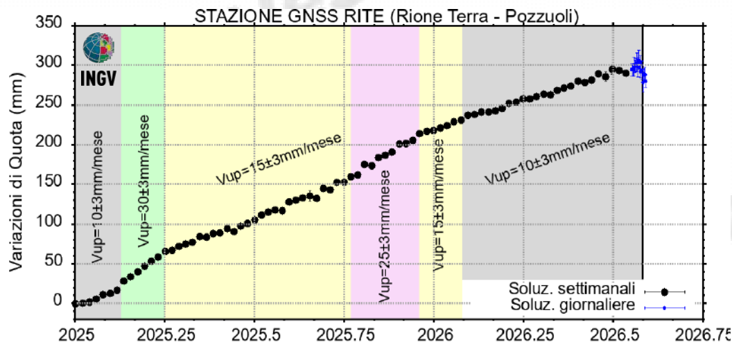
Figura 2.1.2 - Serie temporale delle variazioni in quota della stazione GNSS di RITE dal 01/01/2025 al 04/08/2026. Elaborazione dati in modalità differenziale singola baseline con software GNSS Spider. La linea nera verticale indica la data del 31 luglio.
