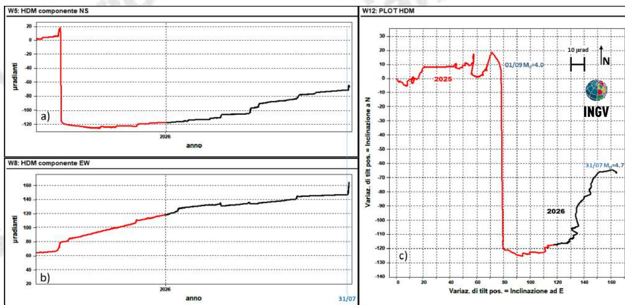
Figura 2.2.2 – Serie temporali e plot (ultimi 12 mesi) del tilt della stazione HDM della rete dei Campi Flegrei.
