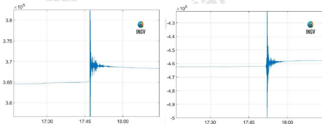
Figura 2.5.4 - Strain registrato dai dilatometri installati a Quarto, a sinistra, e Monterusciello, a destra, in concomitanza dell'evento di M_d = 4.7 avvenuto il giorno 31/07/2026.
