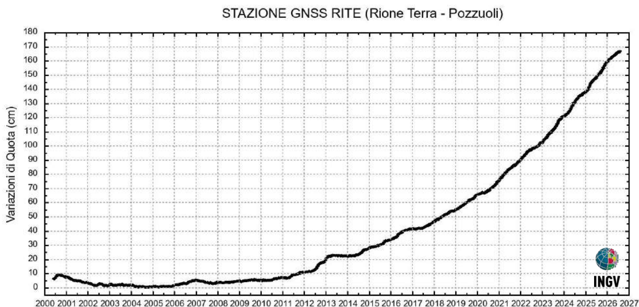
Figura 2.1.6 - Serie temporale delle variazioni settimanali in quota della stazione GNSS di RITE (Pozzuoli - Rione Terra) dal 2000 a luglio 2026.
