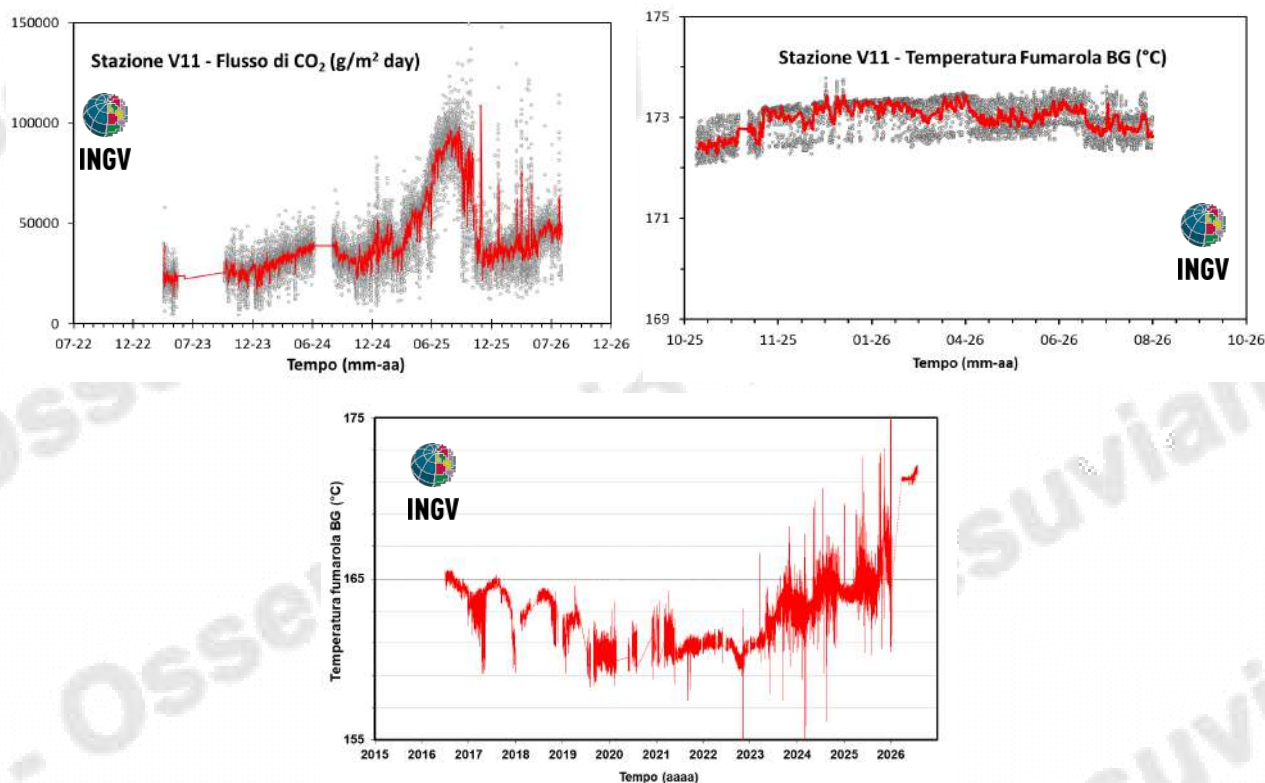
Figura 4.12 – Valori del flusso di CO 2 dal suolo e della temperatura della fumarola BG misurati dalla stazione V11 installata nel cratere della Solfatara, a pochi metri dalla fumarola principale BG.
