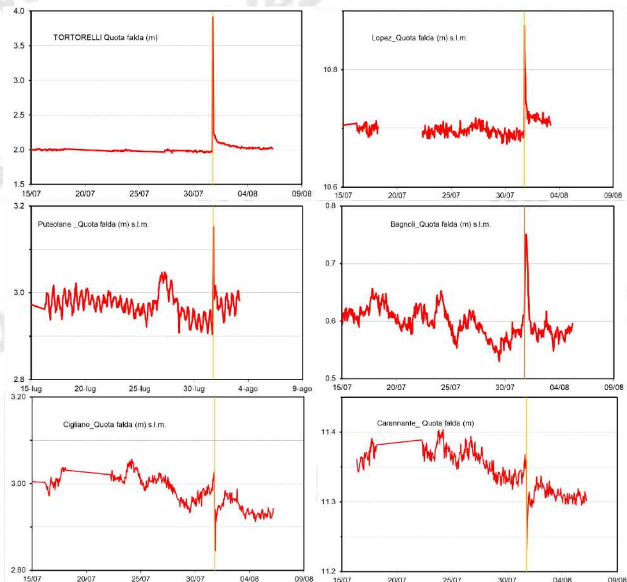
Figura 4.17 - variazione del livello di falda misurato ad alcune stazioni della rete di monitoraggio multiparametrico in continuo della falda flegrea. La linea verticale arancione marca l'evento sismico di maggiore intensità dello sciame del 31 luglio.
