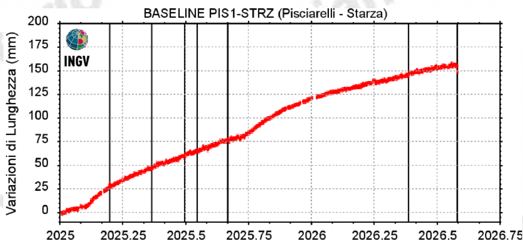
Figura 2.1.4 - Serie temporale delle variazioni di lunghezza della baseline tra le stazioni GNSS di PIS1 e STRZ dal 01/01/2025 al 02/08/2026. Elaborazione dati con software GNSS Bernese. Le linee nere verticali indicano le date di occorrenza nel periodo degli eventi sismici di M_d \geq 4.0
