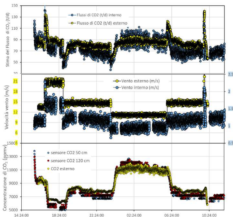
Figura 4.24 - Confronto tra i dati acquisiti dalla stazione interna e quella installata all'esterno della galleria nei 8-9 luglio durante l'aerazione forzata della galleria. I dati di concentrazione e le stime di flusso evidenziano valori simili.
