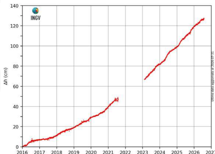
Figura 2.3.2 – Movimenti verticali del suolo, nel periodo gennaio 2016 –luglio 2026, ottenuti dall'analisi dei dati acquisiti dalla stazione mareografica di Pozzuoli Porto (POPT), area centrale della caldera Flegrea. Le variazioni, riportate in cm, rappresentano le medie giornaliere e sono riferite alla stazione mareografica di Napoli, molo San Vincenzo (NAMM).
