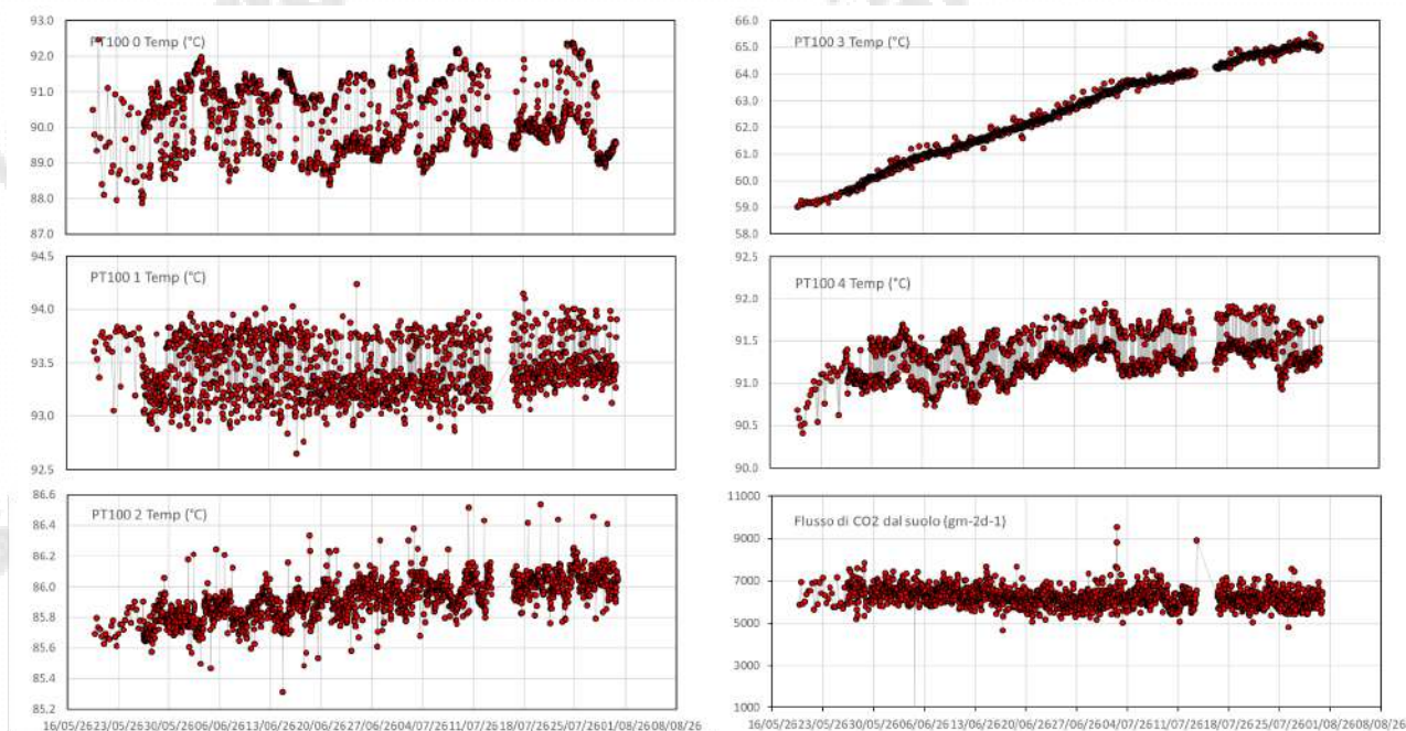
Figura 4.20 - Alcuni parametri acquisiti dalla stazione geochimica installata il 19 maggio 2026 presso l'Istituto Professionale "Lucio Petronio".
