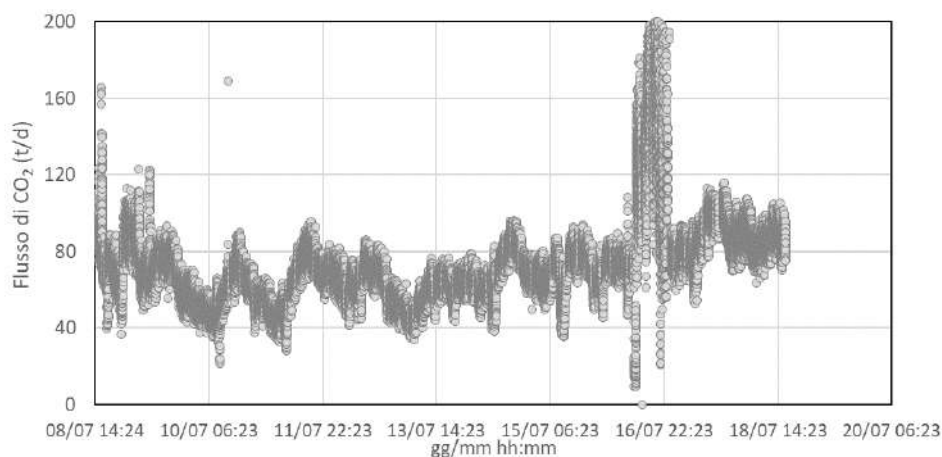
Figura 4.27 - Cronogramma dei valori di flusso di CO 2 espressi in t/d stimati per la galleria in esame durante il periodo di aerazione forzata.
