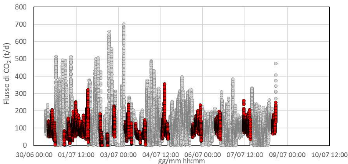
Figura 4.22 - Cronogramma dei valori di flusso di CO 2 stimati per la galleria in esame, espressi in t/d. I soli periodi indicati con i simboli rossi sono stati utilizzati per la stima del flusso medio.
