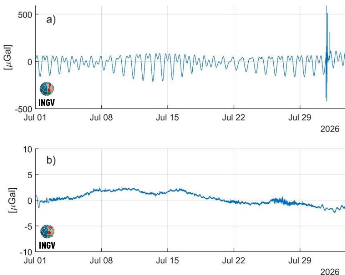
Figura 2.4.1 - a: serie temporale (risoluzione temporale 1 minuto) raw registrata dal gravimetro iGrav a Rione Terra. Si osserva il contributo dominante delle maree e dello sciame sismico a fine Luglio, con evento sismico di magnitudo max Md 4.7. b: serie residua di gravità.
