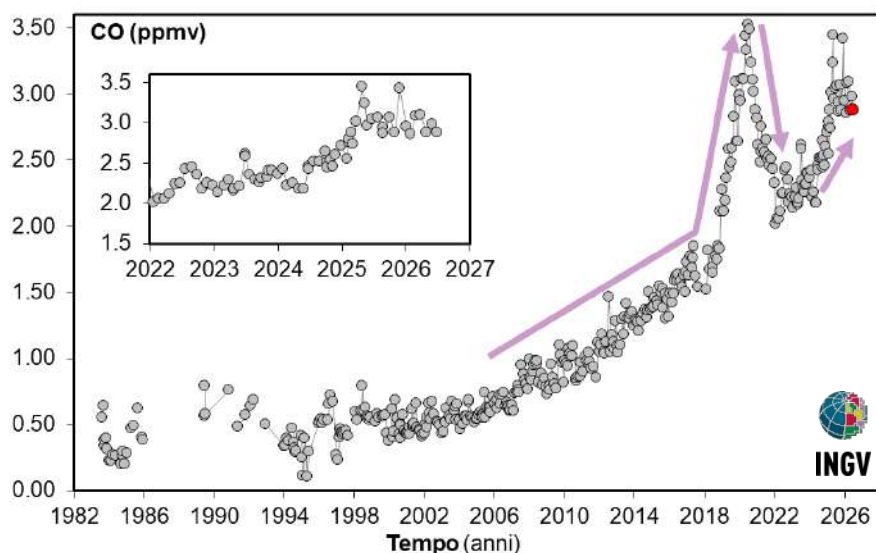
Figura 4.3 – Variazioni della concentrazione di monossido di carbonio (CO) misurato alla fumarola BG a partire dal 1983. Con il simbolo rosso è evidenziato il campione di luglio 2026. In generale alti contenuti di CO caratterizzano sistemi vulcanici a elevata temperatura, mentre fumarole alimentate da sistemi idrotermali mostrano concentrazioni più basse, in tali sistemi un aumento delle concentrazioni di CO può riflettere un incremento delle condizioni di pressione e temperatura. Nel riquadro un dettaglio dal 2022.
