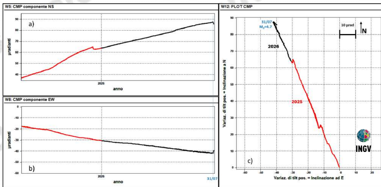
Figura 2.2.4 – Serie temporali e plot (ultimi 12 mesi) del tilt della stazione CMP della rete dei Campi Flegrei.
