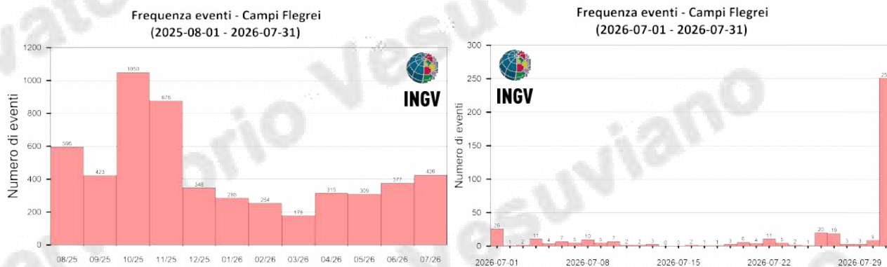
Figura 1.2 - A sinistra numero di eventi registrati ai Campi Flegrei nel corso degli ultimi 12 mesi (in totale 5437), mentre a destra quelli avvenuti nell'ultimo mese (in totale 426).
