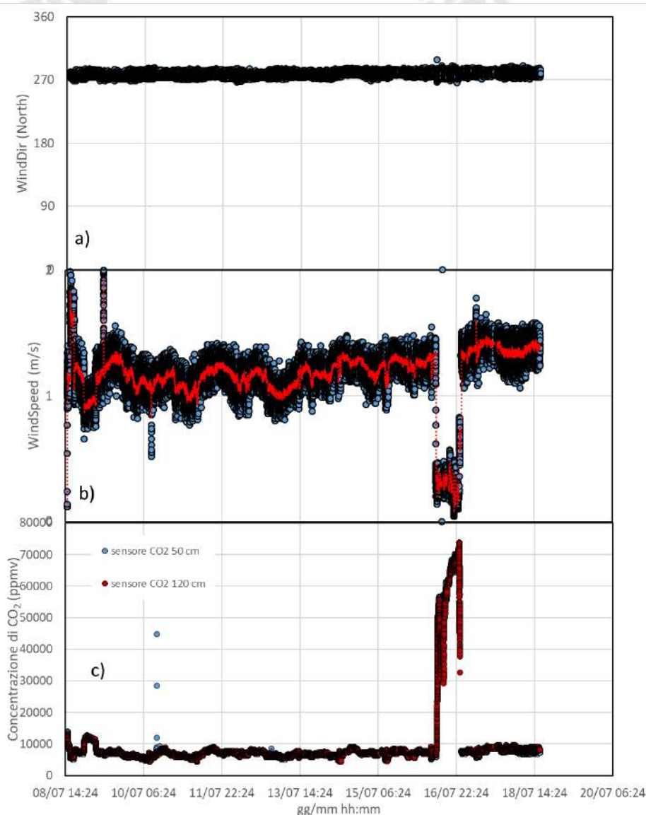
Figura 4.26 - Dati acquisiti dalla stazione installata nella galleria della Linea 2 della Metropolitana di Napoli, tratta Pozzuoli Solfatara - Napoli Campi Flegrei, nel periodo di aerazione forzata operato con due turbine dal 8 luglio al 18 luglio 2026: a) direzione del vento in gradi da Nord in senso orario; b) intensità del vento in m/s; c) concentrazione di CO 2 in aria, espressa in ppmv, a tre differenti quote dal suolo (50 cm, 120 cm).
