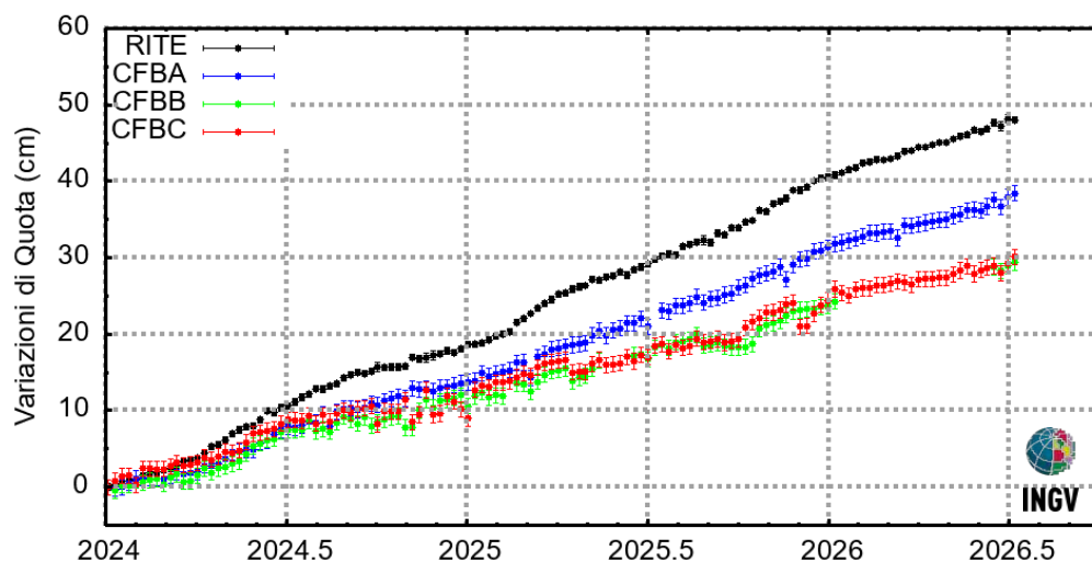
Figura 2.1.8 – Serie temporali delle variazioni settimanali in quota delle stazioni GNSS dell'infrastruttura marina MEDUSA nell'intervallo gennaio 2024 - luglio 2026, confrontate con quella della stazione RITE
