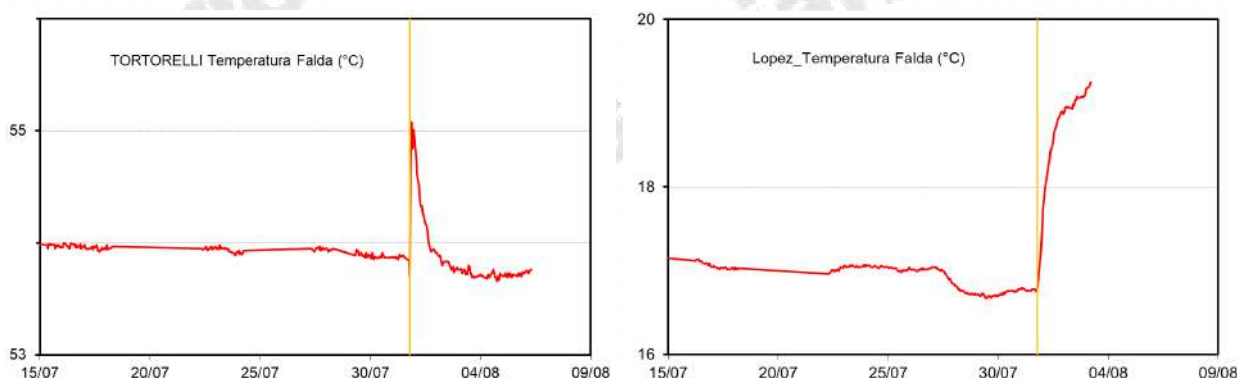
Figura 4.18 - variazione della temperatura della falda misurata alle stazioni Tortorelli e Lopez della rete di monitoraggio multiparametrico in continuo della falda flegrea. La linea verticale arancione marca l'evento sismico di maggiore intensità dello sciame del 31 luglio.
