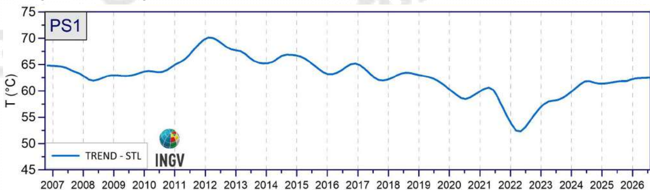
Figura 3.1.4 - Stazione PS1: Trend a lungo termine dei valori di temperatura massima rilevati nelle immagini IR ottenuti mediante applicazione dell'algoritmo STL.
