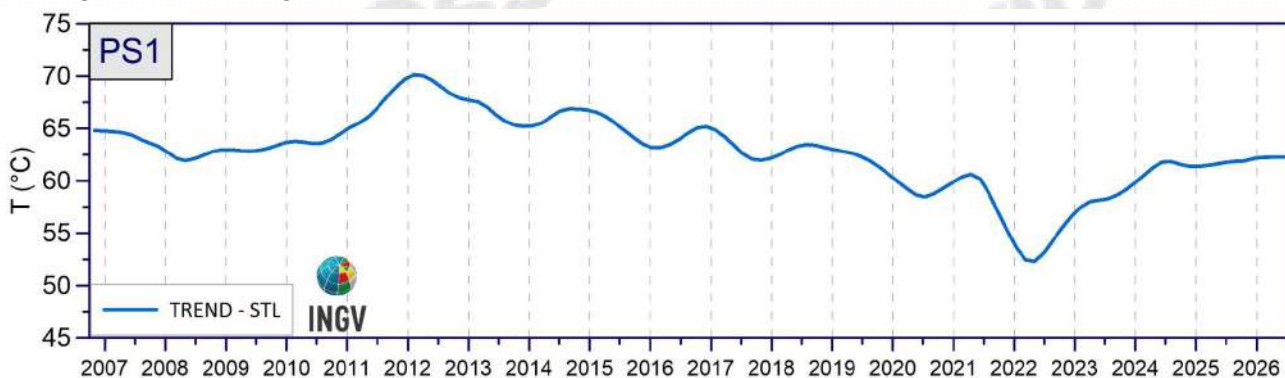
Figura 3.1.4 - Stazione PS1: Trend a lungo termine dei valori di temperatura massima rilevati nelle immagini IR ottenuti mediante applicazione dell'algoritmo STL.
