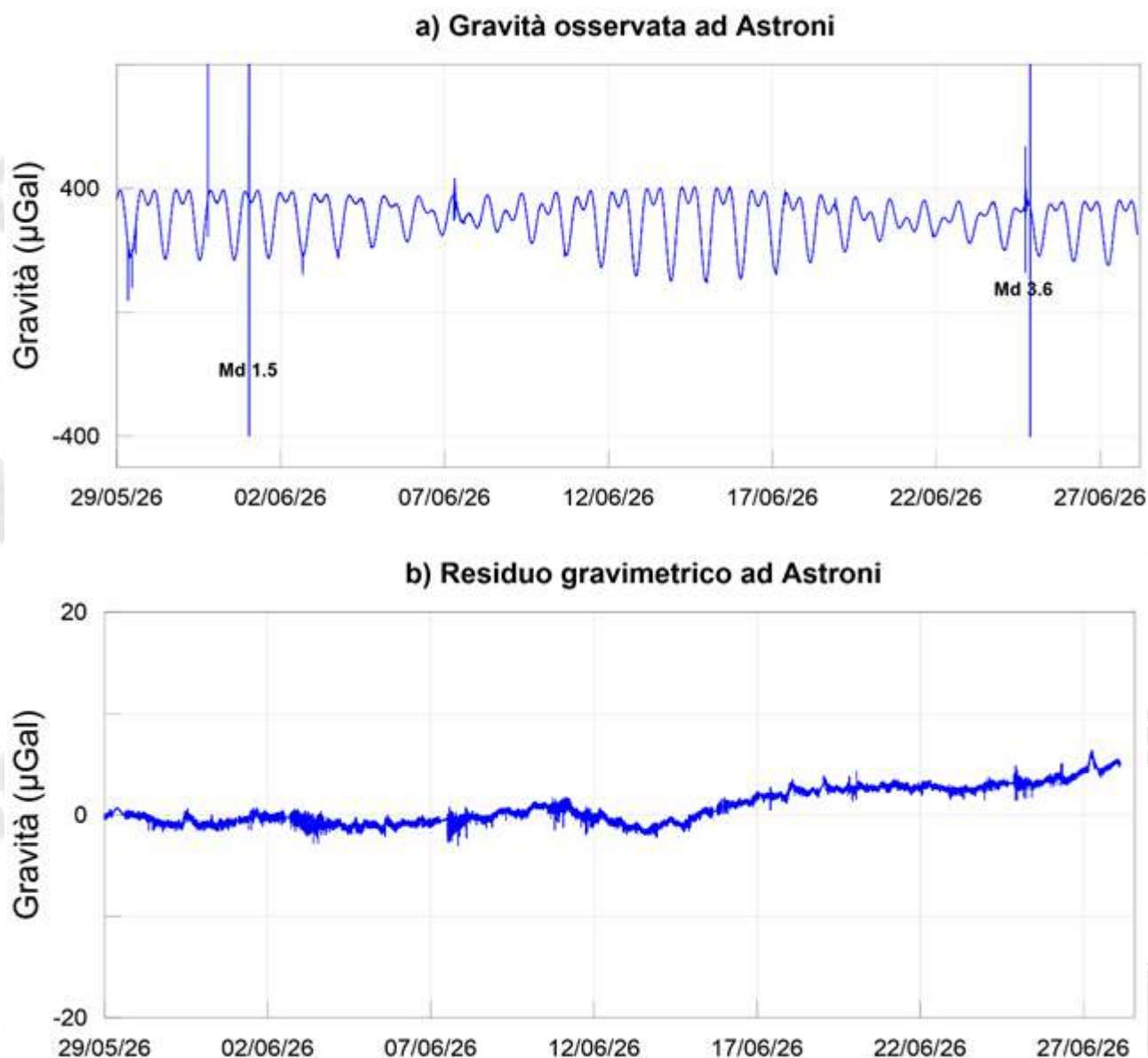
Figura 2.4.1 - a: serie temporale (risoluzione temporale 1 minuto) raw registrata dal gPhone. Si osserva il contributo dominante delle maree. b: serie residua di gravità.
