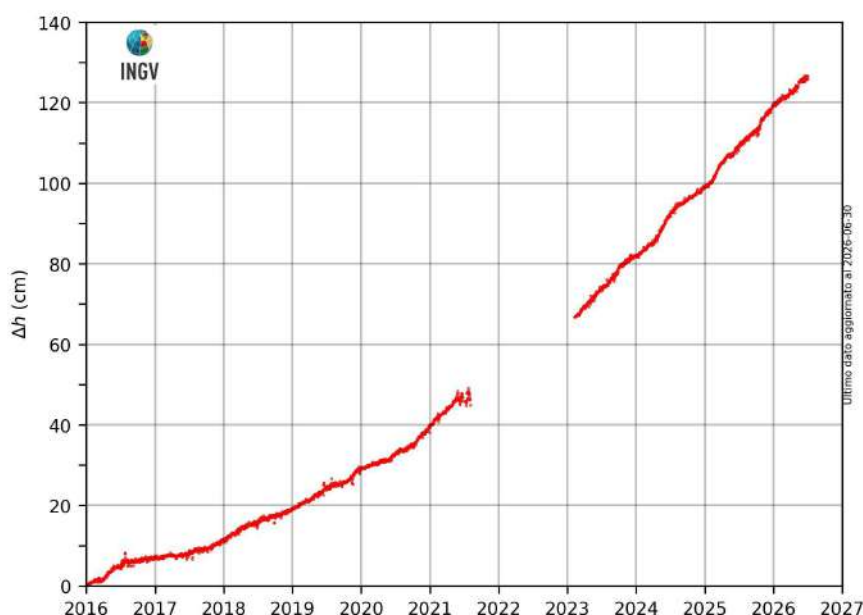
Figura 2.3.2 – Movimenti verticali del suolo, nel periodo gennaio 2016 – giugno 2026, ottenuti dall'analisi dei dati acquisiti dalla stazione mareografica di Pozzuoli Porto (POPT), area centrale della caldera Flegrea. Le variazioni, riportate in cm, rappresentano le medie giornaliere e sono riferite alla stazione mareografica di Napoli, molo San Vincenzo (NAMM).
