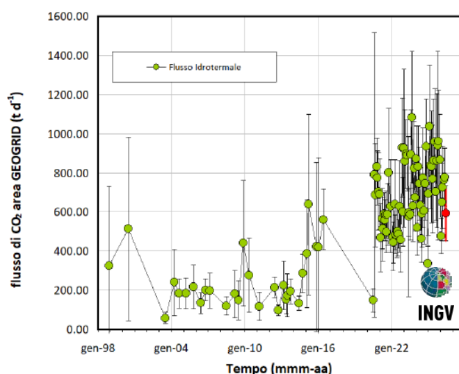
Figura 5.1.2 - Cronogramma dell'output di CO 2 diffuso dal suolo stimato per l'area di interesse. Le misure eseguite ad agosto 2020 hanno mostrato un valore tra i più bassi misurati, mentre quelle successive mostrano un aumento medio dei valori, con ~600 tonnellate di CO 2 al giorno per le misure di giugno 2026 (simbolo rosso). Le barre verticali rappresentano l'intervallo di confidenza del 95%.
