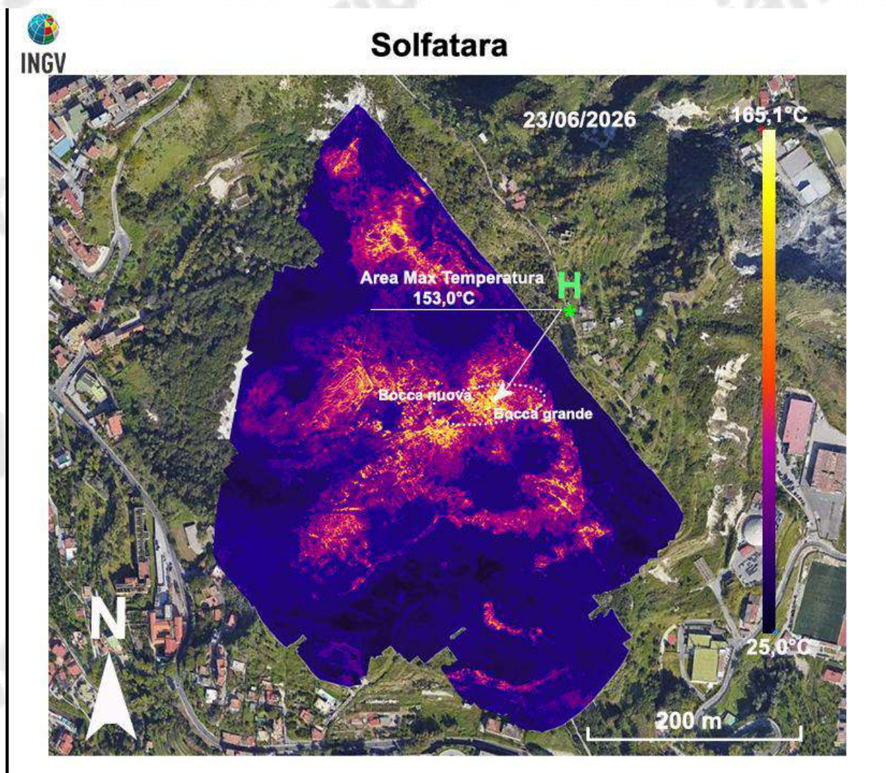
Figura 3.2.4 – Fotocomposizione di immagini termiche rilevate da drone nel mese di giugno 2026 su La Solfatara (Solf in figura 3.2.1.B). H* indica il sito di decollo e di atterraggio del drone corrispondente al punto S1 di Fig.3.2.1.B.
