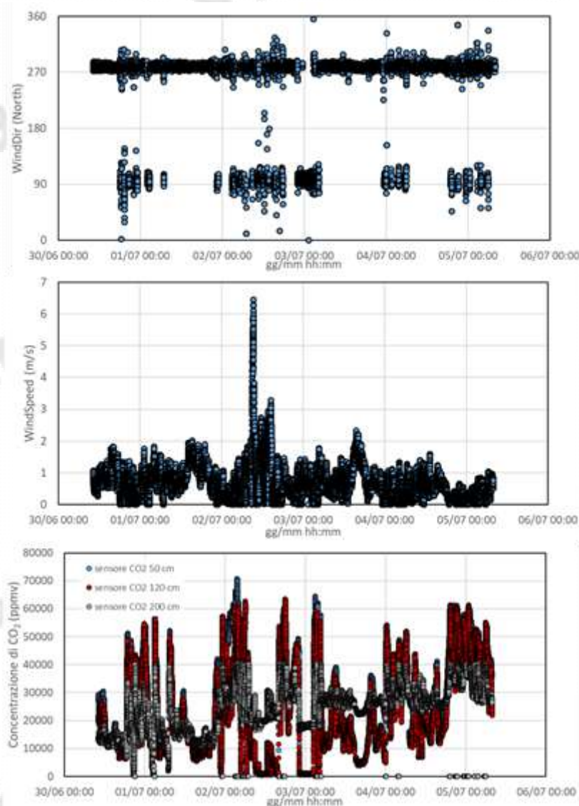
Figura 4.19 - Dati acquisiti dalla stazione installata nella galleria della Linea 2 della Metropolitana di Napoli, tratta Pozzuoli Solfatara - Napoli Campi Flegrei, nel periodo 30 giugno - 5 luglio 2026: a) direzione del vento in gradi da Nord in senso orario; b) intensità del vento in m/s; c) concentrazione di CO 2 in aria, espressa in ppmv, a tre differenti quote dal suolo (50 cm, 120 cm e 200 cm). Nel periodo considerato sono state misurate concentrazioni fino a circa il 7% in volume, corrispondenti a circa 70.000 ppmv.
