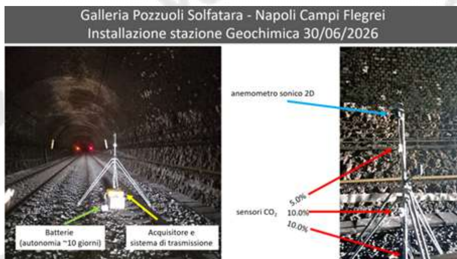
Figura 4.18 - Stazione geochimica installata il 30 giugno 2026 a circa 50 m dall'ingresso lato Bagnoli della galleria della Linea 2 della Metropolitana di Napoli, tratta Pozzuoli Solfatara - Napoli Campi Flegrei. La stazione misura la concentrazione di CO 2 in aria a tre differenti altezze dal suolo mediante sensori NDIR e la direzione e velocità del vento mediante anemometro sonico.
