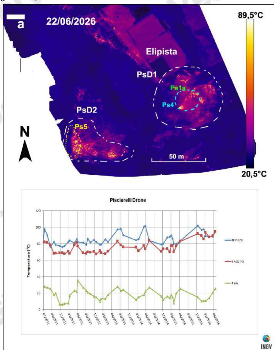
Figura 3.2.2 – Fotocomposizione di immagini termiche rilevate da drone nel mese di maggio 2026 (a) e valori massimi di temperatura (T) delle aree a maggiore anomalia termica (PsD1 e PsD2), confrontati con la temperatura dell'aria misurata nel momento del rilievo termico, da luglio 2021 a giugno 2026 (b).
