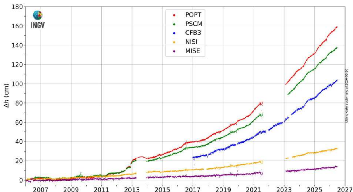
Figura 2.3.4 - Movimenti verticali del suolo nel periodo gennaio 2006 – giugno 2026, ottenuti dall'analisi dei dati acquisiti da tutte le stazioni mareografiche dell'area della caldera Flegrea. Le variazioni, riportate in cm, rappresentano le medie giornaliere e sono tutte riferite alla stazione mareografica di Napoli, molo San Vincenzo (NAMM).
