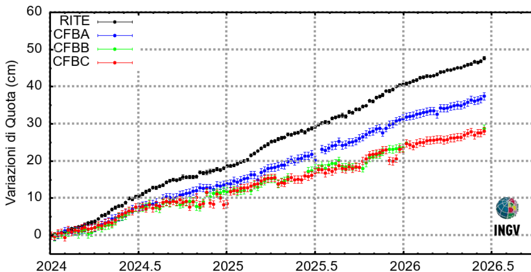
Figura 2.1.6 – Serie temporali delle variazioni settimanali in quota delle stazioni GNSS dell'infrastruttura marina MEDUSA nell'intervallo gennaio 2024 - giugno 2026, confrontate con quella della stazione RITE
