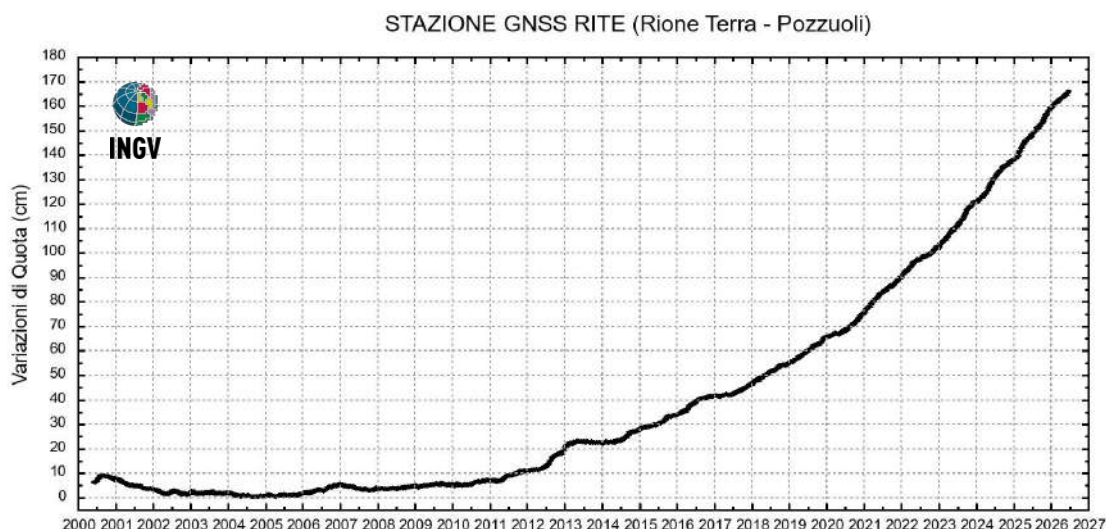
Figura 2.1.4 - Serie temporale delle variazioni settimanali in quota della stazione di RITE (Pozzuoli – Rione Terra) dal 2000 a giugno 2026.
