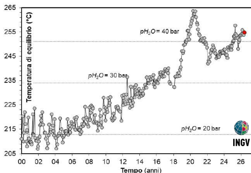
Figura 4.4 – Cronogramma delle temperature di equilibrio per il sistema CO-CO 2 , relativo alla fumarola BG, stimate assumendo condizioni redox fissate dalla relazione di D'Amore and Panichi (1980). Tali temperature, rappresentative della parte più superficiale del sistema idrotermale (Caliro et al., 2007), mostrano un trend in aumento a partire dai primi anni del 2000. Con il simbolo rosso è evidenziato il campione di giugno 2026.
