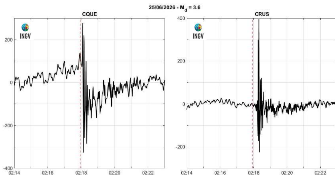
Figura 2.5.4 - Strain registrato dai dilatometri installati a Quarto e Monterusciello in concomitanza dell'evento di M_d = 3.6 avvenuto il giorno 25/06/2026.
