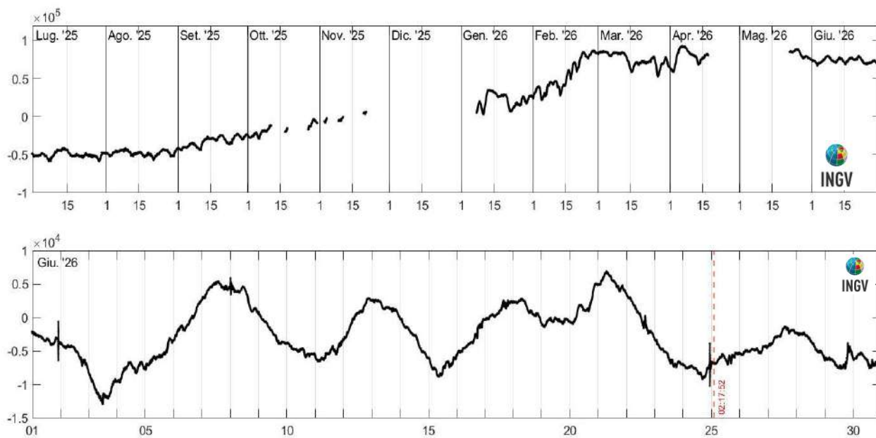
Figura 2.5.2 - Strain registrato dalla stazione dilatometrica di Quarto. In alto è mostrato lo strain registrato nell'ultimo anno, dalle 00:00 UTC del 1/07/2025 alle 24:00 UTC del 30/06/2026. In basso, i dati di strain disponibili nell'ultimo periodo, dalle 00:00 UTC del 01/06/2026 alle 24:00 UTC del 30/06/2026.
