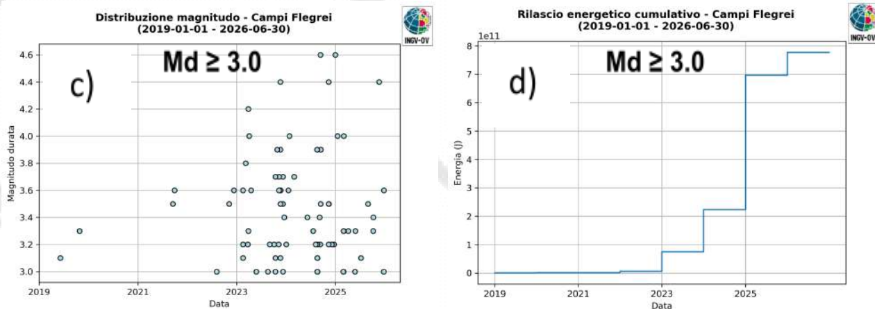
Figura 1.9 - Localizzazioni e andamento dei principali parametri sismologici dei terremoti con M_d \geq 3.0 a partire dal 2019: a) frequenza di accadimento; b) profondità ipocentrali; c) magnitudo; d) energia cumulativa.
