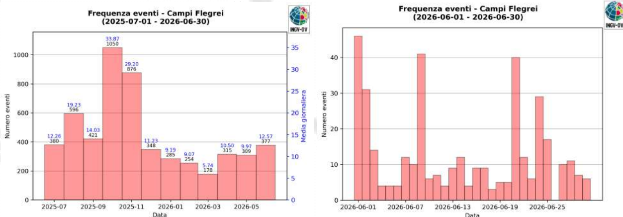
Figura 1.2 - A sinistra numero di eventi registrati ai Campi Flegrei nel corso degli ultimi 12 mesi (in totale 5389), mentre a destra quelli avvenuti nell'ultimo mese (in totale 377).
