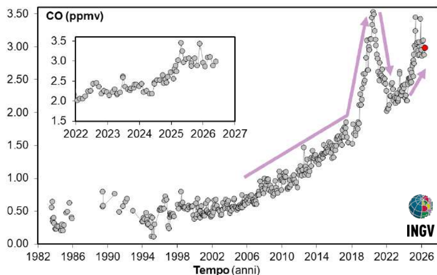
Figura 4.3 – Variazioni della concentrazione di monossido di carbonio (CO) misurato alla fumarola BG a partire dal 1983. Con il simbolo rosso è evidenziato il campione di giugno 2026. In generale alti contenuti di CO caratterizzano sistemi vulcanici a elevata temperatura, mentre fumarole alimentate da sistemi idrotermali mostrano concentrazioni più basse, in tali sistemi un aumento delle concentrazioni di CO può riflettere un incremento delle condizioni di pressione e temperatura. Nel riquadro un dettaglio dal 2022.
