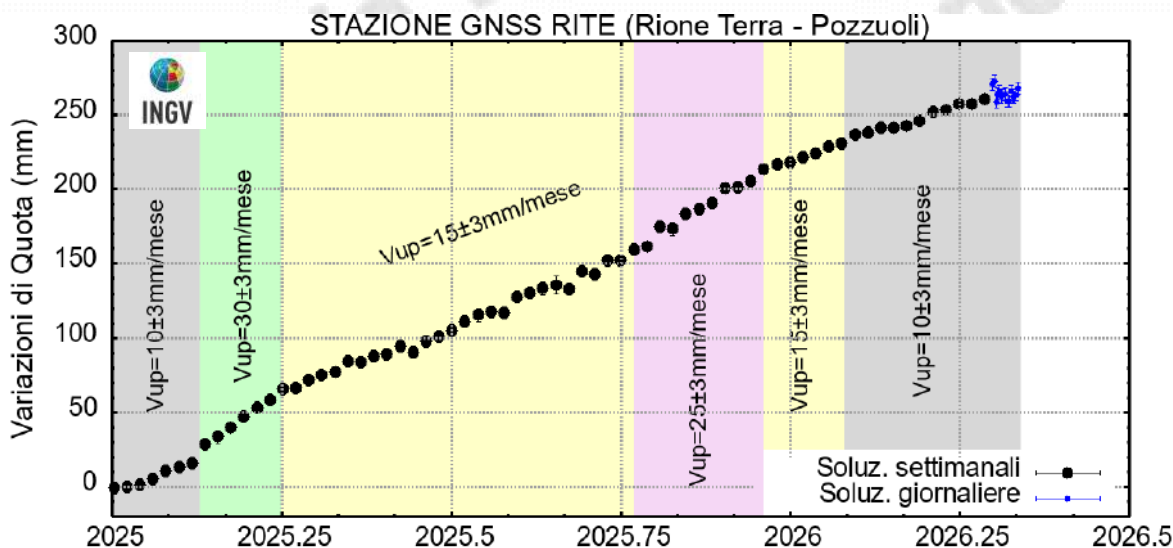
Figura 2.1.2 - Serie temporale delle variazioni in quota della stazione GNSS di RITE dal 01/01/2025 al 03/05/2026. Elaborazione dati in modalità differenziale singola baseline con software GNSS Spider.
