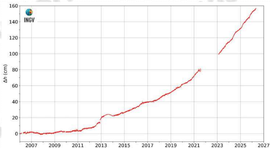
Figura 2.3.3 - Movimenti verticali del suolo nel periodo gennaio 2006 – aprile 2026, ottenuti dall'analisi dei dati acquisiti dalla stazione mareografica di Pozzuoli Porto (POPT) (area centrale della caldera Flegrea). Le variazioni, riportate in cm, rappresentano le medie giornaliere e sono riferite alla stazione mareografica di Napoli, molo San Vincenzo (NAMM).
