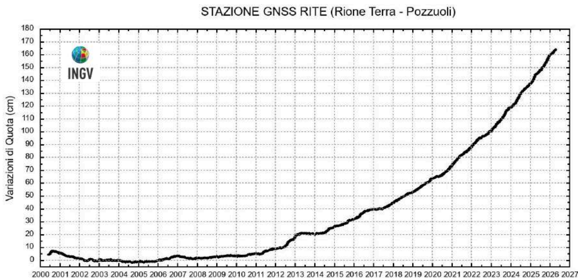
Figura 2.1.4 - Serie temporale delle variazioni settimanali in quota della stazione di RITE (Pozzuoli – Rione Terra) dal 2000 ad aprile 2026.
