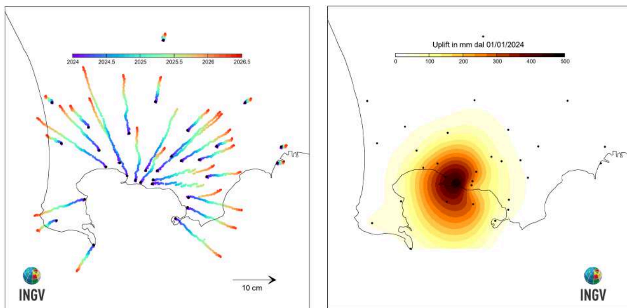
Figura 2.1.5 - Mappa degli spostamenti GNSS orizzontali (a) e verticali (b) registrati nell'area flegrea da gennaio 2024 ad aprile 2026.
