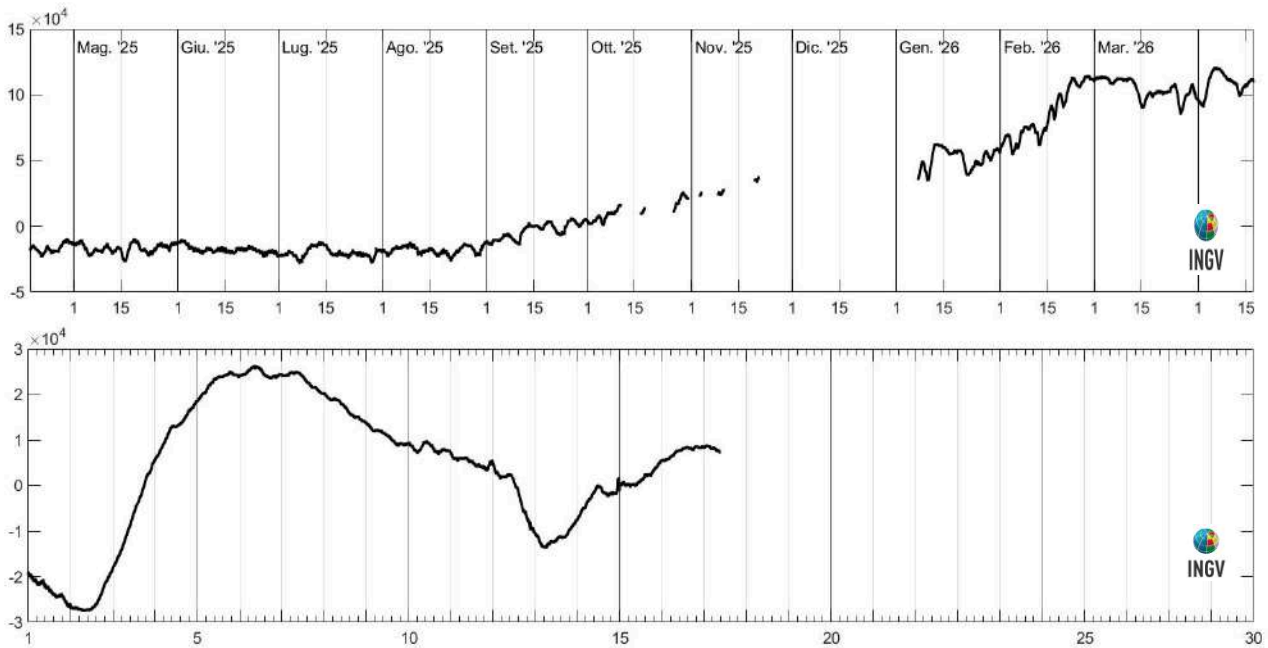
Figura 2.5.2 - Strain registrato dalla stazione dilatometrica di Quarto. In alto è mostrato lo strain registrato nell'ultimo anno, dalle 00:00 UTC del 1/05/2025 alle 9:00 UTC del 17/04/2026. In basso, i dati di strain disponibili nell'ultimo periodo, dalle 00:00 UTC del 1/04/2026 alle 9:00 UTC del 17/04/2026.
