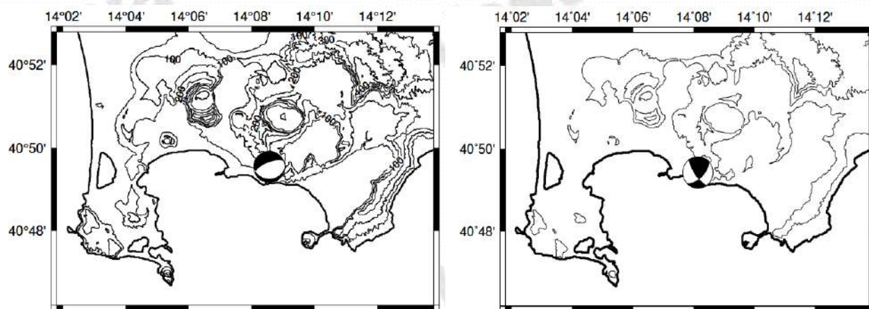
Figura 1.7 - Localizzazioni ipocentrali e meccanismi focali dell'evento del 07/04/2026 alle ore 02:32 UTC di M_d 3.3 \pm 0.3 (a sinistra) e dell'evento del 08/04/2026 alle ore 14:48 UTC di M_d 3.4 \pm 0.3
