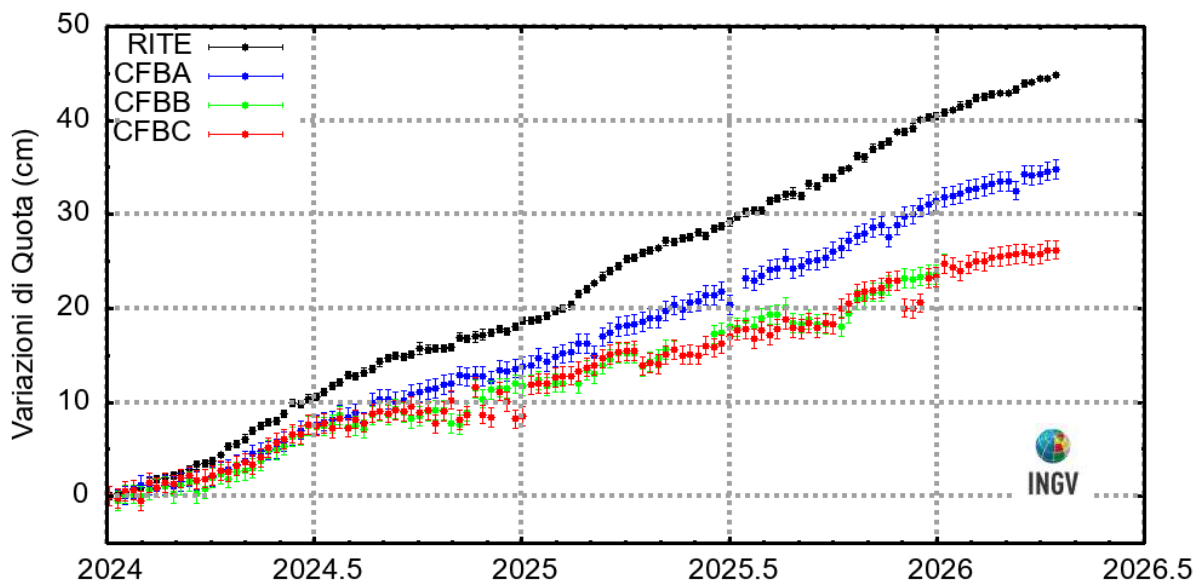
Figura 2.1.6 – Serie temporali delle variazioni settimanali in quota delle stazioni GNSS dell'infrastruttura marina MEDUSA nell'intervallo gennaio 2024 - aprile 2026, confrontate con quella della stazione RITE
