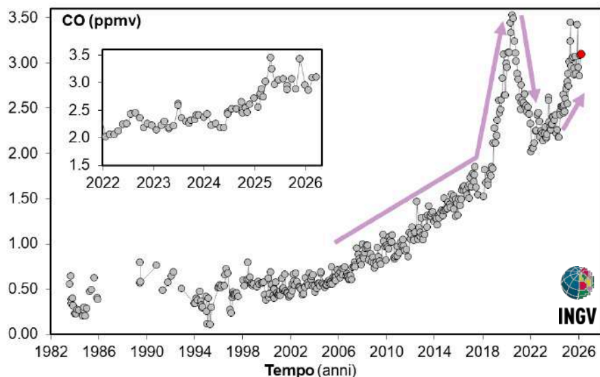
Figura 4.3 – Variazioni della concentrazione di monossido di carbonio (CO) misurato alla fumarola BG a partire dal 1983. Con il simbolo rosso è evidenziato il campione di aprile 2026. In generale alti contenuti di CO caratterizzano sistemi vulcanici a elevata temperatura, mentre fumarole alimentate da sistemi idrotermali mostrano concentrazioni più basse, in tali sistemi un aumento delle concentrazioni di CO può riflettere un incremento delle condizioni di pressione e temperatura. Nel riquadro un dettaglio dal 2022.
