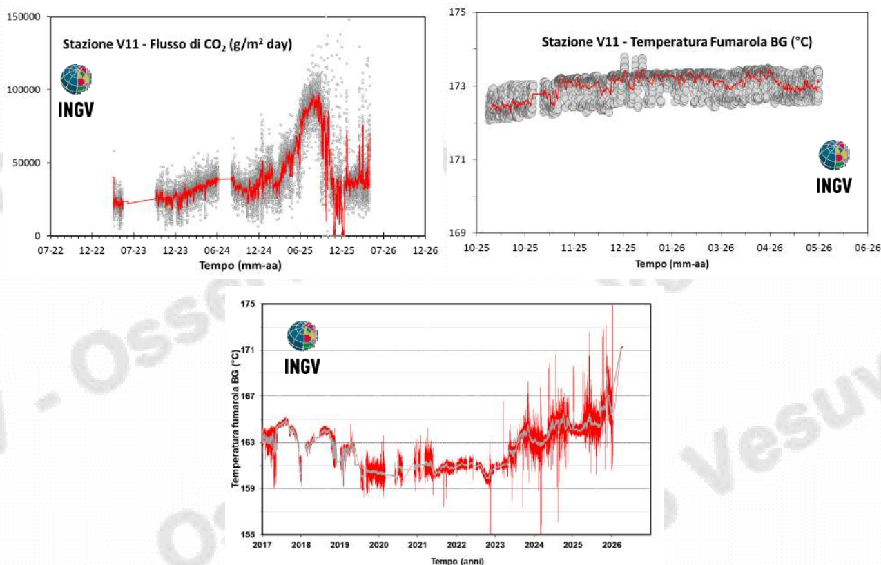
Figura 4.12 – Valori del flusso di \text{CO}_2 dal suolo e della temperatura della fumarola BG misurati dalla stazione V11 installata nel cratere della Solfatara, a pochi metri dalla fumarola principale BG.
