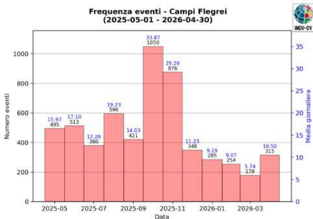
Figura 1.2 - A sinistra numero di eventi registrati ai Campi Flegrei nel corso degli ultimi 12 mesi (in totale 5711), mentre a destra quelli avvenuti nell'ultimo mese (in totale 315).
