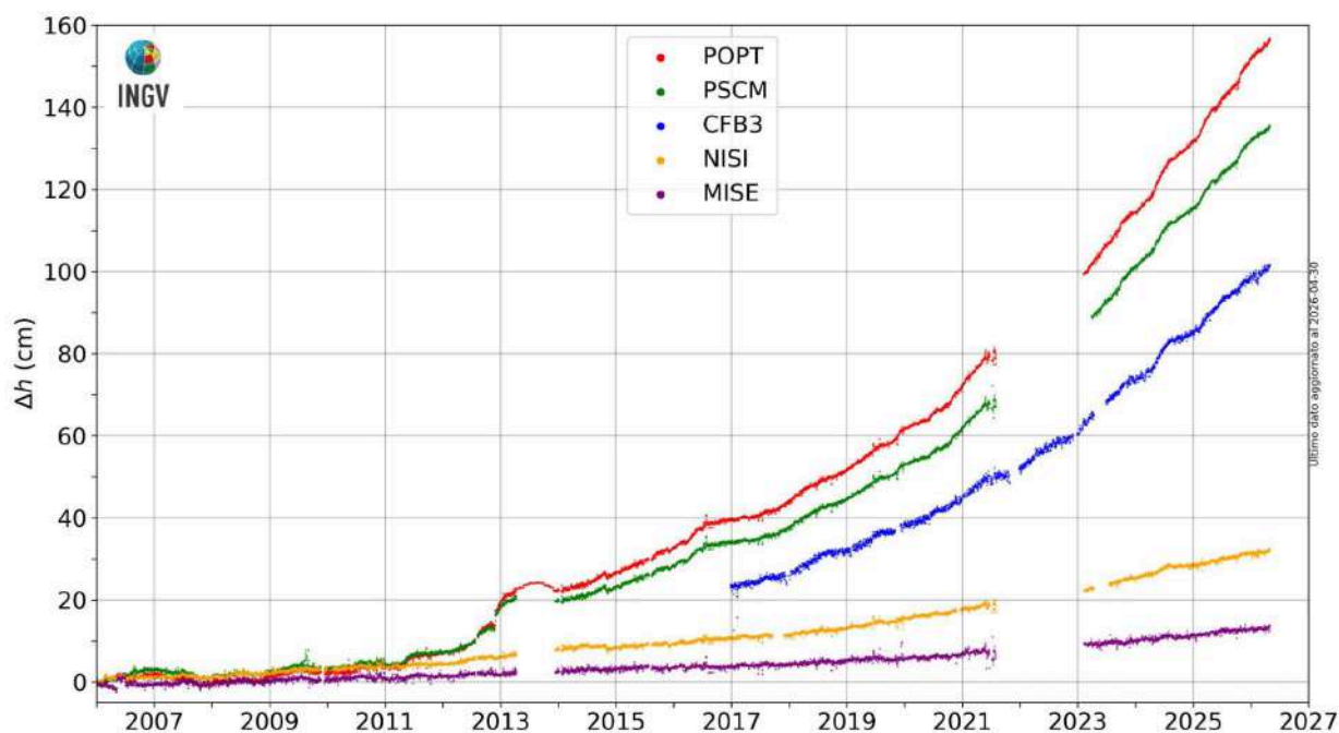
Figura 2.3.4 - Movimenti verticali del suolo nel periodo gennaio 2006 – aprile 2026, ottenuti dall'analisi dei dati acquisiti da tutte le stazioni mareografiche dell'area della caldera Flegrea. Le variazioni, riportate in cm, rappresentano le medie giornaliere e sono tutte riferite alla stazione mareografica di Napoli, molo San Vincenzo (NAMM).
