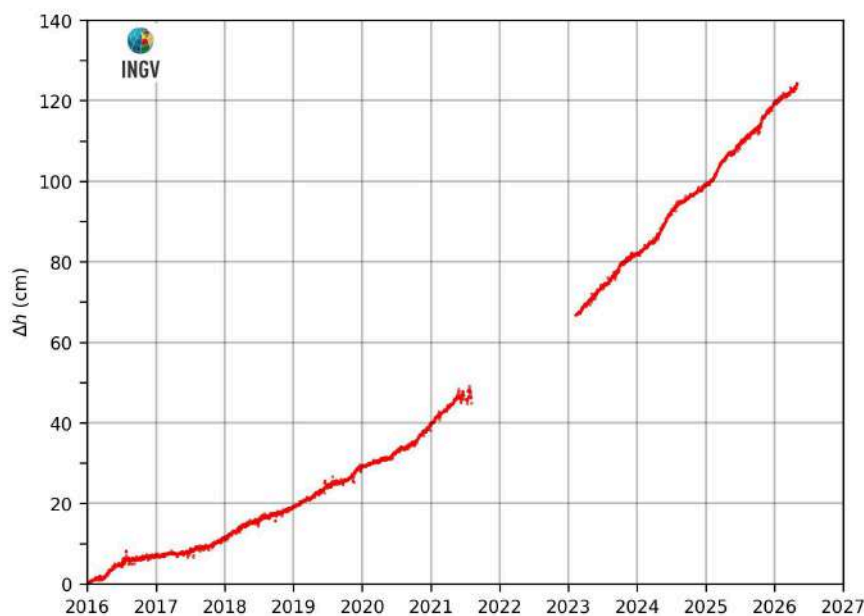
Figura 2.3.2 – Movimenti verticali del suolo, nel periodo gennaio 2016 – aprile 2026, ottenuti dall'analisi dei dati acquisiti dalla stazione mareografica di Pozzuoli Porto (POPT), area centrale della caldera Flegrea. Le variazioni, riportate in cm, rappresentano le medie giornaliere e sono riferite alla stazione mareografica di Napoli, molo San Vincenzo (NAMM).
