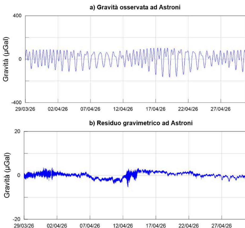
Figura 2.4.1 - a) serie temporale raw (risoluzione temporale 1 minuto) registrata dal gPhone. Si osserva il contributo dominante delle maree. b) serie residua di gravità con variazioni nell'ordine di \pm 3 \mu\text{Gal} .
