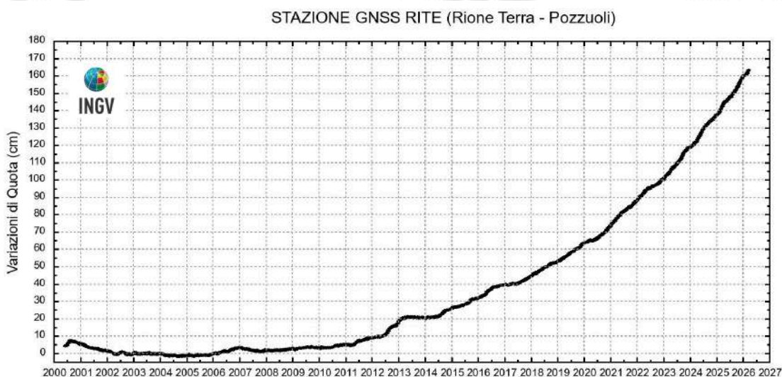
Figura 2.1.4 - Serie temporale delle variazioni settimanali in quota della stazione di RITE (Pozzuoli - Rione Terra) dal 2000 a marzo 2026.
