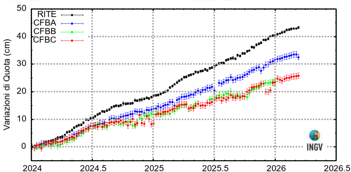
Figura 2.1.6 – Serie temporali delle variazioni settimanali in quota delle stazioni GNSS dell'infrastruttura marina MEDUSA nell'intervallo gennaio 2024 - marzo 2026, confrontate con quella della stazione RITE
