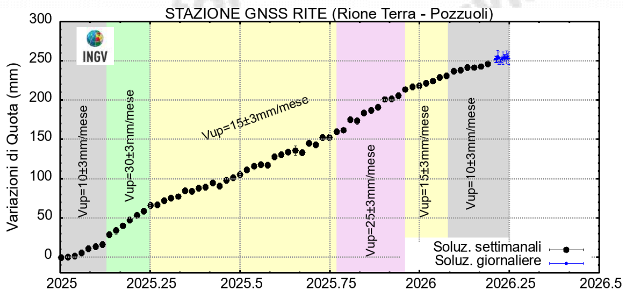
Figura 2.1.2 - Serie temporale delle variazioni in quota della stazione GNSS di RITE dal 01/01/2025 al 01/04/2026. Elaborazione dati in modalità differenziale singola baseline con software GNSS Spider.
