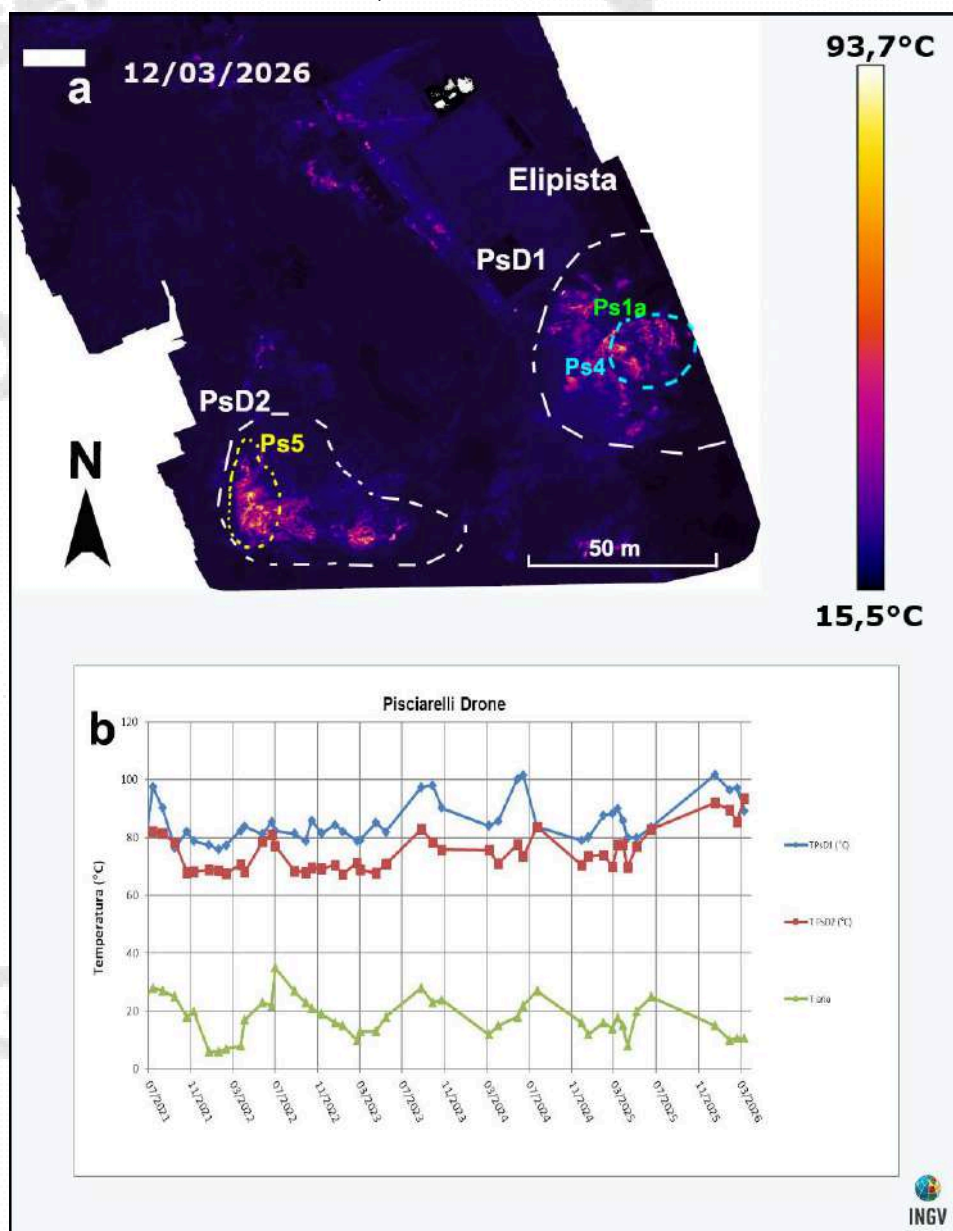
Figura 3.2.2 – Fotocomposizione di immagini termiche rilevate da drone nel mese di marzo 2026 (a) e valori massimi di temperatura ( T ) delle aree a maggiore anomalia termica (PsD1 e PsD2), confrontati con la temperatura dell'aria misurata nel momento del rilievo termico, da luglio 2021 a marzo 2026 (b).
