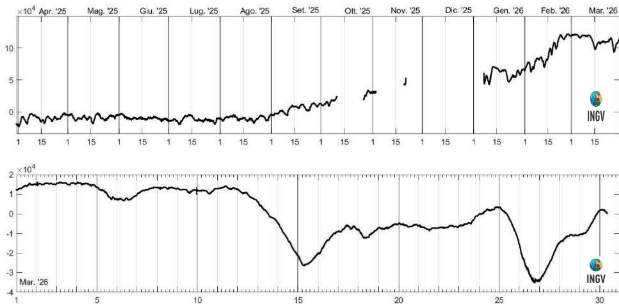
Figura 2.5.2 - Strain registrato dalla stazione dilatometrica di Quarto. In alto è mostrato lo strain registrato nell'ultimo anno, dalle 00:00 UTC del 1/04/2025 alle 10:00 UTC del 30/03/2026. In basso, i dati di strain disponibili nell'ultimo periodo, dalle 00:00 UTC del 1/03/2026 alle 10:00 UTC del 30/03/2026.
