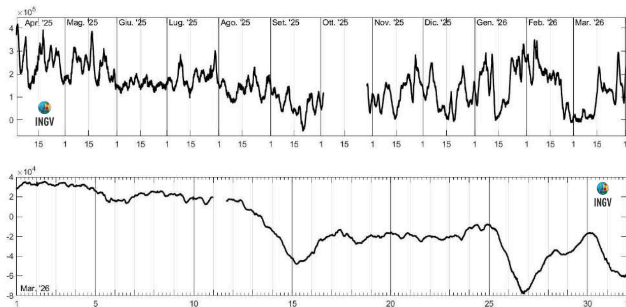
Figura 2.5.3 - In alto: Strain registrato nell'ultimo anno alla stazione di Monterusciello, dalle 00:00 UTC del 01/04/2025 alle 24:00 UTC del giorno 31/03/2026. In basso: Strain registrato nell'ultima settimana alla stazione di Monterusciello, dalle 00:00 del 1/03/2026 alle 24:00 del 31/03/2026.
