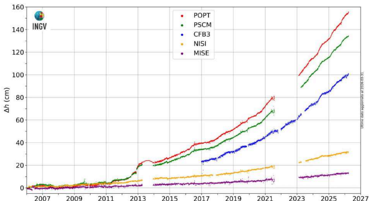
Figura 2.3.4 - Movimenti verticali del suolo nel periodo gennaio 2006 – marzo 2026, ottenuti dall'analisi dei dati acquisiti da tutte le stazioni mareografiche dell'area della caldera Flegrea. Le variazioni, riportate in cm, rappresentano le medie giornaliere e sono tutte riferite alla stazione mareografica di Napoli, molo San Vincenzo (NAMM).
