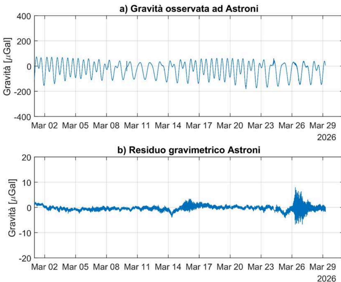
Figura 2.4.5 - a) serie temporale raw (risoluzione temporale 1 minuto) registrata dal gPhone. Si osserva il contributo dominante delle maree. b) serie residua di gravità con variazioni massime dell'ordine di \pm 5 \mu\text{Gal} .
