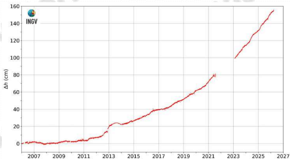
Figura 2.3.3 - Movimenti verticali del suolo nel periodo gennaio 2006 – marzo 2026, ottenuti dall'analisi dei dati acquisiti dalla stazione mareografica di Pozzuoli Porto (POPT) (area centrale della caldera Flegrea). Le variazioni, riportate in cm, rappresentano le medie giornaliere e sono riferite alla stazione mareografica di Napoli, molo San Vincenzo (NAMM).
