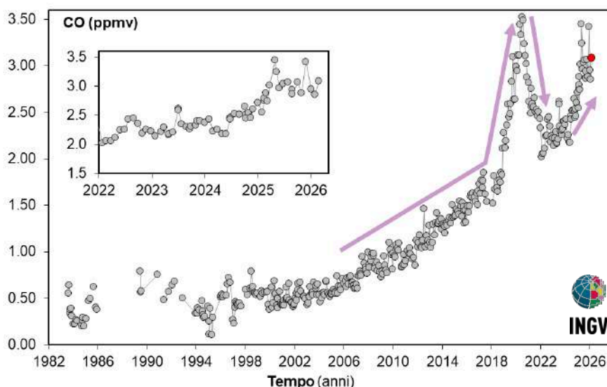
Figura 4.3 – Variazioni della concentrazione di monossido di carbonio (CO) misurato alla fumarola BG a partire dal 1983. Con il simbolo rosso è evidenziato il campione di marzo 2026. In generale alti contenuti di CO caratterizzano sistemi vulcanici a elevata temperatura, mentre fumarole alimentate da sistemi idrotermali mostrano concentrazioni più basse, in tali sistemi un aumento delle concentrazioni di CO può riflettere un incremento delle condizioni di pressione e temperatura. Nel riquadro un dettaglio dal 2022.
