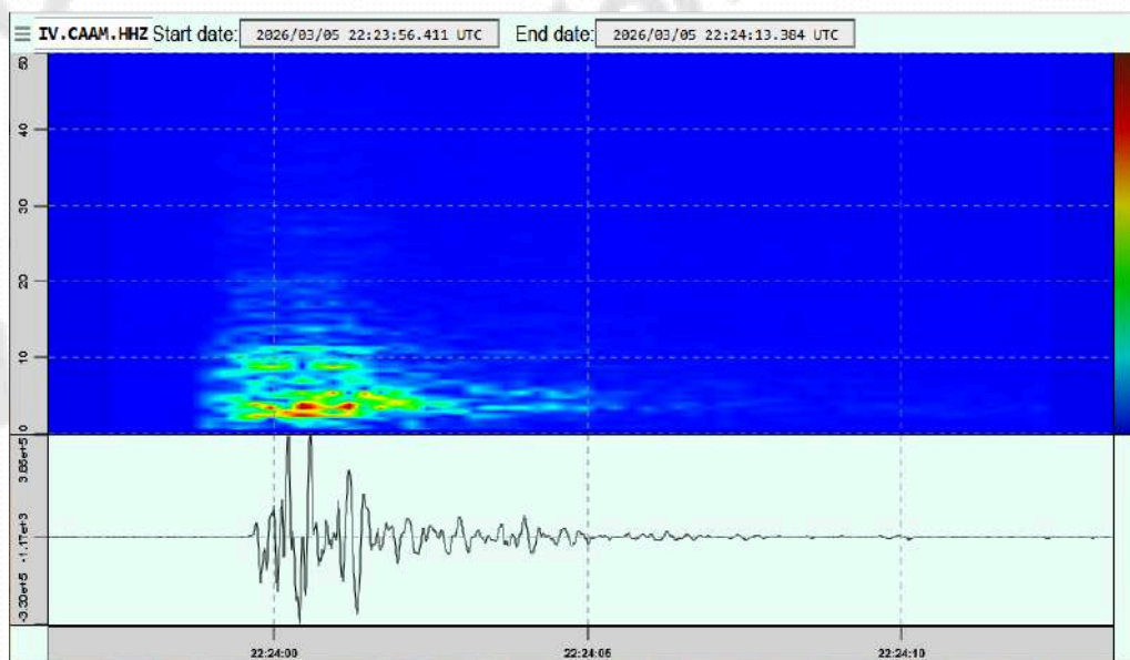
Figura 1.3 - Spettrogramma alla stazione CAAM dell'evento del 05/03/2026 alle 22:23 UTC.
