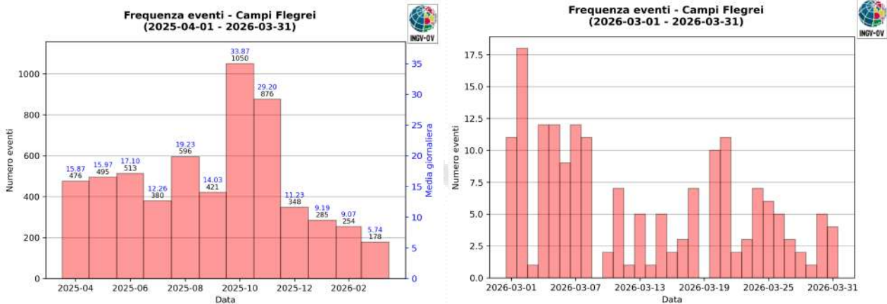
Figura 1.2 - A sinistra numero di eventi registrati ai Campi Flegrei nel corso degli ultimi 12 mesi (in totale 5872), mentre a destra quelli avvenuti nell'ultimo mese (in totale 178).
