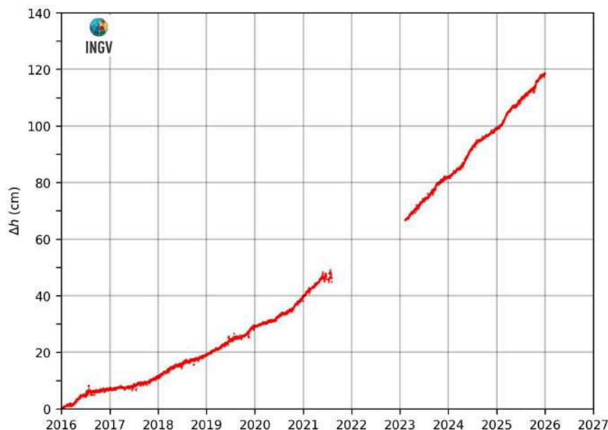
Figura 2.3.2 – Movimenti verticali del suolo, nel periodo gennaio 2016 – dicembre 2025, ottenuti dall'analisi dei dati acquisiti dalla stazione mareografica di Pozzuoli Porto (POPT), area centrale della caldera Flegrea. Le variazioni, riportate in cm, rappresentano le medie giornaliere e sono riferite alla stazione mareografica di Napoli, molo San Vincenzo (NAMM).
