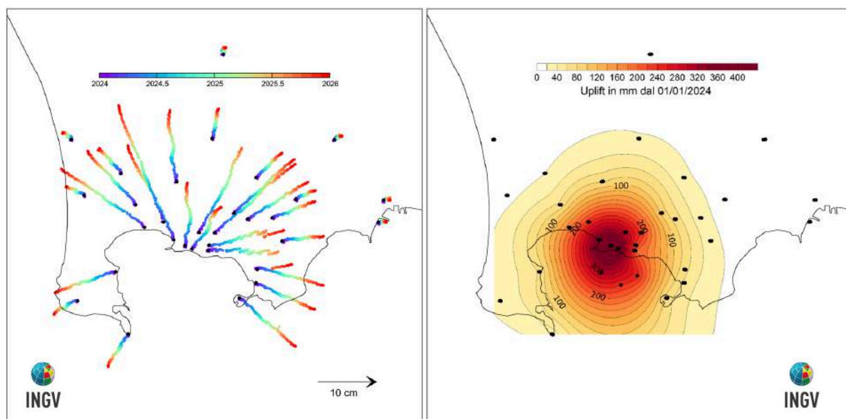
Figura 2.1.5 - Mappa degli spostamenti GNSS orizzontali (a) e verticali (b) registrati nell’area flegrea da gennaio 2024 a dicembre 2025.
