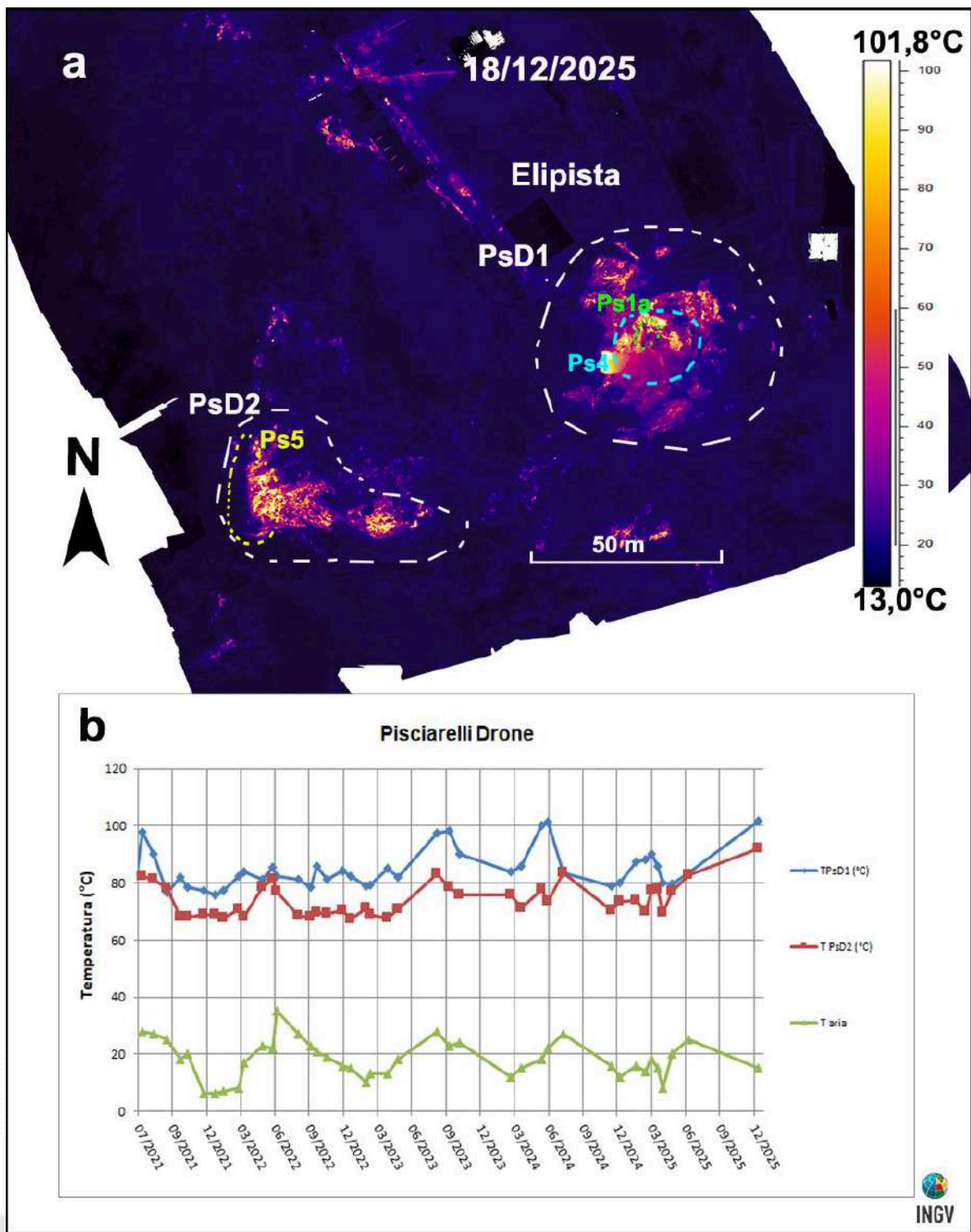
Figura 3.2.2 – Immagine termica, rilevata nel mese di dicembre 2025, dell’area denominata Ps4 (Fig.3.2.1b) (a) e valori massimi di temperatura (T) delle aree a maggiore anomalia termica (PsD1 e PsD2) confrontati con la temperatura dell’aria (Taria) misurata nel momento del rilievo termico da luglio 2021 a dicembre 2025 (b).
