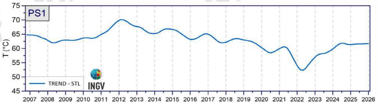
Figura 3.1.4 - Stazione PS1: Trend a lungo termine dei valori di temperatura massima rilevati nelle immagini IR ottenute mediante applicazione dell’algoritmo STL.
