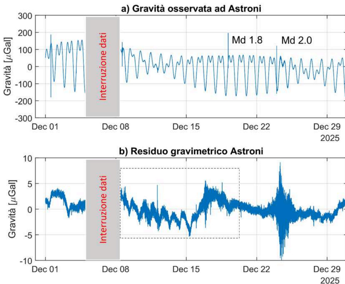
Figura 2.4.1 a: serie temporale raw (risoluzione temporale 1 minuto) registrata dal gPhone. Si osserva il contributo dominante delle maree e l'effetto di alcuni terremoti avvenuti nell'area dei Campi Flegrei. b: serie residua di gravità.
