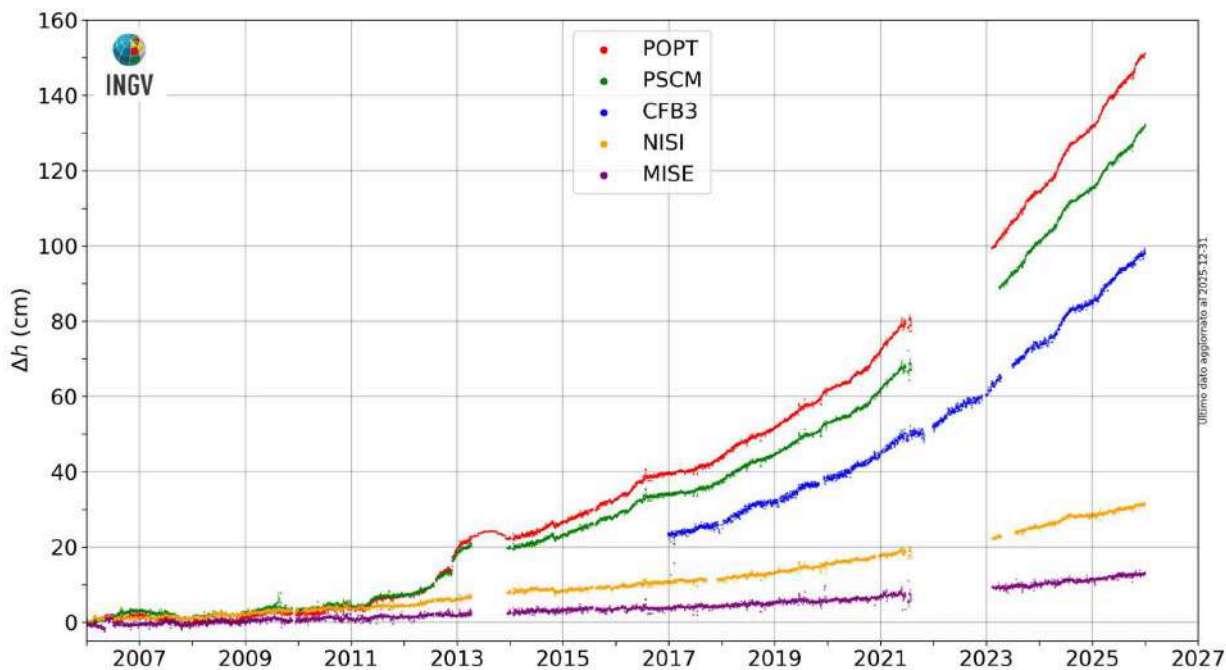
Figura 2.3.4 - Movimenti verticali del suolo nel periodo gennaio 2006 – dicembre 2025, ottenuti dall'analisi dei dati acquisiti da tutte le stazioni mareografiche dell'area della caldera Flegrea. Le variazioni, riportate in cm, rappresentano le medie giornaliere e sono tutte riferite alla stazione mareografica di Napoli, molo San Vincenzo (NAMM).
