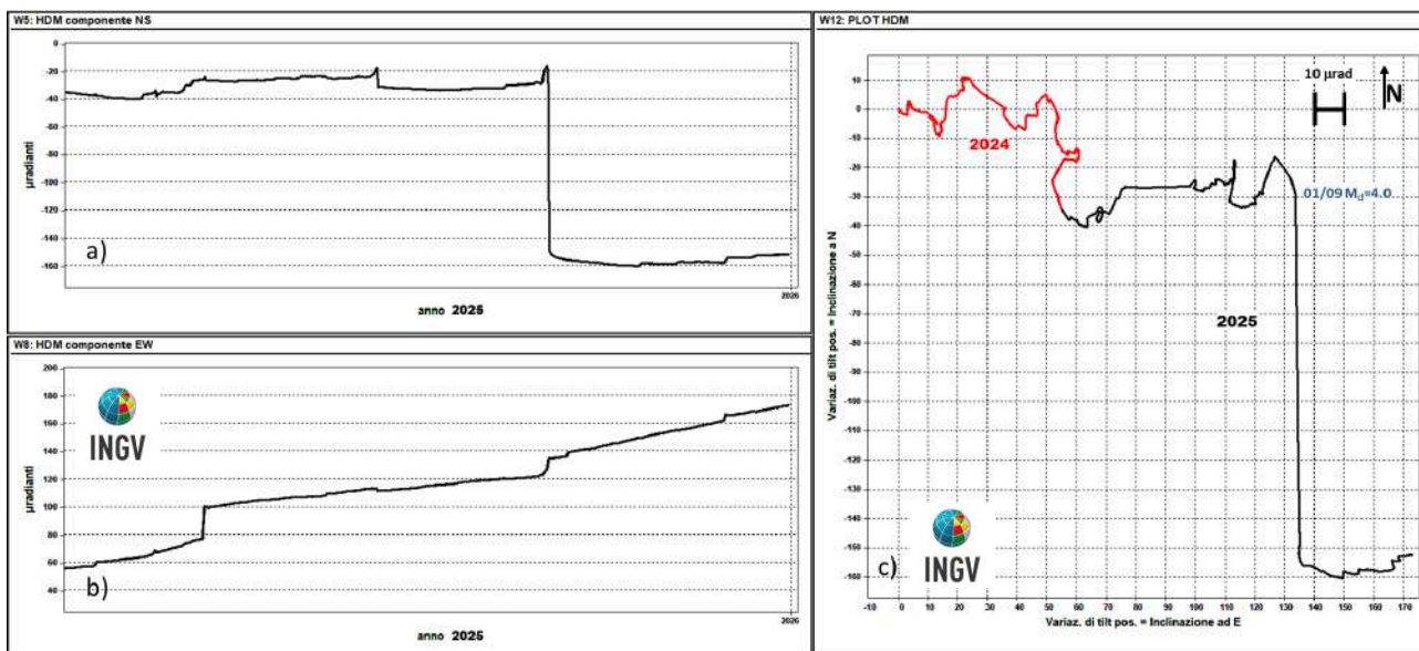
Figura 2.2.2 – Serie temporali (ultimi 12 mesi) e plot (2024-2025) del tilt della stazione HDM della rete dei Campi Flegrei.
