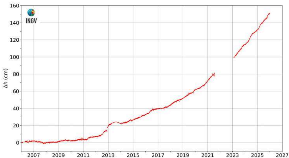
Figura 2.3.3 - Movimenti verticali del suolo nel periodo gennaio 2006 – dicembre 2025, ottenuti dall'analisi dei dati acquisiti dalla stazione mareografica di Pozzuoli Porto (POPT) (area centrale della caldera Flegrea). Le variazioni, riportate in cm, rappresentano le medie giornaliere e sono riferite alla stazione mareografica di Napoli, molo San Vincenzo (NAMM).
