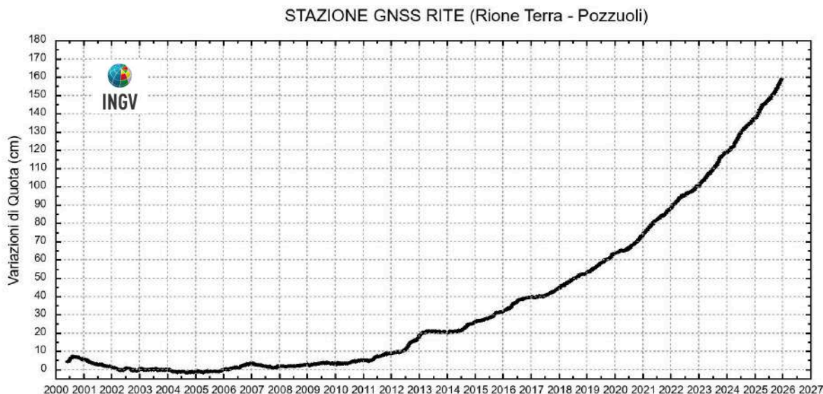
Figura 2.1.4 - Serie temporale delle variazioni settimanali in quota della stazione di RITE (Pozzuoli – Rione Terra) dal 2000 a dicembre 2025.
