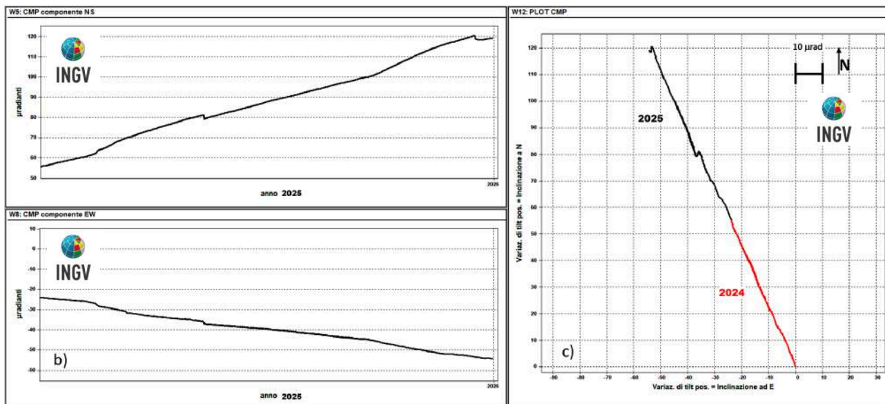
Figura 2.2.4 – Serie temporali (ultimi 12 mesi) e plot (2024-2025) del tilt della stazione CMP della rete dei Campi Flegrei.
