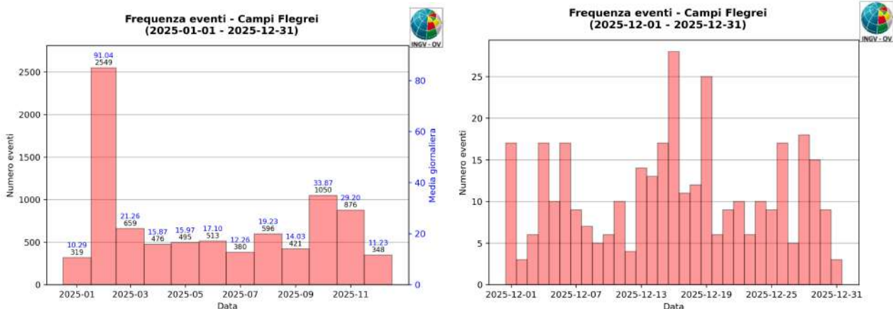
Figura 1.2 - A sinistra numero di eventi registrati ai Campi Flegrei nel corso degli ultimi 12 mesi (in totale 8682), mentre a destra quelli avvenuti nell'ultimo mese (in totale 348).
