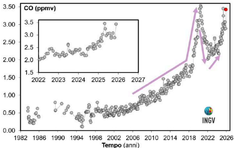
Figura 4.3 – Variazioni della concentrazione di monossido di carbonio (CO) misurato alla fumarola BG a partire dal 1983. Con il simbolo rosso è evidenziato il campione di dicembre 2025. In generale alti contenuti di CO caratterizzano sistemi vulcanici a elevata temperatura, mentre fumarole alimentate da sistemi idrotermali mostrano concentrazioni più basse, in tali sistemi un aumento delle concentrazioni di CO può riflettere un incremento delle condizioni di pressione e temperatura. Nel riquadro un dettaglio dal 2022.
