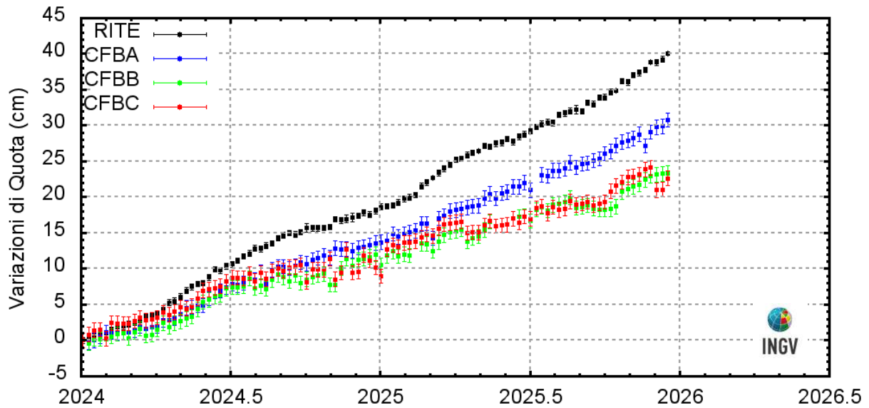
Figura 2.1.7 – Serie temporali delle variazioni settimanali in quota delle stazioni GNSS dell'infrastruttura marina MEDUSA nell'intervallo gennaio 2024 - dicembre 2025, confrontate con quella della stazione RITE
