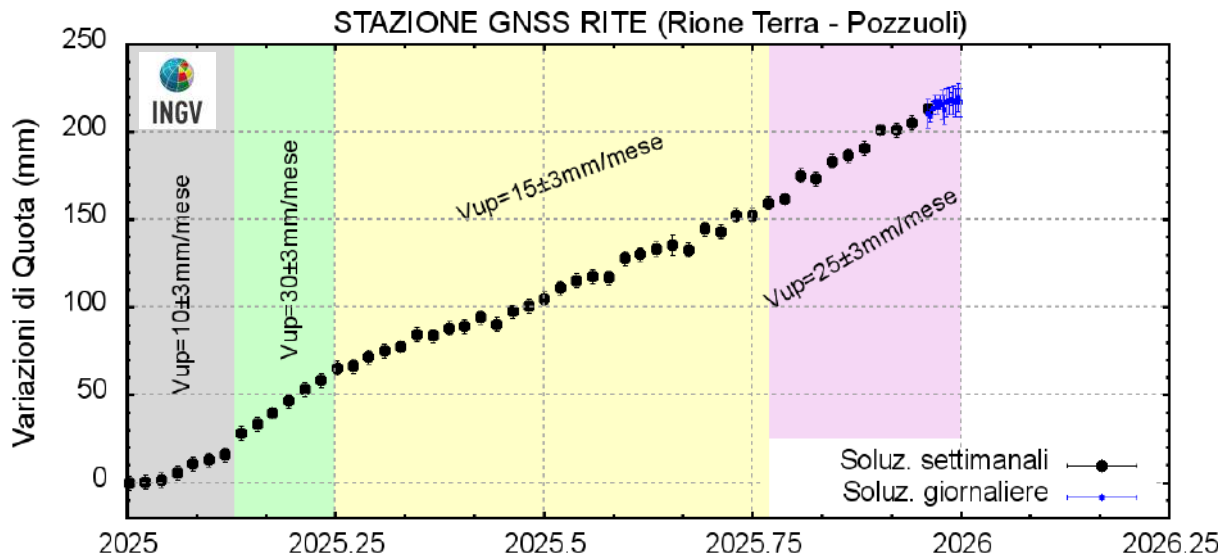
Figura 2.1.2 - Serie temporale delle variazioni in quota della stazione GNSS di RITE dal 01/01/2025 al 31/12/2025. Elaborazione dati in modalità differenziale singola baseline con software GNSS Spider.
