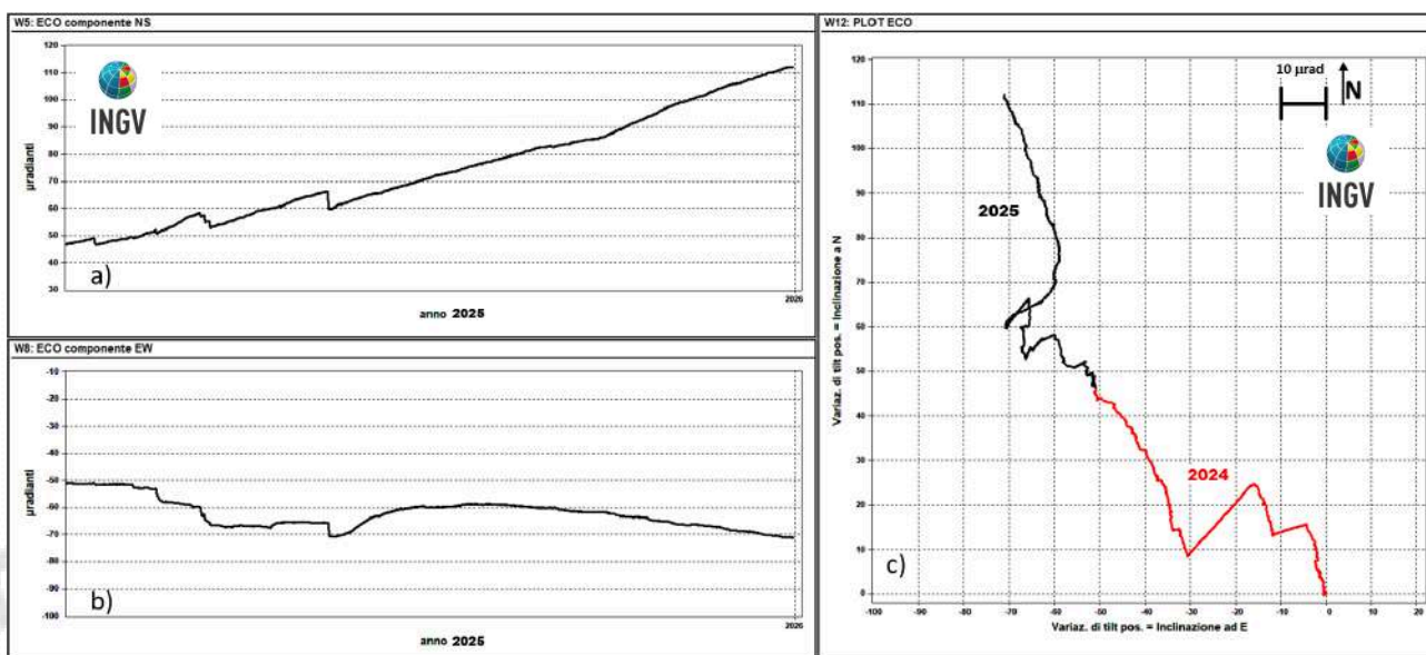
Figura 2.2.3 – Serie temporali (ultimi 12 mesi) e plot (2024-2025) del tilt della stazione ECO della rete dei Campi Flegrei.
