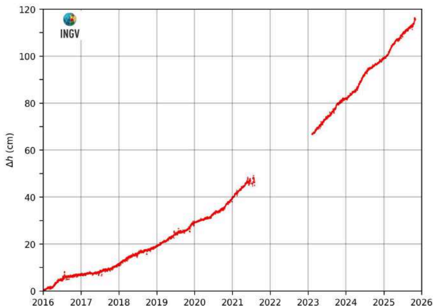
Figura 2.3.2 – Movimenti verticali del suolo, nel periodo gennaio 2016 – ottobre 2025, ottenuti dall'analisi dei dati acquisiti dalla stazione mareografica di Pozzuoli Porto (POPT), area centrale della caldera Flegrea. Le variazioni, riportate in cm, rappresentano le medie giornaliere e sono riferite alla stazione mareografica di Napoli, molo San Vincenzo (NAMM).
