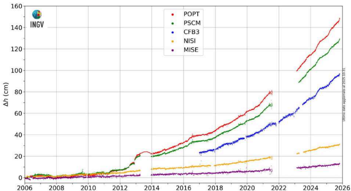
Figura 2.3.4 - Movimenti verticali del suolo nel periodo gennaio 2006 – ottobre 2025, ottenuti dall'analisi dei dati acquisiti da tutte le stazioni mareografiche dell'area della caldera Flegrea. Le variazioni, riportate in cm, rappresentano le medie giornaliere e sono tutte riferite alla stazione mareografica di Napoli, molo San Vincenzo (NAMM).
