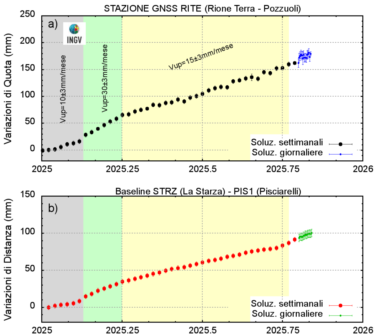
Figura 2.1.2 - a) Serie temporale delle variazioni in quota della stazione GNSS di RITE dal 01/01/2025 al 02/11/2025; b) Serie temporale delle variazioni di distanza (baseline) tra le stazioni GNSS di STRZ e PIS1 dal 01/01/2025 al 02/11/2025.
