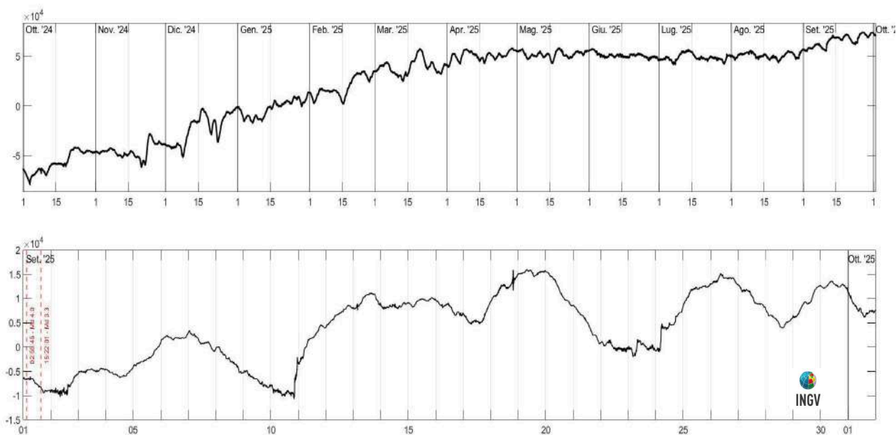
Figura 2.5.2 - In alto: Strain registrato nell'ultimo anno alla stazione di Quarto, dalle 00:00 UTC del 01/10/2024 alle 24:00 UTC del giorno 01/10/2025. In basso: Strain registrato nell'ultimo mese, dalle 00:00 UTC del giorno 01/09/2025 alle 24:00 UTC del giorno 01/10/2025.
