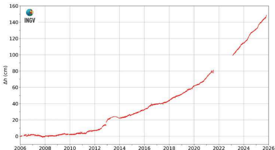
Figura 2.3.3 - Movimenti verticali del suolo nel periodo gennaio 2006 – ottobre 2025, ottenuti dall'analisi dei dati acquisiti dalla stazione mareografica di Pozzuoli Porto (POPT) (area centrale della caldera Flegrea). Le variazioni, riportate in cm, rappresentano le medie giornaliere e sono riferite alla stazione mareografica di Napoli, molo San Vincenzo (NAMM).
