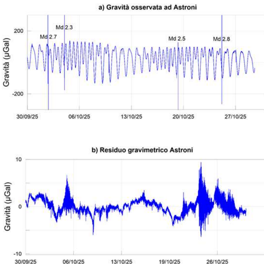
Figura 2.4.5 a: serie temporale raw (risoluzione temporale 1 minuto) registrata dal gPhone. Si osserva il contributo dominante delle maree e l'effetto di alcuni terremoti avvenuti nell'area dei Campi Flegrei. b: serie residua di gravità.
