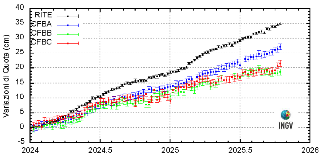
Figura 2.1.7 - Serie temporali delle variazioni settimanali in quota delle stazioni GNSS dell'infrastruttura marina MEDUSA nell'intervallo gennaio 2024 - ottobre 2025, confrontate con quella della stazione RITE
