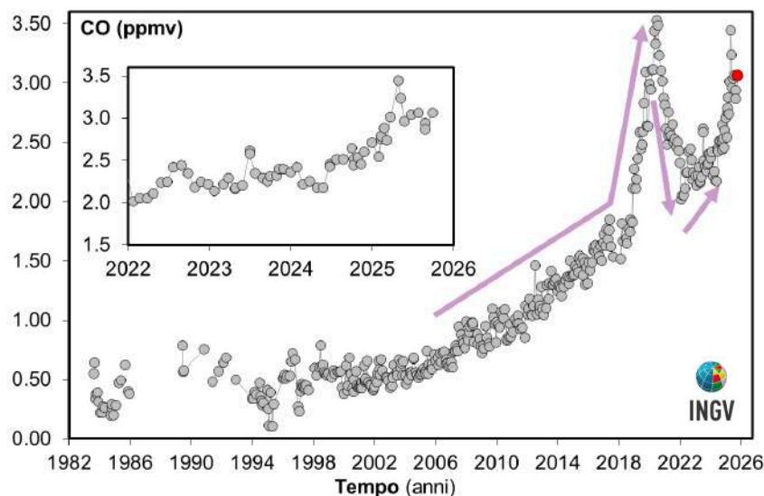
Figura 4.3 – Variazioni della concentrazione di monossido di carbonio (CO) misurato alla fumarola BG a partire dal 1983. Con il simbolo rosso sono evidenziati i campioni di ottobre 2025. In generale alti contenuti di CO caratterizzano sistemi vulcanici a elevata temperatura, mentre fumarole alimentate da sistemi idrotermali mostrano concentrazioni più basse, in tali sistemi un aumento delle concentrazioni di CO può riflettere un incremento delle condizioni di pressione e temperatura. Nel riquadro un dettaglio dal 2022.
