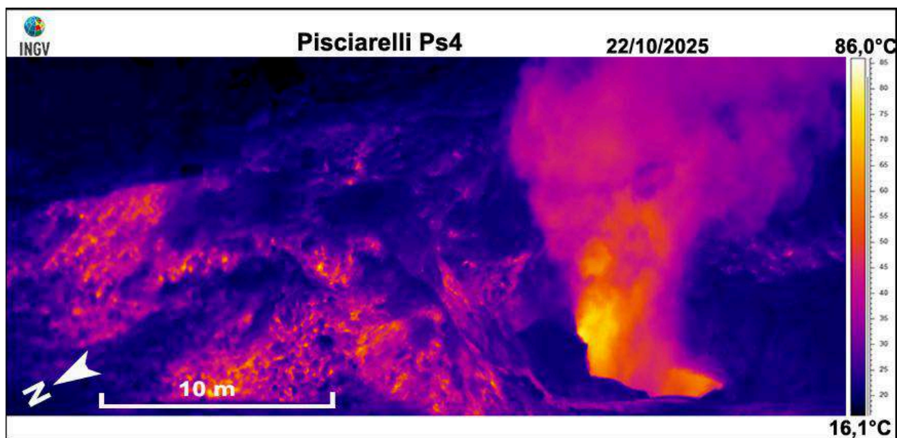
Figura 3.2.2 – Immagine termica, rilevata nel mese di ottobre 2025, dell'area denominata Ps4 (Fig.3.2.1b).
