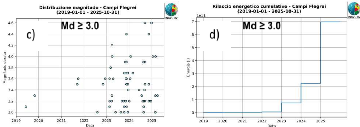
Figura 1.8 - Localizzazioni e andamento dei principali parametri sismologici dei terremoti con Md \geq 3.0 a partire dal 2019: a) frequenza di accadimento; b) profondità ipocentrali; c) magnitudo; d) energia cumulativa.
