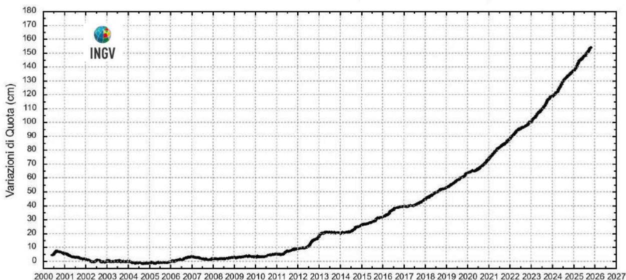
Figura 2.1.4 - Serie temporale delle variazioni settimanali in quota della stazione di RITE (Pozzuoli – Rione Terra) dal 2000 a ottobre 2025.
