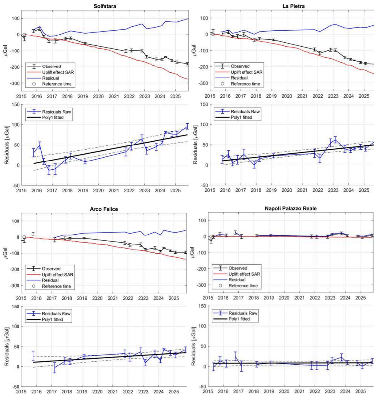
Figura 2.4.4. Serie temporali gravimetriche osservate (linee nere), dell'effetto gravimetrico dovuto ai movimenti verticali del caposaldo (linee rosse) e residue (linee blu) per alcune stazioni della rete gravimetrica dei Campi Flegrei.
