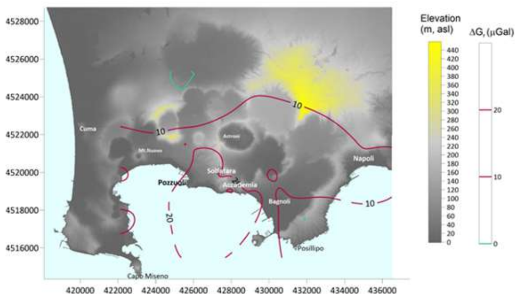
Figura 2.4.3. Residui di gravità ( \Delta_{gr} ) ottenuti tra la campagna gravimetrica di ottobre e febbraio 2025. Valori positivi di gravità (intorno ai 20\mu\text{Gal} ) si osservano nella zona centrale della caldera tra il porto di Pozzuoli, Solfatara e Accademia.
