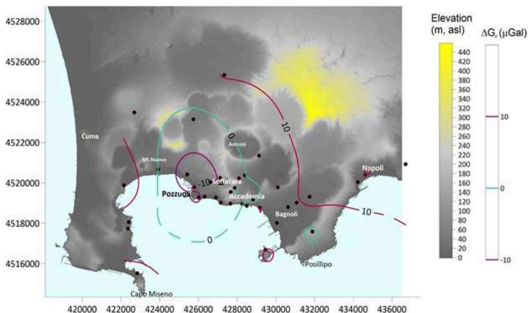
Figura 2.4.2. Differenze di gravità ottenute tra le campagne gravimetriche ottobre e febbraio 2025. I valori osservati non sono corretti per il contributo del sollevamento.
