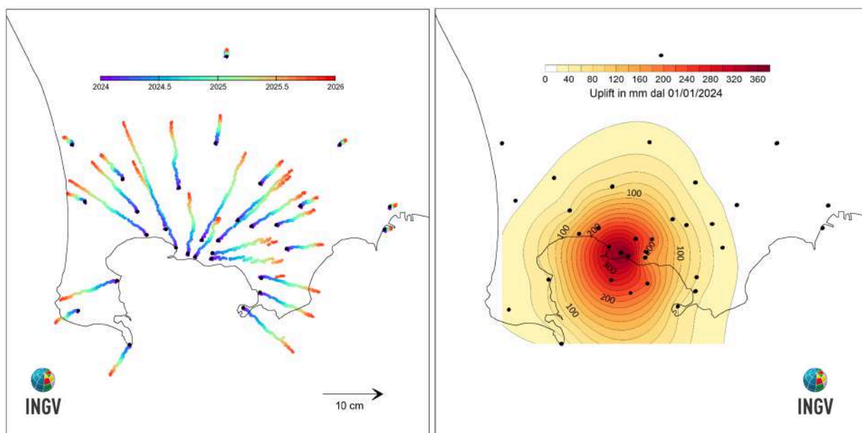
Figura 2.1.5 - Mappa degli spostamenti GNSS orizzontali (a) e verticali (b) registrati nell'area flegrea da gennaio 2024 a ottobre 2025.
