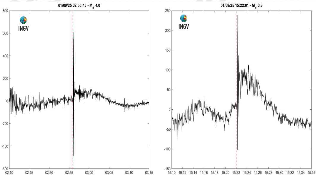
Figura 2.5.3 - Strain registrato dal dilatometro installato a Quarto in concomitanza degli eventi di M_d \geq 3.0 avvenuti durante il mese di Settembre. A sx viene riportato lo strain registrato in concomitanza dell'evento di M_d=4.0 del 01/09/2025 alle 02:55:45 UTC; a dx viene riportato lo strain relativo all'evento di M_d=3.3 del 01/09/2025 alle 15:22:01 UTC.
