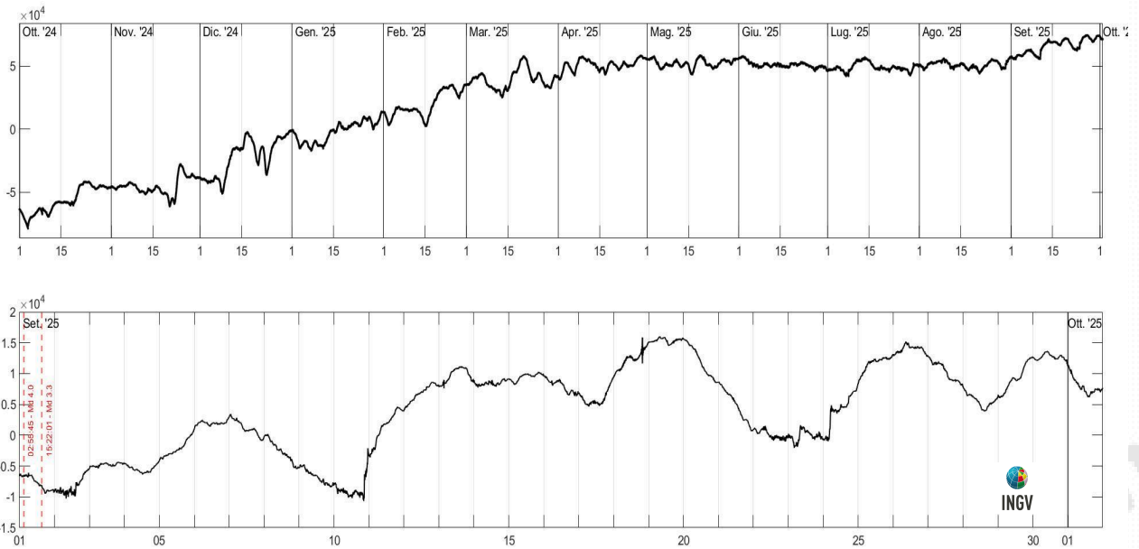
Figura 2.5.2 - In alto: Strain registrato nell'ultimo anno alla stazione di Quarto, dalle 00:00 UTC del 01/10/2024 alle 24:00 UTC del giorno 01/10/2025. In basso: Strain registrato nell'ultimo mese, dalle 00:00 UTC del giorno 01/09/2025 alle 24:00 UTC del giorno 01/10/2025.
