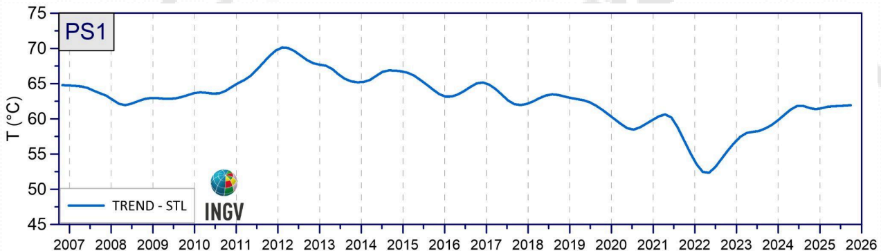
Figura 3.1.4 - Stazione PS1: Trend a lungo termine dei valori di temperatura massima rilevati nelle immagini IR ottenute mediante applicazione dell'algoritmo STL.
