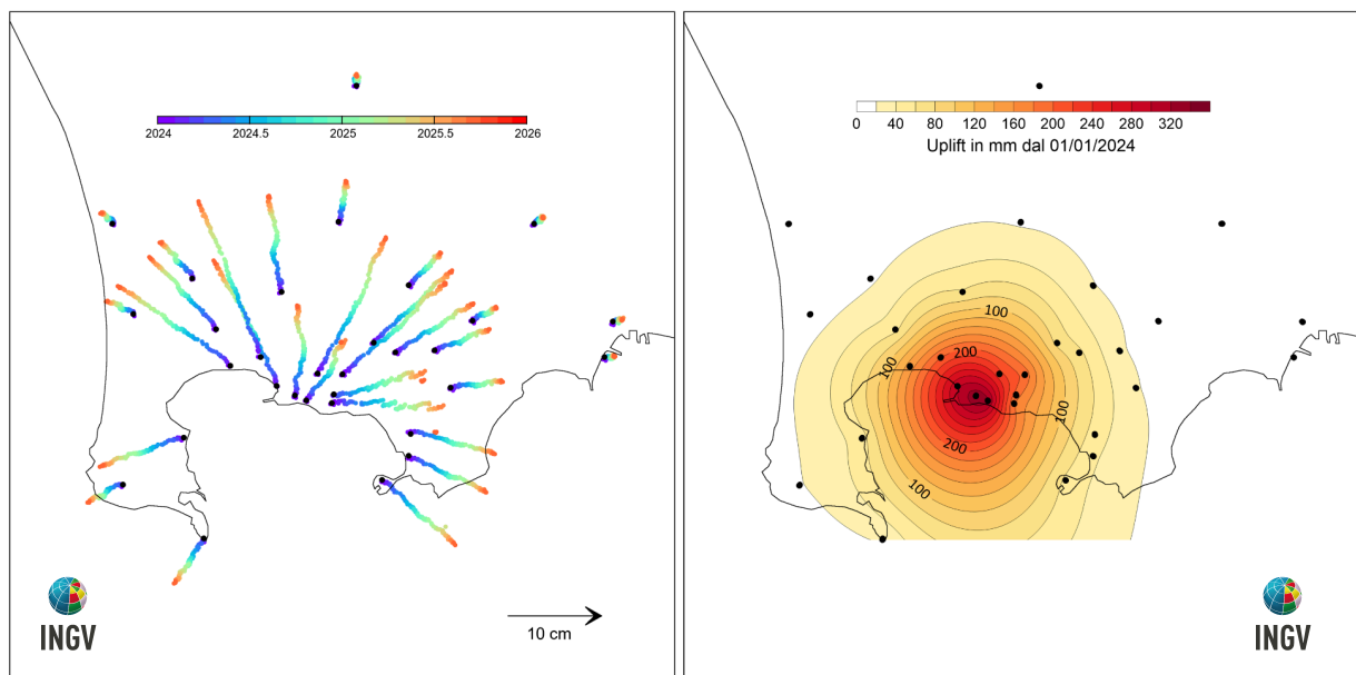
Figura 2.1.5 - Mappa degli spostamenti GNSS orizzontali (a) e verticali (b) registrati nell’area flegrea da gennaio 2024 a settembre 2025.
