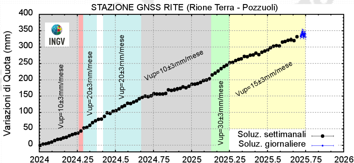
Figura 2.1.2 - Serie temporale delle variazioni in quota della stazione GNSS di RITE dal 01/01/2024 al 01/10/2025. Elaborazione dati in modalità differenziale singola baseline con software GNSS Spider.
