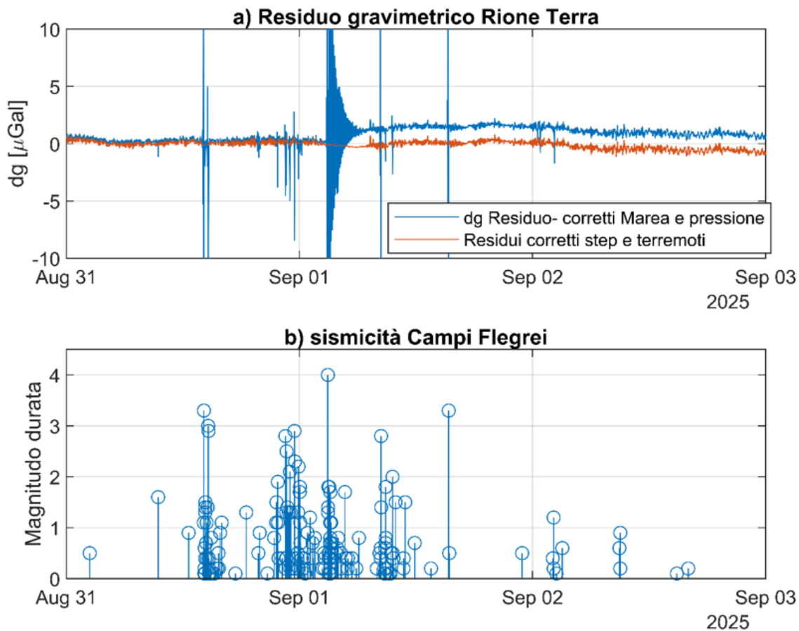
Figura 2.4.2 a: serie temporale (risoluzione temporale 1 minuto) residua registrata dal gravimetro iGrav#029. In blu: residuo gravimetrico corretto per maree e effetti di pressione atmosferica; sono evidenti gli effetti del terremoto Md 4.0 e di diversi altri sismi occorsi nell'area. In rosso: serie temporale residua, corretta di step ed effetti indotti dalla sismicità. b: Sismicità ai Campi Flegrei nel periodo considerato.
