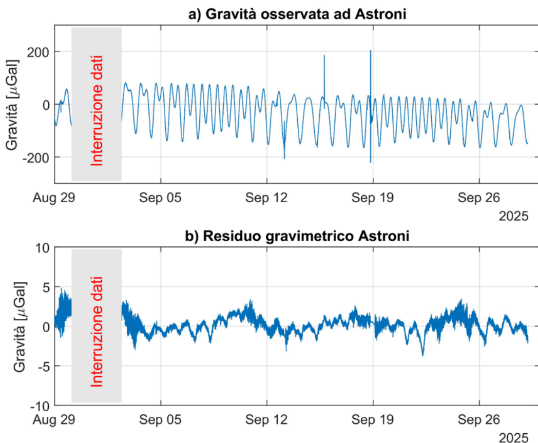
Figura 2.4.1 a: serie temporale (risoluzione temporale 1 minuto) raw registrata dal gPhone. Si osserva il contributo dominante delle maree e l'effetto di alcuni terremoti avvenuti nell'area dei Campi Flegrei. b: serie residua di gravità.
