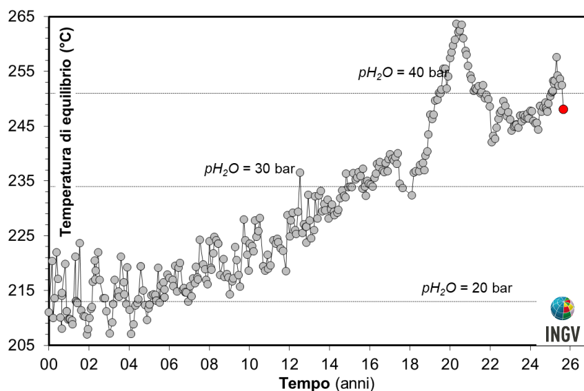
Figura 4.4 – Cronogramma delle temperature di equilibrio per il sistema CO-CO 2 relativo alla fumarola BG, stimate assumendo condizioni redox fissate dalla relazione di D'Amore and Panichi (1980). Tali temperature, rappresentative della parte più superficiale del sistema idrotermale (Caliro et al., 2007), mostrano un trend in aumento a partire dai primi anni del 2000. Con il simbolo rosso sono evidenziati i campioni di settembre 2025.
