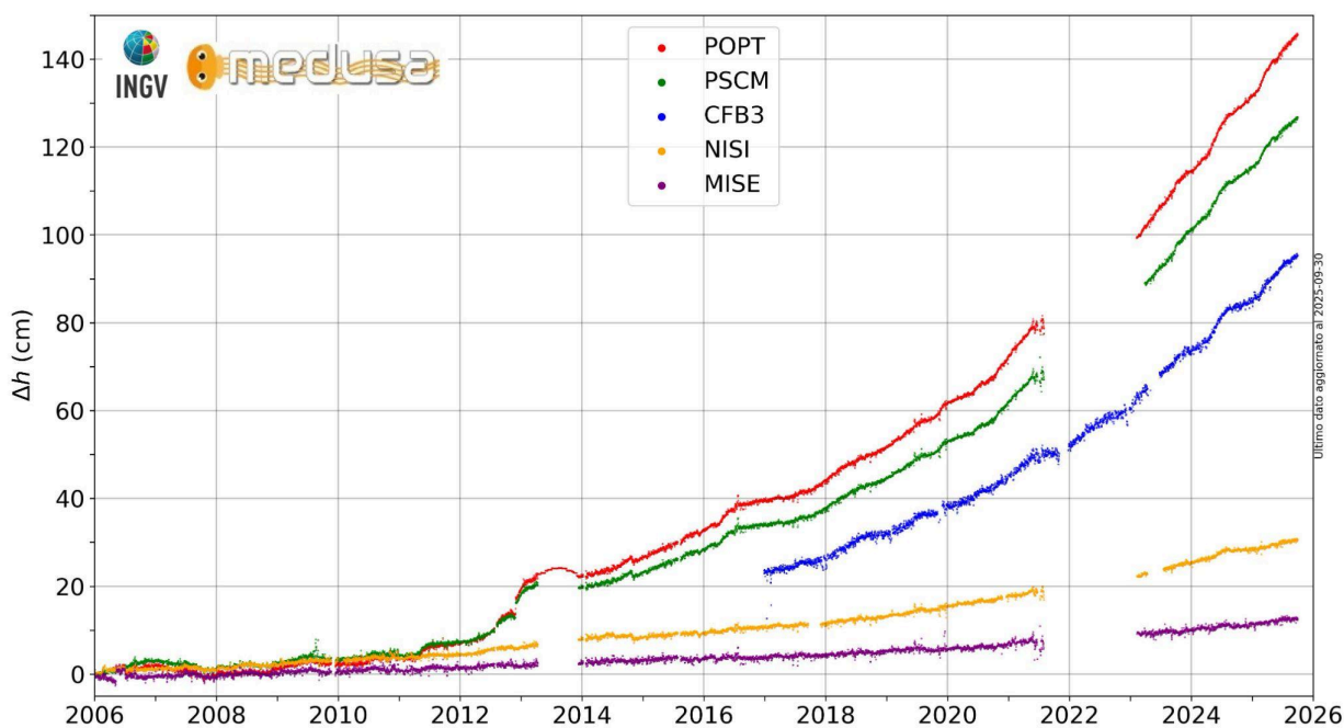
Figura 2.3.4 - Movimenti verticali del suolo nel periodo gennaio 2006 – settembre 2025, ottenuti dall’analisi dei dati acquisiti da tutte le stazioni mareografiche dell’area della caldera Flegrea. Le variazioni, riportate in cm, rappresentano le medie giornaliere e sono tutte riferite alla stazione mareografica di Napoli, molo San Vincenzo (NAMM).
