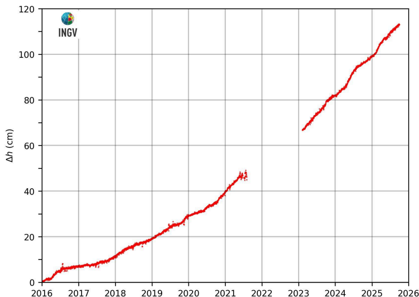
Figura 2.3.2 – Movimenti verticali del suolo, nel periodo gennaio 2016 – settembre 2025, ottenuti dall'analisi dei dati acquisiti dalla stazione mareografica di Pozzuoli Porto (POPT), area centrale della caldera Flegrea. Le variazioni, riportate in cm, rappresentano le medie giornaliere e sono riferite alla stazione mareografica di Napoli, molo San Vincenzo (NAMM).
