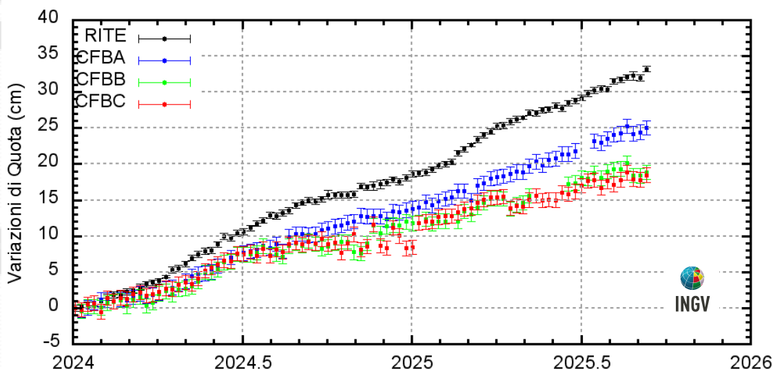
Figura 2.1.7 – Serie temporali delle variazioni settimanali in quota delle stazioni GNSS dell'infrastruttura marina MEDUSA nell'intervallo gennaio 2024 - settembre 2025, confrontate con quella della stazione RITE
