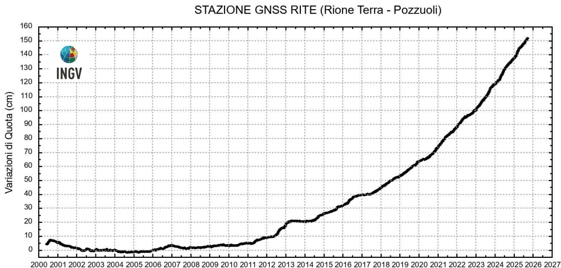
Figura 2.1.4 - Serie temporale delle variazioni settimanali in quota della stazione di RITE (Pozzuoli – Rione Terra) dal 2000 a settembre 2025.
