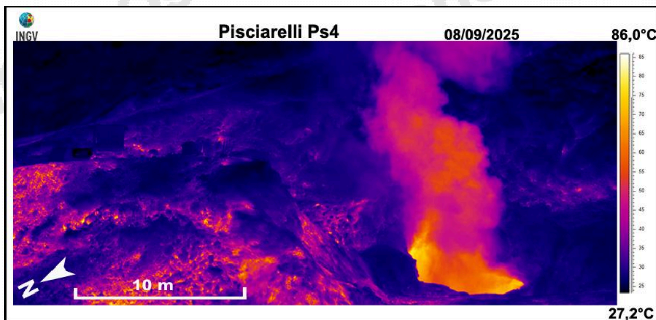
Figura 3.2.2 – Immagine termica, rilevata nel mese di settembre 2025, dell'area denominata Ps4 (Fig.3.2.1b).
