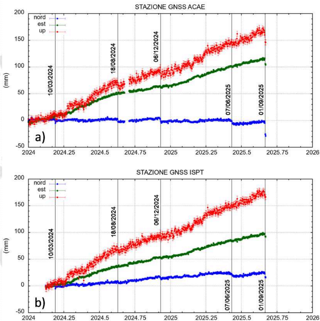
Figura 2.1.6 - Serie temporali delle variazioni giornaliere lungo le componenti Nord, Est e UP della stazione GNSS di ACAE (Accademia Aeronautica) dal 01/01/2024 al 01/09/2025. Elaborazione dati con software GNSS Bernese.
