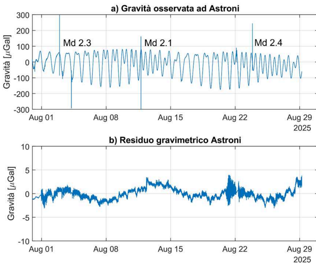
Figura 2.4.1 a: serie temporale (risoluzione temporale 1 minuto) raw registrata dal gPhoneX (#116). Si osserva il contributo dominante delle maree e l'effetto di alcuni terremoti. b: serie residua di gravità.
