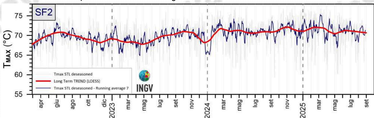
Figura 5.2.2 - Stazione ANTN. Serie temporale dei valori di temperatura massima giornaliera rilevata nelle immagini IR destagionalizzate mediante applicazione dell'algoritmo STL [medie settimanali (blu); trend a lungo termine (rosso)].
