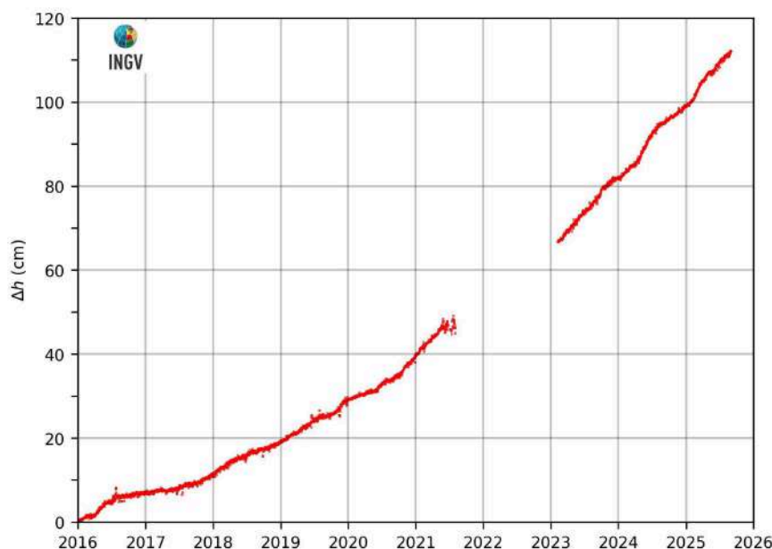
Figura 2.3.2 – Movimenti verticali del suolo, nel periodo gennaio 2016 – agosto 2025, ottenuti dall'analisi dei dati acquisiti dalla stazione mareografica di Pozzuoli Porto (POPT), area centrale della caldera Flegrea. Le variazioni, riportate in cm, rappresentano le medie giornaliere e sono riferite alla stazione mareografica di Napoli, molo San Vincenzo (NAMM).
