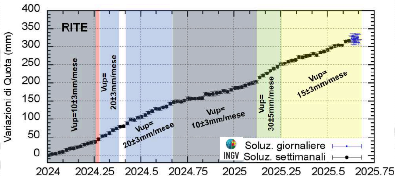
Figura 2.1.2 - Serie temporale delle variazioni in quota della stazione GNSS di RITE dal 01/01/2024 al 31/08/2025. Elaborazione dati in modalità differenziale singola baseline con software GNSS Spider.
