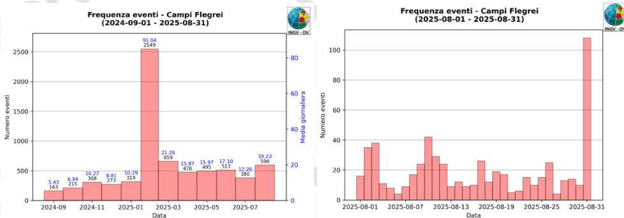
Figura 1.2 - A sinistra numero di eventi registrati ai Campi Flegrei nel corso degli ultimi 12 mesi (in totale 6946), mentre a destra quelli avvenuti nell'ultimo mese (in totale 596).
