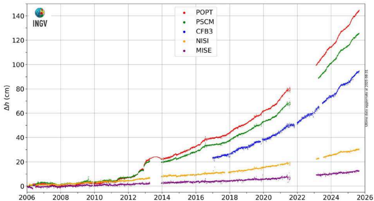
Figura 2.3.4 - Movimenti verticali del suolo nel periodo gennaio 2006 – agosto 2025, ottenuti dall'analisi dei dati acquisiti da tutte le stazioni mareografiche dell'area della caldera Flegrea. Le variazioni, riportate in cm, rappresentano le medie giornaliere e sono tutte riferite alla stazione mareografica di Napoli, molo San Vincenzo (NAMM).
