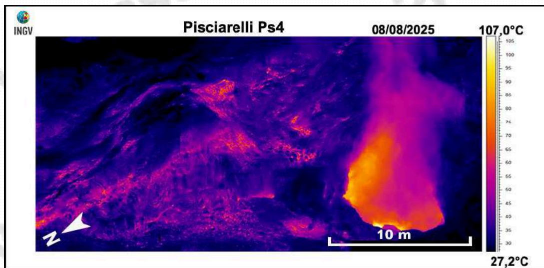
Figura 3.2.2 – Immagine termica, rilevata nel mese di agosto 2025, dell'area denominata Ps4 (Fig.3.2.1b).
