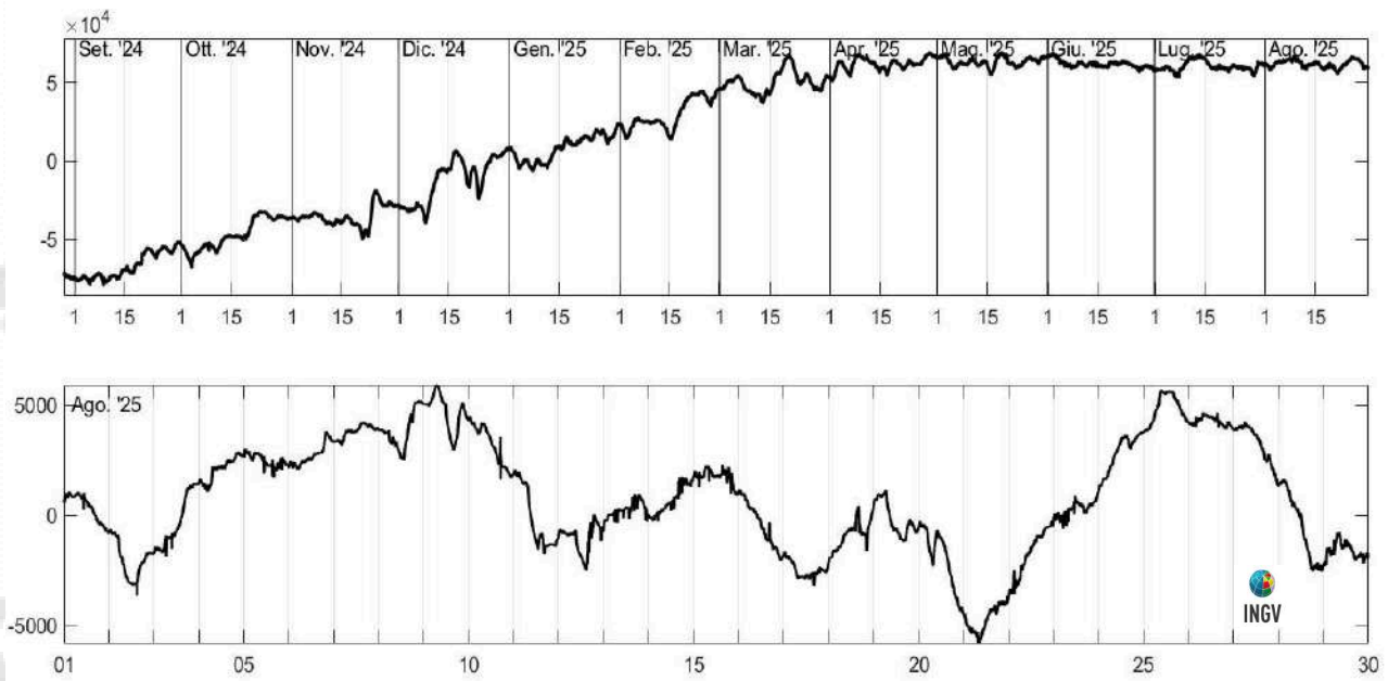
Figura 2.5.2 - In alto: Strain registrato nell'ultimo anno alla stazione di Quarto, dalle 00:00 UTC del 29/08/2024 alle 24:00 UTC del giorno 29/08/2025. In basso: Strain registrato nell'ultimo mese, dalle 00:00 UTC del giorno 01/08/2025 alle 24:00 UTC del giorno 29/08/2025.
