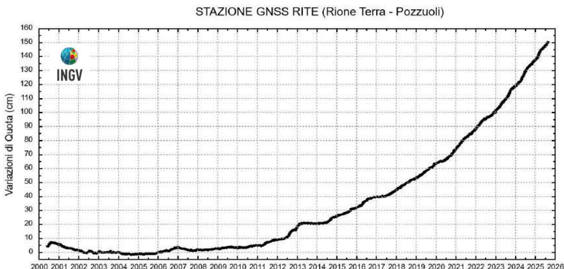
Figura 2.1.4 - Serie temporale delle variazioni settimanali in quota della stazione di RITE (Pozzuoli – Rione Terra) dal 2000 ad agosto 2025.
