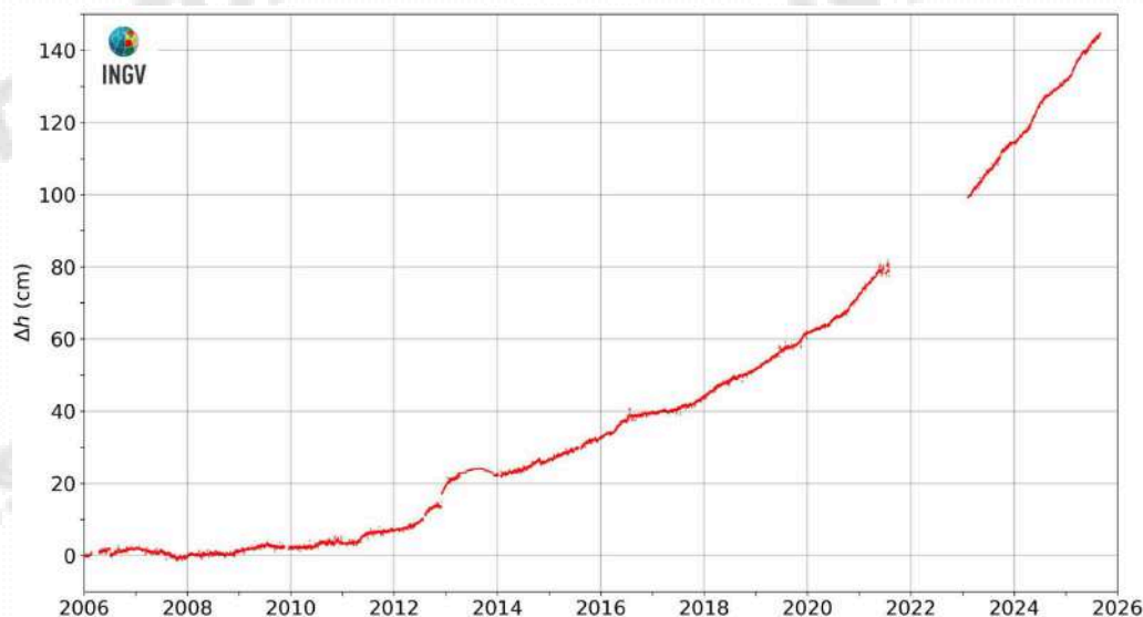
Figura 2.3.3 - Movimenti verticali del suolo nel periodo gennaio 2006 – agosto 2025, ottenuti dall'analisi dei dati acquisiti dalla stazione mareografica di Pozzuoli Porto (POPT) (area centrale della caldera Flegrea). Le variazioni, riportate in cm, rappresentano le medie giornaliere e sono riferite alla stazione mareografica di Napoli, molo San Vincenzo (NAMM).
