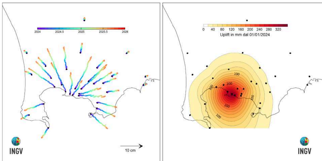
Figura 2.1.5 - Mappa degli spostamenti GNSS orizzontali (a) e verticali (b) registrati nell'area flegrea da gennaio 2024 ad agosto 2025.
