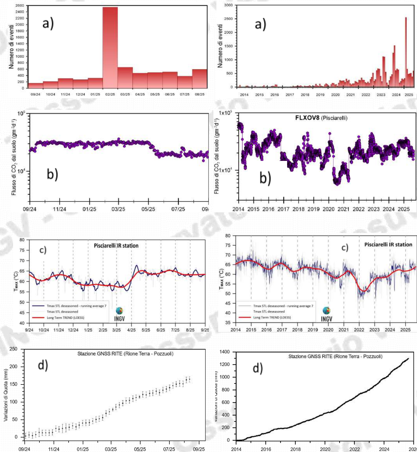
Figura 6.1 – Frequenza di accadimento degli eventi sismici (a), variazioni del flusso di CO 2 alla stazione geochimica di Pisciarelli (b), trend delle temperature massime superficiali destagionalizzate delle telecamera all’infrarosso termico a Pisciarelli (c) e andamento delle deformazioni del suolo alla stazione GNSS di RITE (d), negli ultimi dodici mesi (a sinistra) e dal 2014 (a destra).
