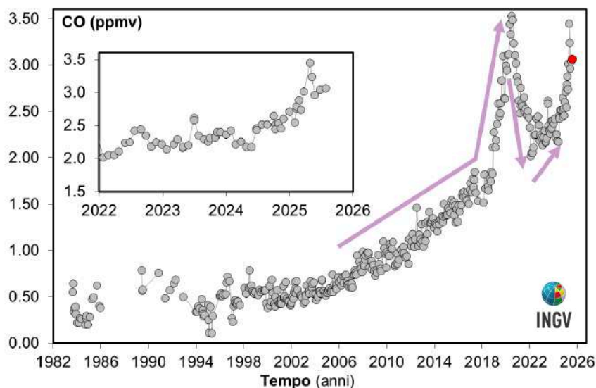
Figura 4.3 – Variazioni della concentrazione di monossido di carbonio (CO) misurato alla fumarola BG a partire dal 1983. Con il simbolo rosso è evidenziato il campione di agosto 2025. In generale alti contenuti di CO caratterizzano sistemi vulcanici a elevata temperatura, mentre fumarole alimentate da sistemi idrotermali mostrano concentrazioni più basse, in tali sistemi un aumento delle concentrazioni di CO può riflettere un incremento delle condizioni di pressione e temperatura.
