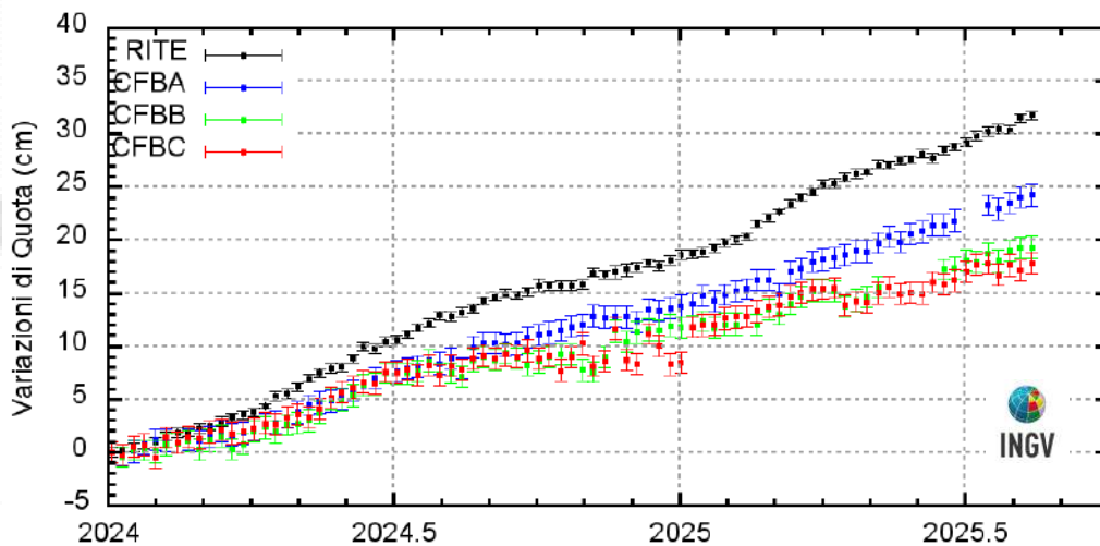
Figura 2.1.7 – Serie temporali delle variazioni settimanali in quota delle stazioni GNSS dell’infrastruttura marina MEDUSA nell’intervallo gennaio 2024 - agosto 2025, confrontate con quella della stazione RITE
