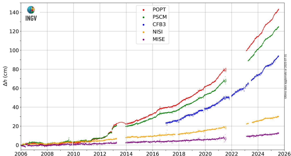
Figura 2.3.4 - Movimenti verticali del suolo nel periodo gennaio 2006 – luglio 2025, ottenuti dall'analisi dei dati acquisiti da tutte le stazioni mareografiche dell'area della caldera Flegrea. Le variazioni, riportate in cm, rappresentano le medie giornaliere e sono tutte riferite alla stazione mareografica di Napoli, molo San Vincenzo (NAMM).
