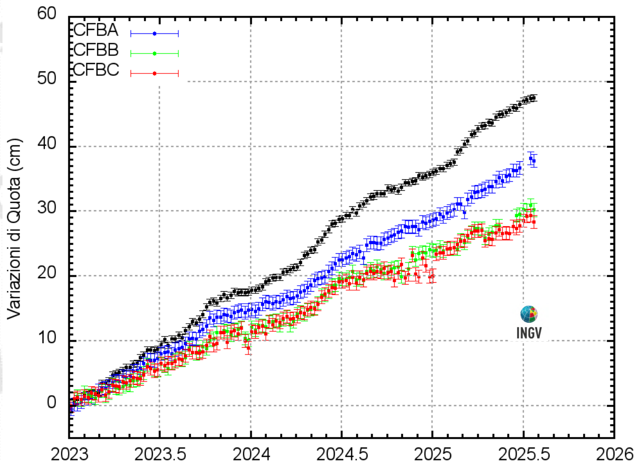
Figura 2.1.7 – Serie temporali delle variazioni settimanali in quota delle stazioni GNSS dell'infrastruttura marina MEDUSA nell'intervallo gennaio 2023 - luglio 2025, confrontate con quella della stazione RITE
