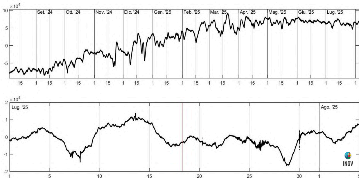
Figura 2.5.2 - In alto: Strain registrato nell'ultimo anno alla stazione di Quarto, dalle 00:00 UTC del 4/8/2024 alle 24:00 UTC del giorno 4/8/2025. In basso: Strain registrato nell'ultimo mese, dalle 00:00 UTC del giorno 1/7/2025 alle 24:00 UTC del giorno 4/8/2025. La linea verticale rossa indica l'occorrenza di evento sismico di magnitudo maggiore di 3.
