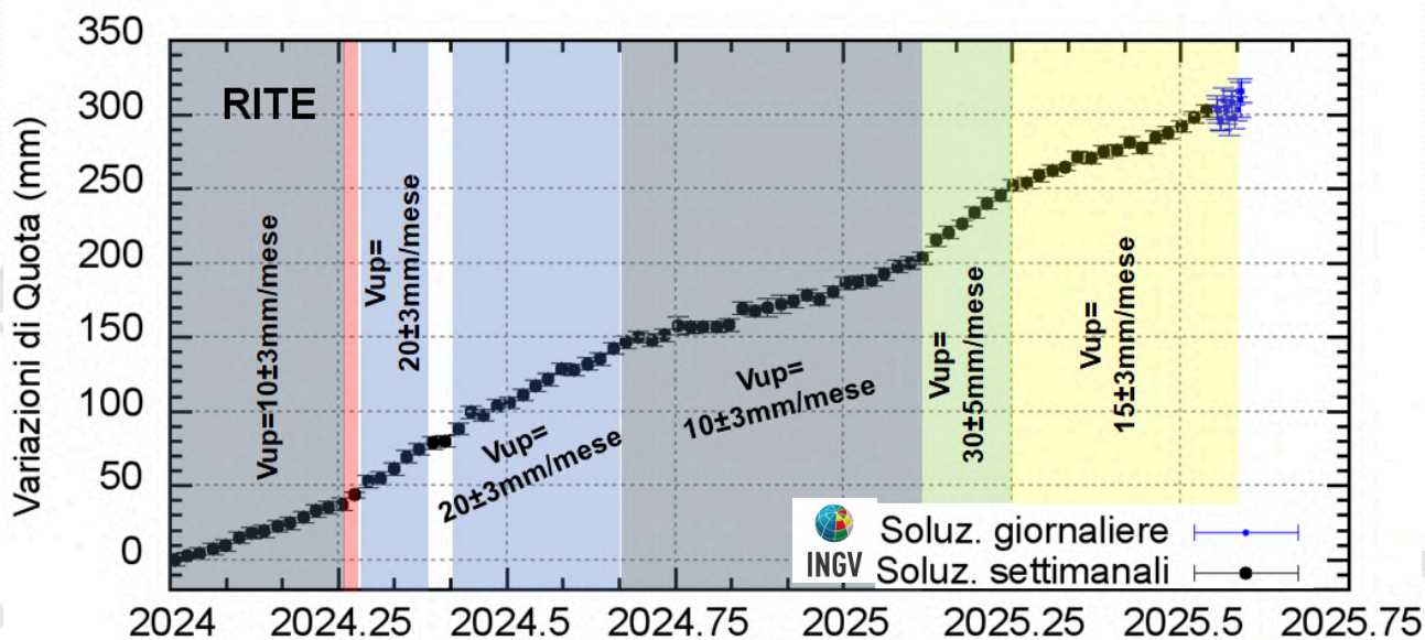
Figura 2.1.2 - Serie temporale delle variazioni in quota della stazione GNSS di RITE dal 01/01/2024 al 04/08/2025. Elaborazione dati in modalità differenziale singola baseline con software GNSS Spider.
