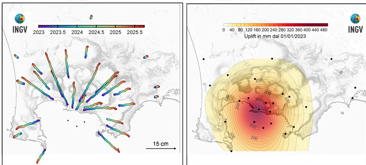
Figura 2.1.5 - Mappa degli spostamenti GNSS orizzontali (a) e verticali (b) registrati nell'area flegrea da gennaio 2023 a luglio 2025.
