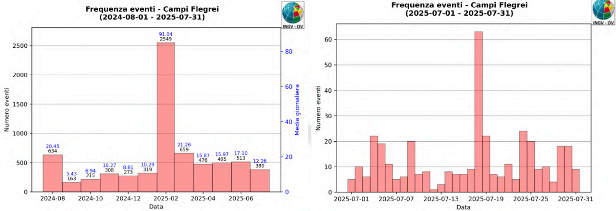
Figura 1.2 - A sinistra numero di eventi registrati ai Campi Flegrei nel corso degli ultimi 12 mesi (in totale 6984), mentre a destra quelli avvenuti nell'ultimo mese (in totale 380).
