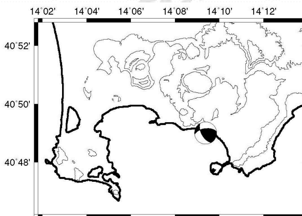
Figura 1.7 - Localizzazione ipocentrale e meccanismo focale dell'evento del 18/07/2025 alle ore 07:14 UTC di M_d 4.0 \pm 0.3 .
