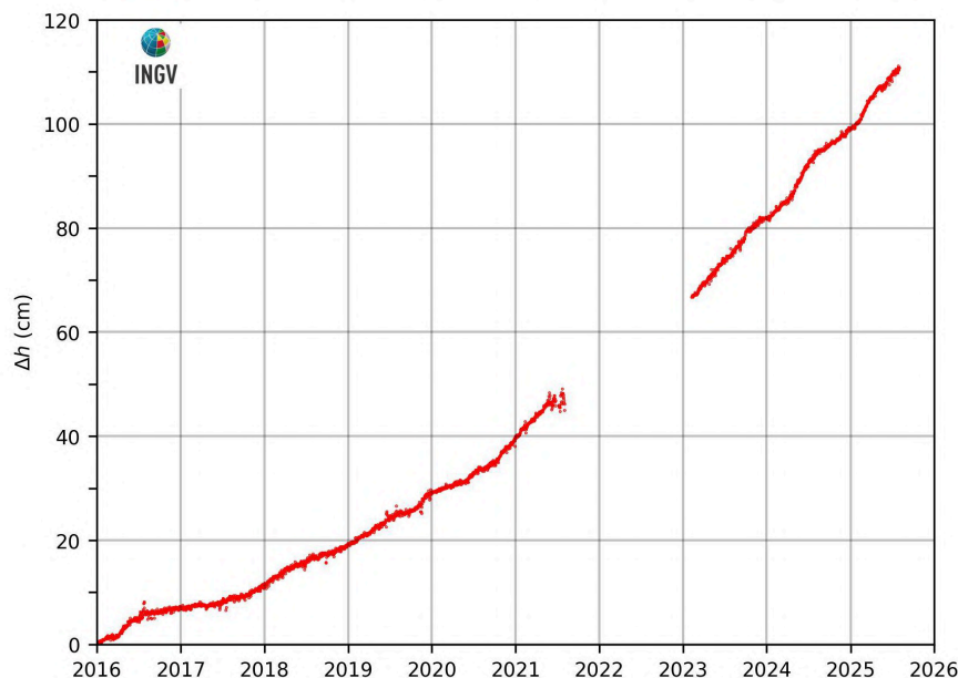
Figura 2.3.2 – Movimenti verticali del suolo, nel periodo gennaio 2016 – luglio 2025, ottenuti dall'analisi dei dati acquisiti dalla stazione mareografica di Pozzuoli Porto (POPT), area centrale della caldera Flegrea. Le variazioni, riportate in cm, rappresentano le medie giornaliere e sono riferite alla stazione mareografica di Napoli, molo San Vincenzo (NAMM).
