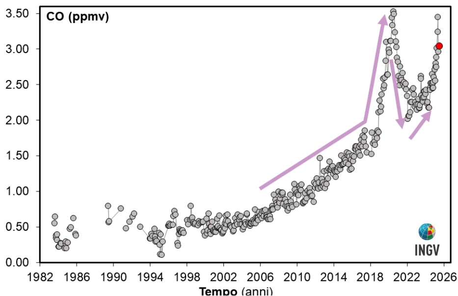
Figura 4.3 – Variazioni della concentrazione di monossido di carbonio (CO) misurato alla fumarola BG a partire dal 1983. Con il simbolo rosso è evidenziato il campione di luglio 2025. In generale alti contenuti di CO caratterizzano sistemi vulcanici a elevata temperatura, mentre fumarole alimentate da sistemi idrotermali mostrano concentrazioni più basse, in tali sistemi un aumento delle concentrazioni di CO può riflettere un incremento delle condizioni di pressione e temperatura.
