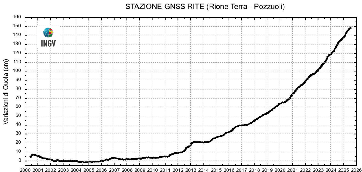
Figura 2.1.4 - Serie temporale delle variazioni settimanali in quota della stazione di RITE (Pozzuoli – Rione Terra) dal 2000 a luglio 2025.
