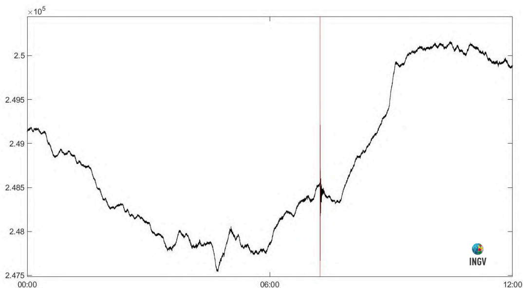
Figura 2.5.3 - strain registrato dal dilatometro installato a Quarto in concomitanza dell'event0 di M_d=4.0 avvenuto il 18 luglio.
