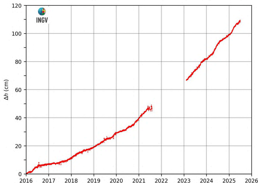
Figura 2.3.2 – Movimenti verticali del suolo, nel periodo gennaio 2016 – giugno 2025, ottenuti dall'analisi dei dati acquisiti dalla stazione mareografica di Pozzuoli Porto (POPT), area centrale della caldera Flegrea. Le variazioni, riportate in cm, rappresentano le medie giornaliere e sono riferite alla stazione mareografica di Napoli, molo San Vincenzo (NAMM).
