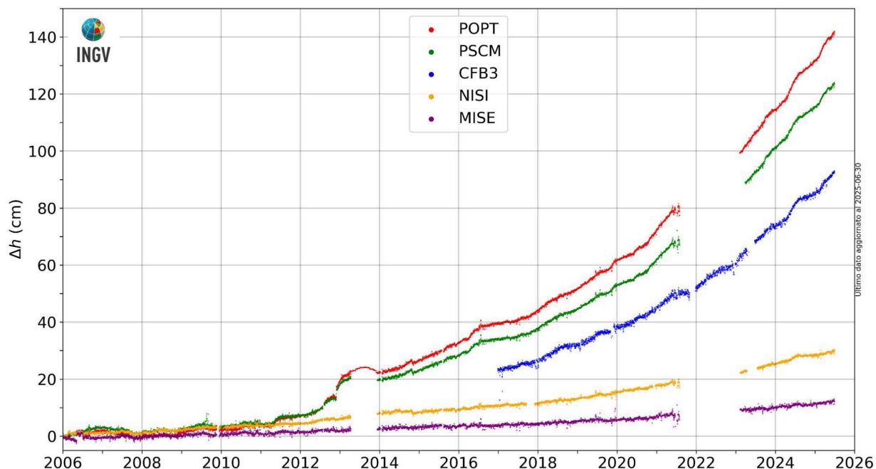
Figura 2.3.4 - Movimenti verticali del suolo nel periodo gennaio 2006 – giugno 2025, ottenuti dall'analisi dei dati acquisiti da tutte le stazioni mareografiche dell'area della caldera Flegrea. Le variazioni, riportate in cm, rappresentano le medie giornaliere e sono tutte riferite alla stazione mareografica di Napoli, molo San Vincenzo (NAMM).
