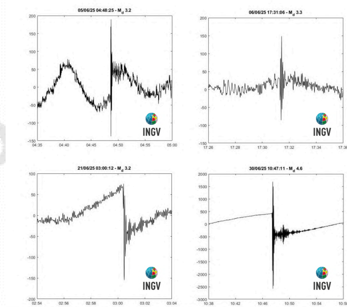
Figura 2.5.3 - Variazioni cosismiche ad alta frequenza registrate dal dilatometro installato a Quarto in concomitanza degli eventi di M_d \geq 3.0 avvenuti nel periodo di analisi.
