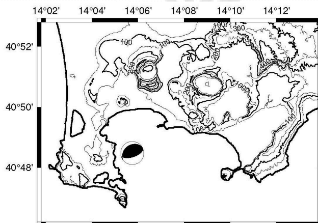
Figura 1.7 - Localizzazione ipocentrale e meccanismo focale dell'evento del 30/06/2025 alle ore 10:47 UTC di Md 4.6 \pm 0.3 .
