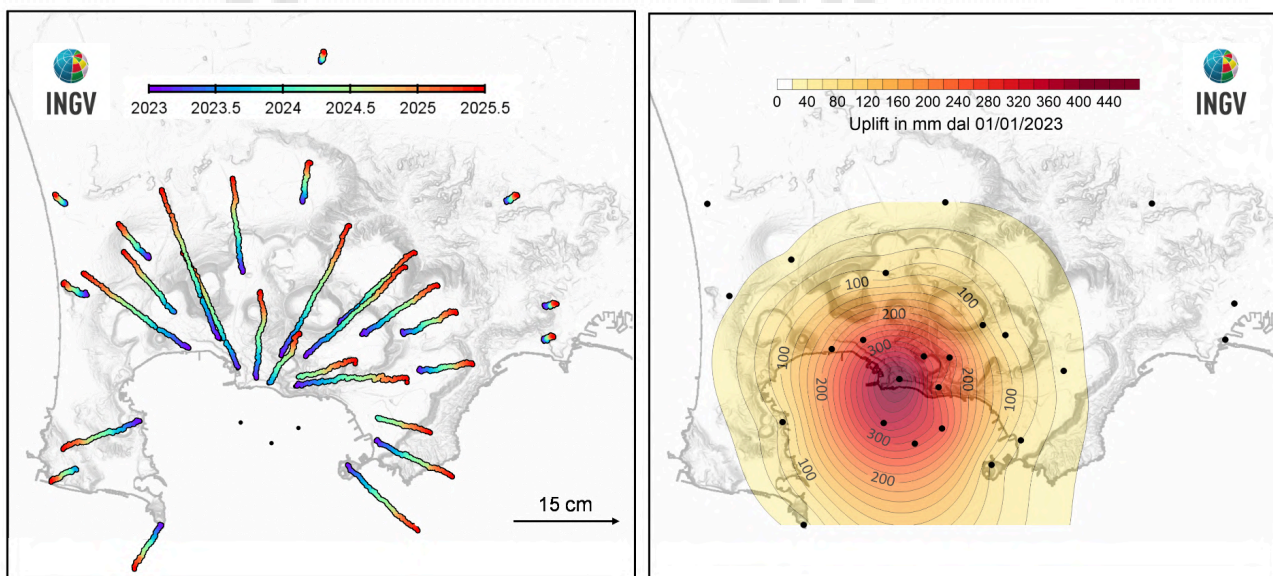
Figura 2.1.5 - Mappa degli spostamenti GNSS orizzontali (a) e verticali (b) registrati nell'area flegrea da gennaio 2023 a giugno 2025.
