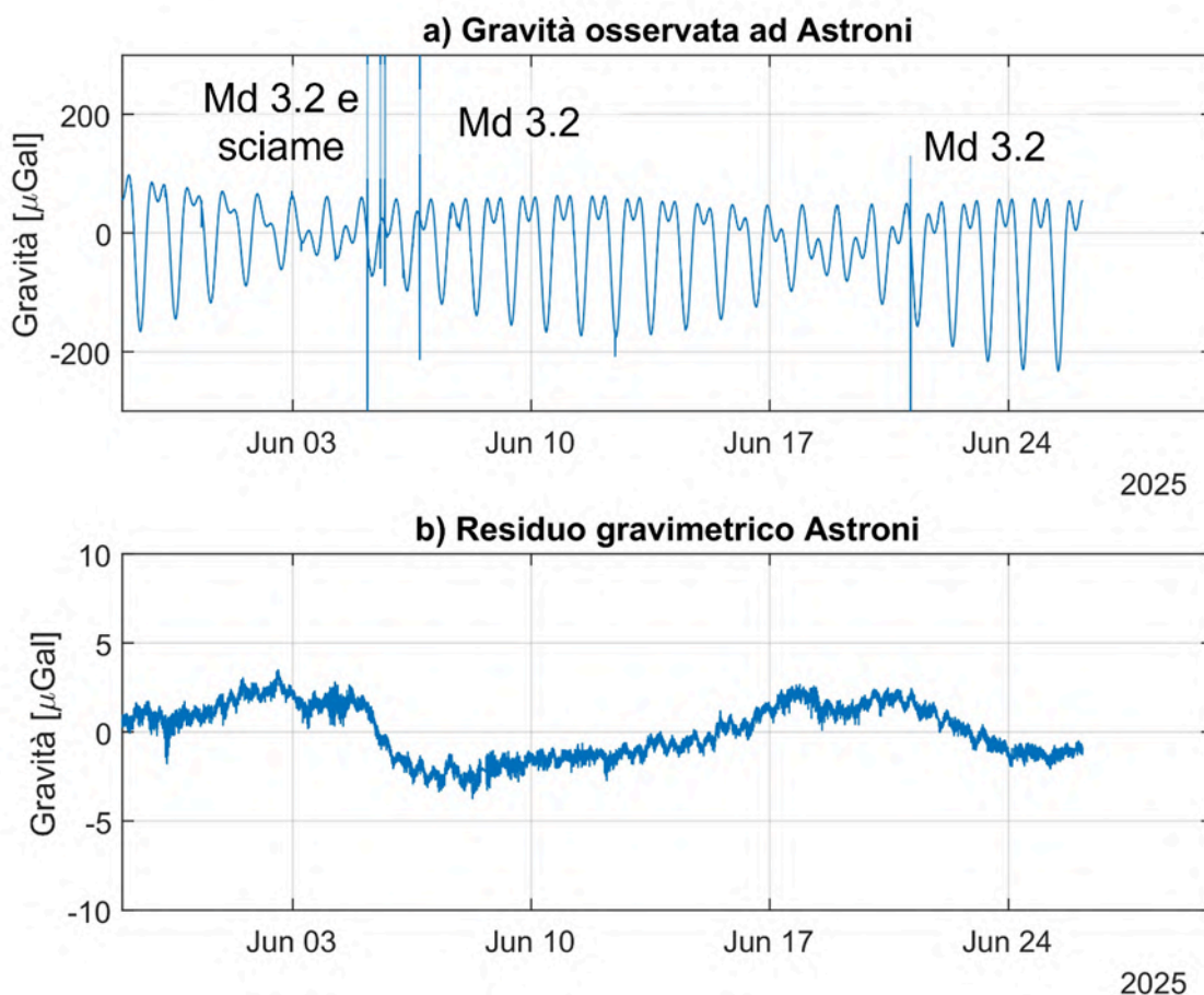
Figura 2.4.1 a: serie temporale (risoluzione temporale 1 minuto) raw registrata dal gPhoneX (#116). Si osserva il contributo dominante delle maree. b: serie residua di gravità.
