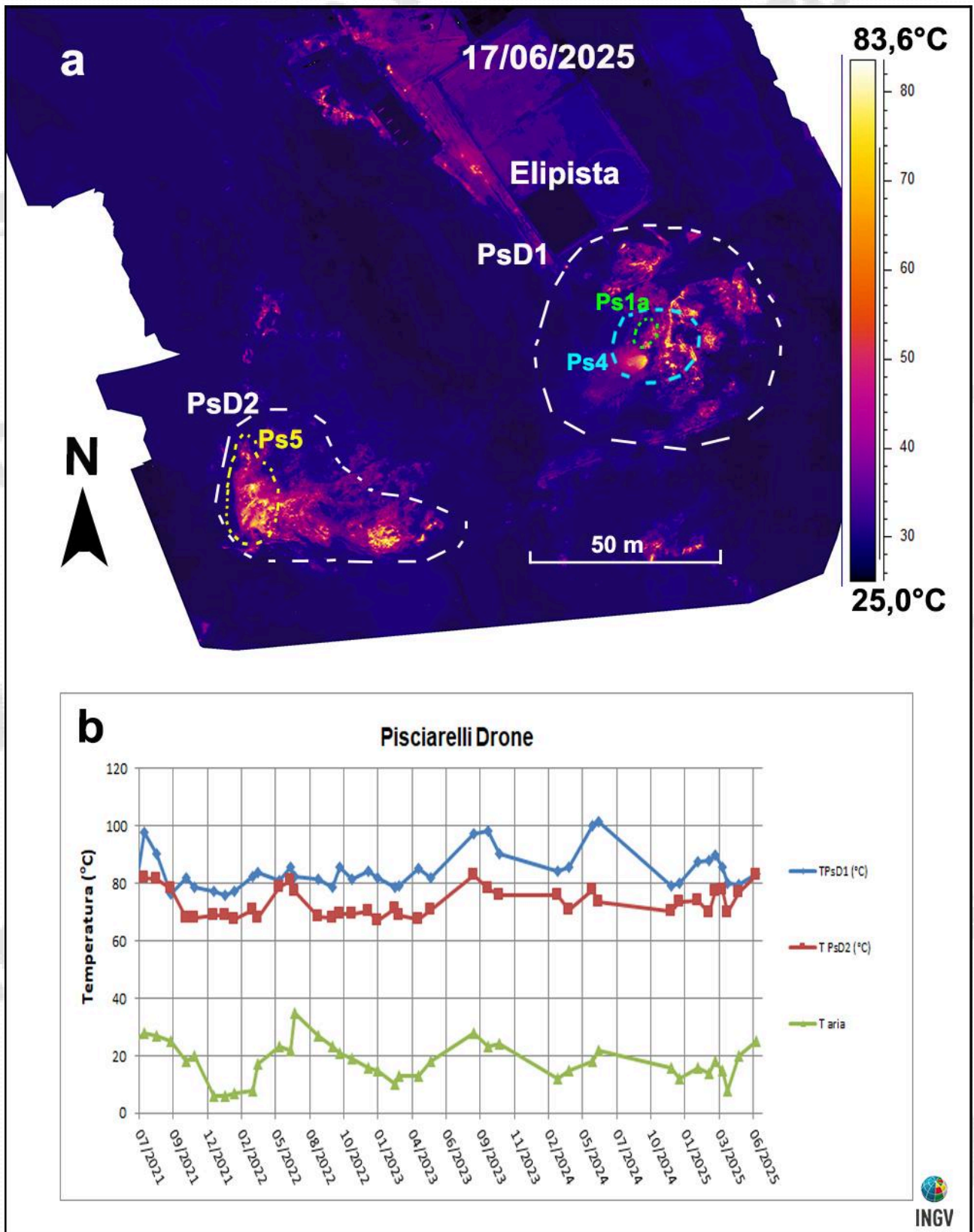
Figura 3.2.2 – Immagine termica, rilevata nel mese di giugno 2025, dell’area denominata Ps4 (Fig.3.2.1b) (a) e valori massimi di temperatura (T) delle aree a maggiore anomalia termica (PsD1 e PsD2) confrontati con la temperatura dell’aria (Taria) misurata nel momento del rilievo termico da luglio 2021 a giugno 2025 (b).
