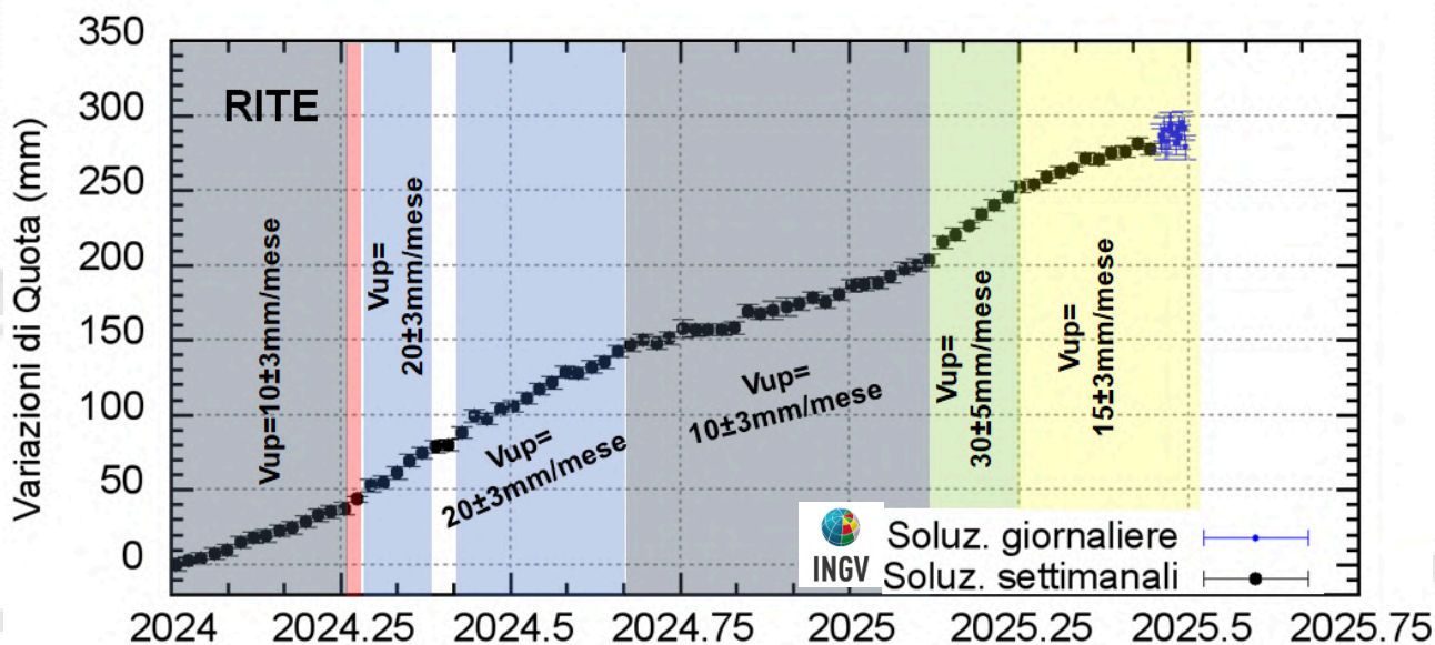
Figura 2.1.2 - Serie temporale delle variazioni in quota della stazione GNSS di RITE dal 01/01/2024 al 30/06/2025. Elaborazione dati in modalità differenziale singola baseline con software GNSS Spider.
