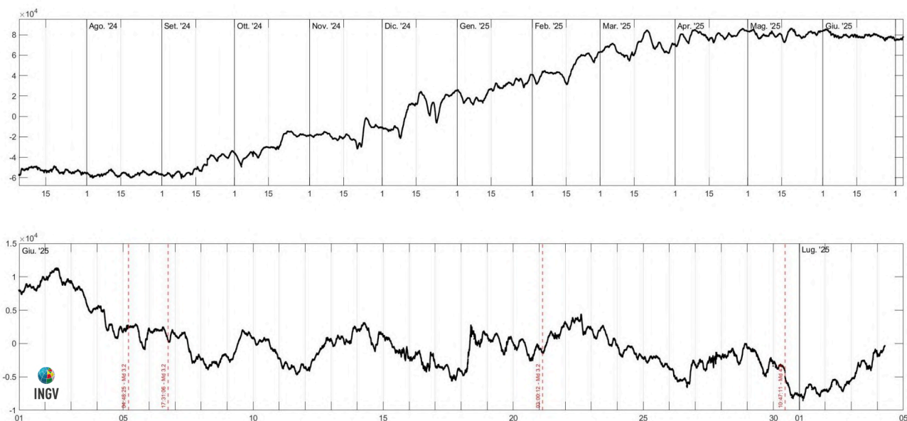
Figura 2.5.2 - In alto: Strain registrato nell'ultimo anno alla stazione di Quarto, dalle 00:00 UTC del 4/7/2024 alle 08:00 UTC del giorno 4/7/2025. In basso: Strain registrato nell'ultimo mese, dalle 00:00 UTC del giorno 1/6/2025 alle 08:00 UTC del giorno 4/7/2025. Le linee verticali rosse indicano l'occorrenza di eventi sismici con magnitudo maggiore di 3.
