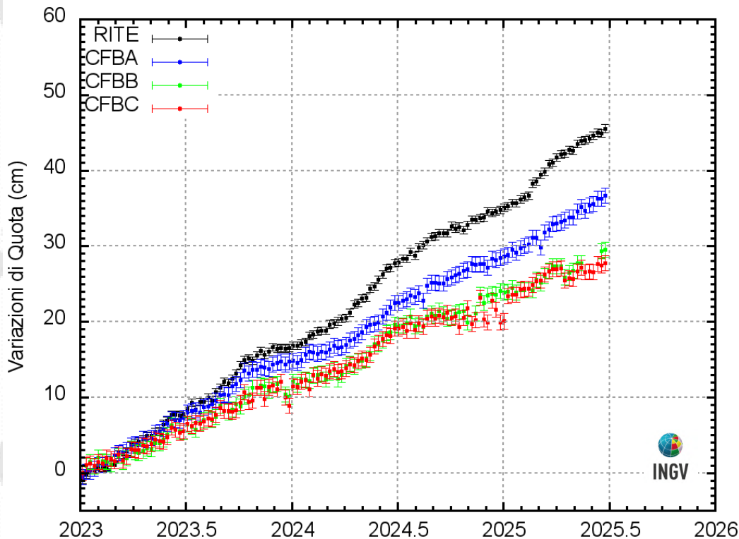
Figura 2.1.7 – Serie temporali delle variazioni settimanali in quota delle stazioni GNSS dell'infrastruttura marina MEDUSA nell'intervallo gennaio 2023 - giugno 2025, confrontate con quella della stazione RITE
