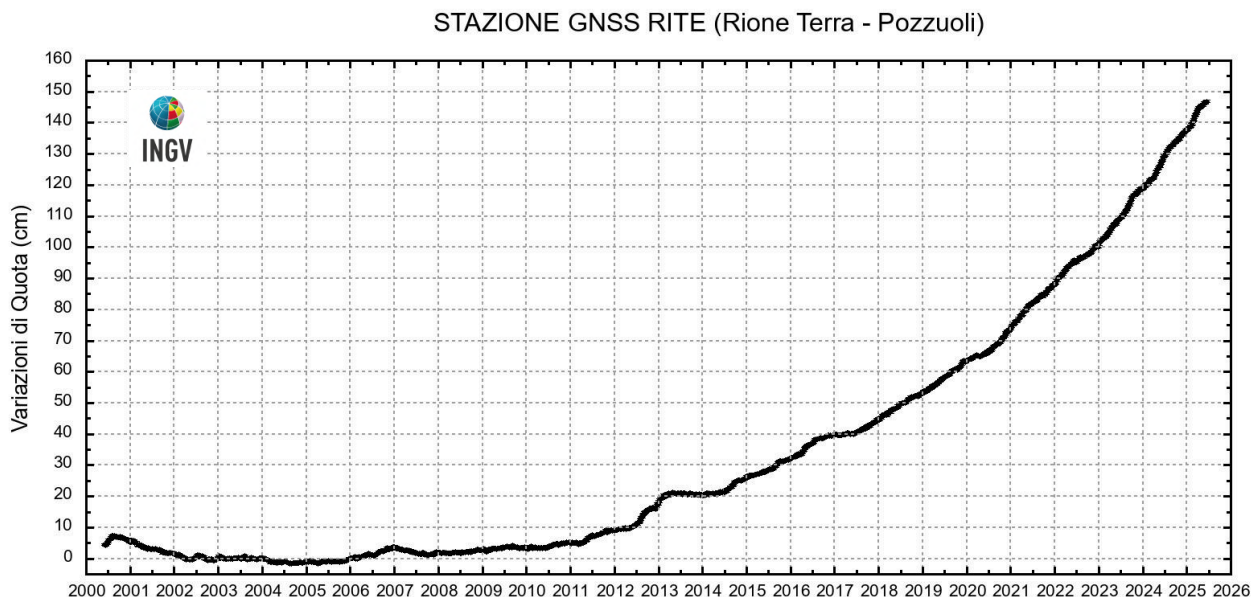
Figura 2.1.4 - Serie temporale delle variazioni settimanali in quota della stazione di RITE (Pozzuoli – Rione Terra) dal 2000 a giugno 2025.
