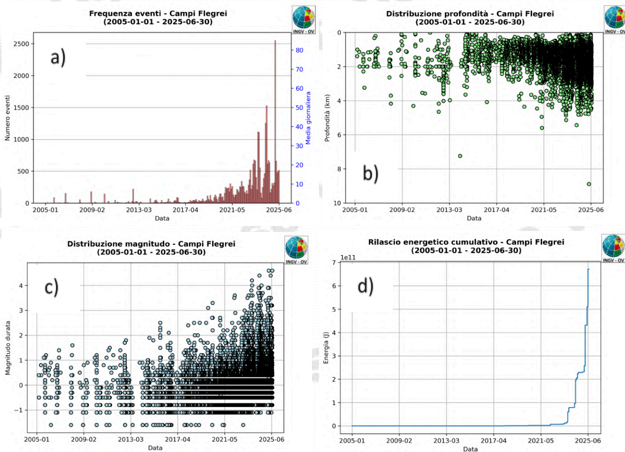
Figura 1.8 - Andamento dei principali parametri sismologici a partire dal 2005: a) frequenza di accadimento mensile; b) profondità ipocentrali; c) magnitudo; d) energia cumulativa.
