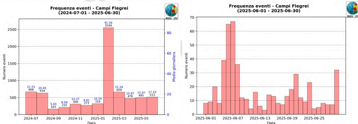
Figura 1.2 - A sinistra numero di eventi registrati ai Campi Flegrei nel corso degli ultimi 12 mesi (in totale 7272), mentre a destra quelli avvenuti nell'ultimo mese (in totale 513).
