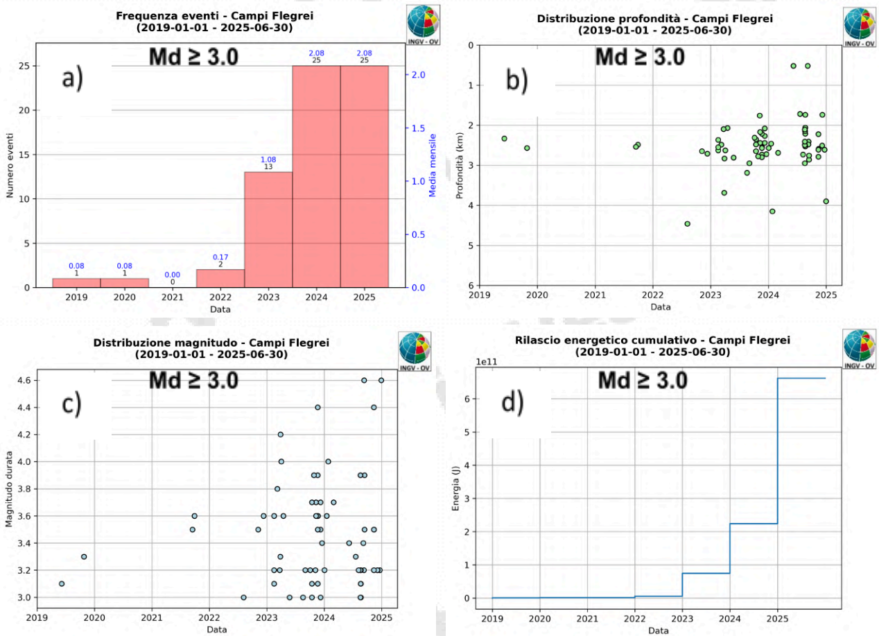
Figura 1.9 - Localizzazioni e andamento dei principali parametri sismologici dei terremoti con M_d \geq 3.0 a partire dal 2019: a) frequenza di accadimento; b) profondità ipocentrali; c) magnitudo; d) energia cumulativa.
