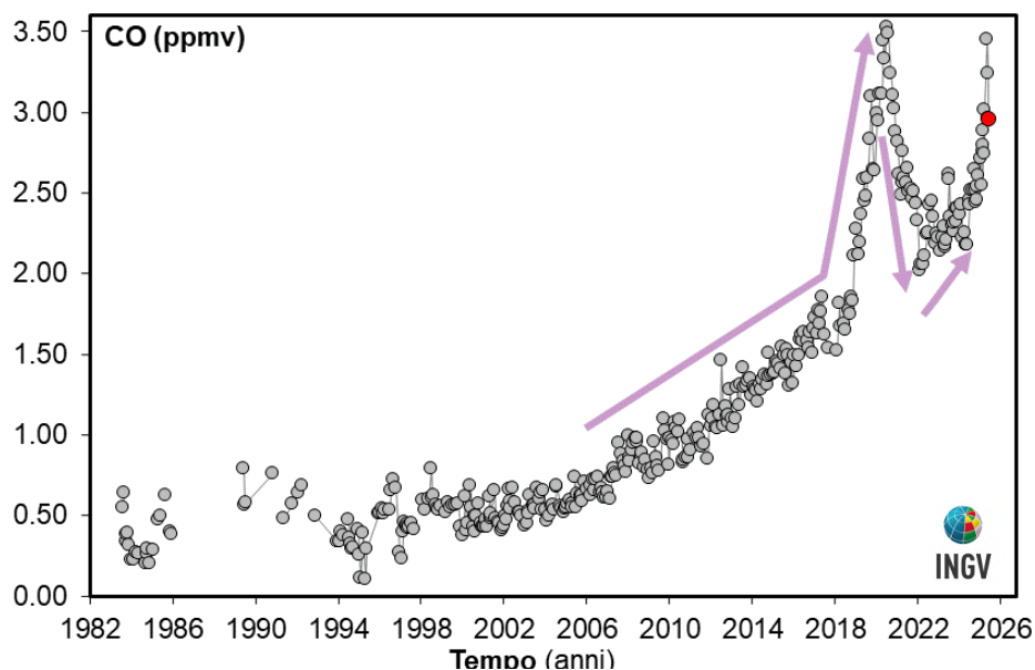
Figura 4.3 – Variazioni della concentrazione di monossido di carbonio (CO) misurato alla fumarola BG a partire dal 1983. Con il simbolo rosso sono evidenziati i campioni di giugno 2025. In generale alti contenuti di CO caratterizzano sistemi vulcanici a elevata temperatura, mentre fumarole alimentate da sistemi idrotermali mostrano concentrazioni più basse, in tali sistemi un aumento delle concentrazioni di CO può riflettere un incremento delle condizioni di pressione e temperatura.
