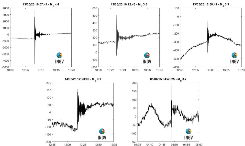
Figura 2.5.3 - Variazioni cosismiche ad alta frequenza registrate dal dilatometro installato a Quarto in concomitanza degli eventi di M_d \geq 3.0 avvenuti nel periodo di analisi.
