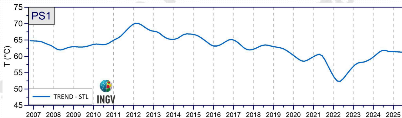
Figura 3.1.4 - Stazione PS1: Trend a lungo termine dei valori di temperatura massima rilevati nelle immagini IR ottenuto mediante applicazione dell'algoritmo STL.
