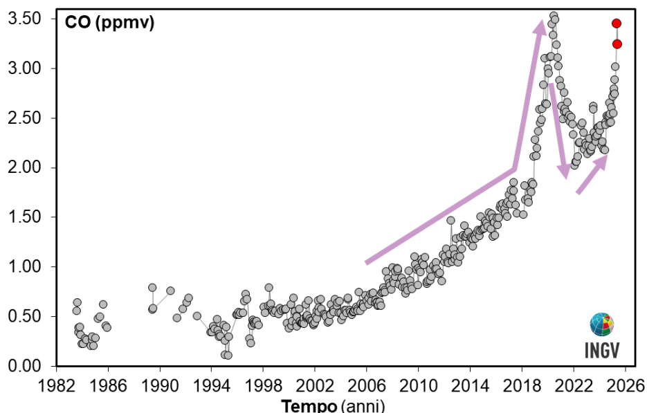
Figura 4.3 – Variazioni della concentrazione di monossido di carbonio (CO) misurato alla fumarola BG a partire dal 1983. Con il simbolo rosso sono evidenziati i campioni di maggio 2025. In generale alti contenuti di CO caratterizzano sistemi vulcanici a elevata temperatura, mentre fumarole alimentate da sistemi idrotermali mostrano concentrazioni più basse, in tali sistemi un aumento delle concentrazioni di CO può riflettere un incremento delle condizioni di pressione e temperatura.
