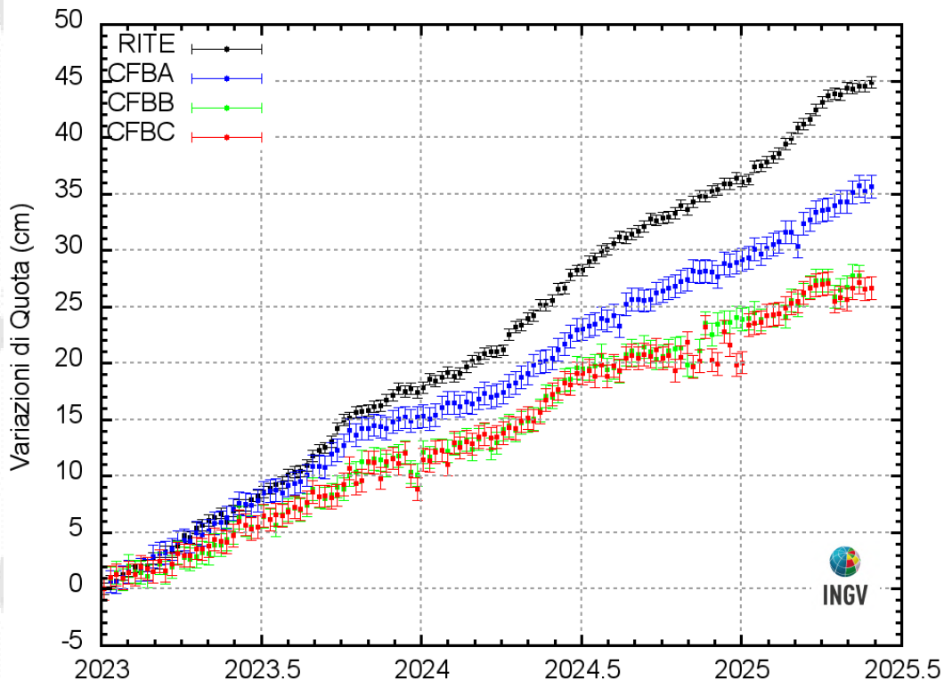
Figura 2.1.7 – Serie temporali delle variazioni settimanali in quota delle stazioni GNSS dell'infrastruttura marina MEDUSA nell'intervallo gennaio 2023 - maggio 2025, confrontate con quella della stazione RITE
