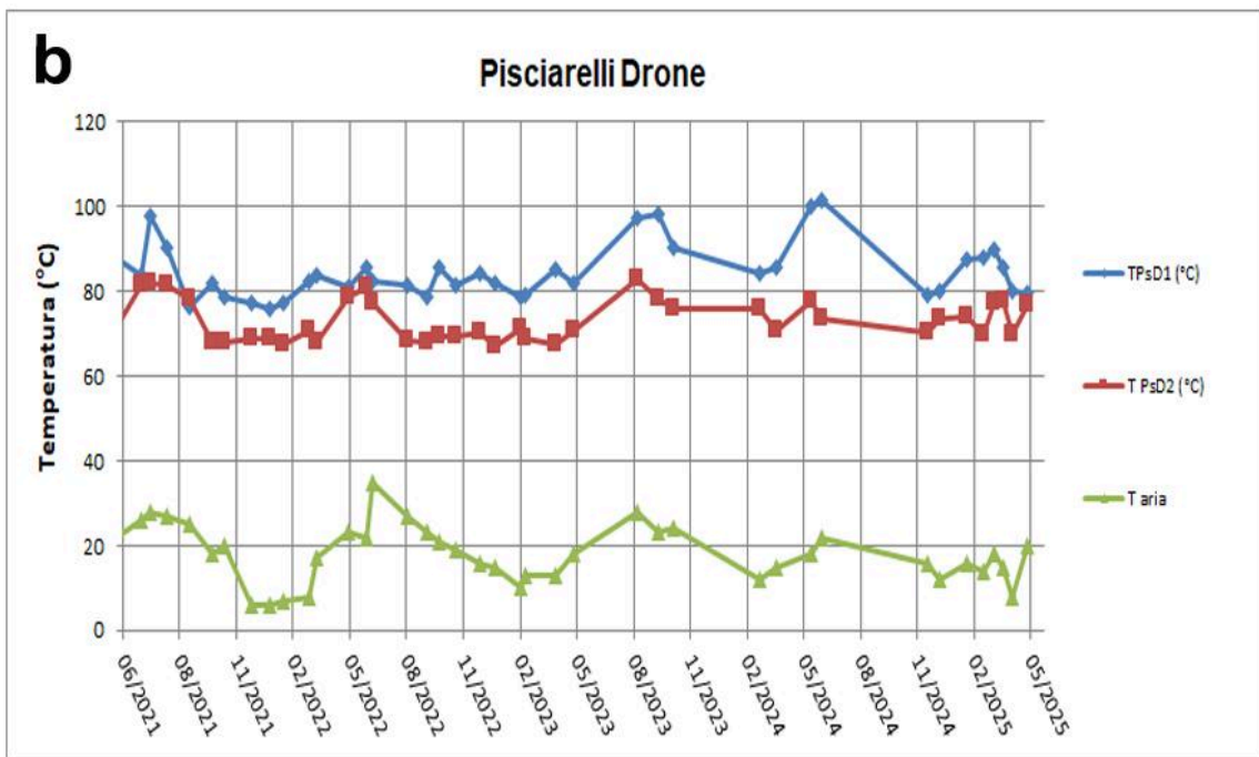
Figura 3.2.2 – Immagine termica, rilevata nel mese di maggio 2025, dell’area denominata Ps4 (Fig.3.2.1b) (a) e valori massimi di temperatura (T) delle aree a maggiore anomalia termica (PsD1 e PsD2) confrontati con la temperatura dell’aria (Taria) misurata nel momento del rilievo termico da giugno 2021 a maggio 2025 (b).
