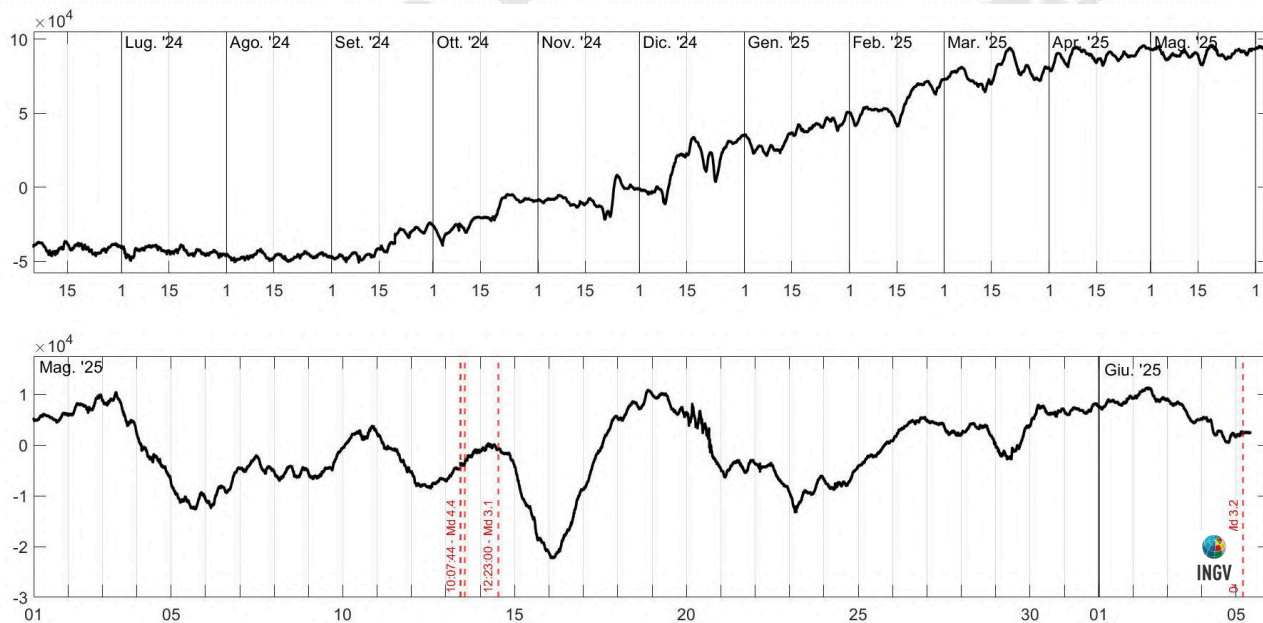
Figura 2.5.2 - In alto: Strain registrato nell'ultimo anno alla stazione di Quarto, dalle 00:00 UTC del 5/6/2024 alle 10:00 UTC del giorno 5/6/2025. In basso: Strain registrato nell'ultimo mese, dalle 00:00 UTC del giorno 1/5/2025 alle 10:00 UTC del giorno 5/6/2025. Le linee verticali rosse indicano l'occorrenza di eventi sismici con magnitudo maggiore di 3.
