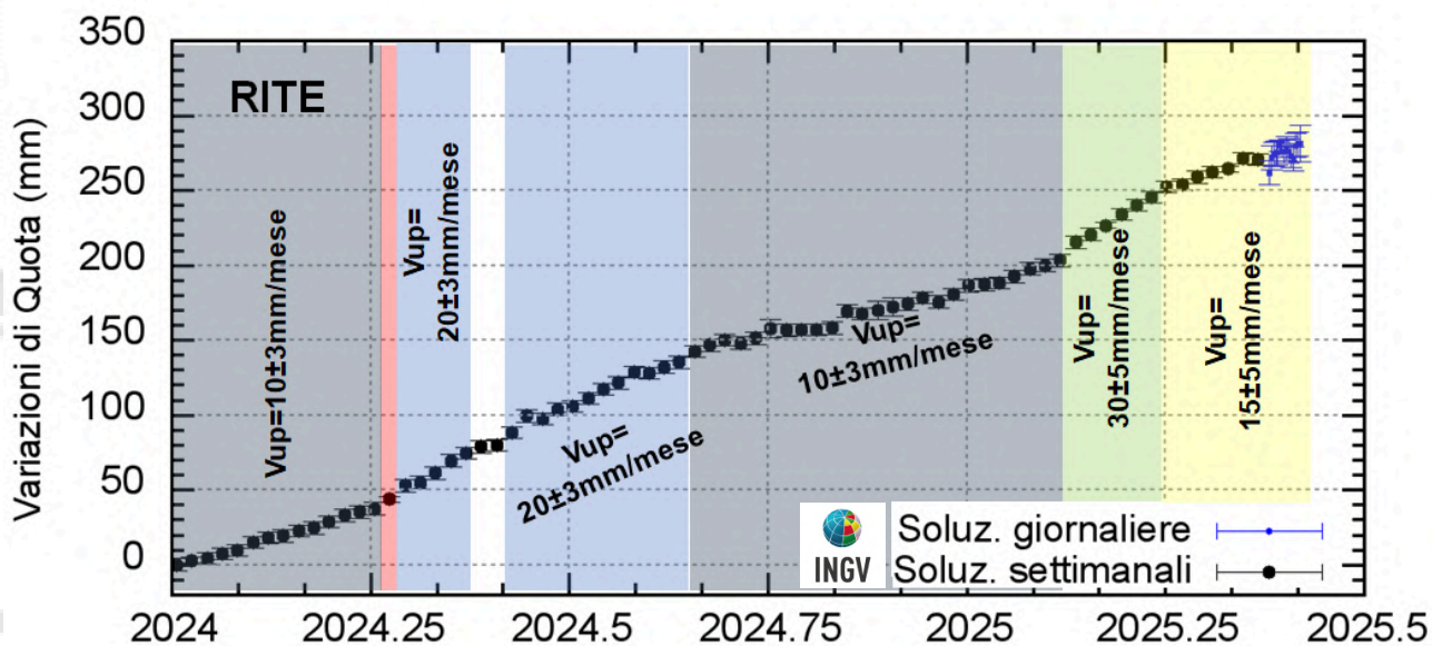
Figura 2.1.2 - Serie temporale delle variazioni in quota della stazione GNSS di RITE dal 01/01/2024 al 02/06/2025. Elaborazione dati in modalità differenziale singola baseline con software GNSS Spider.
