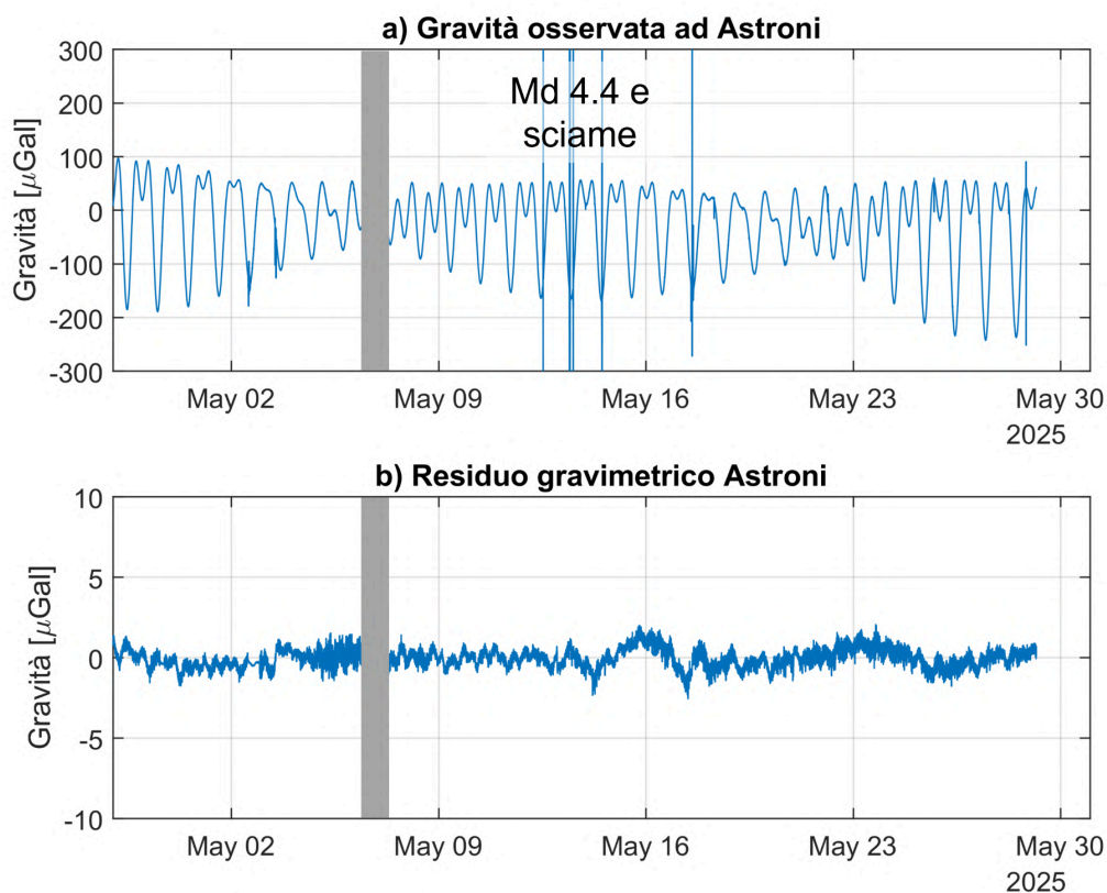
Figura 2.4.1 a: serie temporale (risoluzione temporale 1 minuto) raw registrata dal gPhone. Si osserva il contributo dominante delle maree. b: serie residua di gravità. La banda verticale grigia marca un periodo di interruzione dell'acquisizione dati.
