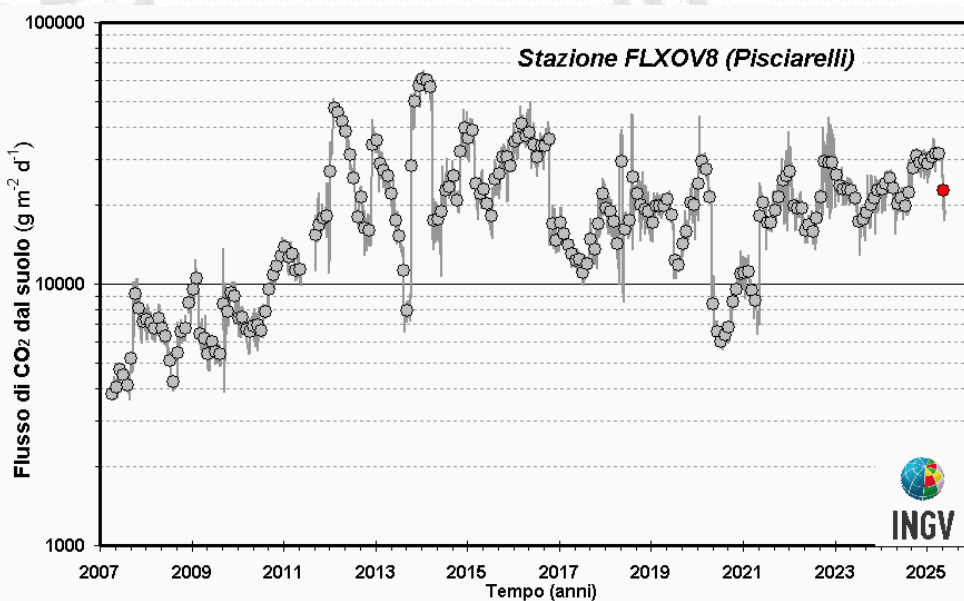
Figura 4.14 - Medie giornaliere (linea) e medie mensili (cerchi) dei flussi di CO 2 misurati dalla stazione automatica a Pisciarelli. È da evidenziare il continuo trend d'aumento nel tempo a partire dal 2007 del flusso CO 2 . La media dei flussi relativa al mese di maggio 2025 è riportata con il simbolo rosso. Il flusso di CO 2 dal suolo misurato dalla stazione FLXOV8, che dal mese di aprile 2020 fino a maggio 2021 aveva mostrato una diminuzione dei valori, negli ultimi periodi ha mostrato valori simili a quelli registrati nei primi mesi del 2020.
