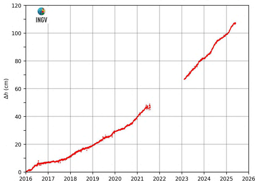
Figura 2.3.2 – Movimenti verticali del suolo, nel periodo gennaio 2016 – maggio 2025, ottenuti dall'analisi dei dati acquisiti dalla stazione mareografica di Pozzuoli Porto (POPT), area centrale della caldera Flegrea. Le variazioni, riportate in cm, rappresentano le medie giornaliere e sono riferite alla stazione mareografica di Napoli, molo San Vincenzo (NAMM).
