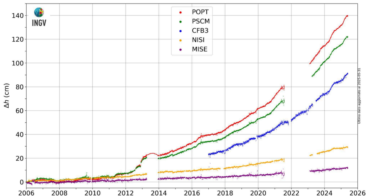
Figura 2.3.4 - Movimenti verticali del suolo nel periodo gennaio 2006 – maggio 2025, ottenuti dall'analisi dei dati acquisiti da tutte le stazioni mareografiche dell'area della caldera Flegrea. Le variazioni, riportate in cm, rappresentano le medie giornaliere e sono tutte riferite alla stazione mareografica di Napoli, molo San Vincenzo (NAMM).
