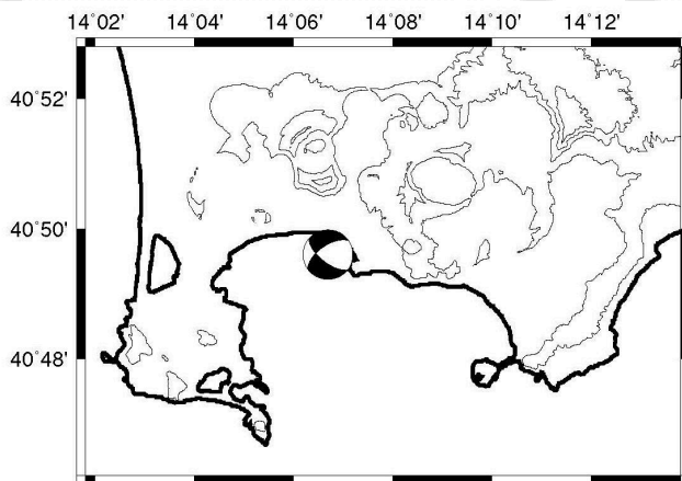
Figura 1.7 - Localizzazione ipocentrale e meccanismo focale dell'evento del 13/05/2025 alle ore 10:07 UTC di M_d 4.4 \pm 0.3 .
