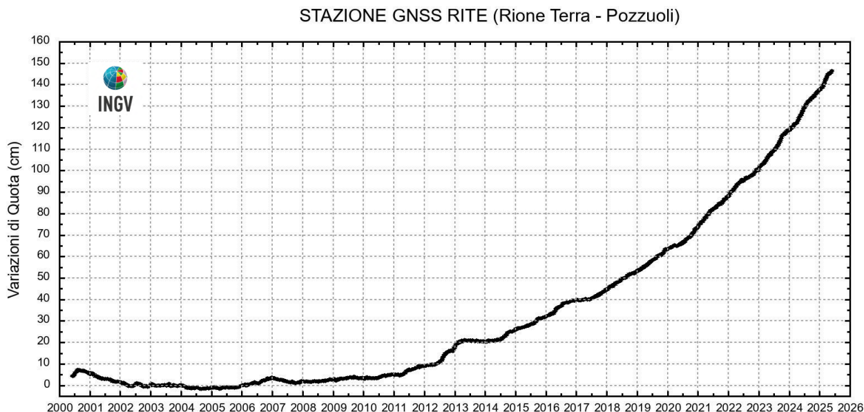
Figura 2.1.4 - Serie temporale delle variazioni settimanali in quota della stazione di RITE (Pozzuoli – Rione Terra) dal 2000 a maggio 2025.
