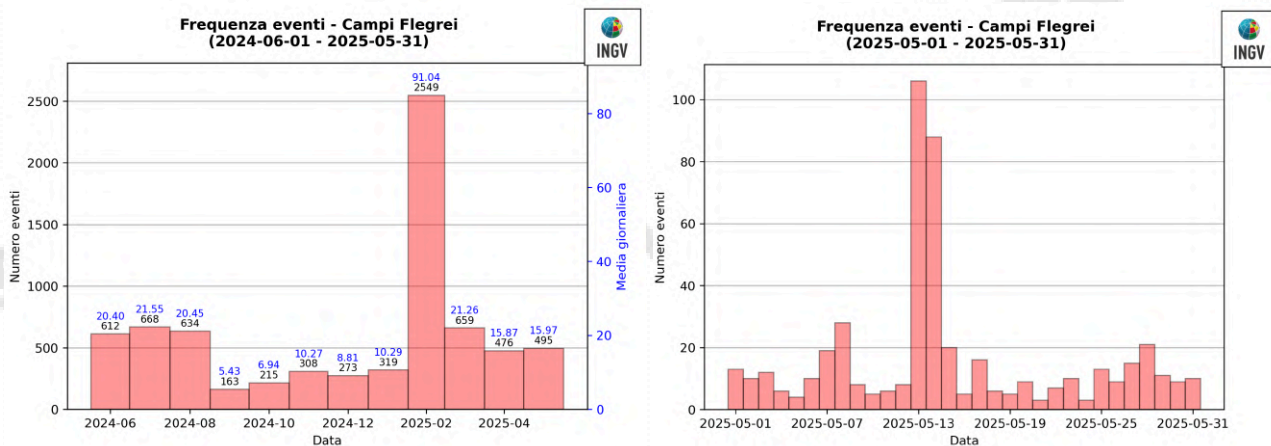
Figura 1.2 - A sinistra numero di eventi registrati ai Campi Flegrei nel corso degli ultimi 12 mesi (in totale 7371), mentre a destra quelli avvenuti nell'ultimo mese (in totale 495).
