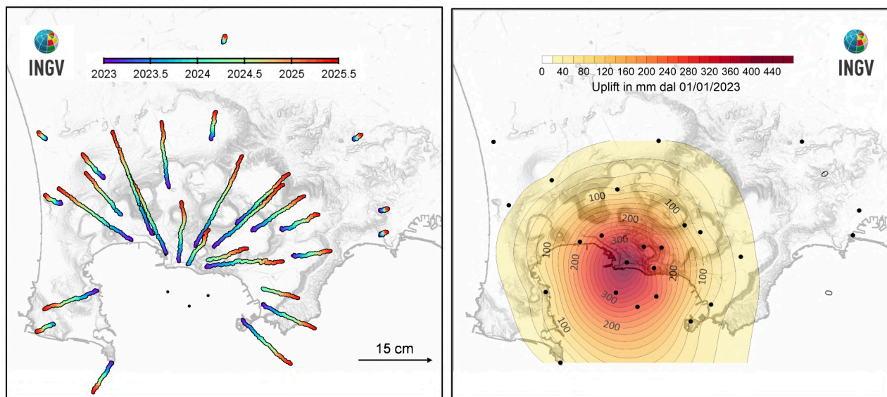
Figura 2.1.5 - Mappa degli spostamenti GNSS orizzontali (a) e verticali (b) registrati nell'area flegrea da gennaio 2023 a maggio 2025.
