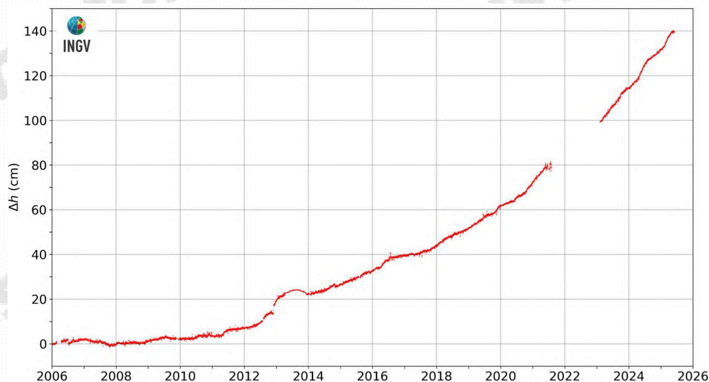
Figura 2.3.3 - Movimenti verticali del suolo nel periodo gennaio 2006 – maggio 2025, ottenuti dall'analisi dei dati acquisiti dalla stazione mareografica di Pozzuoli Porto (POPT) (area centrale della caldera Flegrea). Le variazioni, riportate in cm, rappresentano le medie giornaliere e sono riferite alla stazione mareografica di Napoli, molo San Vincenzo (NAMM).
