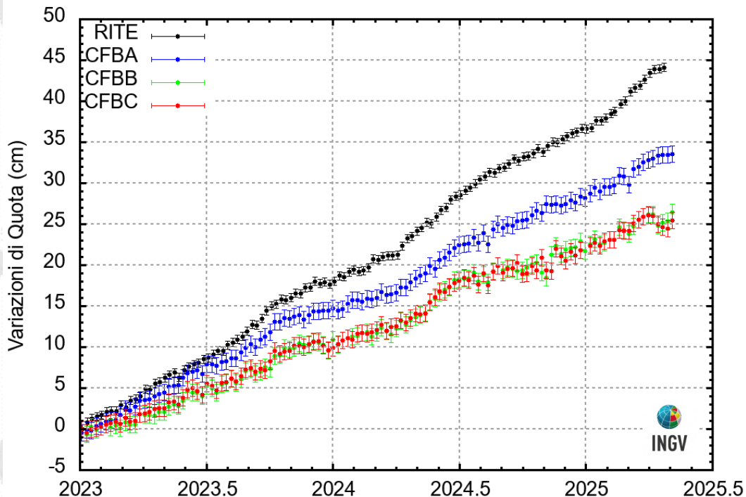
Figura 2.1.7 – Serie temporali delle variazioni settimanali in quota delle stazioni GNSS dell'infrastruttura marina MEDUSA nell'intervallo gennaio 2023 - aprile 2025, confrontate con quella della stazione RITE
