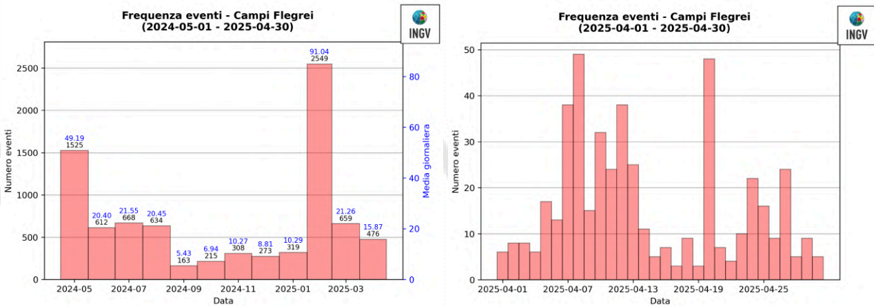
Figura 1.2 - A sinistra numero di eventi registrati ai Campi Flegrei nel corso degli ultimi 12 mesi (in totale 8401), mentre a destra quelli avvenuti nell'ultimo mese (in totale 476).
