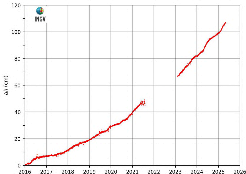
Figura 2.3.2 – Movimenti verticali del suolo, nel periodo gennaio 2016 – aprile 2025, ottenuti dall'analisi dei dati acquisiti dalla stazione mareografica di Pozzuoli Porto (POPT), area centrale della caldera Flegrea. Le variazioni, riportate in cm, rappresentano le medie giornaliere e sono riferite alla stazione mareografica di Napoli, molo San Vincenzo (NAMM).
