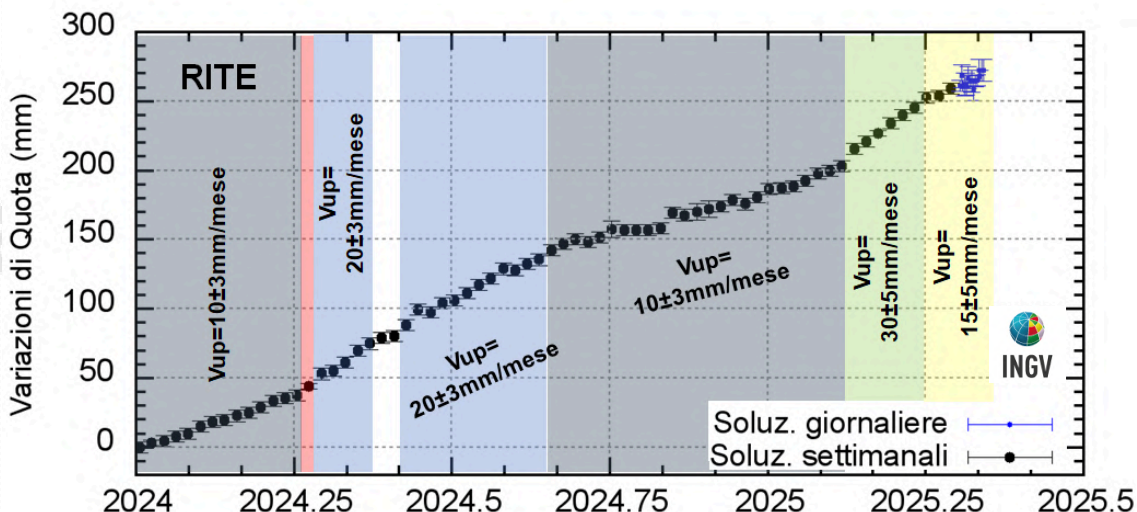
Figura 2.1.2 - Serie temporale delle variazioni in quota della stazione GNSS di RITE dal 01/01/2024 al 05/05/2025. Elaborazione dati in modalità differenziale singola baseline con software GNSS Spider.
