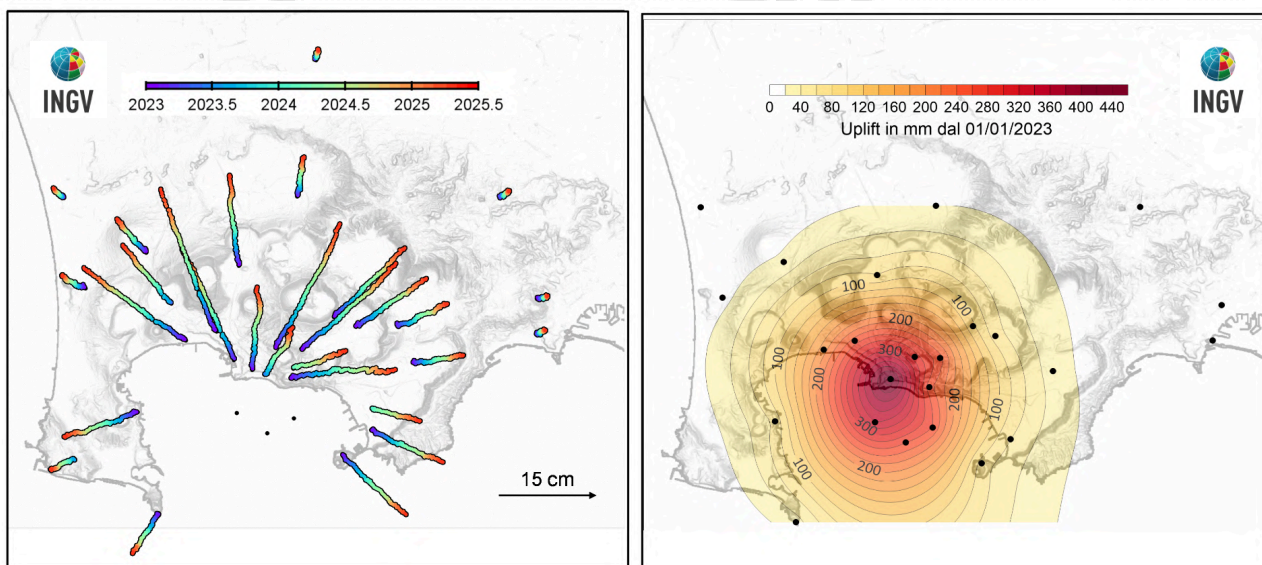
Figura 2.1.5 - Mappa degli spostamenti GNSS orizzontali (a) e verticali (b) registrati nell'area flegrea da gennaio 2023 ad aprile 2025.
