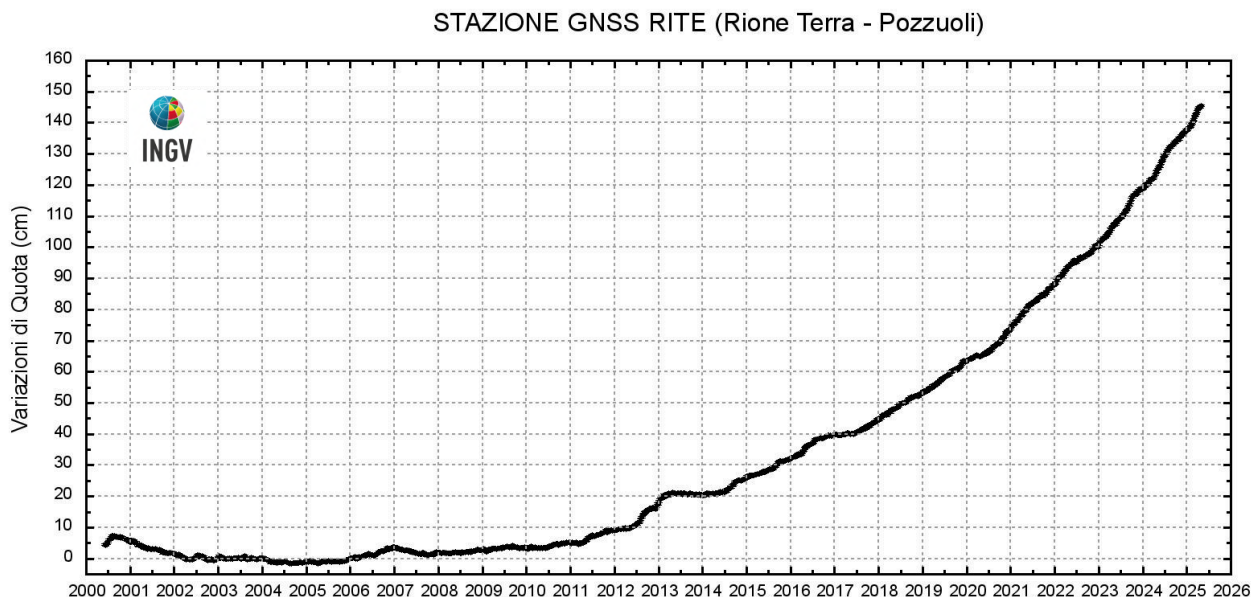
Figura 2.1.4 - Serie temporale delle variazioni settimanali in quota della stazione di RITE (Pozzuoli – Rione Terra) dal 2000 ad aprile 2025.
