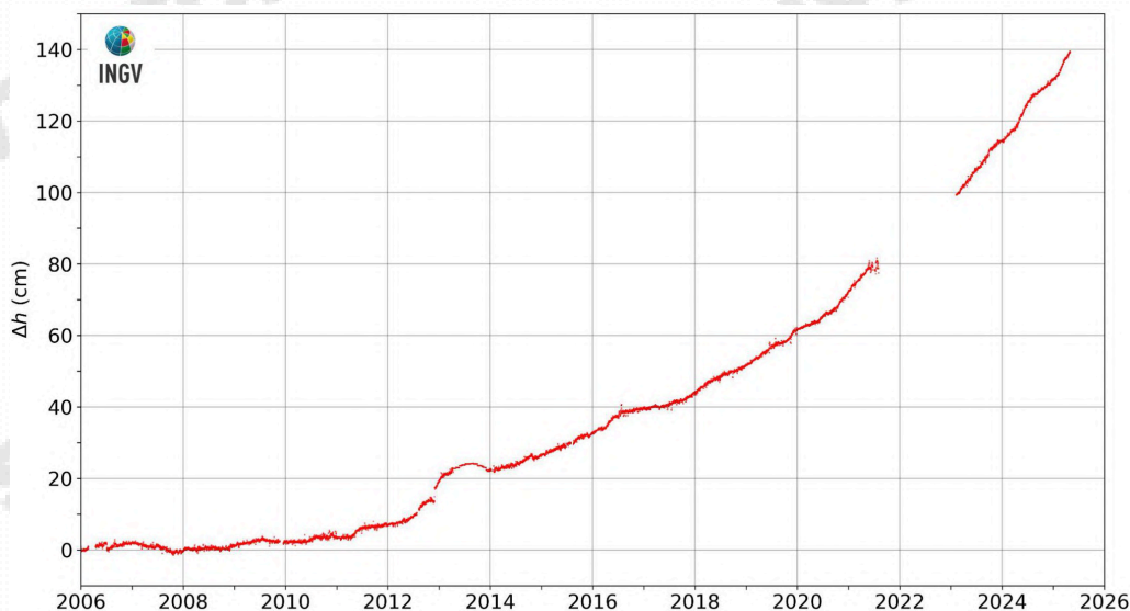
Figura 2.3.3 - Movimenti verticali del suolo nel periodo gennaio 2006 – aprile 2025, ottenuti dall'analisi dei dati acquisiti dalla stazione mareografica di Pozzuoli Porto (POPT) (area centrale della caldera Flegrea). Le variazioni, riportate in cm, rappresentano le medie giornaliere e sono riferite alla stazione mareografica di Napoli, molo San Vincenzo (NAMM).
