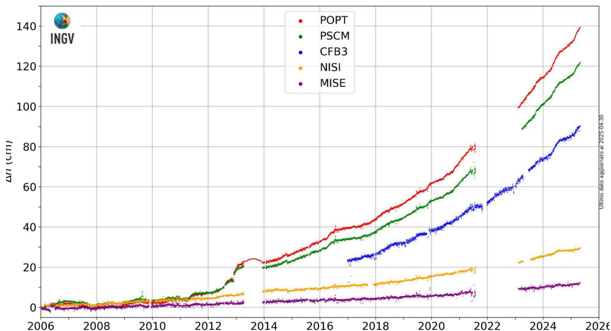
Figura 2.3.4 - Movimenti verticali del suolo nel periodo gennaio 2006 – aprile 2025, ottenuti dall'analisi dei dati acquisiti da tutte le stazioni mareografiche dell'area della caldera Flegrea. Le variazioni, riportate in cm, rappresentano le medie giornaliere e sono tutte riferite alla stazione mareografica di Napoli, molo San Vincenzo (NAMM).
