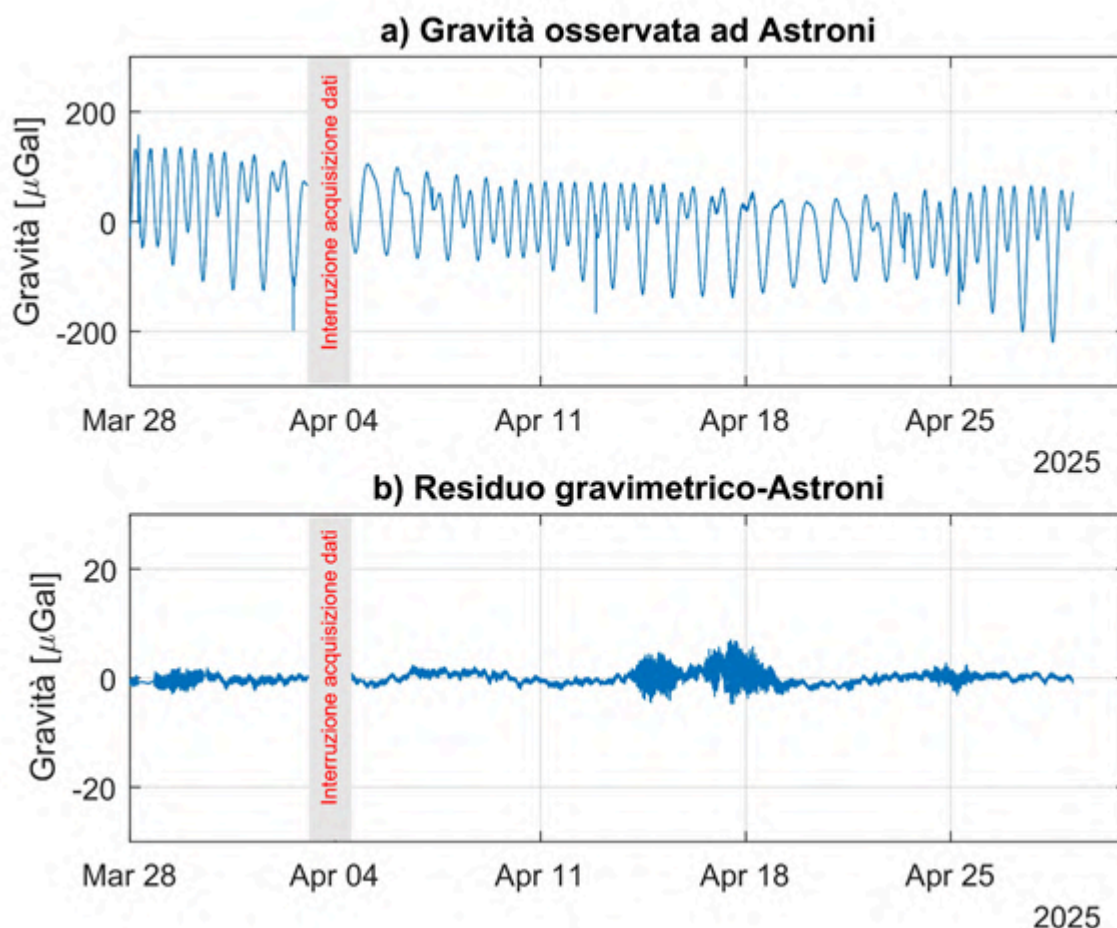
Figura 2.4.1 a: serie temporale (risoluzione temporale 1 minuto) raw registrata dal gPhone. Si osserva il contributo dominante delle maree.; b: serie residua di gravità.
