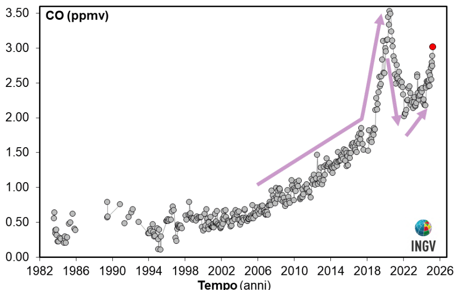
Figura 4.3 – Variazioni della concentrazione di monossido di carbonio (CO) misurato alla fumarola BG a partire dal 1983. Con il simbolo rosso è evidenziato il campione di aprile 2025. In generale alti contenuti di CO caratterizzano sistemi vulcanici a elevata temperatura, mentre fumarole alimentate da sistemi idrotermali mostrano concentrazioni più basse, in tali sistemi un aumento delle concentrazioni di CO può riflettere un incremento delle condizioni di pressione e temperatura.
