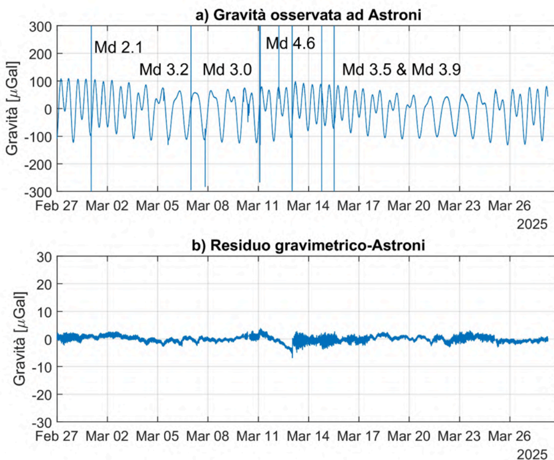
Figura 2.4.1 a: serie temporale (risoluzione temporale 1 minuto) raw registrata dal gPhone. Si osserva il contributo dominante delle maree e disturbi legati all'attività sismica nei Campi Flegrei. b: serie residua di gravità.
