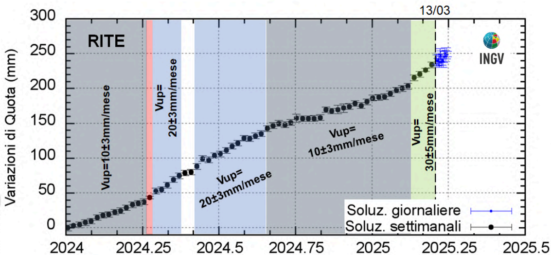
Figura 2.1.2 - Serie temporale delle variazioni in quota della stazione GNSS di RITE dal 01/01/2024 al 31/03/2025. Elaborazione dati in modalità differenziale singola baseline con software GNSS Spider.
