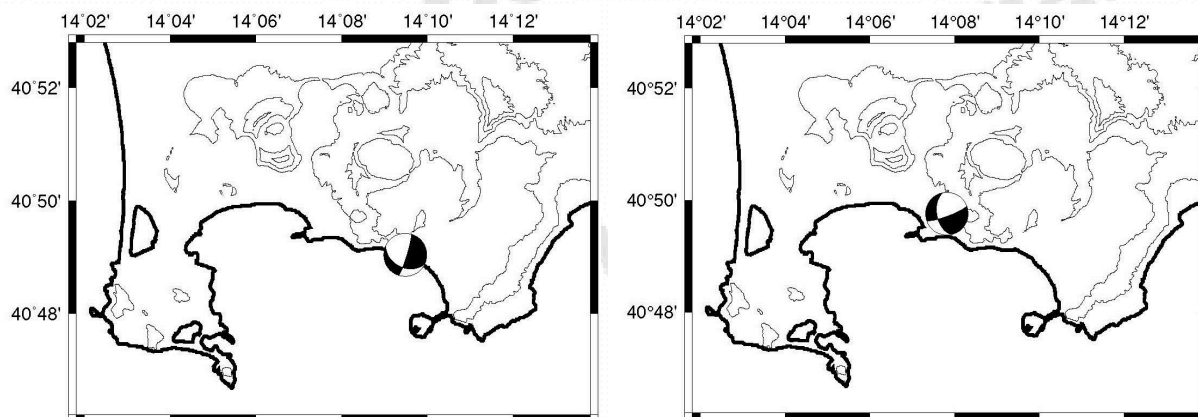
Figura 1.7 - Localizzazioni e meccanismi focali degli eventi del 13/03/2025 alle 00:25 UTC di M_d 4.6(\pm 0.3) (a sinistra) e del 15/03/2025 alle 12:32 UTC di M_d 3.9(\pm 0.3) (a destra).
