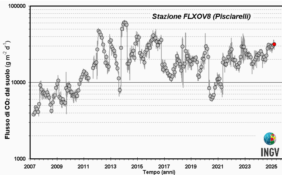
Figura 4.15 - Medie giornaliere (linea) e medie mensili (cerchi) dei flussi di CO 2 misurati dalla stazione automatica a Pisciarelli. È da evidenziare il continuo trend d'aumento nel tempo a partire dal 2007 del flusso CO 2 . La media dei flussi relativa al mese di marzo 2025 è riportata con il simbolo rosso. Il flusso di CO 2 dal suolo misurato dalla stazione FLXOV8, che dal mese di aprile 2020 fino a maggio 2021 aveva mostrato una diminuzione dei valori, negli ultimi periodi ha mostrato valori simili a quelli registrati nei primi mesi del 2020.
