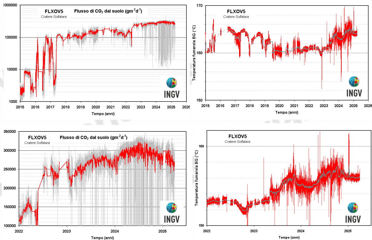
Figura 4.12 – Valori del flusso di CO 2 dal suolo e della temperatura della fumarola BG misurati dalla stazione FLXOV5 installata nel cratere della Solfatara, a pochi metri dalla fumarola principale BG. I valori di flusso di CO 2 dal suolo mostrano, in generale, un significativo incremento a partire dal 2016 (la linea rossa si riferisce alle medie giornaliere). Nei cronogrammi in basso sono riportati i valori di flusso di CO 2 e temperatura a partire da gennaio 2022.
