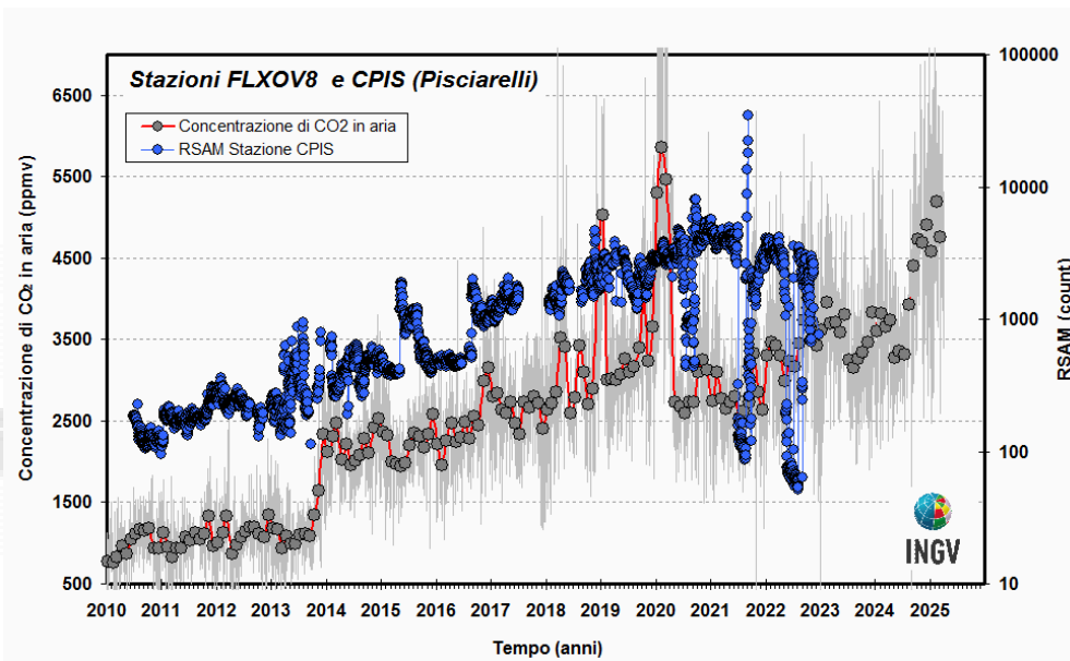
Figura 4.16 - Cronogramma delle medie giornaliere (linea) e medie mensili (cerchi) della concentrazione di CO 2 registrata in aria con frequenza bioraria dalla stazione geochimica per la misura del flusso di CO 2 dal suolo di Pisciarelli (FLXOV8). Nel cronogramma è riportata anche la serie temporale dell'ampiezza del tremore fumarolico su base giornaliera registrata dalla stazione sismica CPIS fino al 2023, installata a pochi metri dalla fumarola principale. Questi parametri risultano strettamente correlati tra di loro e all'intensità dell'attività idrotermale (Chiodini et al., 2017, Giudicepietro et al., 2019). E' da evidenziare il continuo trend d'aumento nel tempo delle concentrazioni di CO 2 in aria e dell'ampiezza del tremore fumarolico dal 2013 al 2021, successivamente i trend mostrano una diminuzione per poi mostrare negli ultimi periodo un nuovo aumento.
