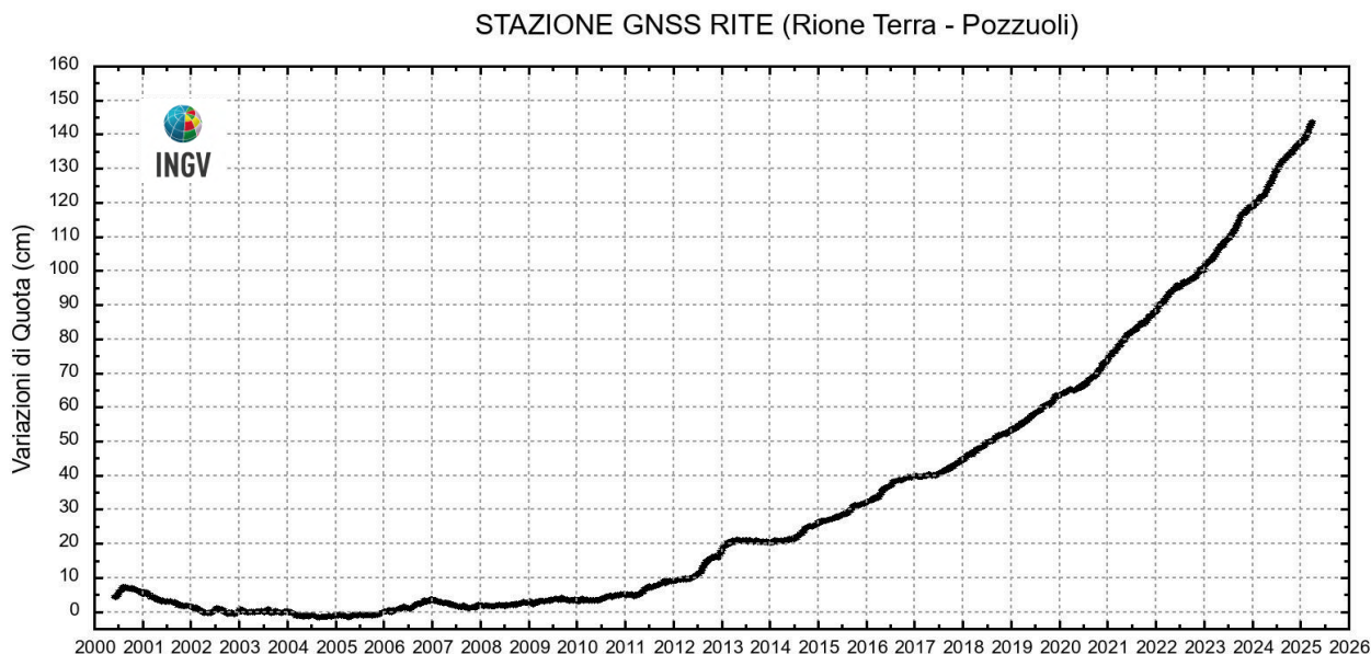
Figura 2.1.4 - Serie temporale delle variazioni settimanali in quota della stazione di RITE (Pozzuoli – Rione Terra) dal 2000 a marzo 2025.
