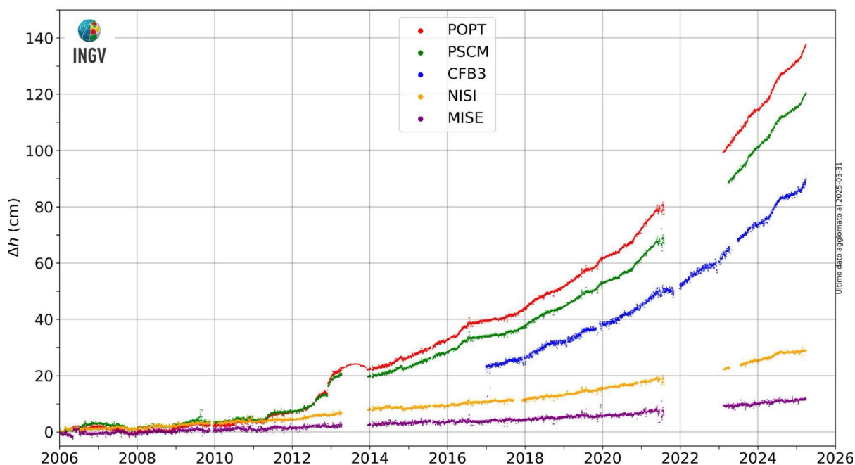
Figura 2.3.4 - Movimenti verticali del suolo nel periodo gennaio 2006 – marzo 2025, ottenuti dall'analisi dei dati acquisiti da tutte le stazioni mareografiche dell'area della caldera Flegrea. Le variazioni, riportate in cm, rappresentano le medie giornaliere e sono tutte riferite alla stazione mareografica di Napoli, molo San Vincenzo (NAMM).
