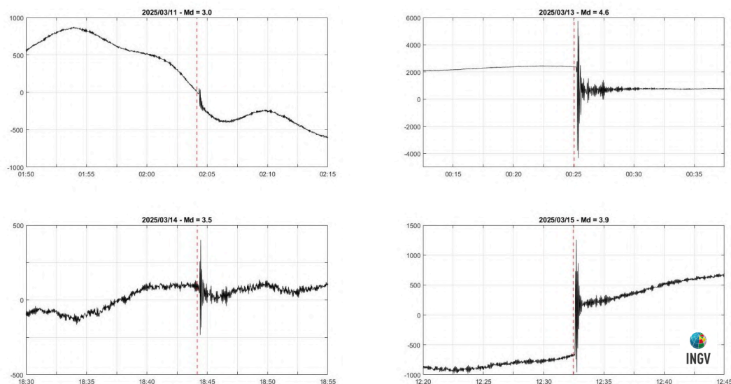
Figura 2.5.3 Dettaglio delle variazioni registrate dal dilatometro CQUE in concomitanza con gli eventi sismici di Magnitudo maggiore di 3.0 avvenuti durante il mese di marzo 2025. Le linee verticali rosse tratteggiate indicano l'onset degli eventi sismici registrati.
