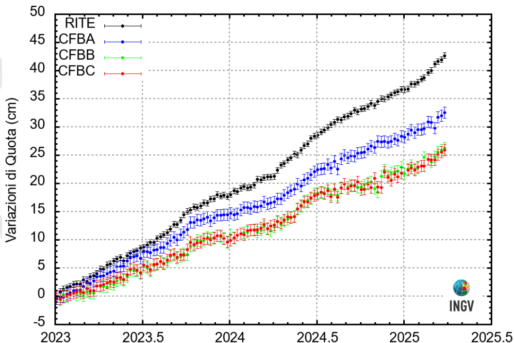
Figura 2.1.7 – Serie temporali delle variazioni settimanali in quota delle stazioni GNSS dell'infrastruttura marina MEDUSA nell'intervallo gennaio 2023 - marzo 2025, confrontate con quella della stazione RITE
