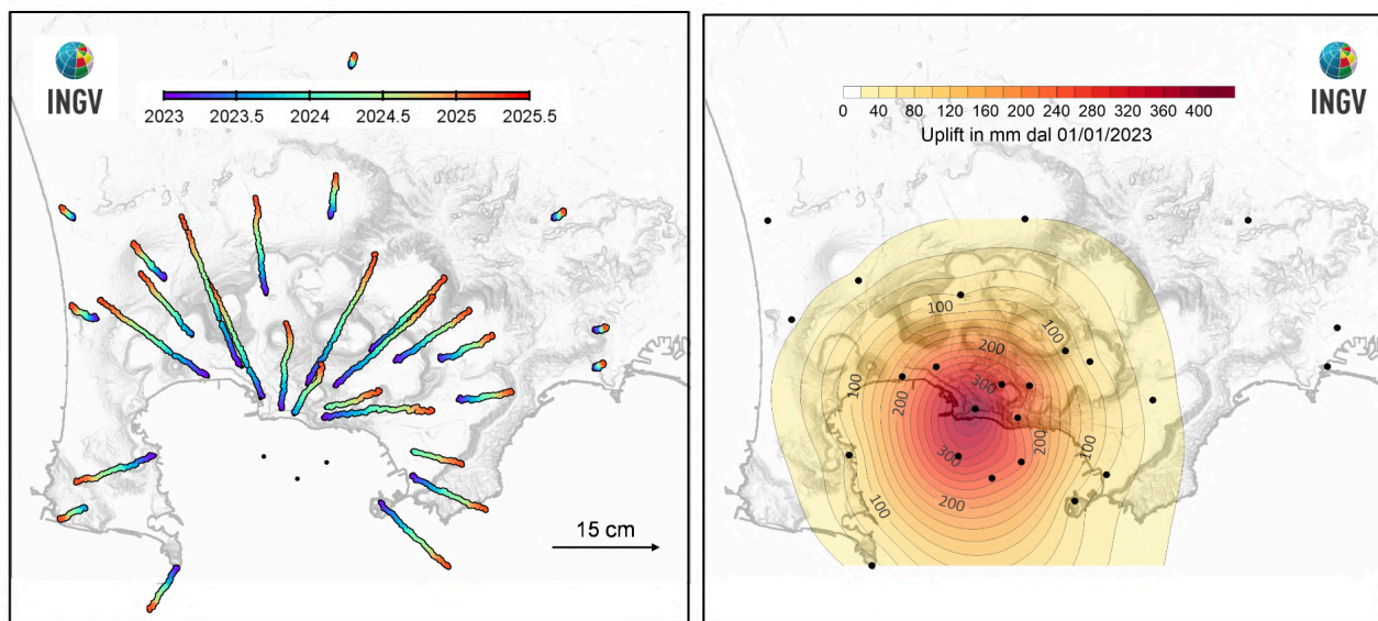
Figura 2.1.5 - Mappa degli spostamenti GNSS orizzontali (a) e verticali (b) registrati nell'area flegrea da gennaio 2023 a marzo 2025.
