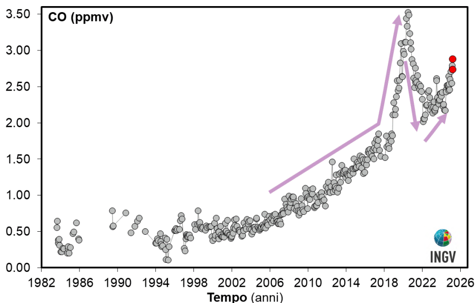
Figura 4.3 – Variazioni della concentrazione di monossido di carbonio (CO) misurato alla fumarola BG a partire dal 1983. Con il simbolo rosso sono evidenziati i campioni di marzo 2025. In generale alti contenuti di CO caratterizzano sistemi vulcanici a elevata temperatura, mentre fumarole alimentate da sistemi idrotermali mostrano concentrazioni più basse, in tali sistemi un aumento delle concentrazioni di CO può riflettere un incremento delle condizioni di pressione e temperatura.
