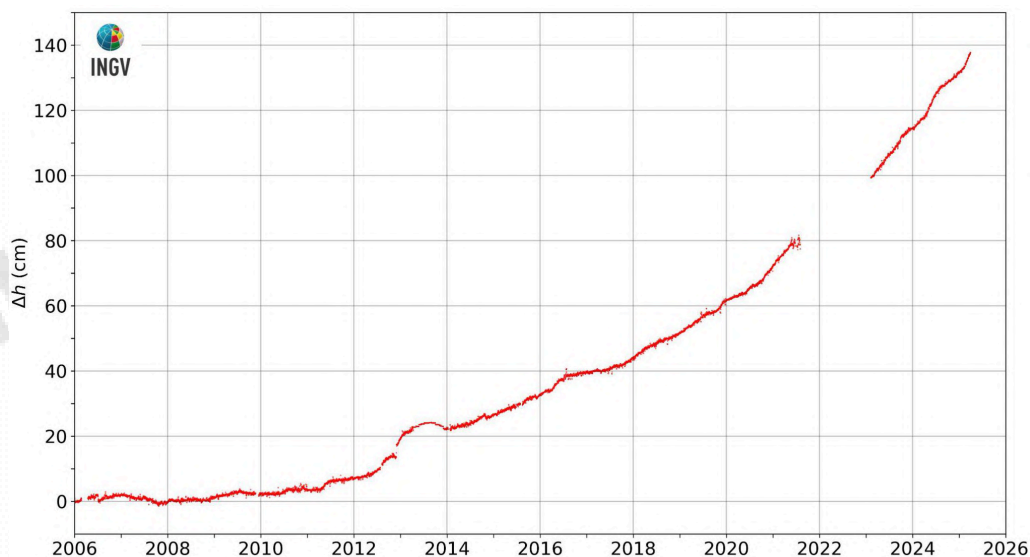
Figura 2.3.3 - Movimenti verticali del suolo nel periodo gennaio 2006 – marzo 2025, ottenuti dall'analisi dei dati acquisiti dalla stazione mareografica di Pozzuoli Porto (POPT) (area centrale della caldera Flegrea). Le variazioni, riportate in cm, rappresentano le medie giornaliere e sono riferite alla stazione mareografica di Napoli, molo San Vincenzo (NAMM).
