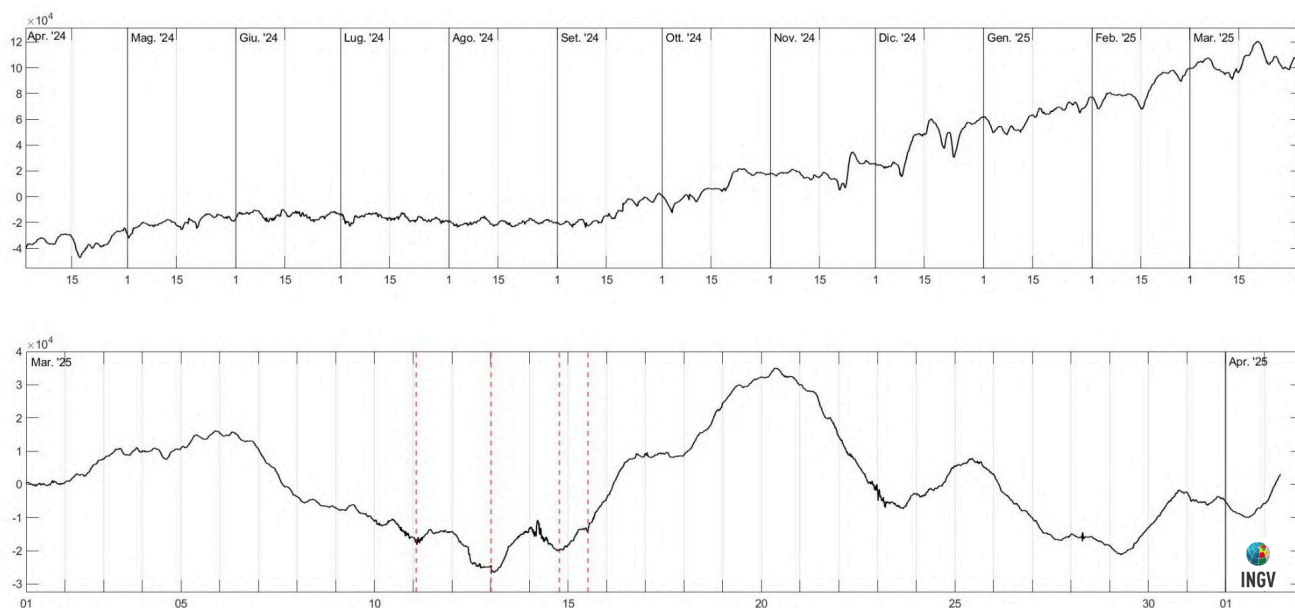
Figura 2.5.2 - In alto: Strain registrato nell'ultimo anno, dalle 00:00 UTC del 2/4/2024 alle 12:00 UTC del giorno 2/4/2025. In basso: Strain registrato nell'ultimo mese, dalle 00:00 UTC del giorno 1/3/2025 alle 12:00 UTC del giorno 2/4/2025. Le linee verticali rosse indicano l'occorrenza di eventi sismici con magnitudo maggiore di 3.
