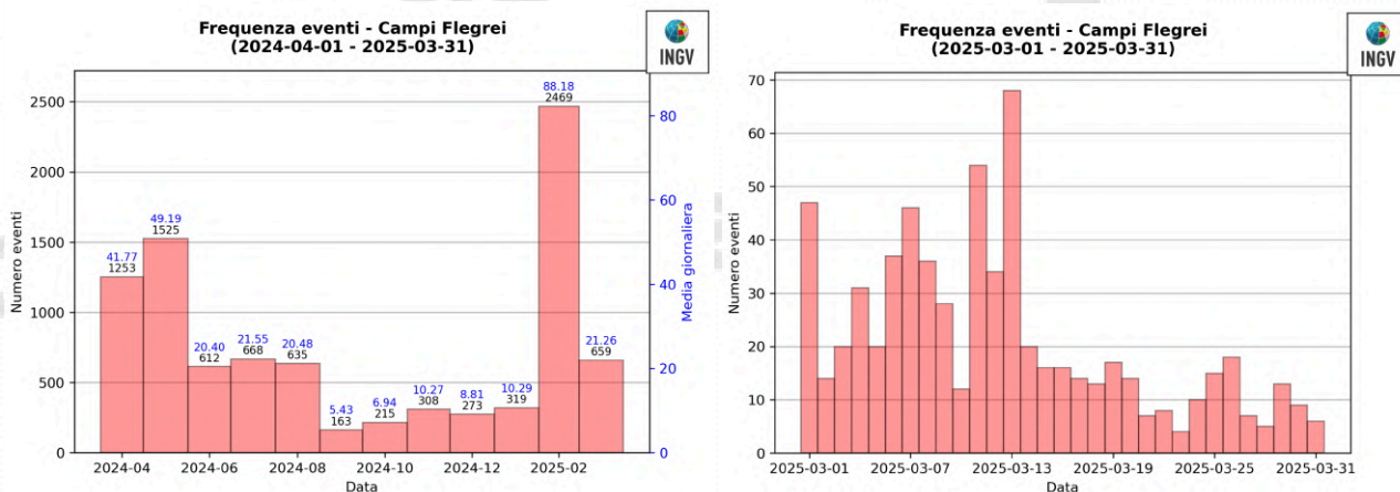
Figura 1.2 - A sinistra numero di eventi registrati ai Campi Flegrei nel corso degli ultimi 12 mesi (in totale 9099), mentre a destra quelli avvenuti nell'ultimo mese (in totale 659).
