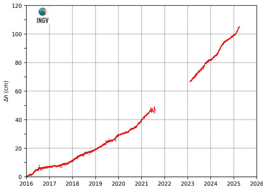
Figura 2.3.2 – Movimenti verticali del suolo, nel periodo gennaio 2016 – marzo 2025, ottenuti dall'analisi dei dati acquisiti dalla stazione mareografica di Pozzuoli Porto (POPT), area centrale della caldera Flegrea. Le variazioni, riportate in cm, rappresentano le medie giornaliere e sono riferite alla stazione mareografica di Napoli, molo San Vincenzo (NAMM).
