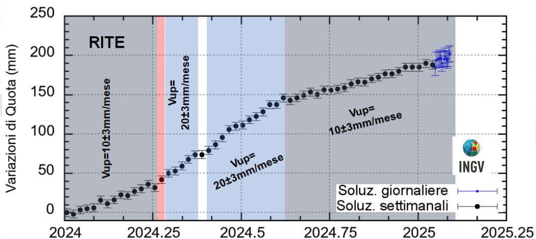
Figura 2.1.2 - Serie temporale delle variazioni in quota della stazione GNSS di RITE dal 01/01/2024 al 02/02/2025. Elaborazione dati in modalità Precise Point Positioning con software PRIDE PPP-AR (Geng et al., 2019).
