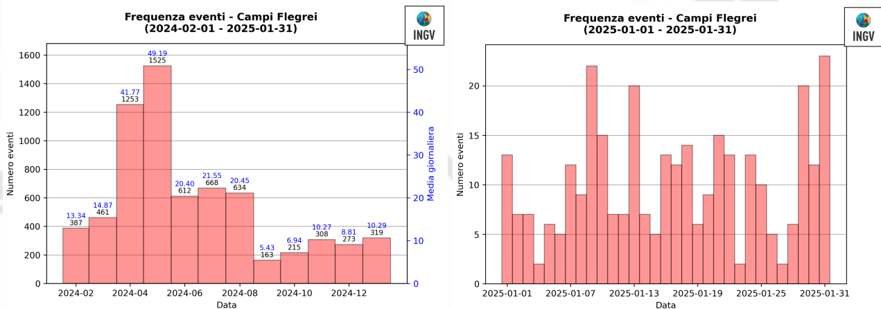
Figura 1.2 - A sinistra numero di eventi registrati ai Campi Flegrei nel corso degli ultimi 12 mesi (in totale 6818), mentre a destra quelli avvenuti nell'ultimo mese (in totale 319).
