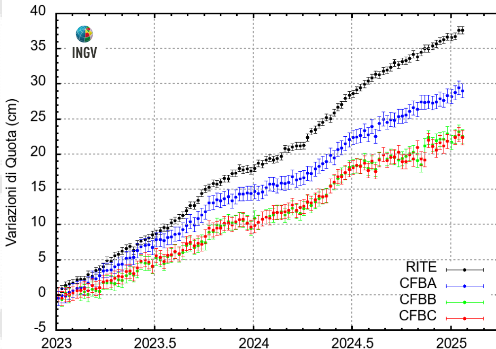
Figura 2.1.7 – Serie temporali delle variazioni settimanali in quota delle stazioni GNSS dell'infrastruttura marina MEDUSA nell'intervallo gennaio 2023 - gennaio 2025, confrontate con quella della stazione RITE
