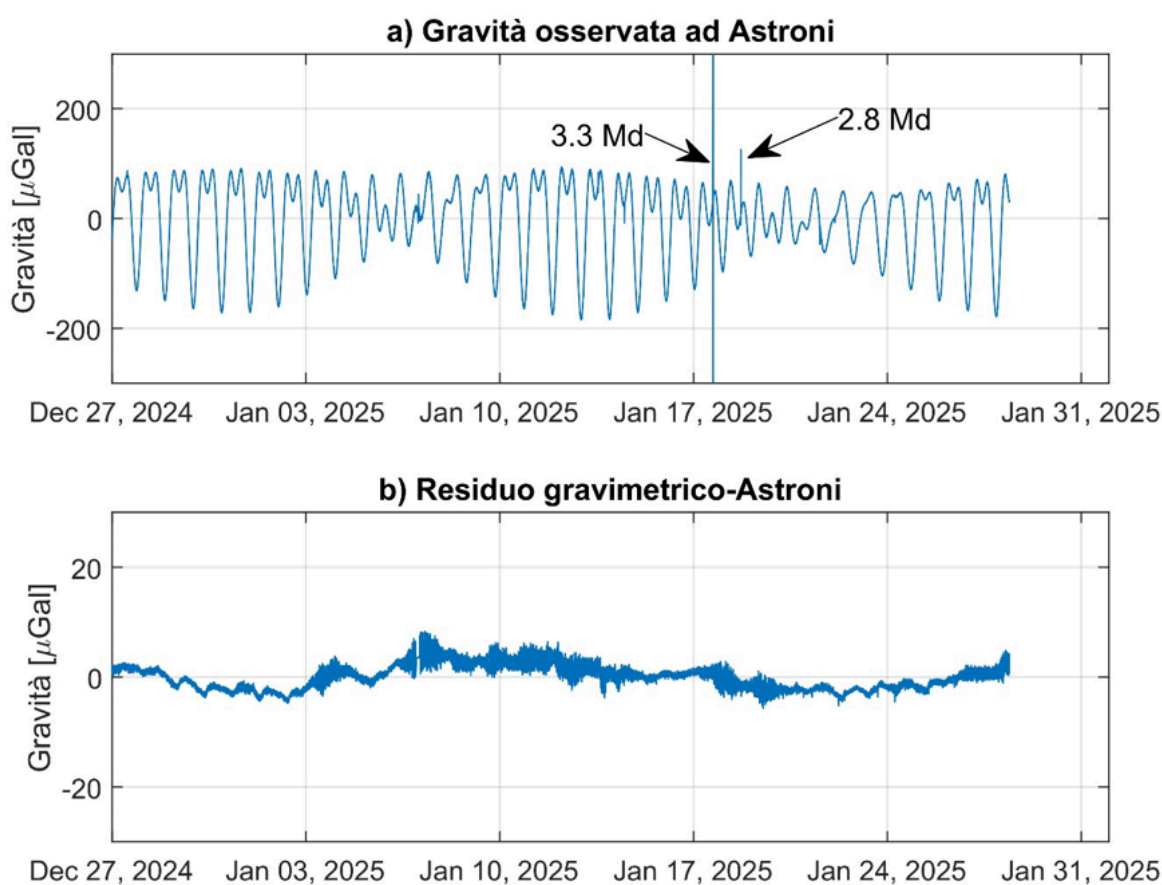
Figura 2.4.1 - a: serie temporale (risoluzione temporale 1 minuto) raw registrata dal gPhone. Si osserva il contributo dominante delle maree e di alcuni disturbi legati all'attività sismica nei Campi Flegrei. b: serie residua di gravità. Si osserva l'aumento in ampiezza dei residui, legato alle variazioni nelle condizioni meteorologiche.
