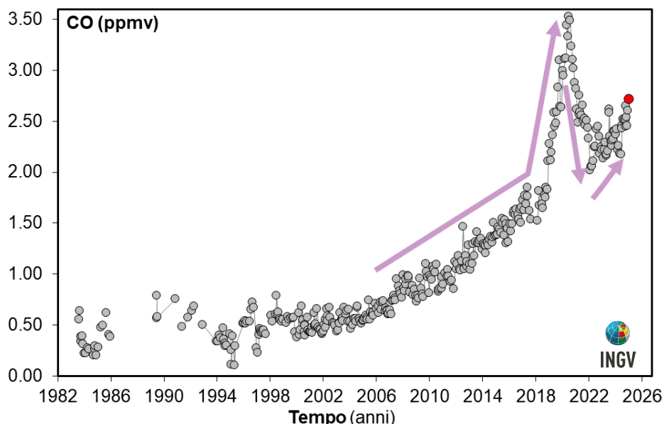
Figura 4.3 – Variazioni della concentrazione di monossido di carbonio (CO) misurato alla fumarola BG a partire dal 1983. Con il simbolo rosso è evidenziato il campione di gennaio 2025. In generale alti contenuti di CO caratterizzano sistemi vulcanici a elevata temperatura, mentre fumarole alimentate da sistemi idrotermali mostrano concentrazioni più basse, in tali sistemi un aumento delle concentrazioni di CO può riflettere un incremento delle condizioni di pressione e temperatura.
