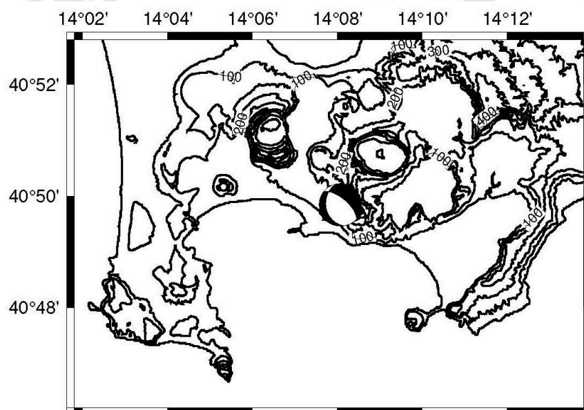
Figura 1.7 - Localizzazione e meccanismo focale dell'evento del 17/01/2024 alle 16:53 UTC M_d 3.3(\pm 0.3)
