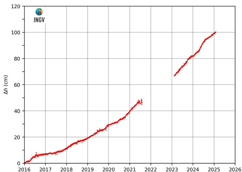
Figura 2.3.2 – Movimenti verticali del suolo, nel periodo gennaio 2016 – gennaio 2025, ottenuti dall'analisi dei dati acquisiti dalla stazione mareografica di Pozzuoli Porto (POPT), area centrale della caldera Flegrea. Le variazioni, riportate in cm, rappresentano le medie giornaliere e sono riferite alla stazione mareografica di Napoli, molo San Vincenzo (NAMI).
