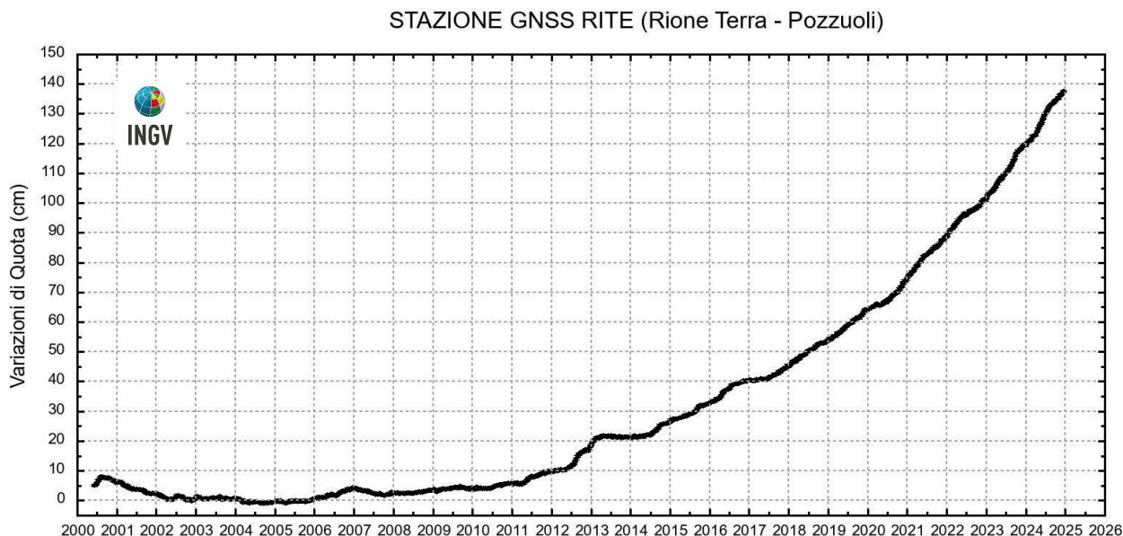
Figura 2.1.4 - Serie temporale delle variazioni settimanali in quota della stazione di RITE (Pozzuoli – Rione Terra) dal 2000 a gennaio 2025.
