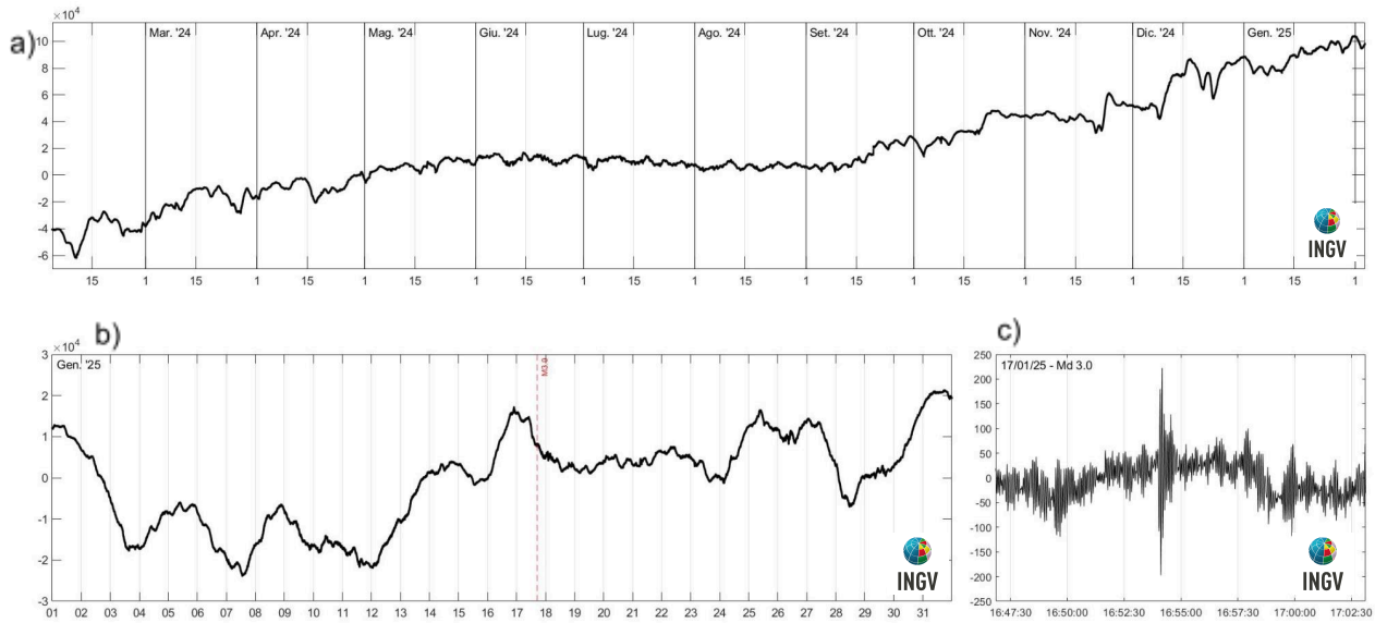
Figura 2.5.2 - a) Strain registrato nell'ultimo anno, dalle 00:00 UTC del 4/2/2024 alle 24:00 UTC del giorno 3/2/2025. b) Strain registrato nell'ultimo mese, dalle 00:00 UTC del giorno 1/1/2025 alle 24:00 UTC del giorno 31/1/2025. c) Variazione ad alta frequenza registrata dal dilatometro CQUE in concomitanza con l'evento sismico di Md3.0 avvenuto il giorno 17/01/2025.
