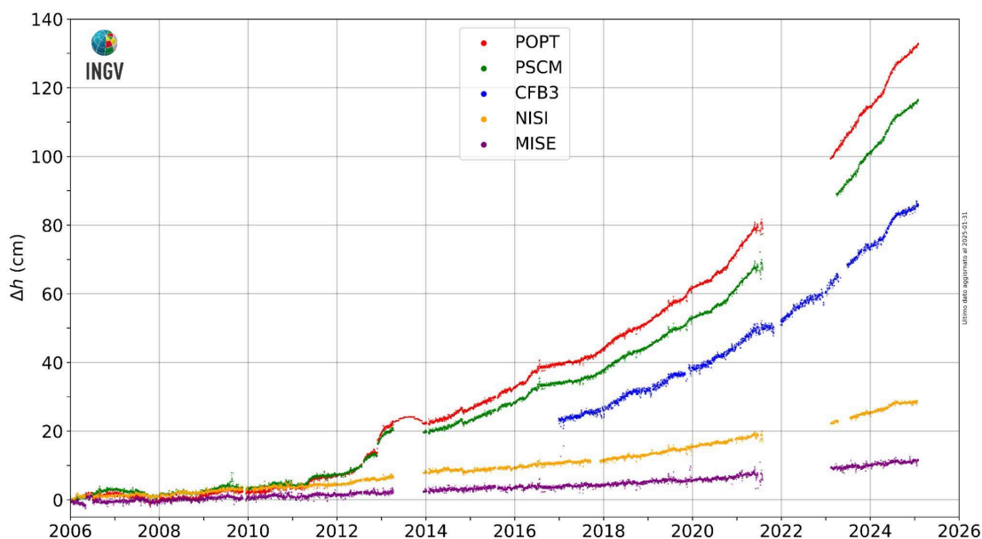
Figura 2.3.4 - Movimenti verticali del suolo nel periodo gennaio 2006 – gennaio 2025, ottenuti dall'analisi dei dati acquisiti da tutte le stazioni mareografiche dell'area della caldera Flegrea. Le variazioni, riportate in cm, rappresentano le medie giornaliere e sono tutte riferite alla stazione mareografica di Napoli, molo San Vincenzo (NAMM).
