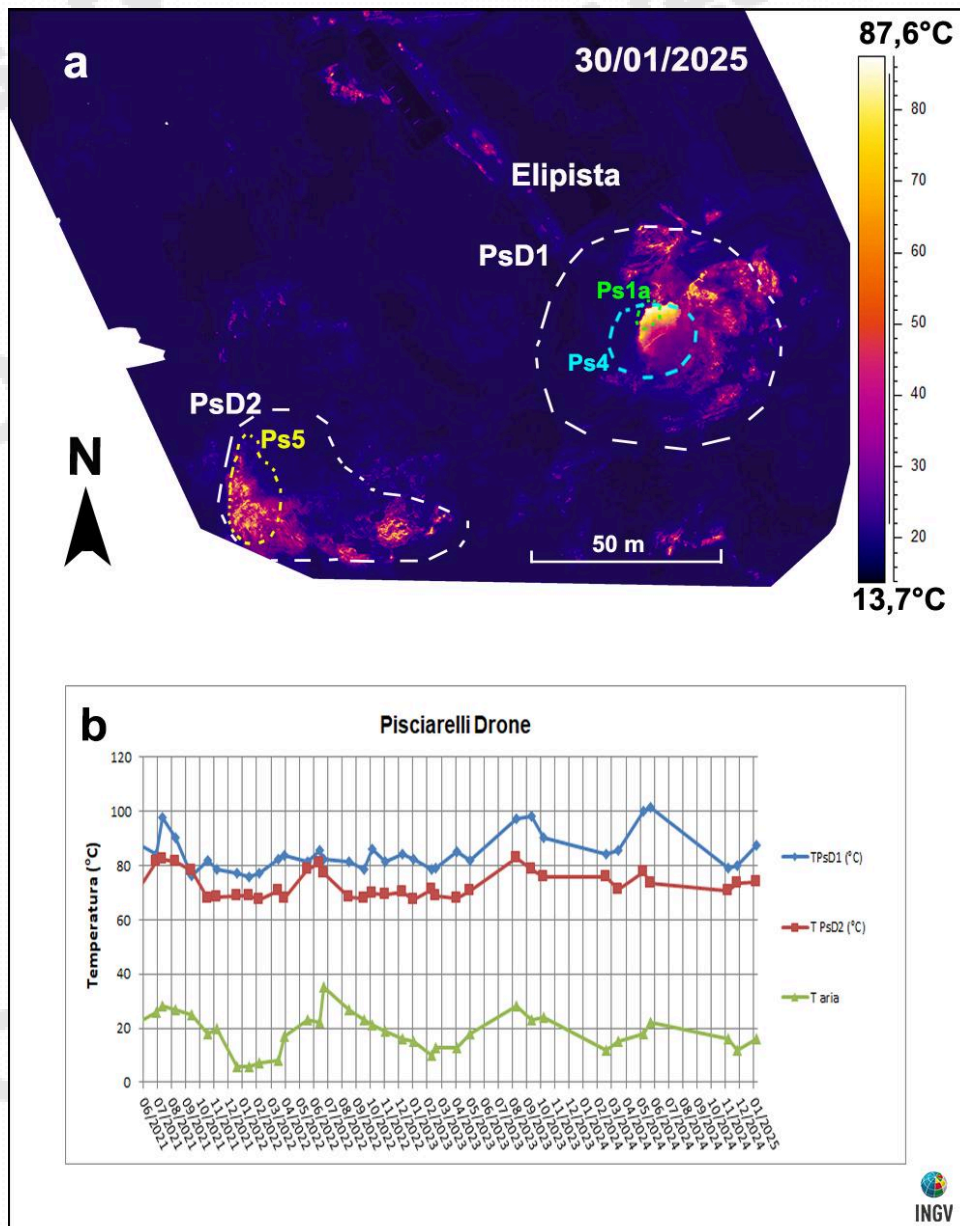
Figura 3.2.2 – Immagine termica, rilevata nel mese di gennaio 2025, dell'area denominata Ps4 (Fig.3.2.1b) (a) e valori massimi di temperatura (T) delle aree a maggiore anomalia termica (PsD1 e PsD2) confrontati con la temperatura dell'aria (Taria) misurata nel momento del rilievo termico da giugno 2021 a gennaio 2025 (b).
