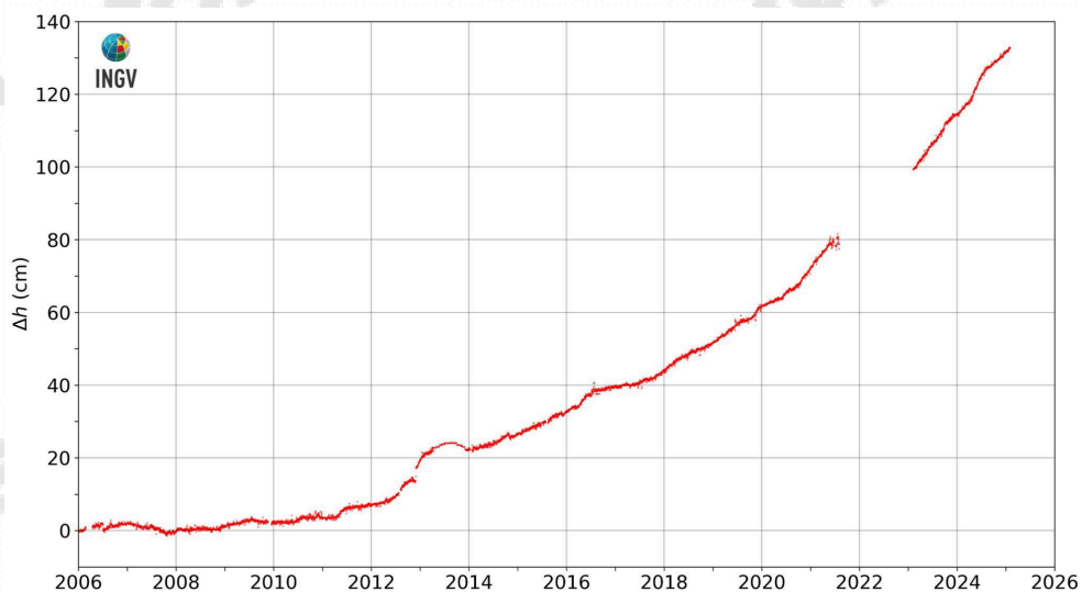
Figura 2.3.3 - Movimenti verticali del suolo nel periodo gennaio 2006 – gennaio 2025, ottenuti dall'analisi dei dati acquisiti dalla stazione mareografica di Pozzuoli Porto (POPT) (area centrale della caldera Flegrea). Le variazioni, riportate in cm, rappresentano le medie giornaliere e sono riferite alla stazione mareografica di Napoli, molo San Vincenzo (NAMM).
