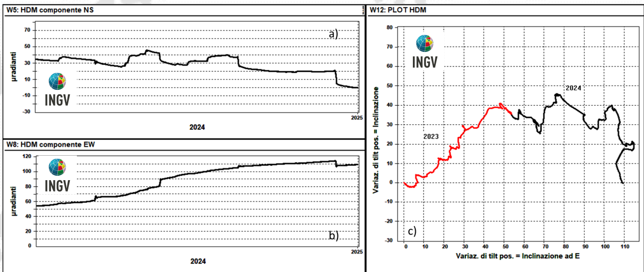
Figura 2.2.3 – Serie temporali (gennaio 2024 - dicembre 2024) e plot (gennaio 2023 - dicembre 2024) del tilt della stazione HDM della rete dei Campi Flegrei.
