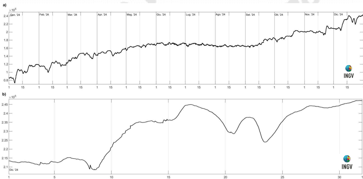
Figura 2.5.2 - a) Strain registrato nell'ultimo anno, dalle 00:00 UTC del 1/1/2024 alle 24:00 UTC del giorno 31/12/2024. b) Strain registrato nell'ultimo mese, dalle 00:00 UTC del giorno 1/12/2024 alle 24:00 UTC del giorno 31/12/2024.
