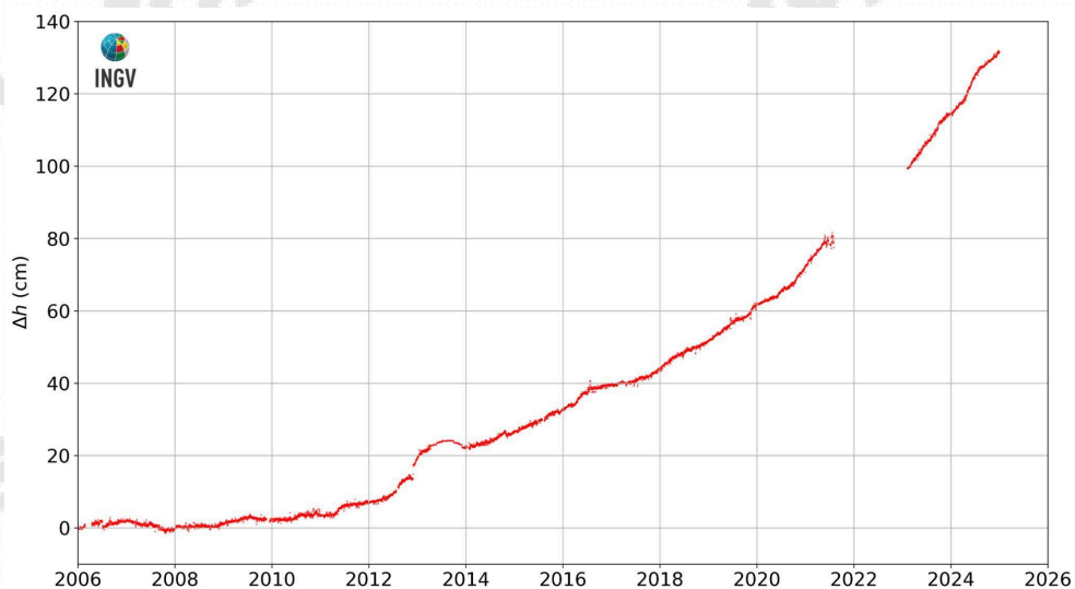
Figura 2.3.3 - Movimenti verticali del suolo nel periodo gennaio 2006 – dicembre 2024, ottenuti dall'analisi dei dati acquisiti dalla stazione mareografica di Pozzuoli Porto (POPT) (area centrale della caldera Flegrea). Le variazioni, riportate in cm, rappresentano le medie giornaliere e sono riferite alla stazione mareografica di Napoli, molo San Vincenzo (NAMM).
