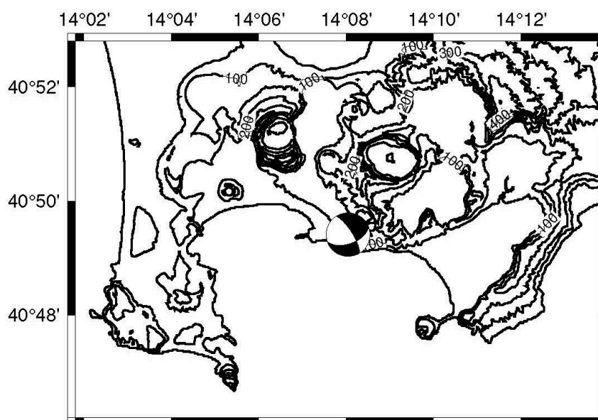
Figura 1.7 - Localizzazione e meccanismo focale dell'evento del 06/12/2024 alle 04:33 UTC M_d 3.4 (\pm 0.3)
