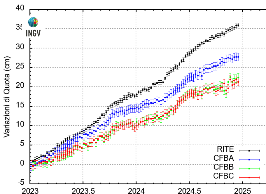
Figura 2.1.7 – Serie temporali delle variazioni settimanali in quota delle stazioni GNSS dell'infrastruttura marina MEDUSA nell'intervallo gennaio 2023 - dicembre 2024, confrontate con quella della stazione RITE
