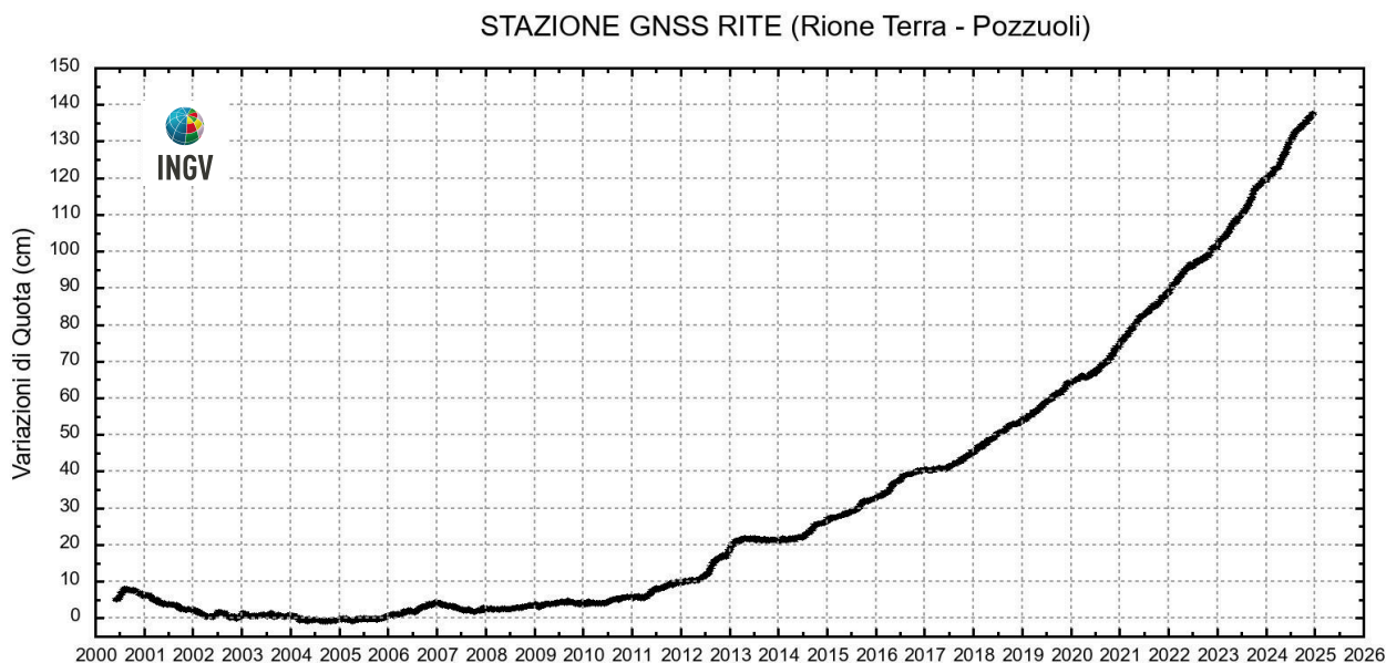
Figura 2.1.4 - Serie temporale delle variazioni settimanali in quota della stazione di RITE (Pozzuoli – Rione Terra) dal 2000 a dicembre 2024.
