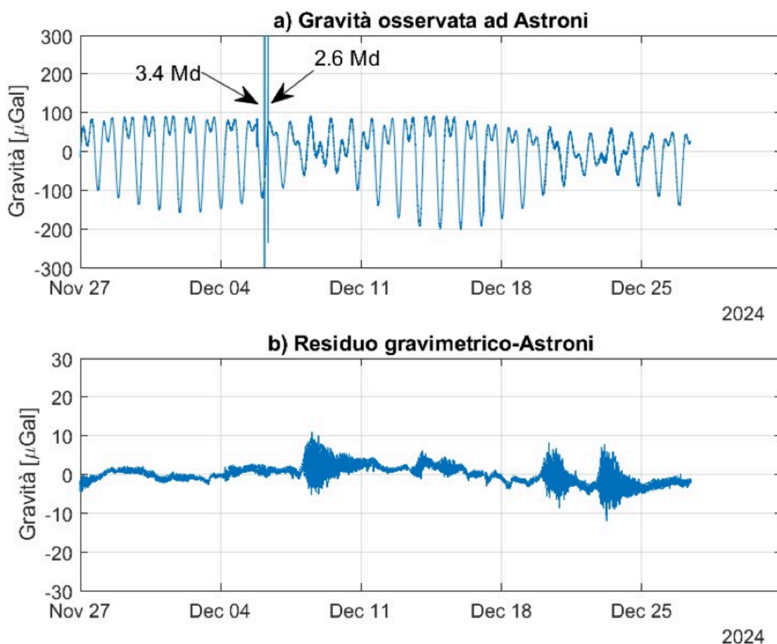
Figura 2.4.1 - a: serie temporale (risoluzione temporale 1 minuto) raw registrata dal gPhone. Si osserva il contributo dominante delle maree e di alcuni disturbi legati all'attività sismica nei Campi Flegrei. b: serie residua di gravità. Si osserva l'aumento in ampiezza dei residui, legato alle variazioni nelle condizioni meteorologiche.
