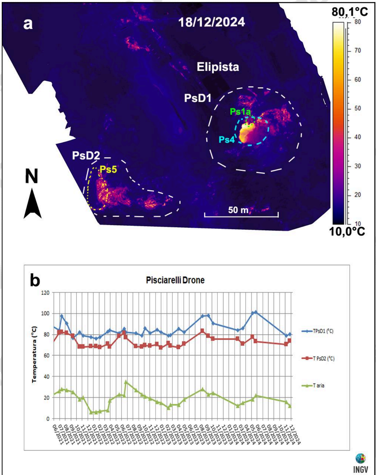
Figura 3.2.2 – Immagine termica, rilevata nel mese di dicembre 2024, dell'area denominata Ps4 (Fig.3.2.1b).
