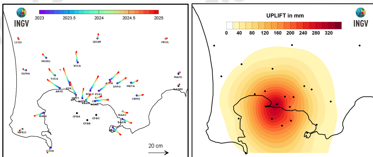
Figura 2.1.5 - Mappa degli spostamenti GNSS orizzontali (a) e verticali (b) registrati nell'area flegrea da gennaio 2023 a dicembre 2024.
