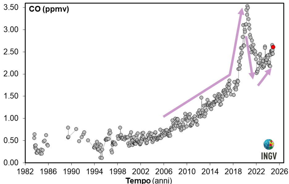
Figura 4.3 – Variazioni della concentrazione di monossido di carbonio (CO) misurato alla fumarola BG a partire dal 1983. Con il simbolo rosso è evidenziato il campione di dicembre 2024. In generale alti contenuti di CO caratterizzano sistemi vulcanici a elevata temperatura, mentre fumarole alimentate da sistemi idrotermali mostrano concentrazioni più basse, in tali sistemi un aumento delle concentrazioni di CO può riflettere un incremento delle condizioni di pressione e temperatura.
