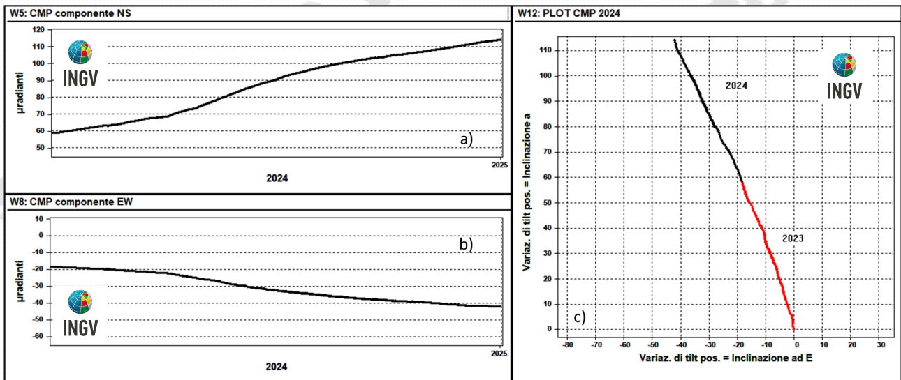
Figura 2.2.3 – Serie temporali (gennaio 2024 - dicembre 2024) e plot (gennaio 2023 - dicembre 2024) del tilt della stazione CMP della rete dei Campi Flegrei.
