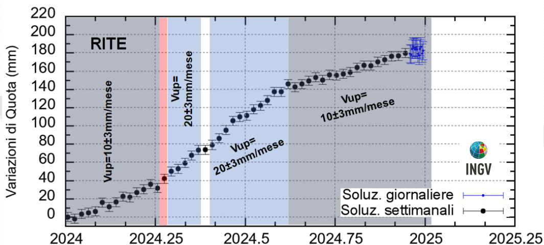
Figura 2.1.2 - Serie temporale delle variazioni in quota della stazione GNSS di RITE dal 01/01/2024 al 29/12/2024. Elaborazione dati in modalità Precise Point Positioning con software PRIDE PPP-AR (Geng et al., 2019).
