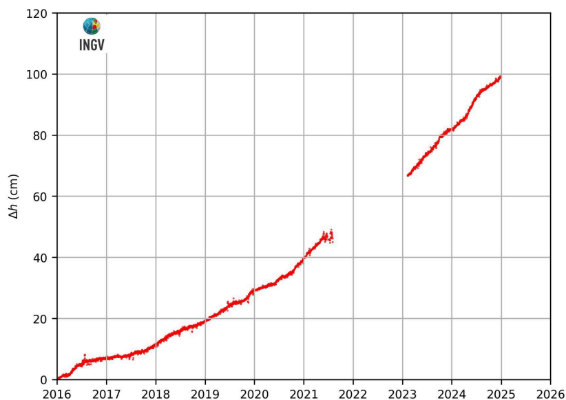
Figura 2.3.2 – Movimenti verticali del suolo, nel periodo gennaio 2016 – dicembre 2024, ottenuti dall'analisi dei dati acquisiti dalla stazione mareografica di Pozzuoli Porto (POPT), area centrale della caldera Flegrea. Le variazioni, riportate in cm, rappresentano le medie giornaliere e sono riferite alla stazione mareografica di Napoli, molo San Vincenzo (NAMI).
