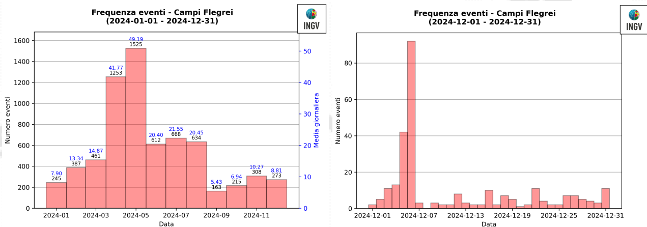
Figura 1.2 - A sinistra numero di eventi registrati ai Campi Flegrei nel corso degli ultimi 12 mesi (in totale 6744), mentre a destra quelli avvenuti nell'ultimo mese (in totale 273).
