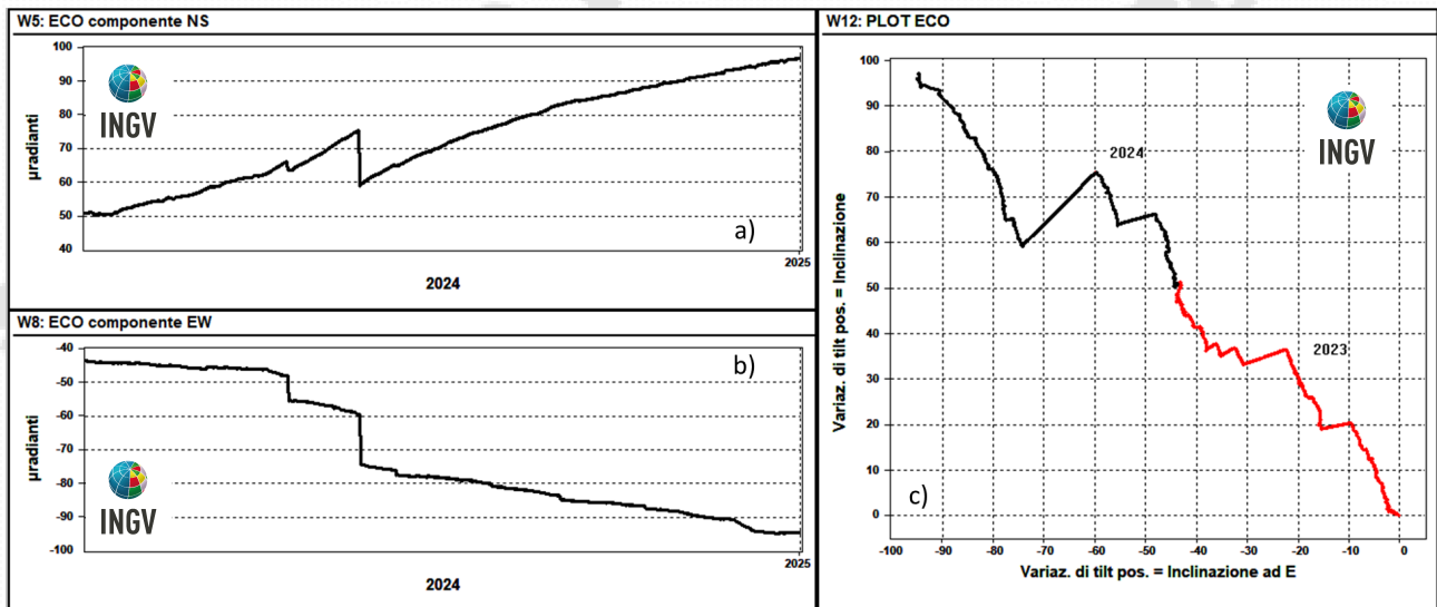
Figura 2.2.2 – Serie temporali (gennaio 2024 - dicembre 2024) e plot (gennaio 2023 - dicembre 2024) del tilt della stazione ECO della rete dei Campi Flegrei.
