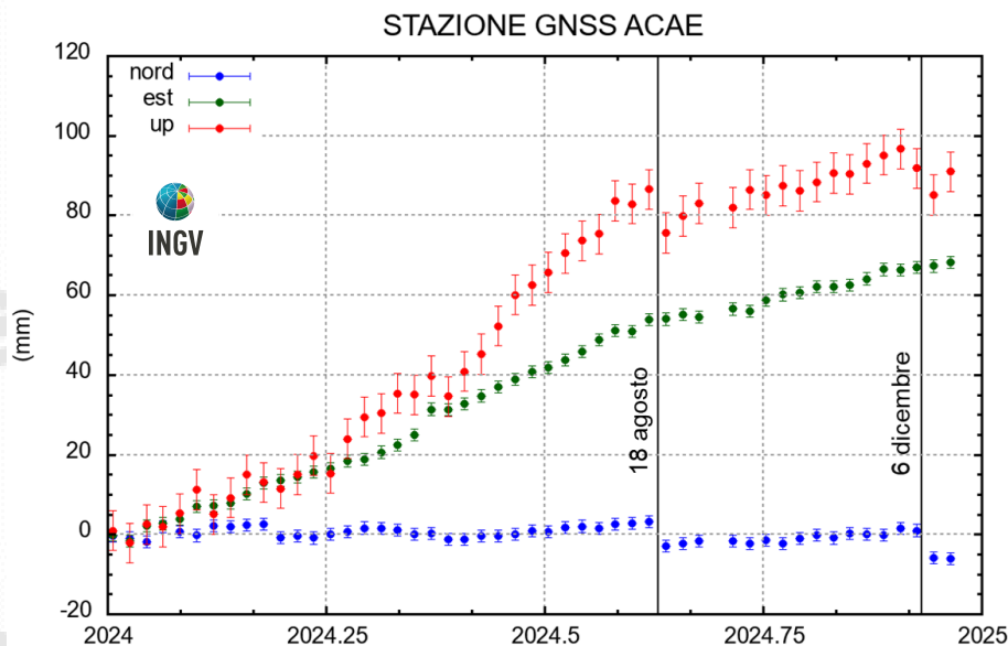
Figura 2.1.6 – Serie temporali delle variazioni settimanali lungo le componenti Nord, Est e Up della stazione GNSS di ACAE nel 2024.
