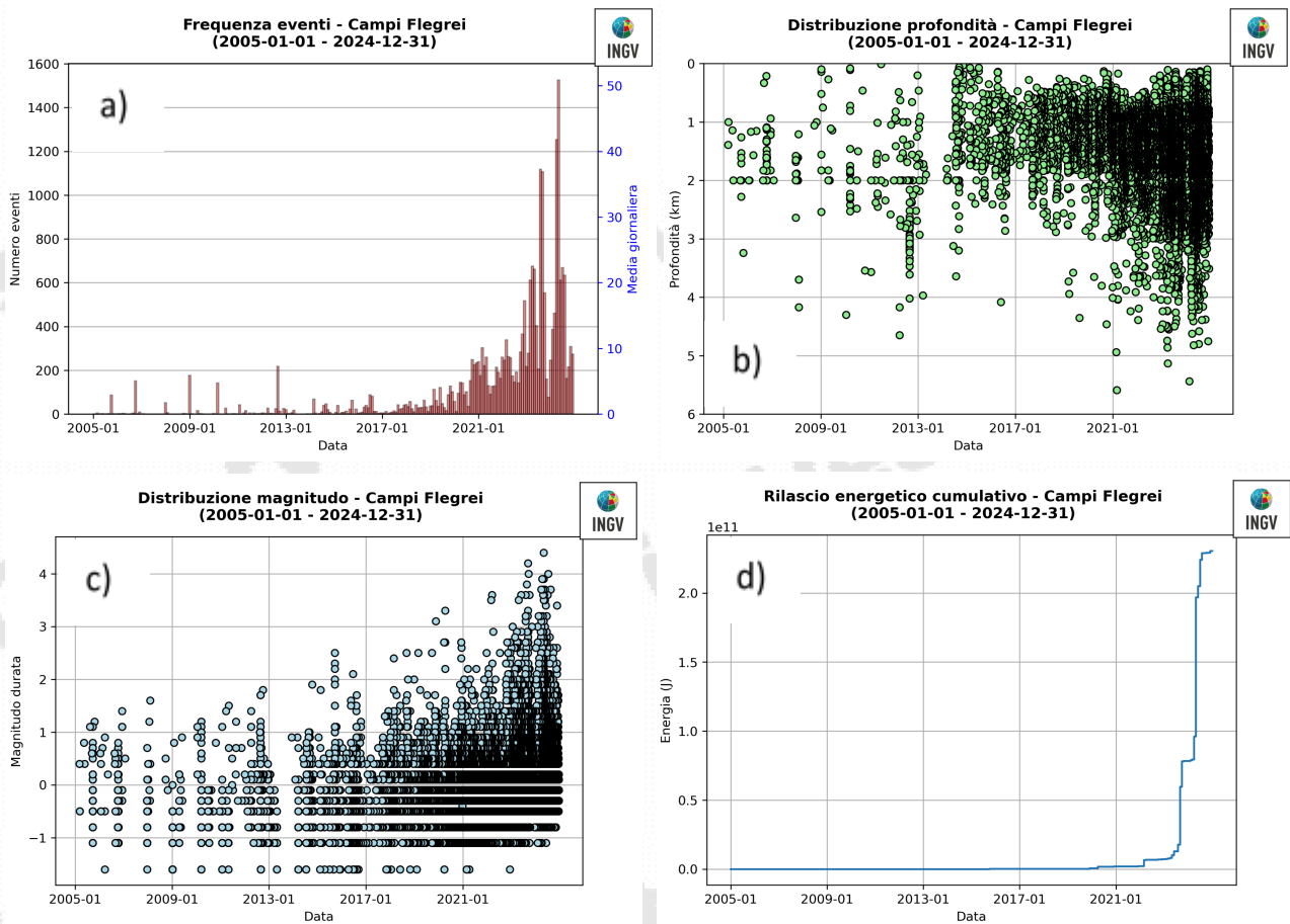
Figura 1.8 - Andamento dei principali parametri sismologici a partire dal 2005: a) frequenza di accadimento; b) profondità ipocentrali; c) magnitudo; d) energia cumulativa.
