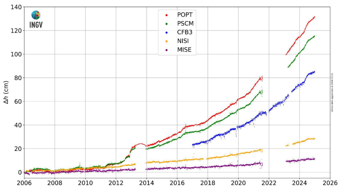
Figura 2.3.4 - Movimenti verticali del suolo nel periodo gennaio 2006 – dicembre 2024, ottenuti dall'analisi dei dati acquisiti da tutte le stazioni mareografiche dell'area della caldera Flegrea. Le variazioni, riportate in cm, rappresentano le medie giornaliere e sono tutte riferite alla stazione mareografica di Napoli, molo San Vincenzo (NAMM).
