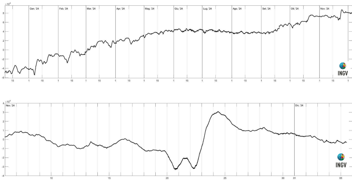
Figura 2.5.2 - a) Strain registrato nell'ultimo anno, dalle 00:00 UTC del 7/12/2023 alle 12:00 UTC del giorno 5/12/2024. b) Strain registrato nell'ultimo mese, dalle 00:00 UTC del giorno 6/11/2024 alle 12:00 UTC del giorno 5/12/2024.
