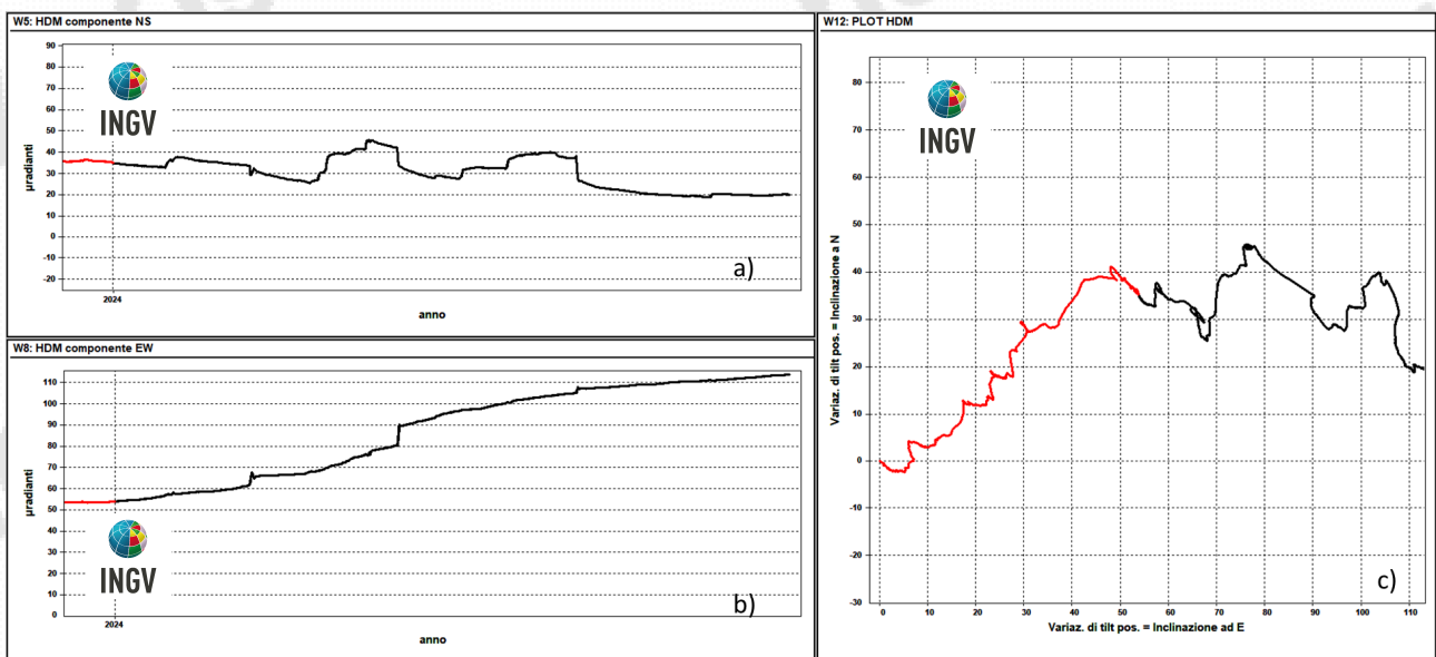
Figura 2.2.3 – Serie temporali e plot del tilt della stazione HDM della rete dei Campi Flegrei registrati negli ultimi 12 mesi (dicembre 2023 - novembre 2024).
