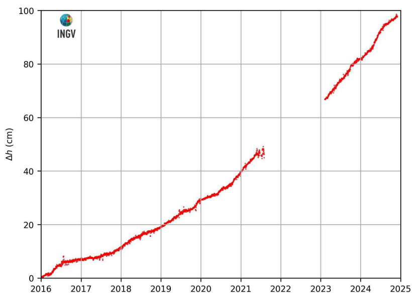
Figura 2.3.2 – Movimenti verticali del suolo, nel periodo gennaio 2016 – novembre 2024, ottenuti dall'analisi dei dati acquisiti dalla stazione mareografica di Pozzuoli Porto (POPT), area centrale della caldera Flegrea. Le variazioni, riportate in cm, rappresentano le medie giornaliere e sono riferite alla stazione mareografica di Napoli, molo San Vincenzo (NAMI).
