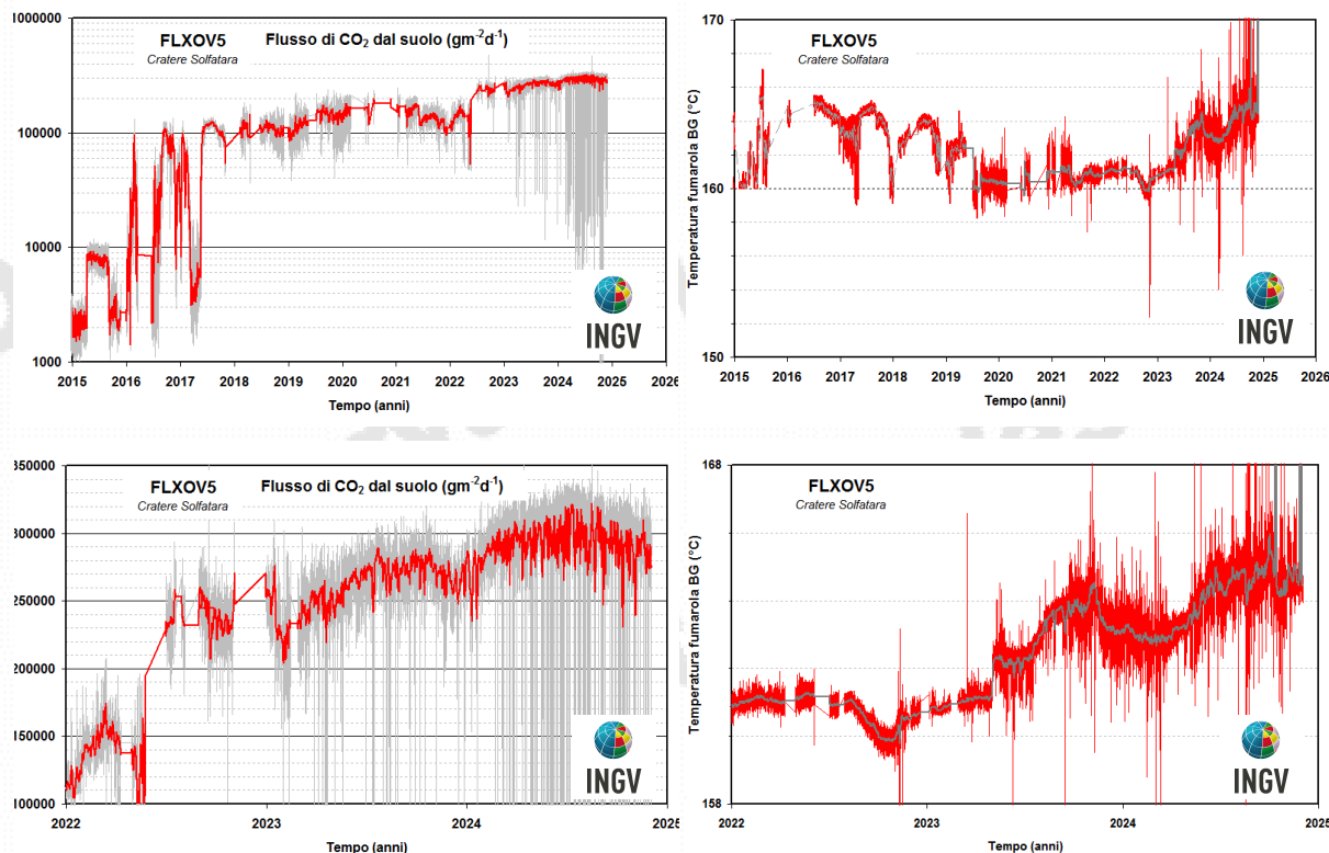
Figura 4.11 – Valori del flusso di CO 2 dal suolo e della temperatura della fumarola BG misurati dalla stazione FLXOV5 installata nel cratere della Solfatara, a pochi metri dalla fumarola principale BG. I valori di flusso di CO 2 dal suolo mostrano, in generale, un significativo incremento a partire dal 2016 (la linea rossa si riferisce alle medie giornaliere). Nei cronogrammi in basso sono riportati i valori di flusso di CO 2 e temperatura a partire da gennaio 2022.
