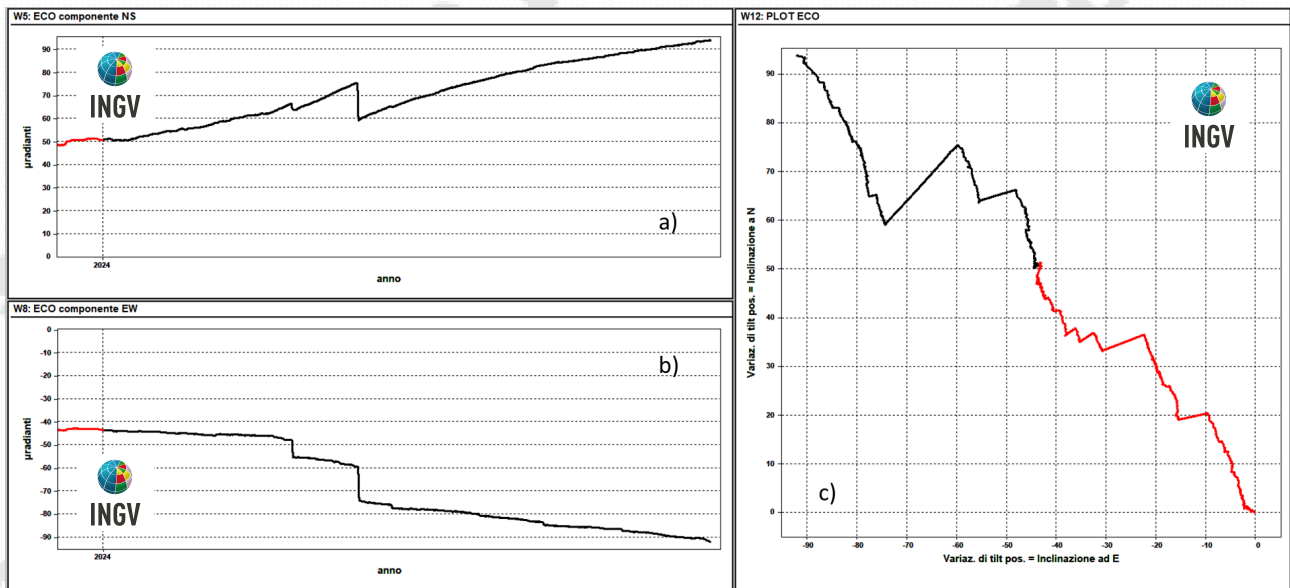
Figura 2.2.2 – Serie temporali e plot del tilt della stazione ECO della rete dei Campi Flegrei registrati negli ultimi 12 mesi (dicembre 2023 - novembre 2024).
