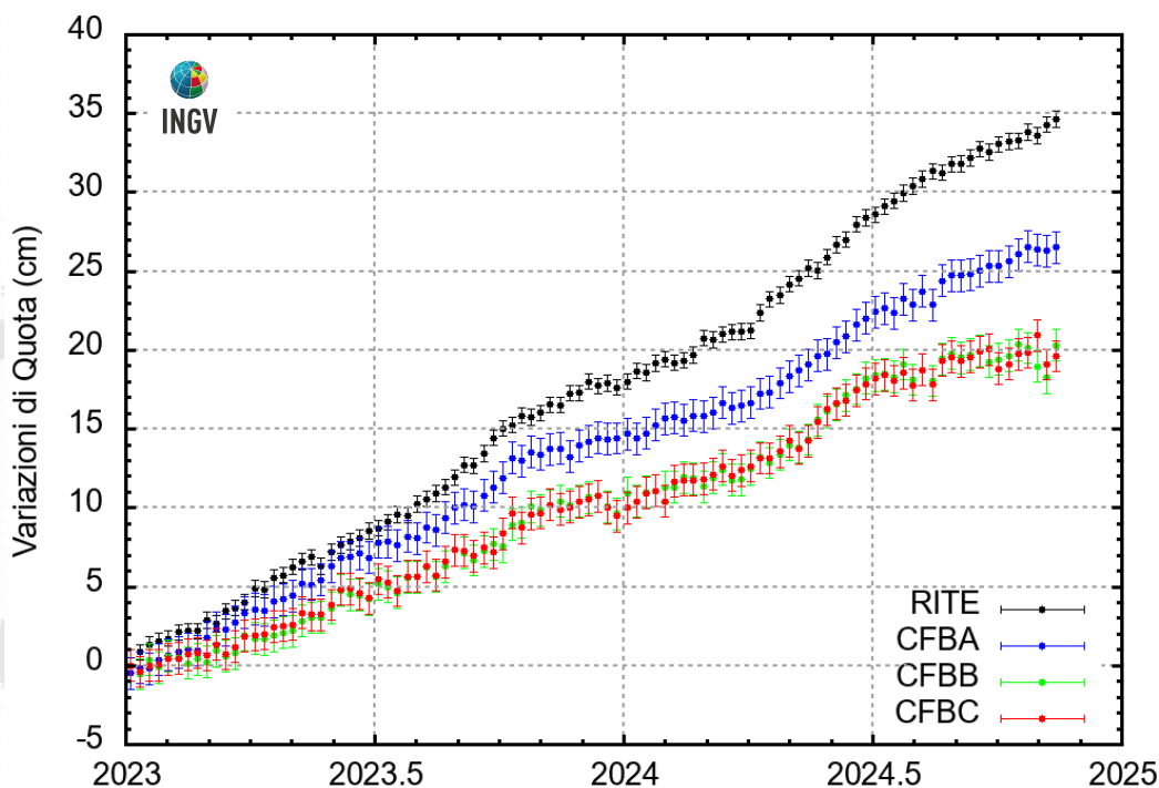
Figura 2.1.6 – Serie temporali delle variazioni settimanali in quota delle stazioni GNSS dell'infrastruttura marina MEDUSA nell'intervallo gennaio 2023 - novembre 2024, confrontate con quella della stazione RITE
