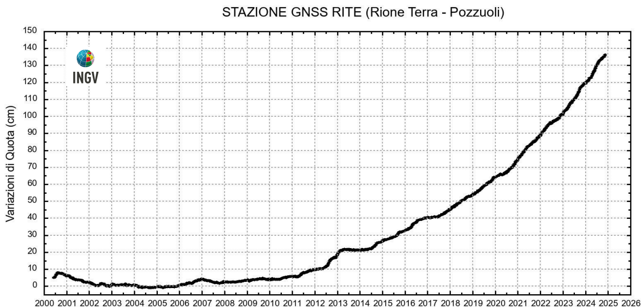
Figura 2.1.4 - Serie temporale delle variazioni settimanali in quota della stazione di RITE (Pozzuoli – Rione Terra) dal 2000 a novembre 2024.
