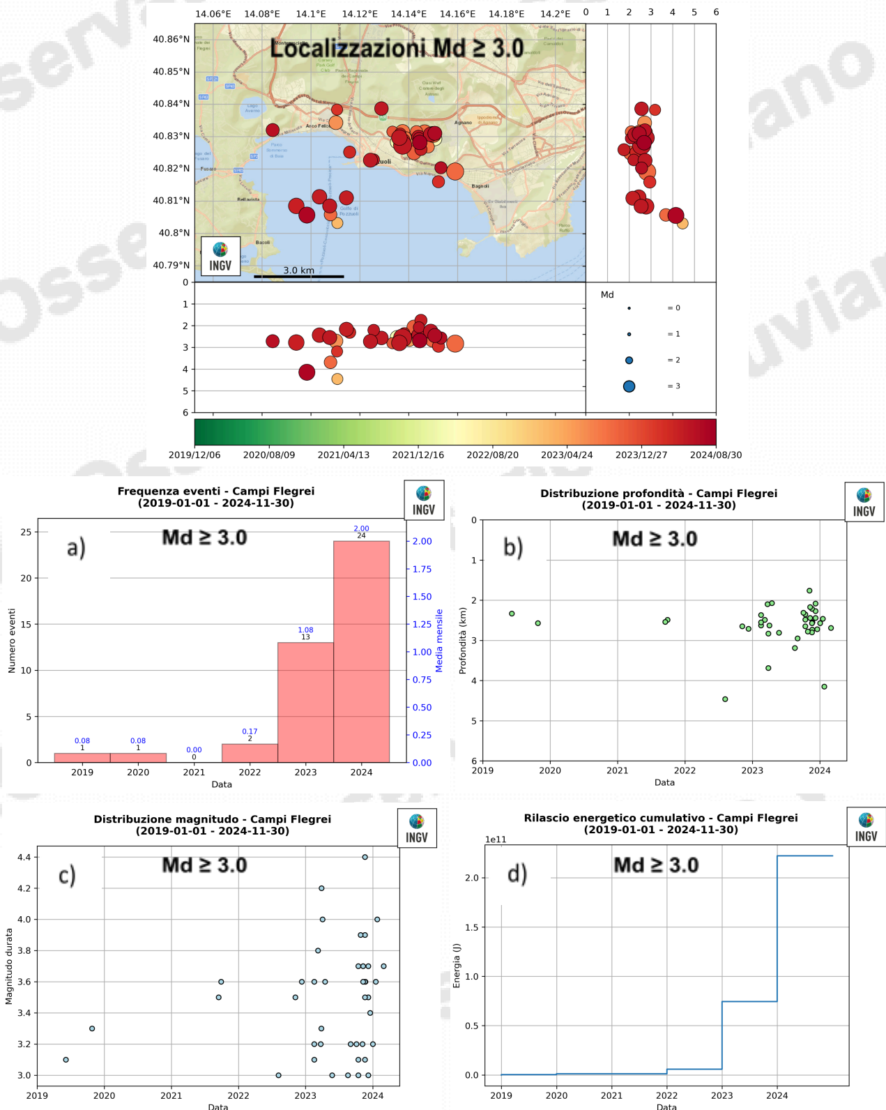
Figura 1.8 - Localizzazioni e andamento dei principali parametri sismologici dei terremoti con Md \geq 3.0 a partire dal 2019: a) frequenza di accadimento; b) profondità ipocentrali; c) magnitudo; d) energia cumulativa.
