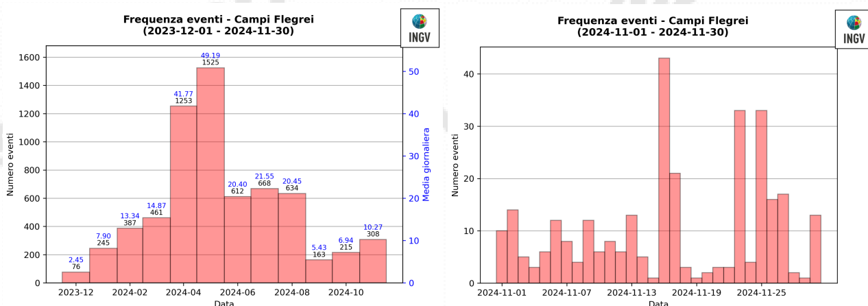
Figura 1.2 - A sinistra numero di eventi registrati ai Campi Flegrei nel corso degli ultimi 12 mesi (in totale 6547), mentre a destra quelli avvenuti nell'ultimo mese (in totale 308).
