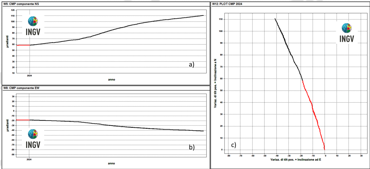
Figura 2.2.3 – Serie temporali e plot del tilt della stazione CMP della rete dei Campi Flegrei registrati negli ultimi 12 mesi (dicembre 2023 - novembre 2024).
