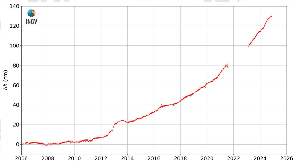
Figura 2.3.3 - Movimenti verticali del suolo nel periodo gennaio 2006 – novembre 2024, ottenuti dall'analisi dei dati acquisiti dalla stazione mareografica di Pozzuoli Porto (POPT) (area centrale della caldera Flegrea). Le variazioni, riportate in cm, rappresentano le medie giornaliere e sono riferite alla stazione mareografica di Napoli, molo San Vincenzo (NAMM).
