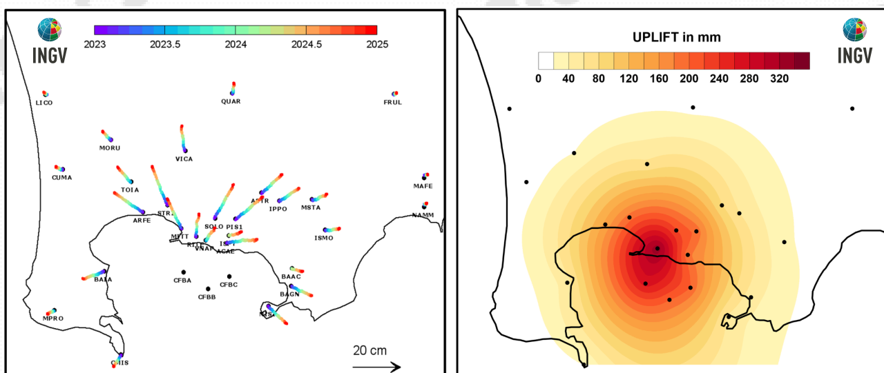
Figura 2.1.5 - Mappa degli spostamenti GNSS orizzontali (a) e verticali (b) registrati nell'area flegrea da gennaio 2023 a novembre 2024.
