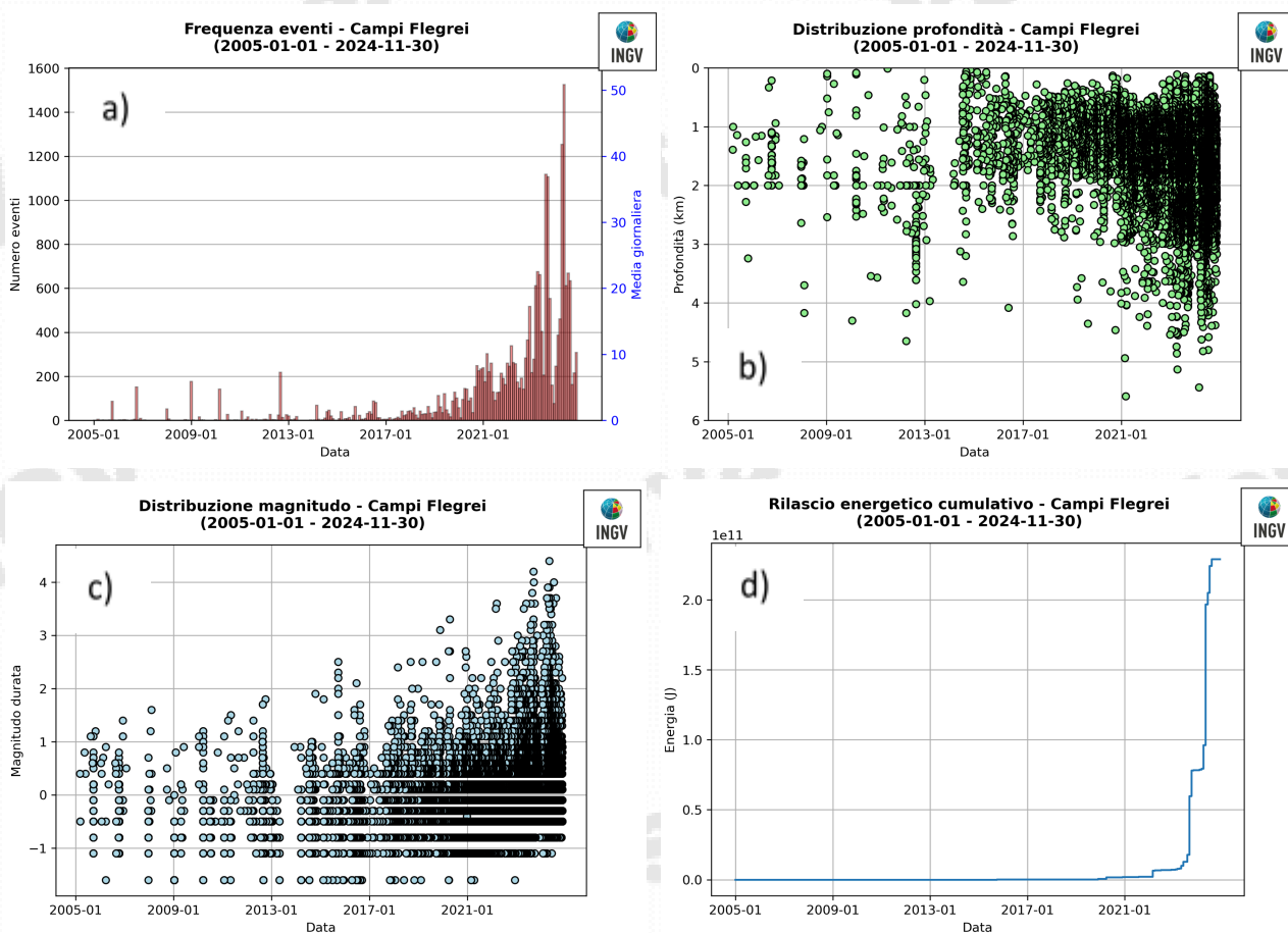
Figura 1.7 - Andamento dei principali parametri sismologici a partire dal 2005: a) frequenza di accadimento; b) profondità ipocentrali; c) magnitudo; d) energia cumulativa.
