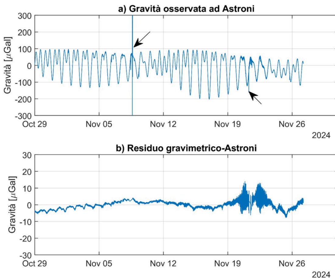
Figura 2.4.1 a: serie temporale (risoluzione temporale 1 minuto) raw registrata dal gPhone. Si osserva il contributo dominante delle maree e di alcuni disturbi legati ai lavori in corso presso l'oasi di Astroni. b: serie residui di gravità. Si osserva l'aumento in ampiezza dei residui a fine mese, legato a condizioni meteorologiche avverse.
