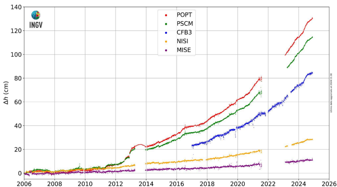
Figura 2.3.4 - Movimenti verticali del suolo nel periodo gennaio 2006 – novembre 2024, ottenuti dall'analisi dei dati acquisiti da tutte le stazioni mareografiche dell'area della caldera Flegrea. Le variazioni, riportate in cm, rappresentano le medie giornaliere e sono tutte riferite alla stazione mareografica di Napoli, molo San Vincenzo (NAMM).
