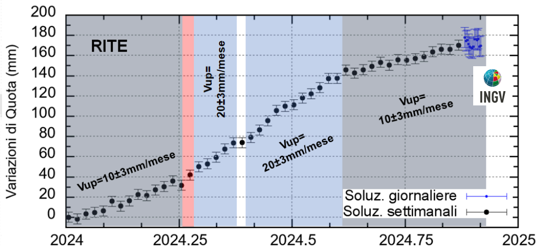
Figura 2.1.2 - Serie temporale delle variazioni in quota della stazione GNSS di RITE dal 01/01/2024 al 01/12/2024. Elaborazione dati in modalità Precise Point Positioning con software PRIDE PPP-AR (Geng et al., 2019).
