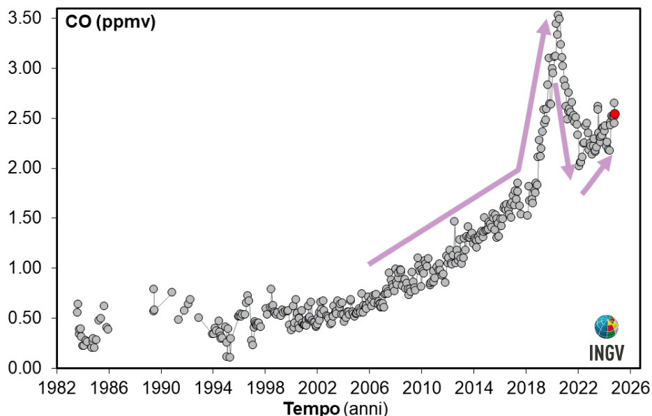
Figura 4.3 – Variazioni della concentrazione di monossido di carbonio (CO) misurato alla fumarola BG a partire dal 1983. Con il simbolo rosso è evidenziato il campione di novembre 2024. In generale alti contenuti di CO caratterizzano sistemi vulcanici a elevata temperatura, mentre fumarole alimentate da sistemi idrotermali mostrano concentrazioni più basse, in tali sistemi un aumento delle concentrazioni di CO può riflettere un incremento delle condizioni di pressione e temperatura.
