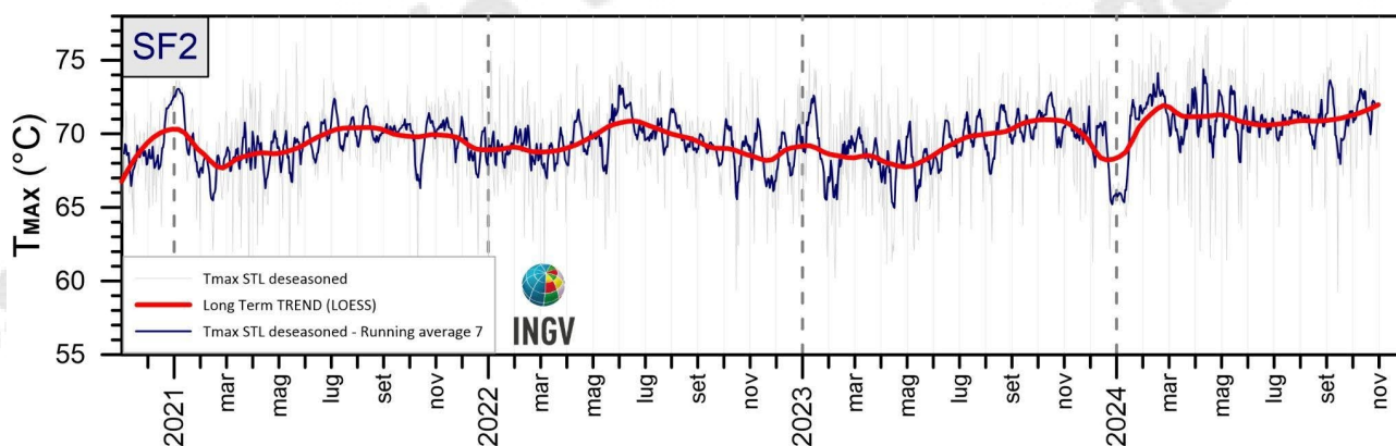
Figura 3.1.2 - Stazione SF2: Serie temporali dei valori di temperatura massima giornaliera rilevata nelle immagini IR, destagionalizzate mediante applicazione dell'algorithmo STL [medie settimanali (blu); trend a lungo termine (rosso)]. Il trend a lungo termine è ottenuto applicando un fitting LOESS di 2° alle temperature massime destagionalizzate.
