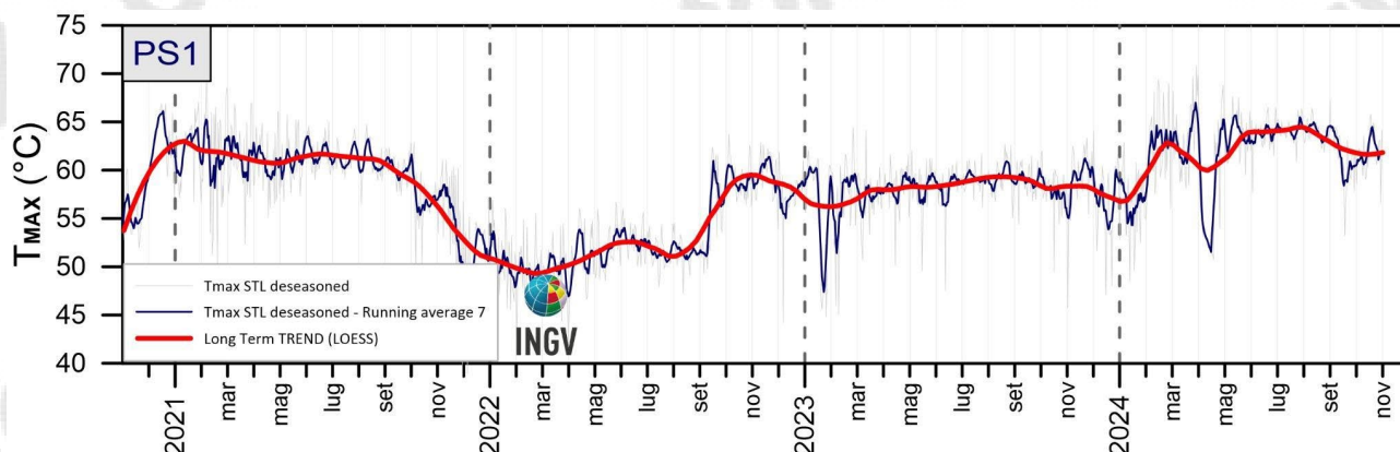
Figura 3.1.3 - Stazione PS1. Serie temporali dei valori di temperatura massima giornaliera rilevata nelle immagini IR destagionalizzate mediante applicazione dell'algorithmo STL [medie settimanali (blu); trend a lungo termine (rosso)]. Il trend a lungo termine è ottenuto applicando un fitting LOESS di 2° alle temperature massime destagionalizzate.
