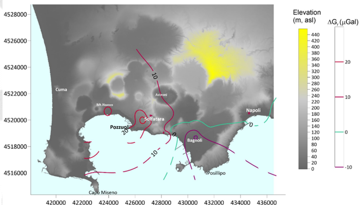
Figura 2.4.2a. Mappa dei residui \Delta g_r ottenuti dopo aver eliminato l'effetto di variazione di g dovuto al sollevamento della caldera misurato tra febbraio e ottobre 2024. La correzione FAG utilizzata è di -289 \text{ mGal/m} (Berrino et al., 1992).
