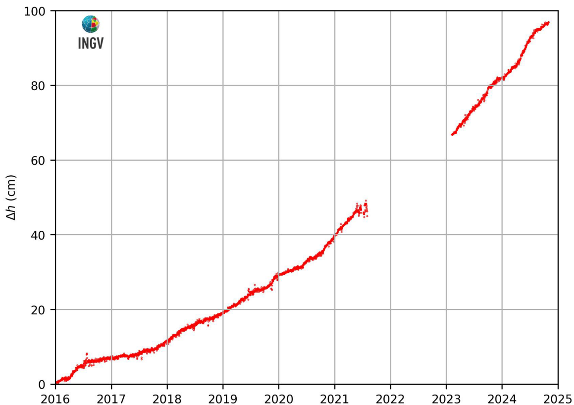
Figura 2.3.2 – Movimenti verticali del suolo, nel periodo gennaio 2016 – ottobre 2024, ottenuti dall’analisi dei dati acquisiti dalla stazione mareografica di Pozzuoli Porto (POPT), area centrale della caldera Flegrea. Le variazioni, riportate in cm, rappresentano le medie giornaliere e sono riferite alla stazione mareografica di Napoli, molo San Vincenzo (NAMM).
