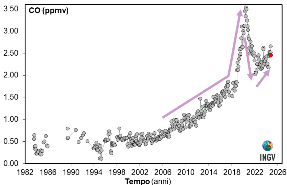
Figura 4.3 – Variazioni della concentrazione di monossido di carbonio (CO) misurato alla fumarola BG a partire dal 1983. Con il simbolo rosso è evidenziato il campione di ottobre 2024. In generale alti contenuti di CO caratterizzano sistemi vulcanici a elevata temperatura, mentre fumarole alimentate da sistemi idrotermali mostrano concentrazioni più basse, in tali sistemi un aumento delle concentrazioni di CO può riflettere un incremento delle condizioni di pressione e temperatura.
