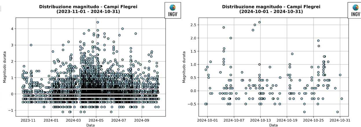
Figura 1.5 - Magnitudo degli eventi registrati ai Campi Flegrei nel corso degli ultimi 12 mesi (a sinistra) e dell'ultimo mese (a destra).
