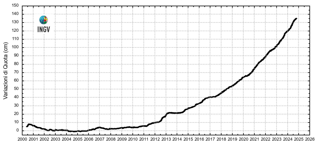
Figura 2.1.4 - Serie temporale delle variazioni settimanali in quota della stazione di RITE (Pozzuoli – Rione Terra) dal 2000 a ottobre 2024.
