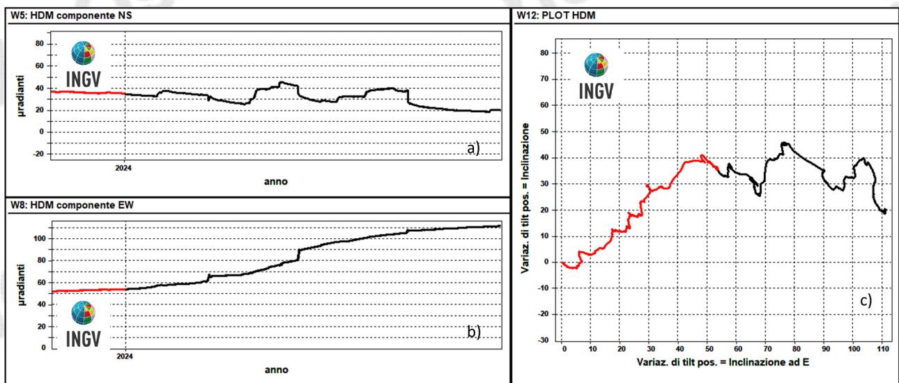
Figura 2.2.3 – Serie temporali e plot del tilt della stazione HDM della rete dei Campi Flegrei registrati negli ultimi 12 mesi (novembre 2023 - ottobre 2024).
