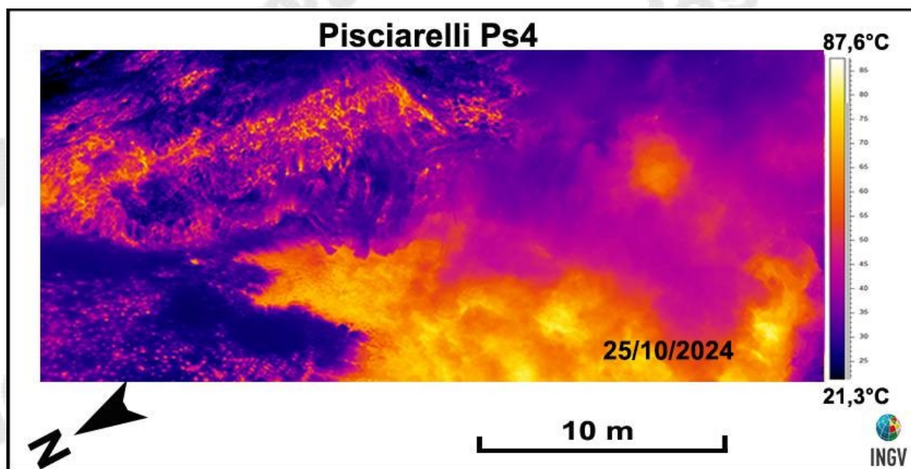
Figura 3.2.2 – Immagine termica, rilevata nel mese di ottobre 2024, dell'area denominata Ps4 (Fig.3.2.1b).
