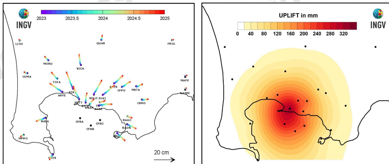
Figura 2.1.5 - Mappa degli spostamenti GNSS orizzontali (a) e verticali (b) registrati nell'area flegrea da gennaio 2023 a ottobre 2024.
