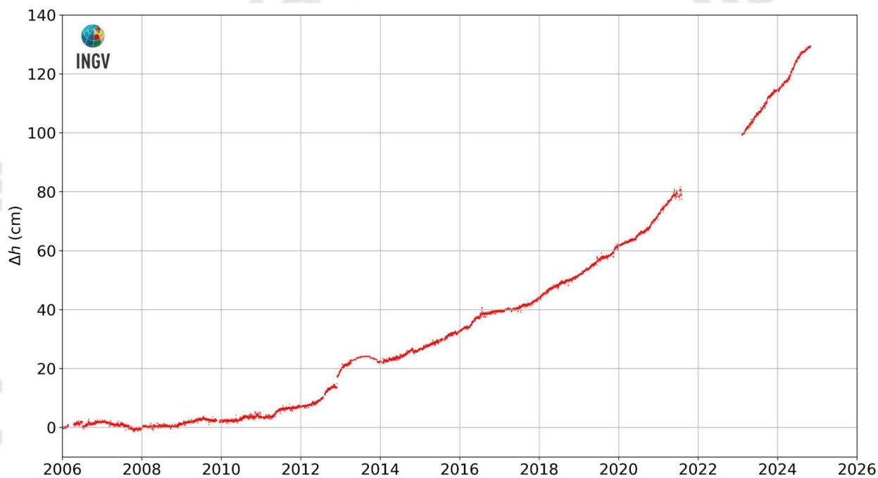
Figura 2.3.3 - Movimenti verticali del suolo nel periodo gennaio 2006 – ottobre 2024, ottenuti dall'analisi dei dati acquisiti dalla stazione mareografica di Pozzuoli Porto (POPT) (area centrale della caldera Flegrea). Le variazioni, riportate in cm, rappresentano le medie giornaliere e sono riferite alla stazione mareografica di Napoli, molo San Vincenzo (NAMM).
