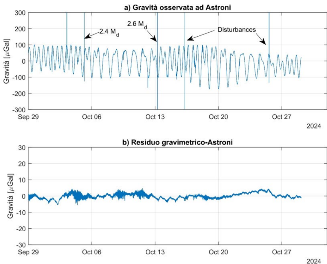
Figura 2.4.3 a: serie temporale (risoluzione temporale 1 minuto) raw registrata dal gPhone. Si osserva il contributo dominante delle maree, di alcuni terremoti e di disturbi legati ai lavori in corso presso l'oasi di Astroni. b: serie residua di gravità.
