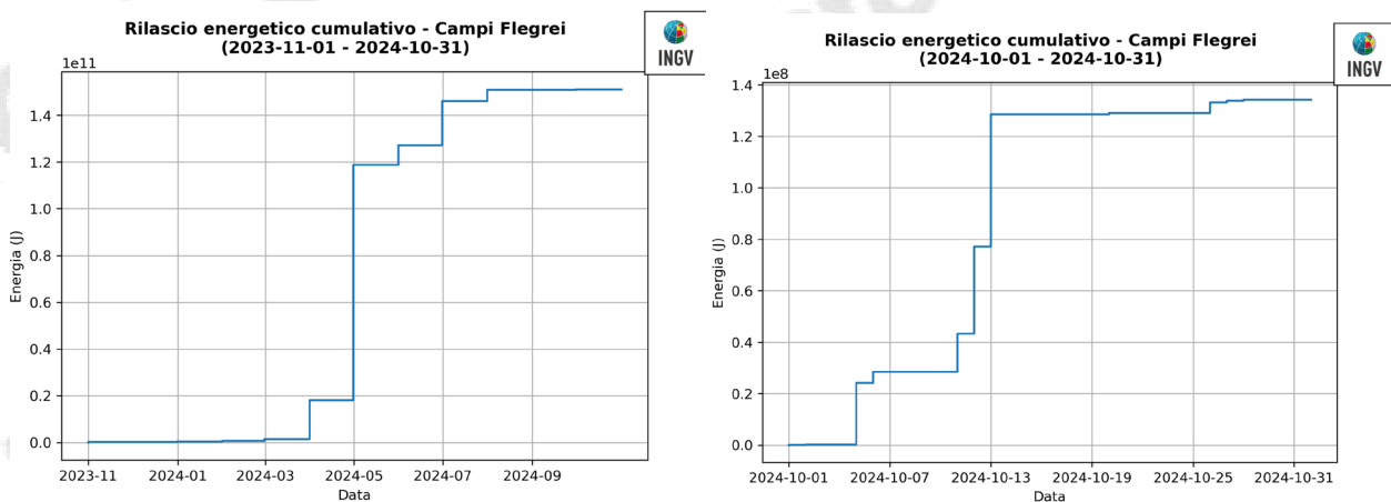
Figura 1.6 - Rilascio cumulativo di energia sismica ai Campi Flegrei nel corso degli ultimi 12 mesi (mensile a sinistra) e dell'ultimo mese (a destra).
