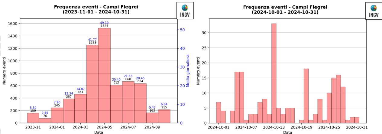
Figura 1.2 - A sinistra numero di eventi registrati ai Campi Flegrei nel corso degli ultimi 12 mesi (in totale 6398), mentre a destra quelli avvenuti nell'ultimo mese (in totale 215).
