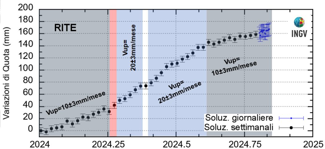
Figura 2.1.2 - Serie temporale delle variazioni in quota della stazione GNSS di RITE dal 01/01/2024 al 01/10/2024. Elaborazione dati in modalità Precise Point Positioning con software PRIDE PPP-AR (Geng et al., 2019).
