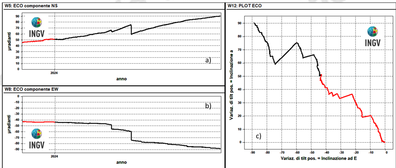
Figura 2.2.2 – Serie temporali e plot del tilt della stazione ECO della rete dei Campi Flegrei registrati negli ultimi 12 mesi (novembre 2023 - ottobre 2024).
