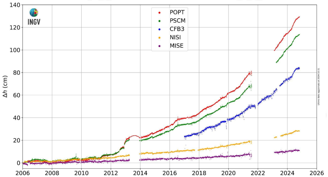
Figura 2.3.4 - Movimenti verticali del suolo nel periodo gennaio 2006 – ottobre 2024, ottenuti dall'analisi dei dati acquisiti da tutte le stazioni mareografiche dell'area della caldera Flegrea. Le variazioni, riportate in cm, rappresentano le medie giornaliere e sono tutte riferite alla stazione mareografica di Napoli, molo San Vincenzo (NAMM).
