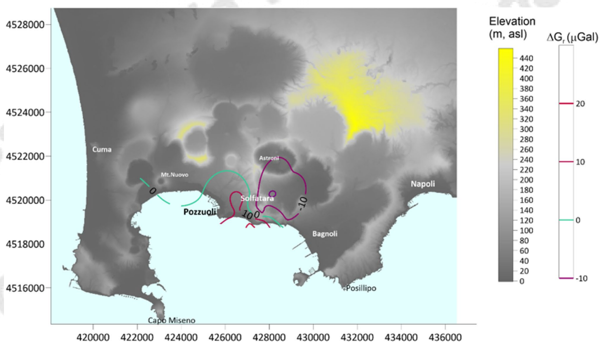
Figura 2.4.2b. Mappa dei residui \Delta G_r ottenuti dopo aver eliminato l'effetto di variazione di g dovuto al sollevamento della caldera misurato tra maggio e ottobre 2024. La correzione FAG utilizzata è di -289 \text{ mGal/m} (Berrino et al., 1992)
