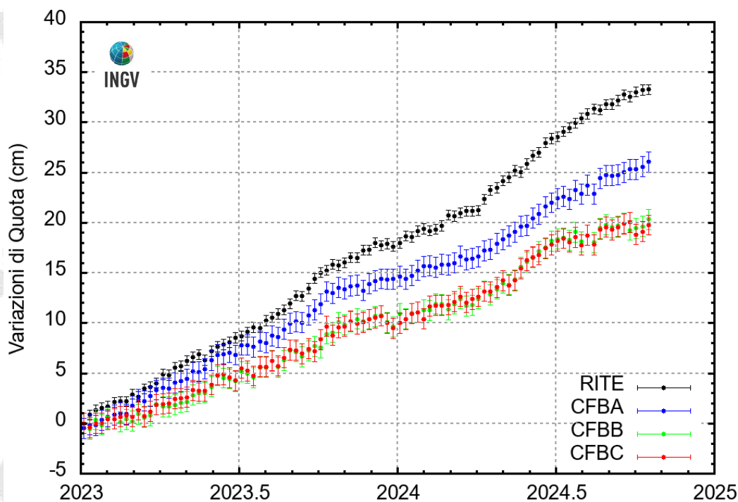
Figura 2.1.6 – Serie temporali delle variazioni settimanali in quota delle stazioni GNSS dell'infrastruttura marina MEDUSA nell'intervallo gennaio 2023 - ottobre 2024, confrontate con quella della stazione RITE
