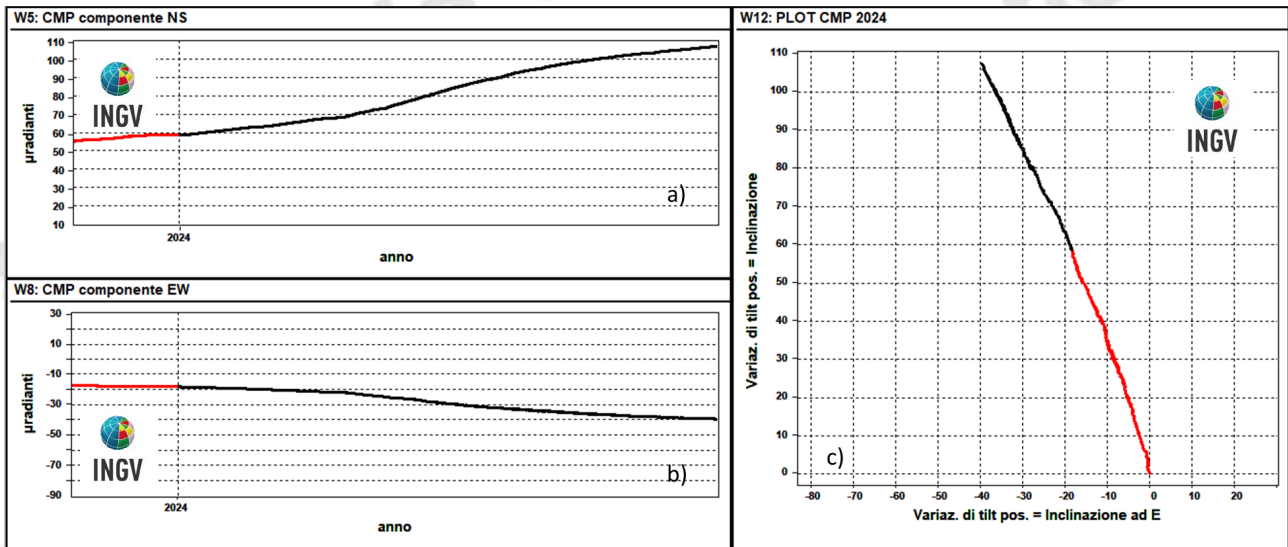
Figura 2.2.3 – Serie temporali e plot del tilt della stazione CMP della rete dei Campi Flegrei registrati negli ultimi 12 mesi (novembre 2023 - ottobre 2024).
