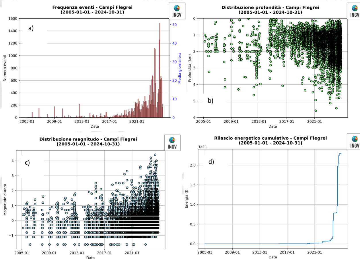
Figura 1.7 - Andamento dei principali parametri sismologici a partire dal 2005: a) frequenza di accadimento; b) profondità ipocentrali; c) magnitudo; d) energia cumulativa.
