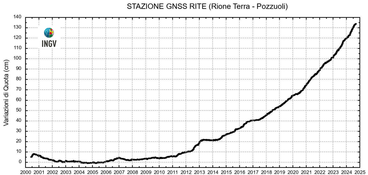
Figura 2.1.4 - Serie temporale delle variazioni settimanali in quota della stazione di RITE (Pozzuoli – Rione Terra) dal 2000 a settembre 2024.
