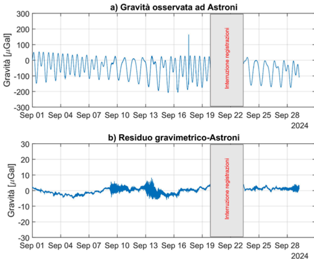
Figura 2.4.1 a: serie temporale raw (risoluzione temporale 1 minuto) registrata dal gPhone. Si osserva il contributo dominante delle maree. b: serie residua di gravità.
