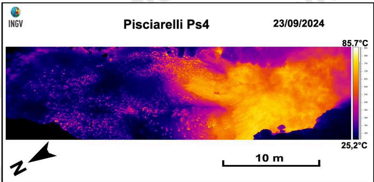
Figura 3.2.2 – Immagine termica, rilevata nel mese di settembre 2024, dell'area denominata Ps4 (Fig.3.2.1b).
