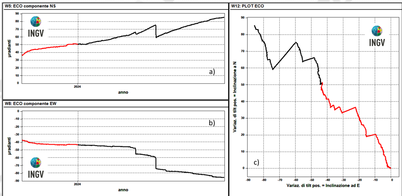
Figura 2.2.2 – Serie temporali e plot del tilt della stazione ECO della rete dei Campi Flegrei registrati negli ultimi 12 mesi (ottobre 2023 - settembre 2024).
