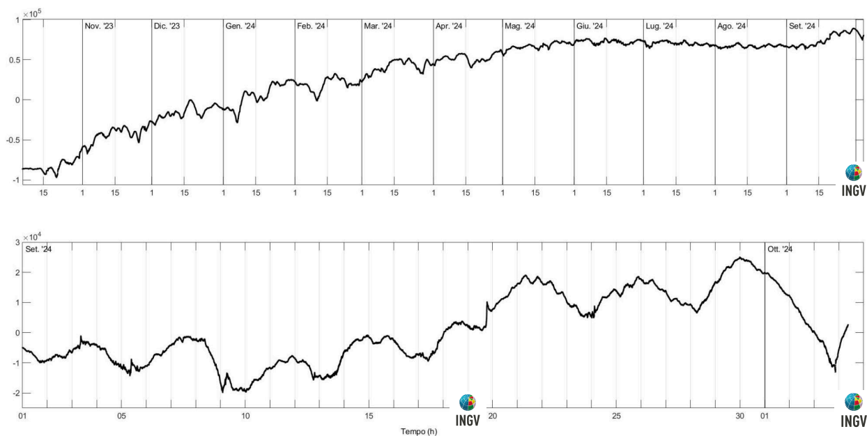
Figura 2.5.2 - a) Strain registrato nell'ultimo anno, dalle 00:00 UTC del 6/10/2023 alle 8:45 UTC del giorno 4/10/2024. b) Strain registrato nell'ultimo mese, dalle 00:00 UTC del giorno 1/9/2024 alle 8:45 UTC del giorno 4/10/2024.
