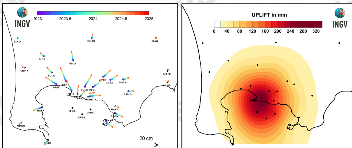
Figura 2.1.5 - Mappa degli spostamenti GNSS orizzontali (a) e verticali (b) registrati nell'area flegrea da gennaio 2023 a settembre 2024.
