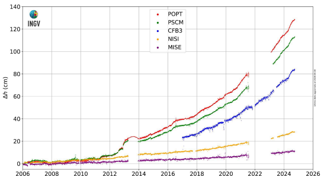
Figura 2.3.4 - Movimenti verticali del suolo nel periodo gennaio 2006 – settembre 2024, ottenuti dall'analisi dei dati acquisiti da tutte le stazioni mareografiche dell'area della caldera Flegrea. Le variazioni, riportate in cm, rappresentano le medie giornaliere e sono tutte riferite alla stazione mareografica di Napoli, molo San Vincenzo (NAMM).
