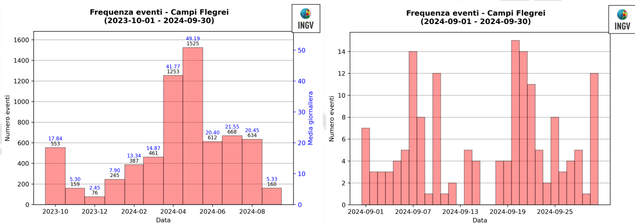
Figura 1.2 - A sinistra numero di eventi registrati ai Campi Flegrei nel corso degli ultimi 12 mesi (in totale 6739), mentre a destra quelli avvenuti nell'ultimo mese (in totale 160).
