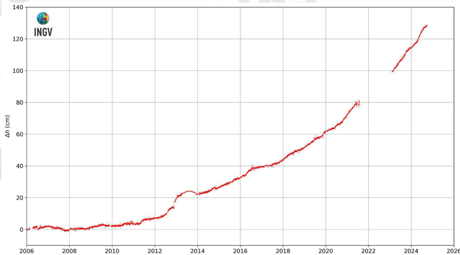
Figura 2.3.3 - Movimenti verticali del suolo nel periodo gennaio 2006 – settembre 2024, ottenuti dall'analisi dei dati acquisiti dalla stazione mareografica di Pozzuoli Porto (POPT) (area centrale della caldera Flegrea). Le variazioni, riportate in cm, rappresentano le medie giornaliere e sono riferite alla stazione mareografica di Napoli, molo San Vincenzo (NAMM).
