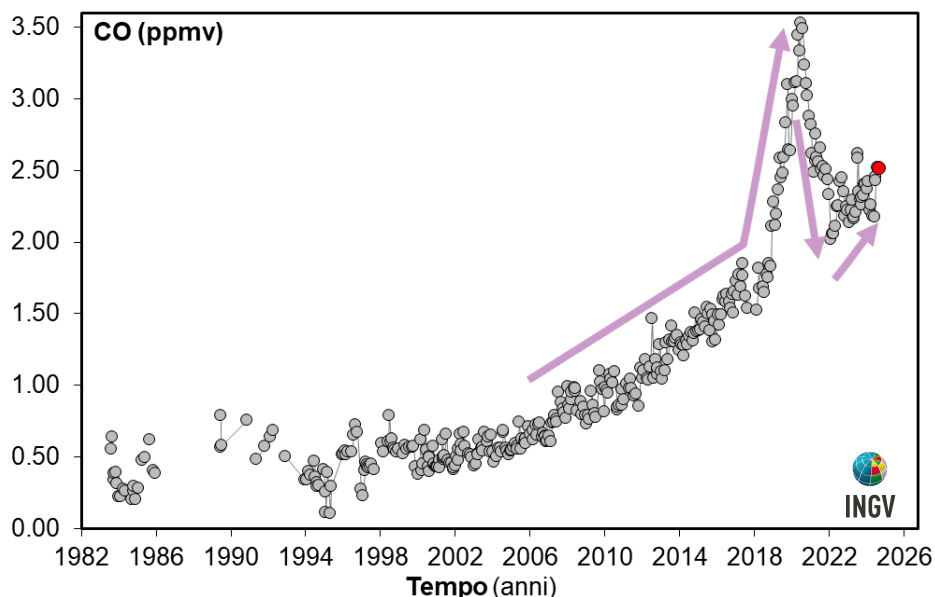
Figura 4.3 – Variazioni della concentrazione di monossido di carbonio (CO) misurato alla fumarola BG a partire dal 1983. Con il simbolo rosso è evidenziato il campione di settembre 2024. In generale alti contenuti di CO caratterizzano sistemi vulcanici a elevata temperatura, mentre fumarole alimentate da sistemi idrotermali mostrano concentrazioni più basse, in tali sistemi un aumento delle concentrazioni di CO può riflettere un incremento delle condizioni di pressione e temperatura.
