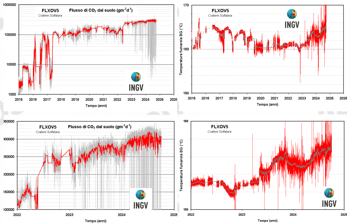
Figura 4.11 – Valori del flusso di \text{CO}_2 dal suolo e della temperatura della fumarola BG misurati dalla stazione FLXOV5 installata nel cratere della Solfatara, a pochi metri dalla fumarola principale BG. I valori di flusso di \text{CO}_2 dal suolo mostrano, in generale, un significativo incremento a partire dal 2016 (la linea rossa si riferisce alle medie giornaliere). Nei cronogrammi in basso sono riportati i valori di flusso di \text{CO}_2 e temperatura a partire da gennaio 2022.
