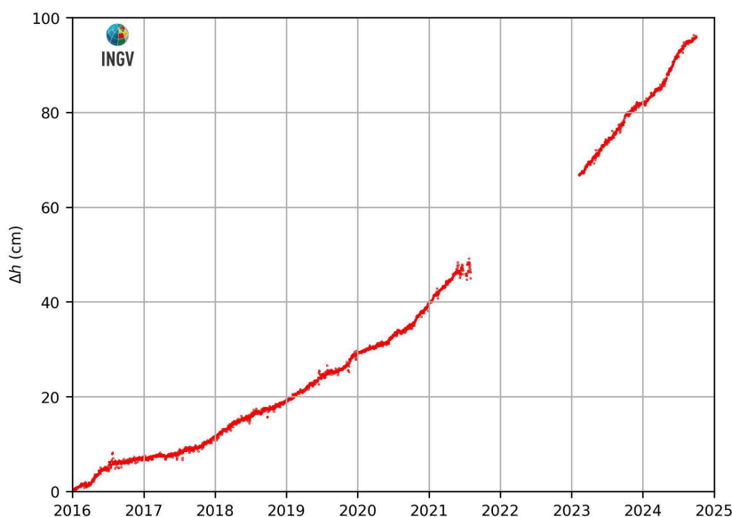
Figura 2.3.2 – Movimenti verticali del suolo, nel periodo gennaio 2016 – settembre 2024, ottenuti dall'analisi dei dati acquisiti dalla stazione mareografica di Pozzuoli Porto (POPT), area centrale della caldera Flegrea. Le variazioni, riportate in cm, rappresentano le medie giornaliere e sono riferite alla stazione mareografica di Napoli, molo San Vincenzo (NAMM).
