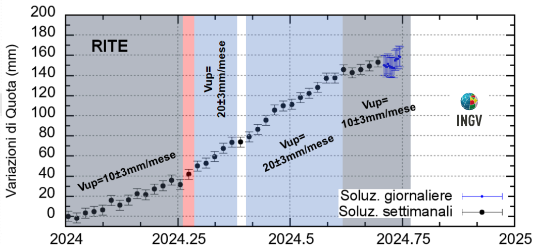
Figura 2.1.2 - Serie temporale delle variazioni in quota della stazione GNSS di RITE dal 01/01/2024 al 29/09/2024. Elaborazione dati in modalità Precise Point Positioning con software PRIDE PPP-AR.
