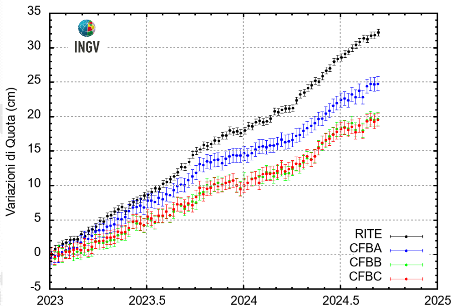
Figura 2.1.6 – Serie temporali delle variazioni settimanali in quota delle stazioni GNSS dell'infrastruttura marina MEDUSA nell'intervallo gennaio 2023 - settembre 2024, confrontate con quella della stazione RITE
