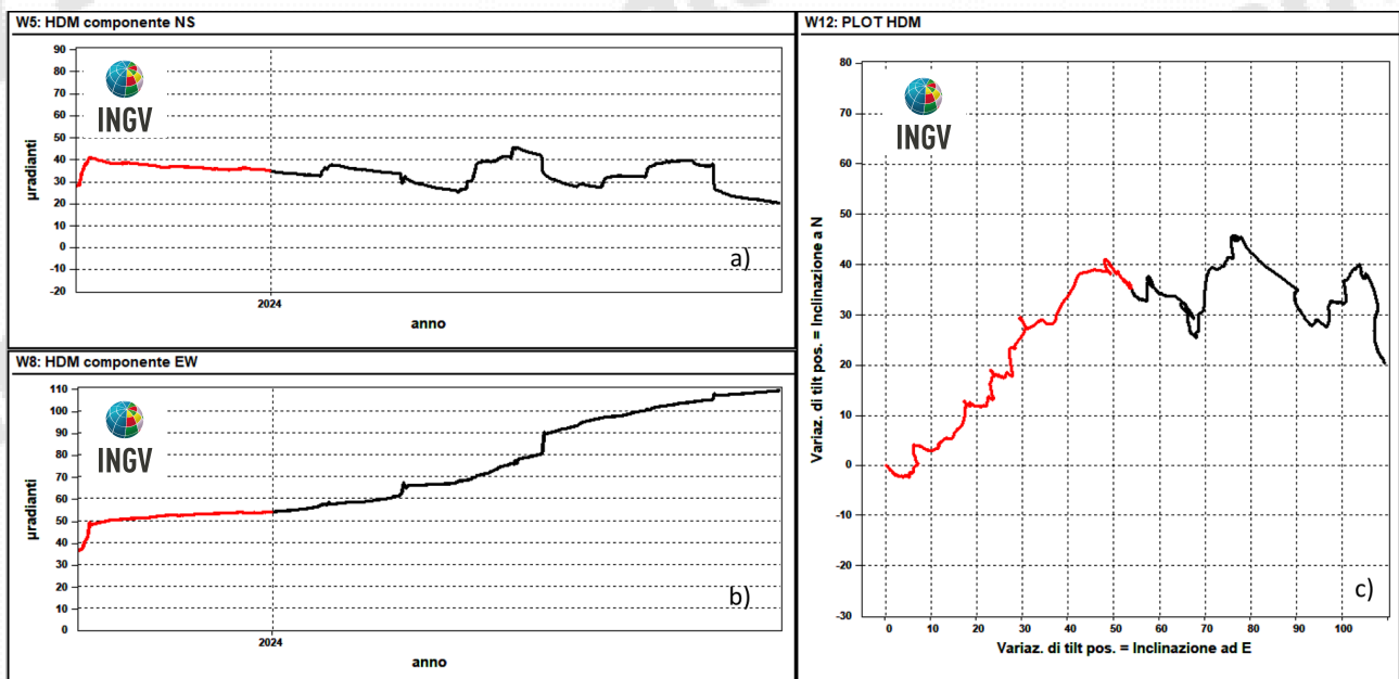
Figura 2.2.3 – Serie temporali e plot del tilt della stazione HDM della rete dei Campi Flegrei registrati negli ultimi 12 mesi (ottobre 2023 - settembre 2024).
