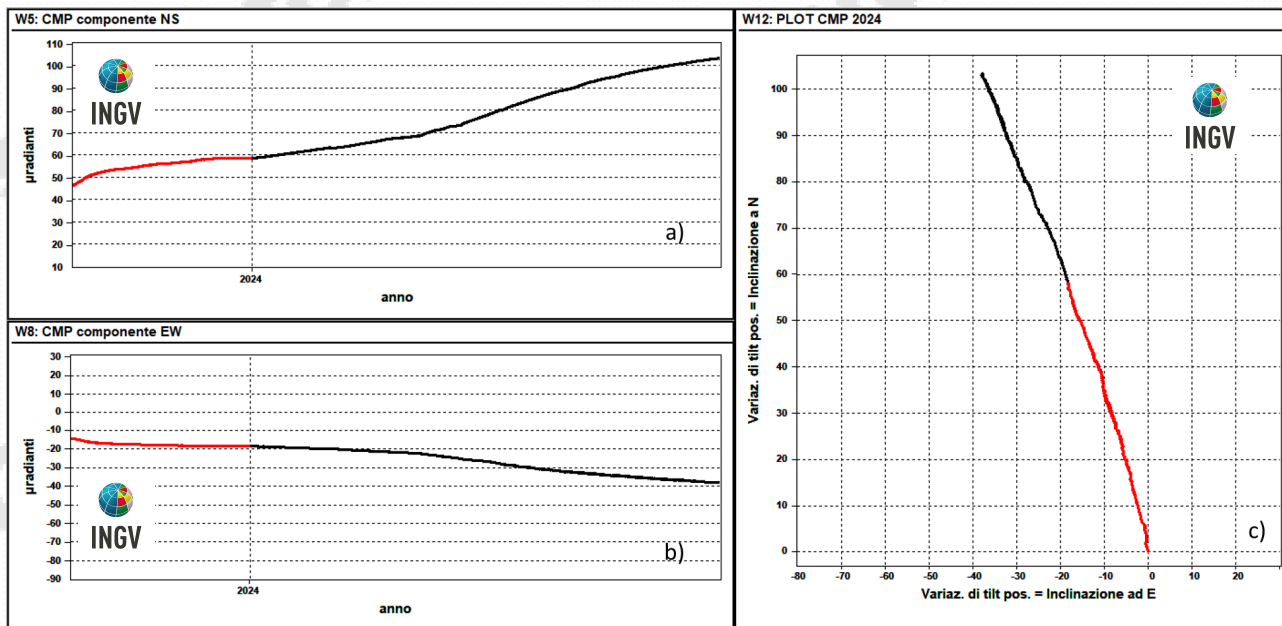
Figura 2.2.3 – Serie temporali e plot del tilt della stazione CMP della rete dei Campi Flegrei registrati negli ultimi 12 mesi (ottobre 2023 - settembre 2024).
