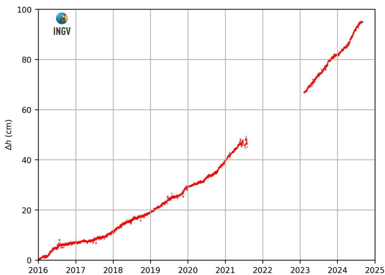
Figura 2.3.2 – Movimenti verticali del suolo, nel periodo gennaio 2016 – agosto 2024, ottenuti dall'analisi dei dati acquisiti dalla stazione mareografica di Pozzuoli Porto (POPT), area centrale della caldera Flegrea. Le variazioni, riportate in cm, rappresentano le medie giornaliere e sono riferite alla stazione mareografica di Napoli, molo San Vincenzo (NAMI).
