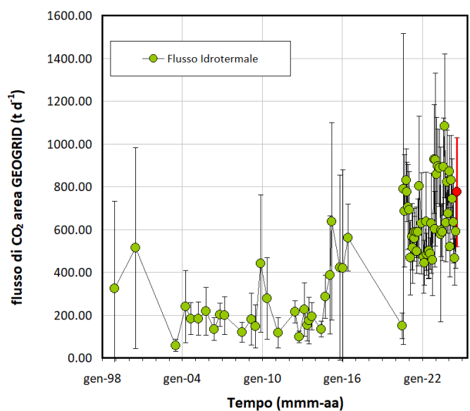
Figura 5.1.2 - Cronogramma dell'output di CO 2 diffuso dal suolo stimato per l'area di interesse. Le misure eseguite ad agosto 2020 hanno mostrato un valore tra i più bassi misurati, mentre quelle successive mostrano un aumento dei valori, con ~750 tonnellate di CO 2 al giorno per le misure di agosto 2024 (simbolo rosso). Le barre verticali rappresentano l'intervallo di confidenza del 95%.
