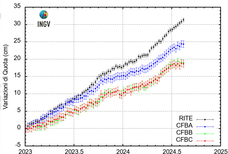
Figura 2.1.7 – Serie temporali delle variazioni settimanali in quota delle stazioni GNSS dell'infrastruttura marina MEDUSA nell'intervallo gennaio 2023 - agosto 2024, confrontate con quella della stazione RITE
