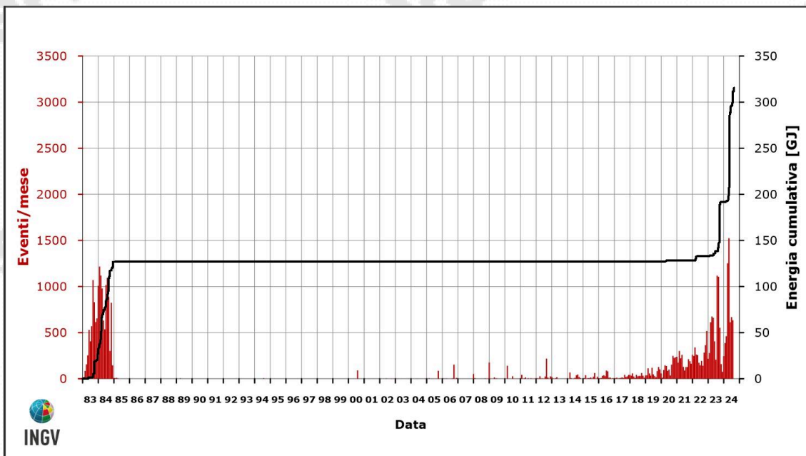
Figura 1.11 – Frequenza di accadimento dei terremoti registrati ai Campi Flegrei dal 1983. La linea nera rappresenta l'energia cumulativa.
