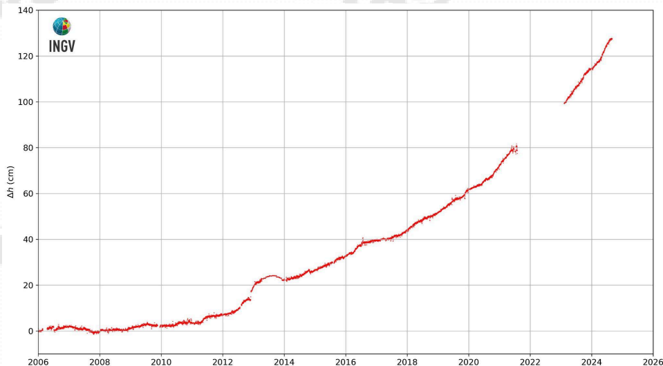
Figura 2.3.3 - Movimenti verticali del suolo nel periodo gennaio 2006 – agosto 2024, ottenuti dall'analisi dei dati acquisiti dalla stazione mareografica di Pozzuoli Porto (POPT) (area centrale della caldera Flegrea). Le variazioni, riportate in cm, rappresentano le medie giornaliere e sono riferite alla stazione mareografica di Napoli, molo San Vincenzo (NAMM).
