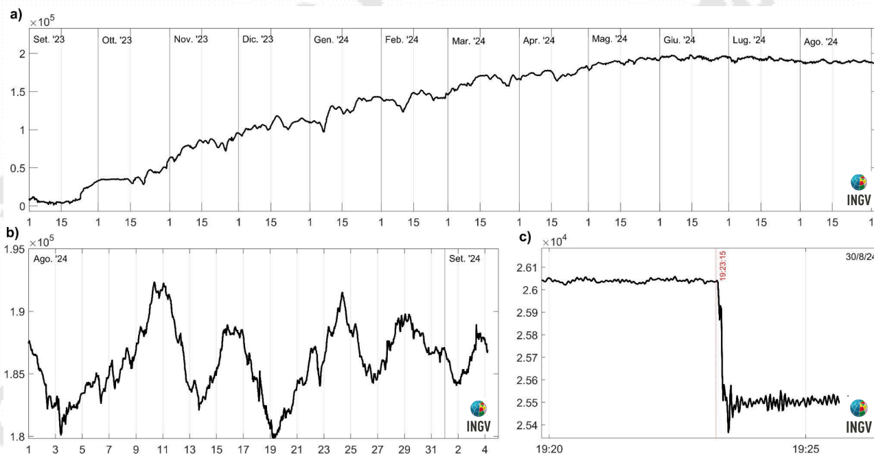
Figura 2.5.2 - a) Strain registrato nell'ultimo anno, dalle 00:00 UTC del 1/8/2023 alle 4:00 UTC del giorno 4/9/2024. b) Strain registrato nell'ultimo mese, dalle 00:00 UTC del giorno 1/8/2024 alle 4:00 UTC del giorno 4/9/2024. c) Variazione dello strain in concomitanza dell'evento di magnitudo maggiore di 3 registrato il 30 agosto
