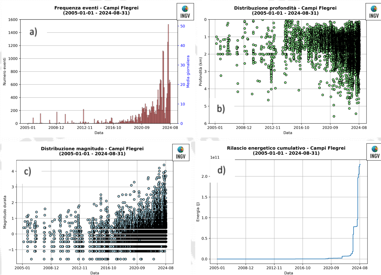
Figura 1.9 - Andamento dei principali parametri sismologici a partire dal 2005: a) frequenza di accadimento; b) profondità ipocentrali; c) magnitudo; d) energia cumulativa.
