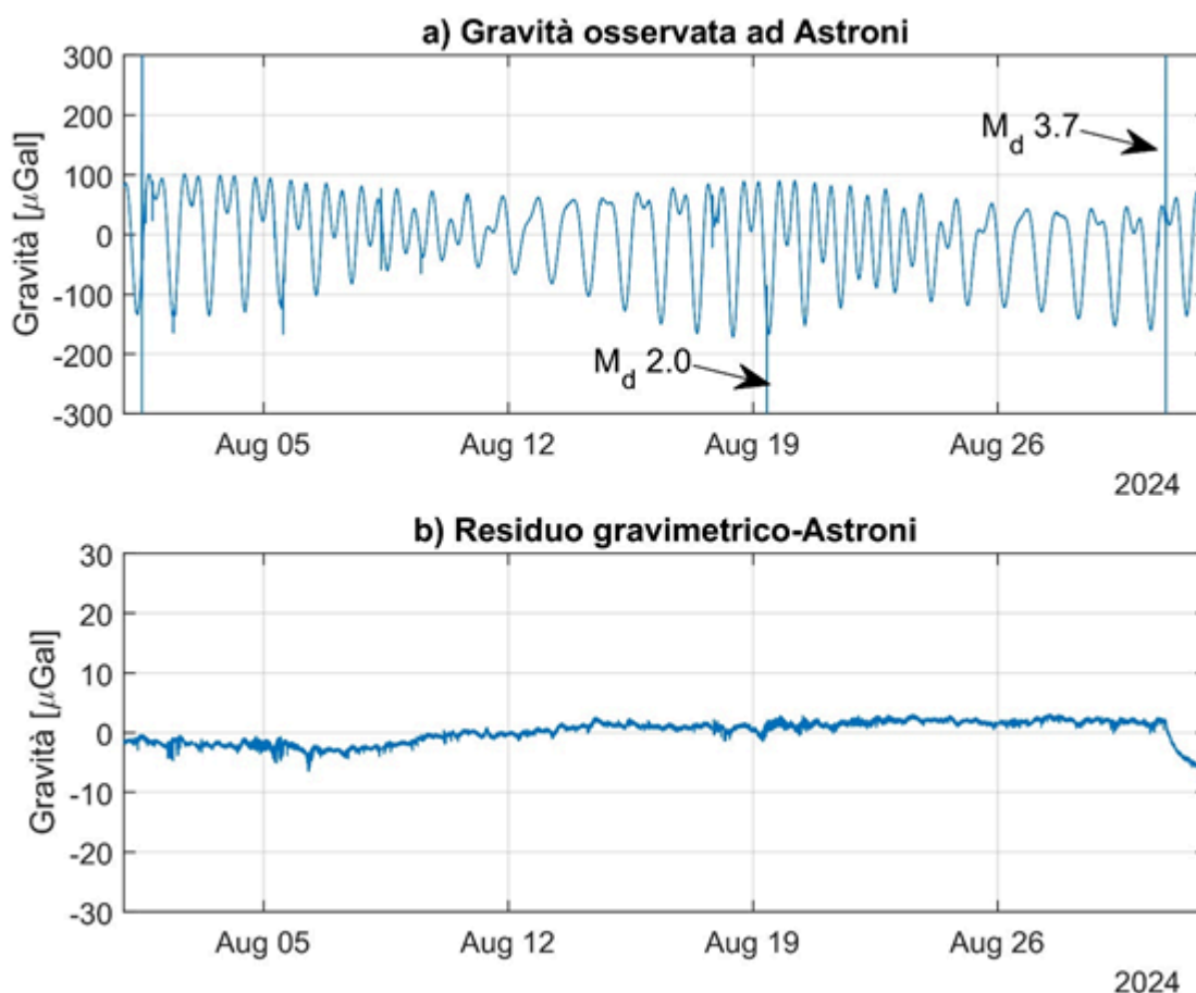
Figura 2.4.1 a: serie temporale (risoluzione temporale 1 minuto) raw registrata dal gPhone. Si osserva il contributo dominante delle maree e di alcuni terremoti avvenuti in area flegrea. b: serie residua di gravità.
