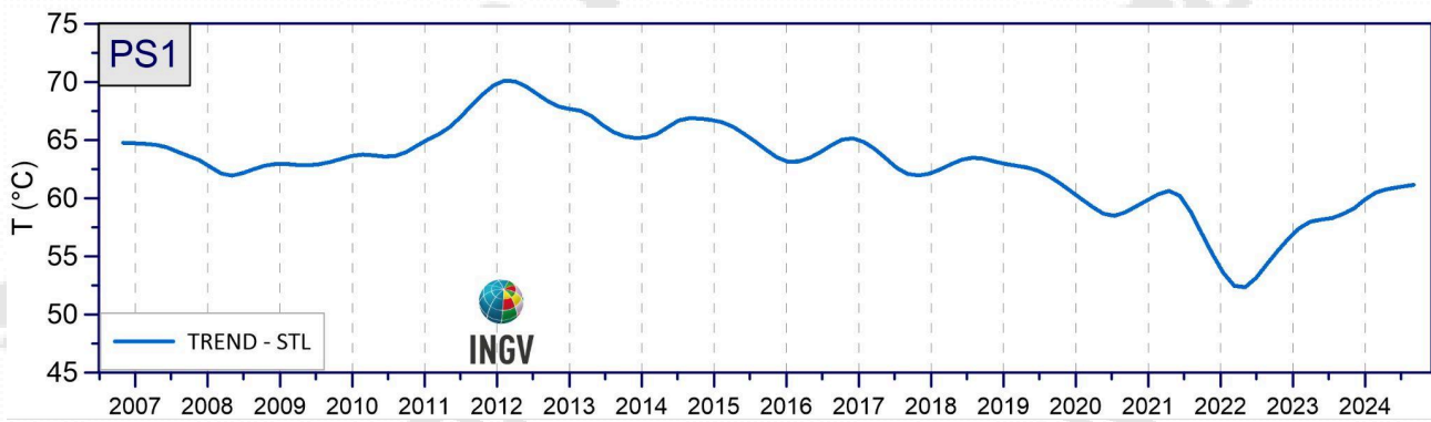
Figura 3.1.4 - Stazione PS1: Trend a lungo termine dei valori di temperatura massima rilevati nelle immagini IR ottenute mediante applicazione dell'algoritmo STL.
