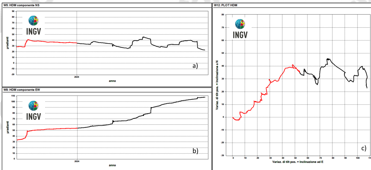
Figura 2.2.3 – Serie temporali e plot del tilt della stazione HDM della rete dei Campi Flegrei registrati negli ultimi 12 mesi (settembre 2023 - agosto 2024).
