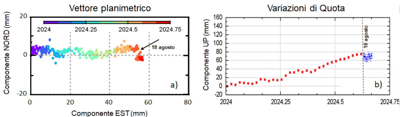
Figura 2.1.6 – Vettore spostamento planimetrico (a) e variazioni in Quota (b) della stazione GNSS di ACAE nel 2024.
