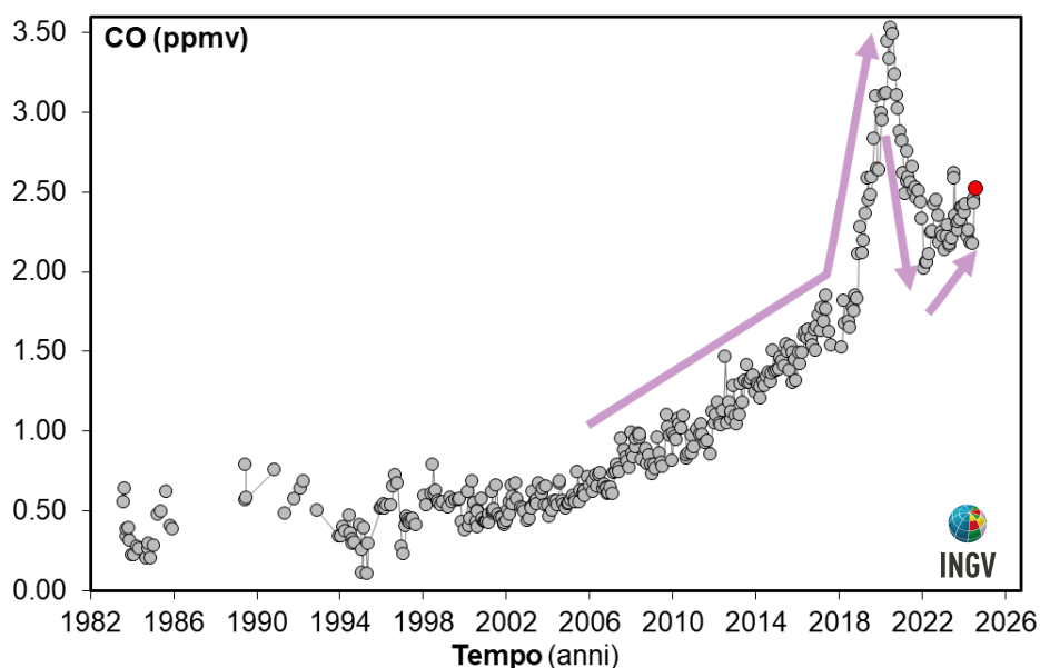
Figura 4.3 – Variazioni della concentrazione di monossido di carbonio (CO) misurato alla fumarola BG a partire dal 1983. Con il simbolo rosso è evidenziato il campione di agosto 2024. In generale alti contenuti di CO caratterizzano sistemi vulcanici a elevata temperatura, mentre fumarole alimentate da sistemi idrotermali mostrano concentrazioni più basse, in tali sistemi un aumento delle concentrazioni di CO può riflettere un incremento delle condizioni di pressione e temperatura.
