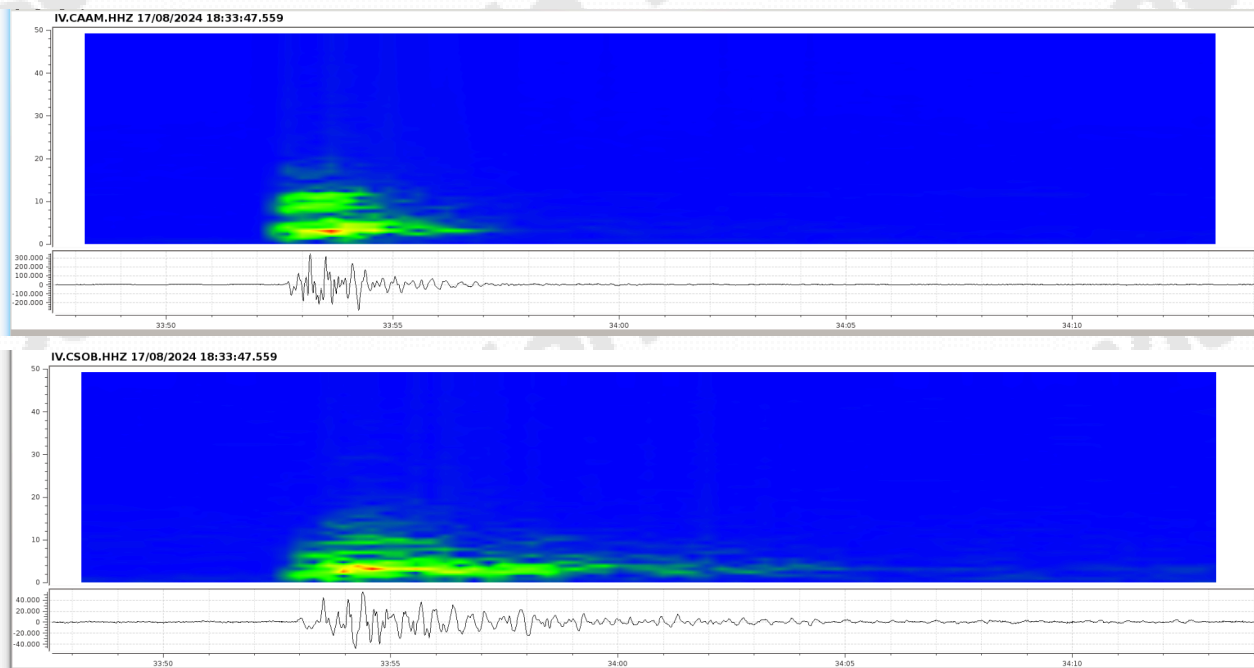
Figura 1.2 - Spettrogramma dell'evento del 17/08/2024 alle 18:33 UTC alle stazioni CAAM e CSOB
