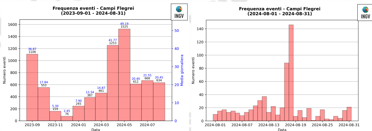
Figura 1.3 - A sinistra numero di eventi registrati ai Campi Flegrei nel corso degli ultimi 12 mesi (in totale 7679), mentre a destra quelli avvenuti nell'ultimo mese (in totale 634).
