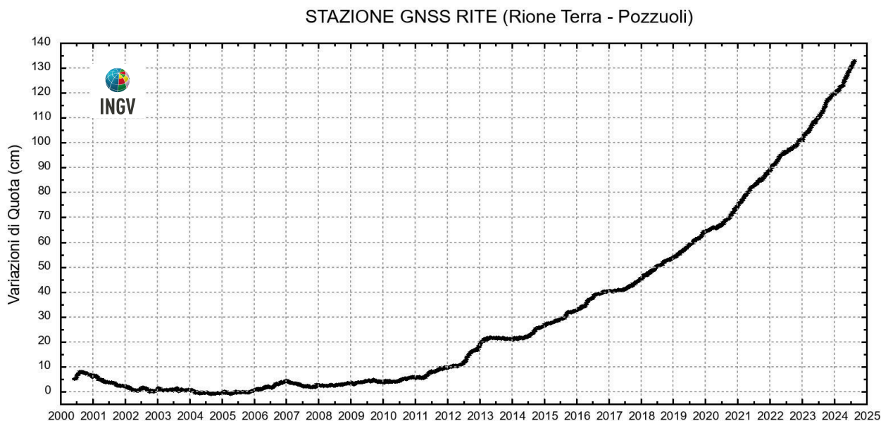
Figura 2.1.4 - Serie temporale delle variazioni settimanali in quota della stazione di RITE (Pozzuoli – Rione Terra) dal 2000 ad agosto 2024.
