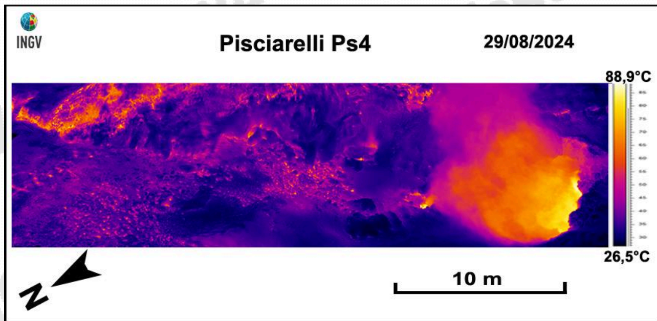
Figura 3.2.2 – Immagine termica, rilevata nel mese di agosto 2024, dell'area denominata Ps4 (Fig.3.2.1b).
