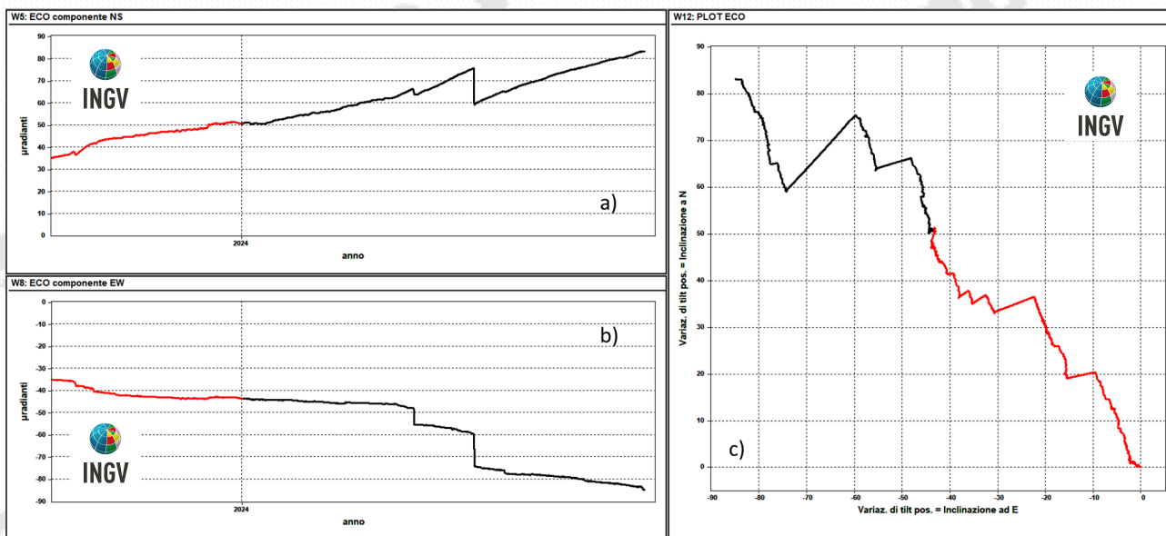
Figura 2.2.2 – Serie temporali e plot del tilt della stazione ECO della rete dei Campi Flegrei registrati negli ultimi 12 mesi (settembre 2023 - agosto 2024).
