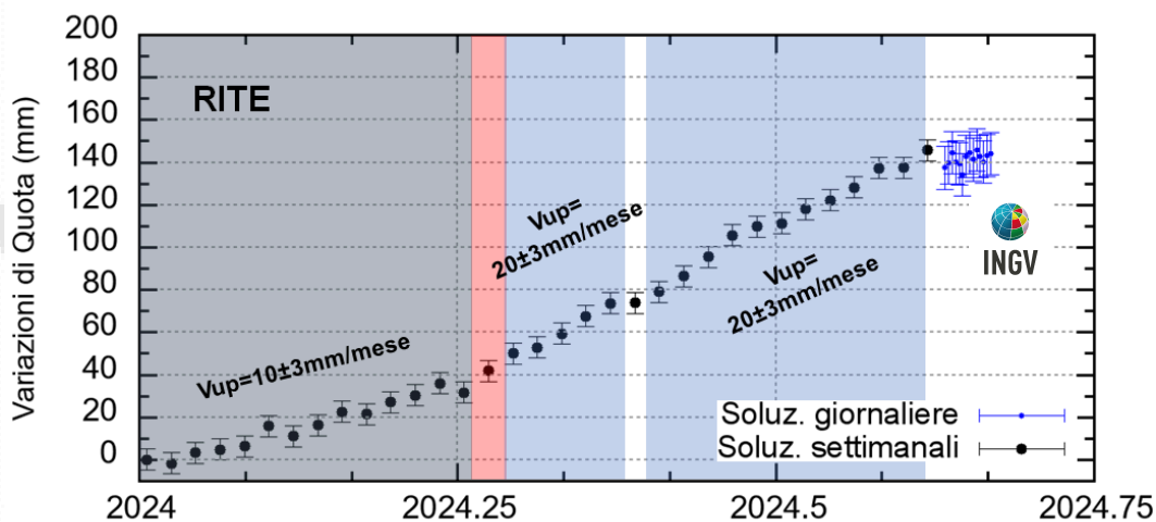
Figura 2.1.2 - Serie temporale delle variazioni in quota della stazione GNSS di RITE dal 01/01/2024 al 01/09/2024. Elaborazione dati in modalità Precise Point Positioning con software PRIDE PPP-AR.
