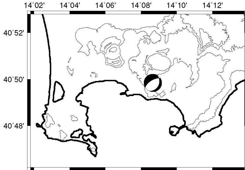
Figura 1.8 - Localizzazione e meccanismo focale dell'evento del 30/08/2024 alle 19:23 UTC Md 3.7( \pm 0.3)
