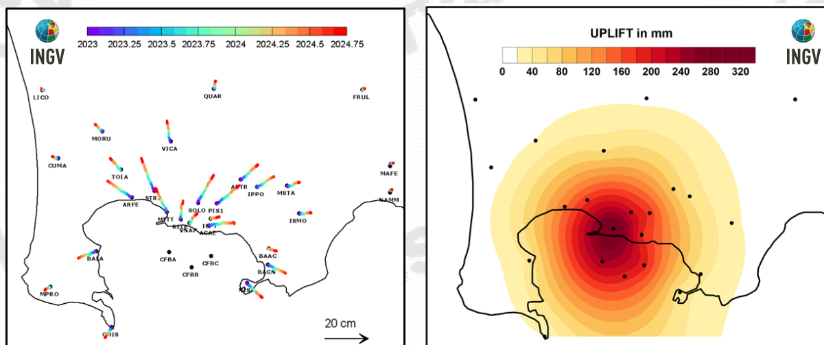
Figura 2.1.5 - Mappa degli spostamenti GNSS orizzontali (a) e verticali (b) registrati nell'area flegrea da gennaio 2023 ad agosto 2024.
