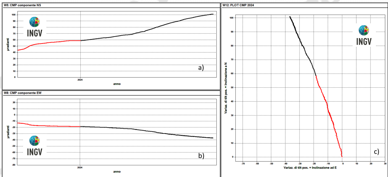
Figura 2.2.3 – Serie temporali e plot del tilt della stazione CMP della rete dei Campi Flegrei registrati negli ultimi 12 mesi (settembre 2023 - agosto 2024).
