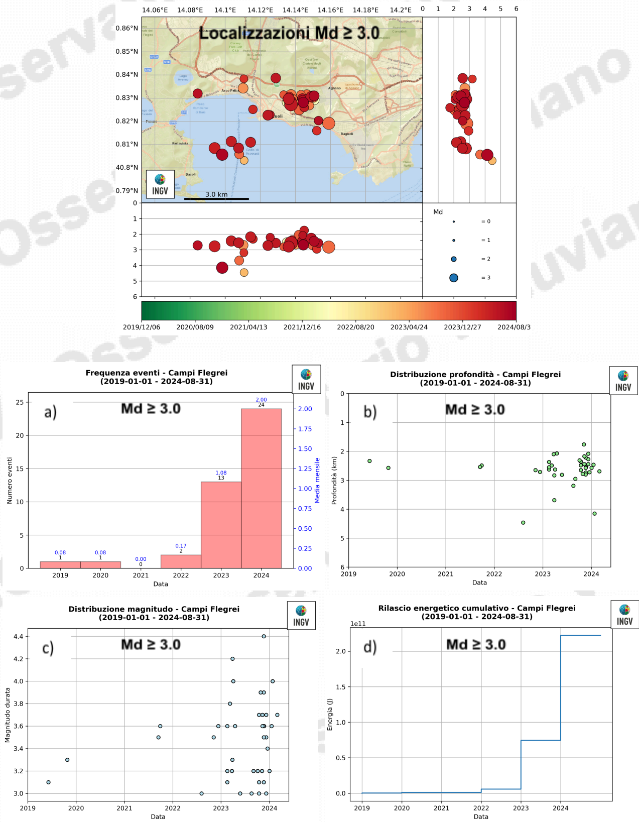
Figura 1.10 - Localizzazioni e andamento dei principali parametri sismologici dei terremoti con Md \geq 3.0 a partire dal 2019: a) frequenza di accadimento; b) profondità ipocentrali; c) magnitudo; d) energia cumulativa.
