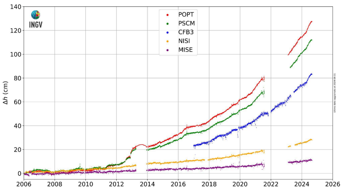
Figura 2.3.4 - Movimenti verticali del suolo nel periodo gennaio 2006 – agosto 2024, ottenuti dall'analisi dei dati acquisiti da tutte le stazioni mareografiche dell'area della caldera Flegrea. Le variazioni, riportate in cm, rappresentano le medie giornaliere e sono tutte riferite alla stazione mareografica di Napoli, molo San Vincenzo (NAMM).
