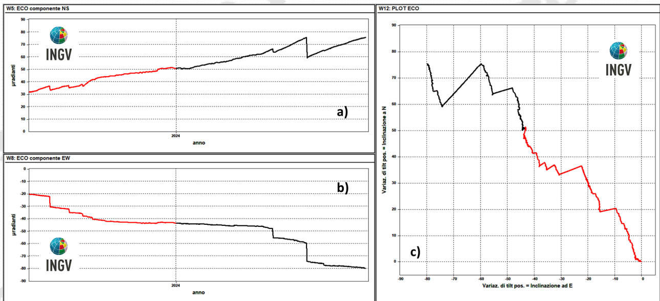
Figura 2.2.2 – Serie temporali e plot del tilt della stazione ECO della rete dei Campi Flegrei registrati negli ultimi 12 mesi (agosto 2023 - luglio 2024).
