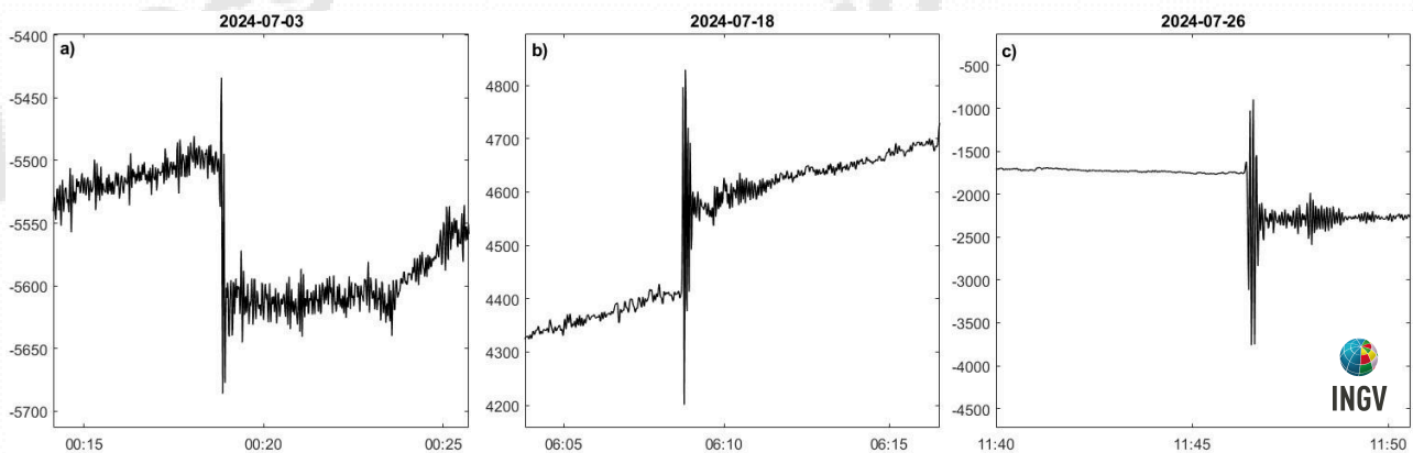
Figura 2.5.3 - a, b, c) Variazione dello strain in concomitanza di 3 eventi di magnitudo maggiori di 3 registrati a luglio.
