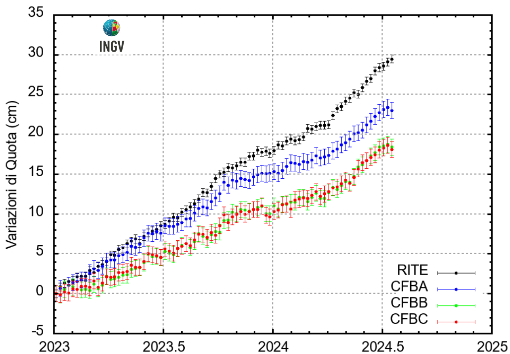
Figura 2.1.6 – Serie temporali delle variazioni settimanali in quota delle stazioni GNSS dell'infrastruttura marina MEDUSA nell'intervallo gennaio 2023 - luglio 2024, confrontate con quella della stazione RITE.
