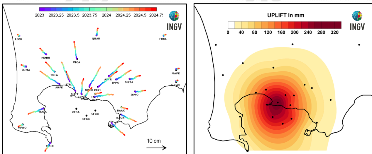
Figura 2.1.5 - Mappa degli spostamenti GNSS orizzontali (a) e verticali (b) registrati nell’area flegrea da gennaio 2023 a luglio 2024.
