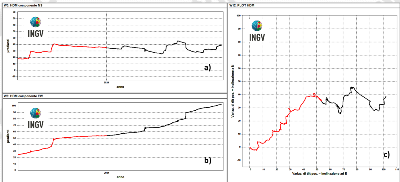
Figura 2.2.3 – Serie temporali e plot del tilt della stazione HDM della rete dei Campi Flegrei registrati negli ultimi 12 mesi (agosto 2023 - luglio 2024).
