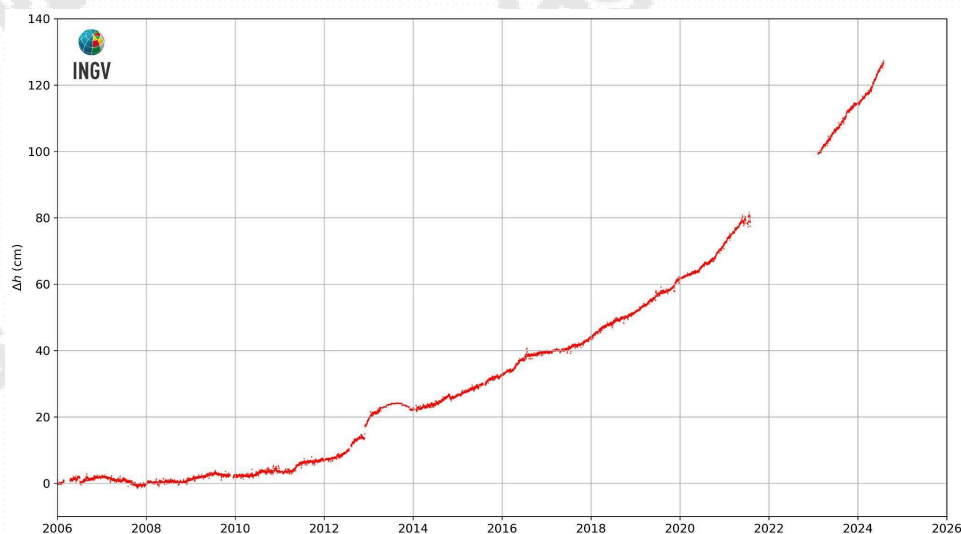
Figura 2.3.3 - Movimenti verticali del suolo nel periodo gennaio 2006 – luglio 2024, ottenuti dall'analisi dei dati acquisiti dalla stazione mareografica di Pozzuoli Porto (POPT) (area centrale della caldera Flegrea). Le variazioni, riportate in cm, rappresentano le medie giornaliere e sono riferite alla stazione mareografica di Napoli, molo San Vincenzo (NAMM).
