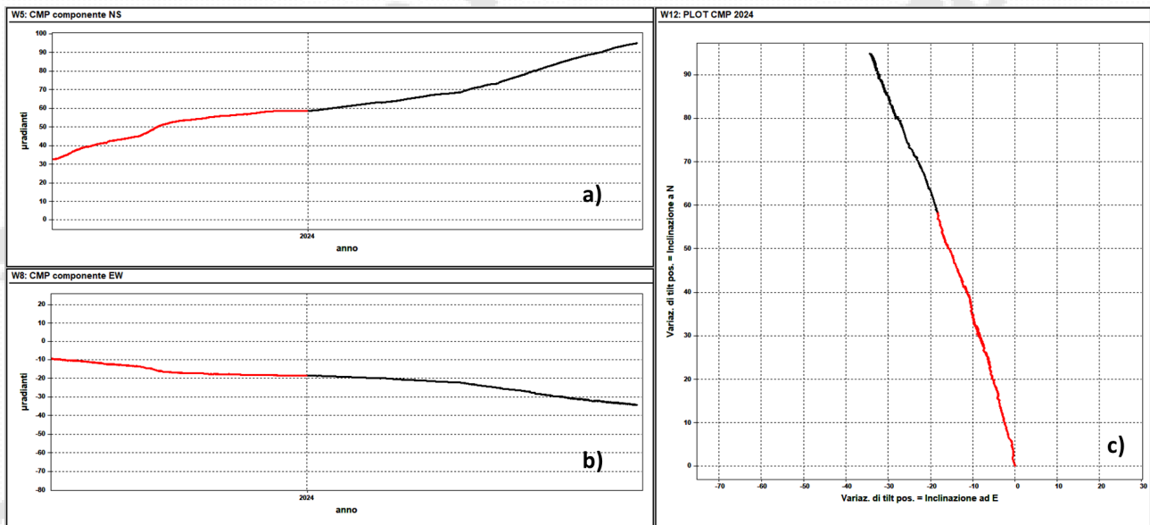
Figura 2.2.3 – Serie temporali e plot del tilt della stazione CMP della rete dei Campi Flegrei registrati negli ultimi 12 mesi (agosto 2023 - luglio 2024).
