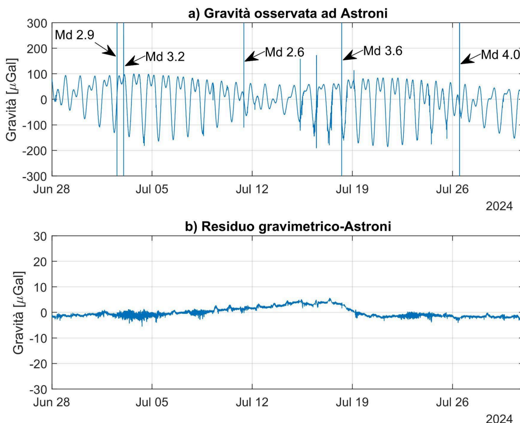
Figura 2.4.1 - a: serie temporale (risoluzione temporale 1 minuto) raw registrata dal gPhone. Si osserva il contributo dominante delle maree e di alcuni terremoti avvenuti in area flegrea. b: serie residua di gravità.
