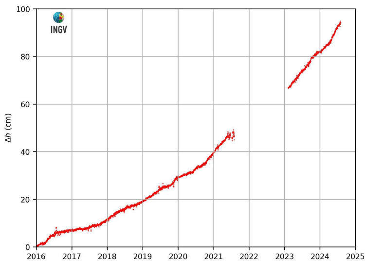
Figura 2.3.2 – Movimenti verticali del suolo, nel periodo gennaio 2016 – luglio 2024, ottenuti dall'analisi dei dati acquisiti dalla stazione mareografica di Pozzuoli Porto (POPT), area centrale della caldera Flegrea. Le variazioni, riportate in cm, rappresentano le medie giornaliere e sono riferite alla stazione mareografica di Napoli, molo San Vincenzo (NAMM).
