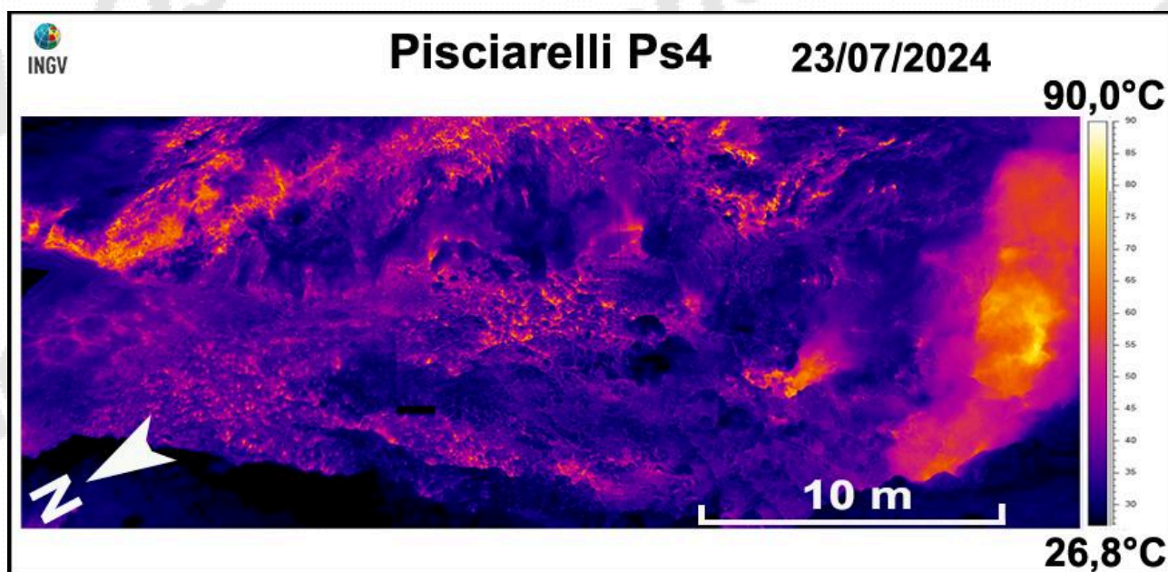
Figura 3.2.2 – Immagine termica, rilevata nel mese di luglio 2024, dell'area denominata Ps4 (Fig.3.2.1b).
