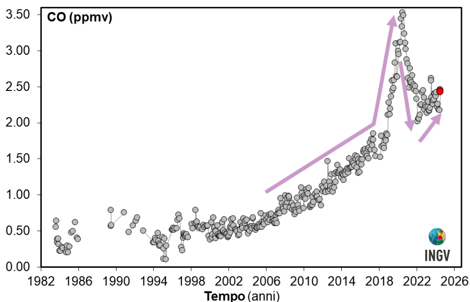
Figura 4.3 – Variazioni della concentrazione di monossido di carbonio (CO) misurato alla fumarola BG a partire dal 1983. Con il simbolo rosso sono evidenziati i campioni di luglio 2024. In generale alti contenuti di CO caratterizzano sistemi vulcanici a elevata temperatura, mentre fumarole alimentate da sistemi idrotermali mostrano concentrazioni più basse, in tali sistemi un aumento delle concentrazioni di CO può riflettere un incremento delle condizioni di pressione e temperatura.
