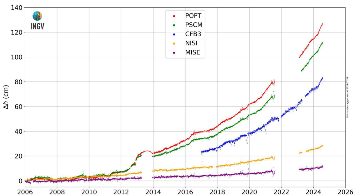
Figura 2.3.4 - Movimenti verticali del suolo nel periodo gennaio 2006 – luglio 2024, ottenuti dall'analisi dei dati acquisiti da tutte le stazioni mareografiche dell'area della caldera Flegrea. Le variazioni, riportate in cm, rappresentano le medie giornaliere e sono tutte riferite alla stazione mareografica di Napoli, molo San Vincenzo (NAMM).
