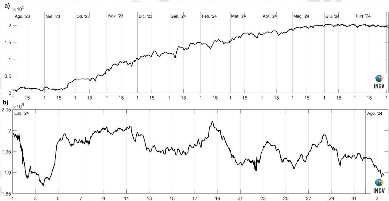
Figura 2.5.2 - a) Strain registrato nell'ultimo anno, dalle 00:00 UTC del 1/7/2023 alle 24:00 UTC del giorno 1/8/2024. b) Strain registrato nell'ultimo mese, dalle 00:00 UTC del giorno 2/8/2024 alle 15:00 UTC del giorno 6/7/2024.
