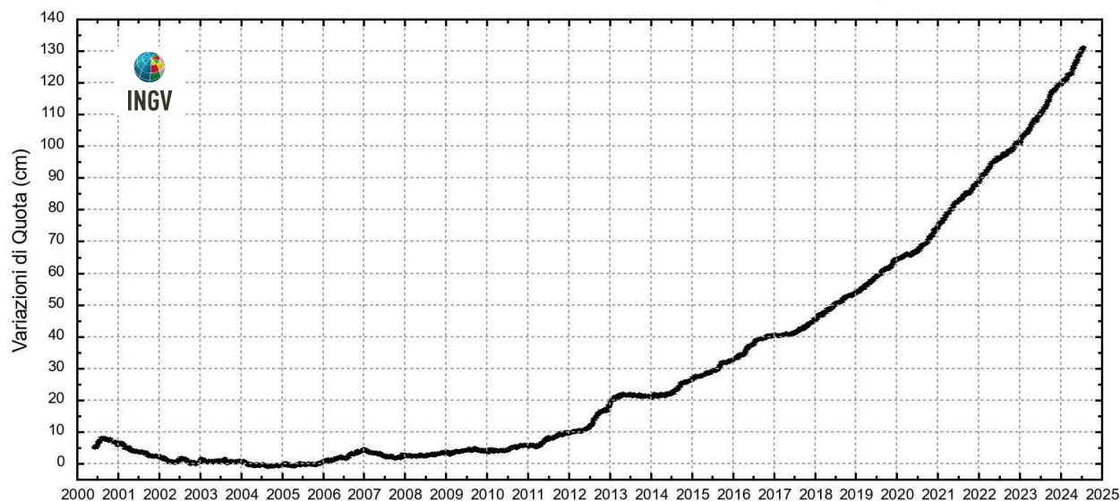
Figura 2.1.4 - Serie temporale delle variazioni settimanali in quota della stazione di RITE (Pozzuoli – Rione Terra) dal 2000 a luglio 2024.
