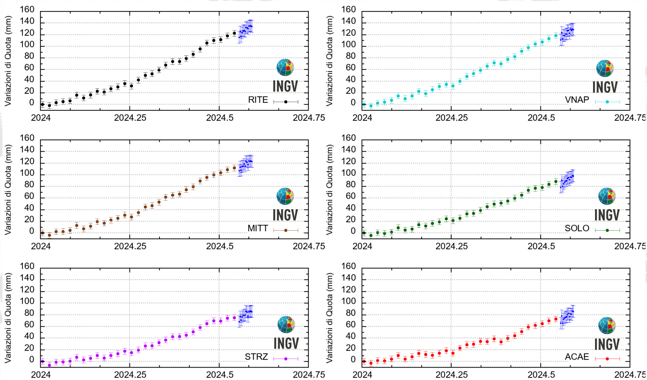
Figura 2.1.3 - Serie temporali delle variazioni in quota delle stazioni di RITE (Pozzuoli - Rione Terra), VNAP (Pozzuoli - Via Napoli), MITT (Pozzuoli - Porto), SOLO (Solfatara), STRZ (Pozzuoli - Cimitero) e ACAE (Accademia Aeronautica) dal 01/01/2024 al 04/08/2024. Elaborazione dati in modalità Precise Point Positioning con software PRIDE PPP-AR.
