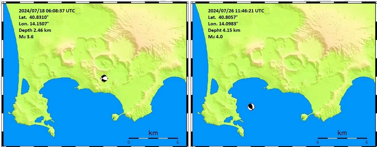
Figura 1.7 - Localizzazione e meccanismo focale dell'evento del 18/07/2024 alle 06:08 UTC Md 3.6(±0.3) (a sinistra) e dell'evento del 26/07/2024 alle 11:46 UTC Md 4.0(±0.3) (a destra)
