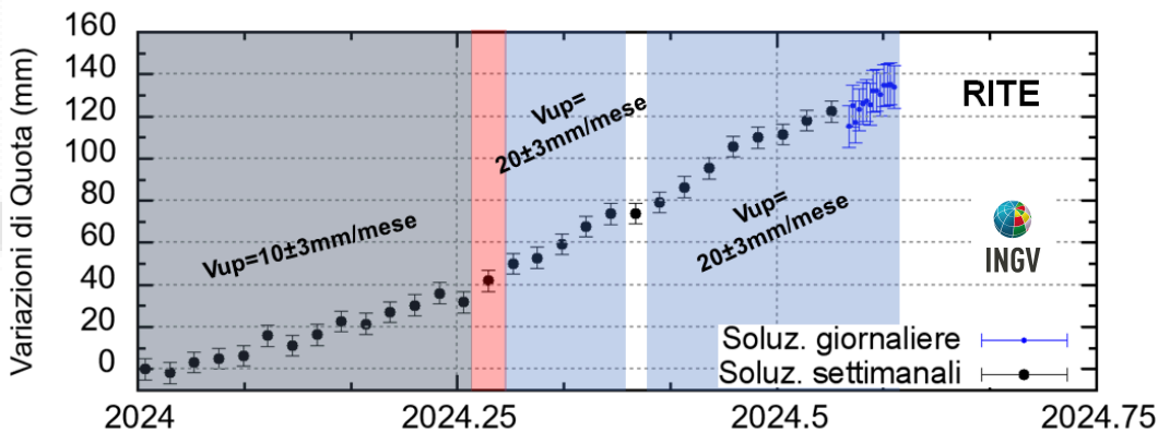
Figura 2.1.2 - Serie temporale delle variazioni in quota della stazione GNSS di RITE dal 01/01/2024 al 04/08/2024. Elaborazione dati in modalità Precise Point Positioning con software PRIDE PPP-AR.
