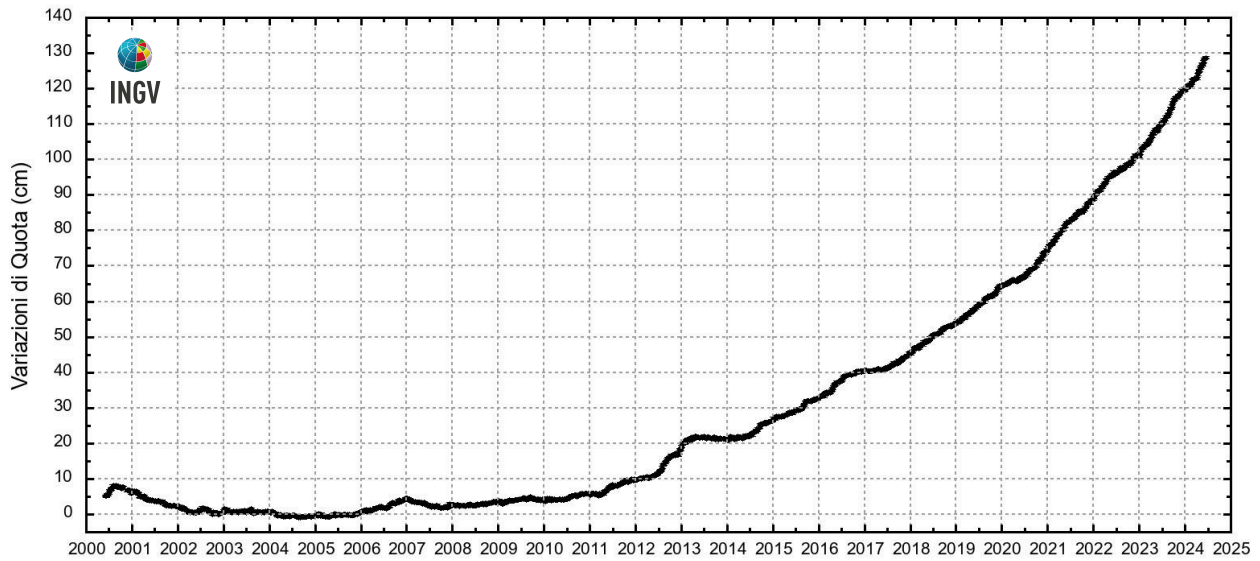
Figura 2.1.4 - Serie temporale delle variazioni settimanali in quota della stazione di RITE (Pozzuoli – Rione Terra) dal 2000 a giugno 2024.
