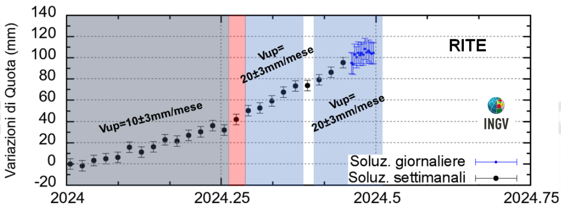
Figura 2.1.2 - Serie temporale delle variazioni in quota della stazione GNSS di RITE dal 01/01/2024 al 30/06/2024. Elaborazione dati in modalità Precise Point Positioning con software PRIDE PPP-AR.
