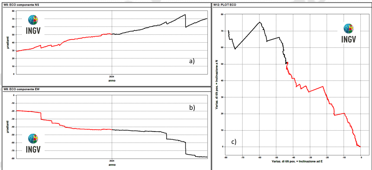
Figura 2.2.2 – Serie temporali e plot del tilt della stazione ECO della rete dei Campi Flegrei registrati negli ultimi 12 mesi (luglio 2023 - giugno 2024).
