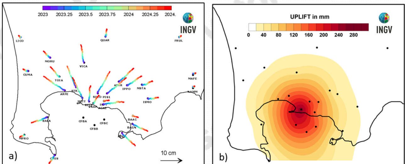
Figura 2.1.5 - Mappa degli spostamenti GNSS orizzontali (a) e verticali (b) registrati nell’area flegrea da gennaio 2023 a giugno 2024.
