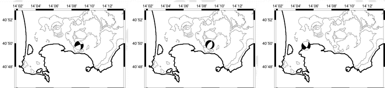
Figura 1.8 - Localizzazione e meccanismo focale dell'evento del 08/06/2024 alle 01:52 UTC Md 3.6(±0.3) (a sinistra), del 08/06/2024 alle 02:09 UTC Md 3.7(±0.3) (al centro) e del 18/06/2024 alle 01:58 UTC Md 3.4(±0.3) (a destra)
