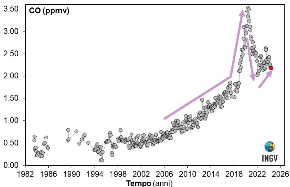
Figura 4.3 – Variazioni della concentrazione di monossido di carbonio (CO) misurato alla fumarola BG a partire dal 1983. Con il simbolo rosso è evidenziato il campione di giugno 2024. In generale alti contenuti di CO caratterizzano sistemi vulcanici a elevata temperatura, mentre fumarole alimentate da sistemi idrotermali mostrano concentrazioni più basse, in tali sistemi un aumento delle concentrazioni di CO può riflettere un incremento delle condizioni di pressione e temperatura.
