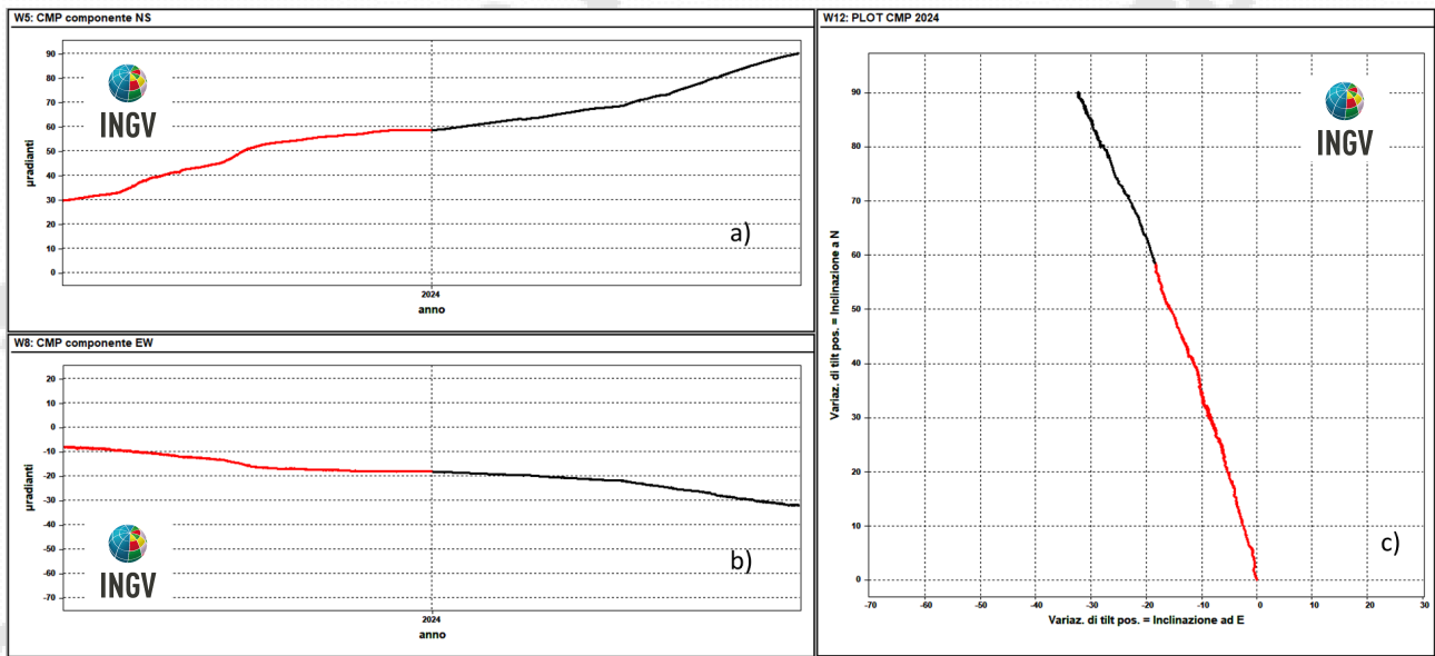
Figura 2.2.3 – Serie temporali e plot del tilt della stazione CMP della rete dei Campi Flegrei registrati negli ultimi 12 mesi ((luglio 2023 - giugno 2024).
