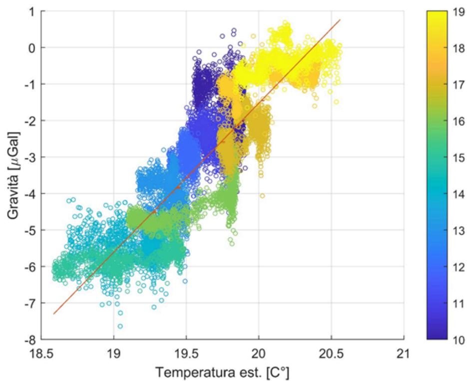
Figura 2.4.2 - Correlazione Temperatura ambientale vs. variazione di gravità nel periodo 10-19 Giugno. Il codice colore dei punti riporta una scala temporale, in particolare le giornate di Giugno. La retta riporta la relazione lineare che meglio approssima i dati ( R^2=0.75 )
