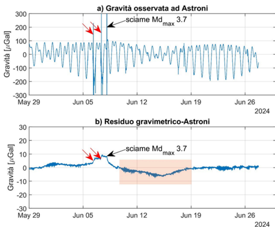
Figura 2.4.1 - a: serie temporale (passo di campionamento: 1 minuto) raw registrata dal gPhone. Si osserva il contributo dominante delle maree. L'inizio dello sciame del 8/6/2024 con magnitudo max 3.7 Md è riportato con la freccia nera; disturbi di probabile origine antropica sono riportati con le frecce rosse. b: serie residua di gravità. La banda arancio riporta un transiente residuo, per la cui interpretazione si rimanda al testo.
