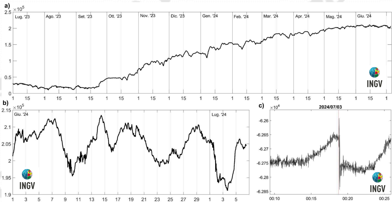
Figura 2.5.2 - a) Strain registrato nell'ultimo anno, dalle 00:00 UTC del 1/6/2023 alle 24:00 UTC del giorno 5/7/2024. b) Strain registrato nell'ultimo mese, dalle 00:00 UTC del giorno 1/6/2024 alle 13:00 UTC del giorno 6/7/2024. c) Variazione dello strain in concomitanza dell'evento del 3/7/2024 di magnitudo 3.2.
