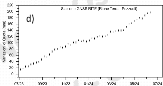
Figura 6.1 – Frequenza di accadimento degli eventi sismici (a), variazioni del flusso di CO 2 alla stazione geochimica di Pisciarelli (b), trend delle temperature massime superficiali destagionalizzate delle telecamera all'infrarosso termico a Pisciarelli (c) e andamento delle deformazioni del suolo alla stazione GNSS di RITE (d), negli ultimi dodici mesi (a sinistra) e dal 2014 (a destra).
