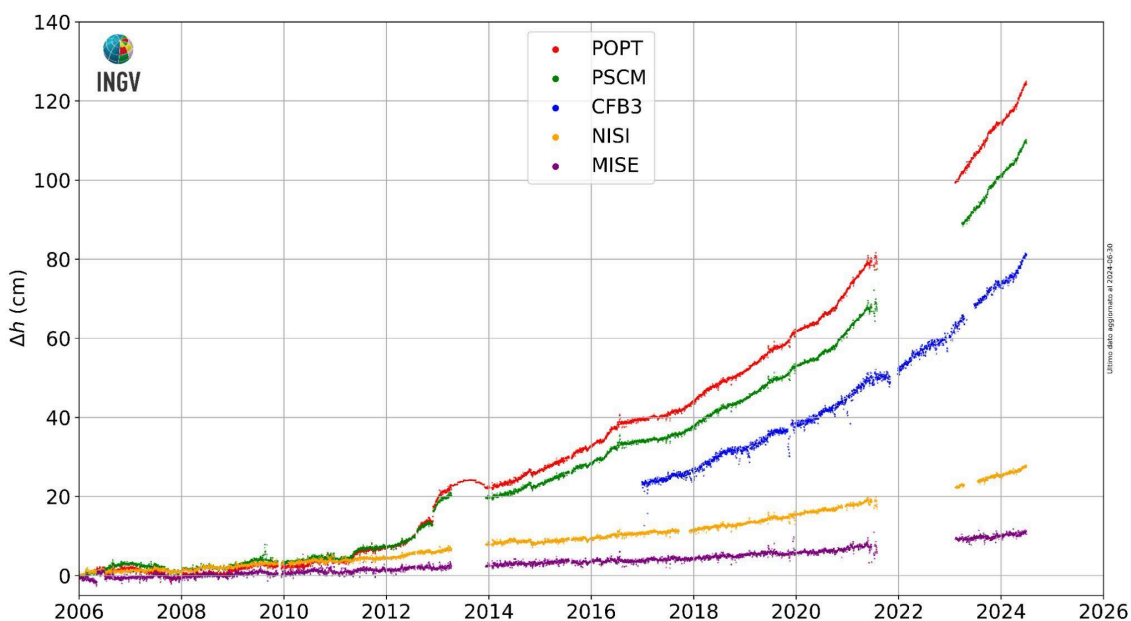
Figura 2.3.4 - Movimenti verticali del suolo nel periodo gennaio 2006 – giugno 2024, ottenuti dall'analisi dei dati acquisiti da tutte le stazioni mareografiche dell'area della caldera Flegrea. Le variazioni, riportate in cm, rappresentano le medie giornaliere e sono tutte riferite alla stazione mareografica di Napoli, molo San Vincenzo (NAMM).
