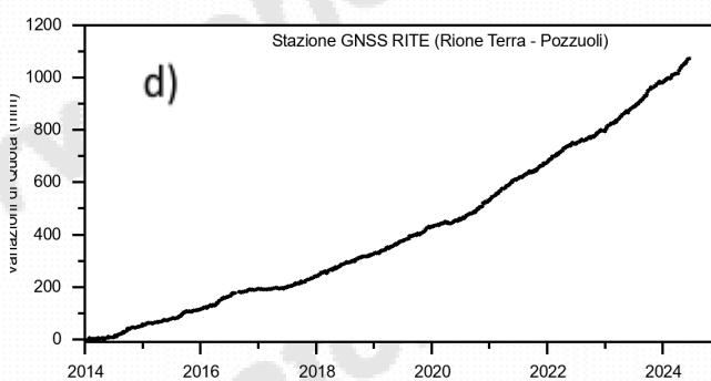
Figura 6.1 – Frequenza di accadimento degli eventi sismici (a), variazioni del flusso di CO 2 alla stazione geochimica di Pisciarelli (b), trend delle temperature massime superficiali destagionalizzate delle telecamera all'infrarosso termico a Pisciarelli (c) e andamento delle deformazioni del suolo alla stazione GNSS di RITE (d), negli ultimi dodici mesi (a sinistra) e dal 2014 (a destra).
