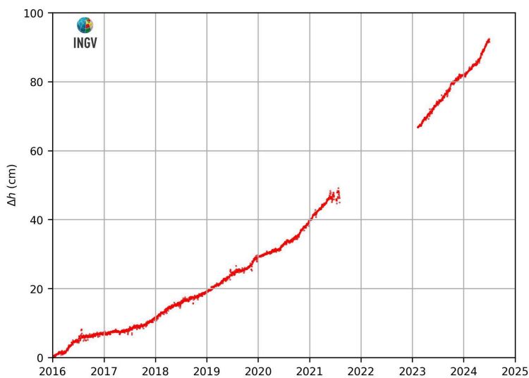
Figura 2.3.2 – Movimenti verticali del suolo, nel periodo gennaio 2016 – giugno 2024, ottenuti dall'analisi dei dati acquisiti dalla stazione mareografica di Pozzuoli Porto (POPT), area centrale della caldera Flegrea. Le variazioni, riportate in cm, rappresentano le medie giornaliere e sono riferite alla stazione mareografica di Napoli, molo San Vincenzo (NAMI).
