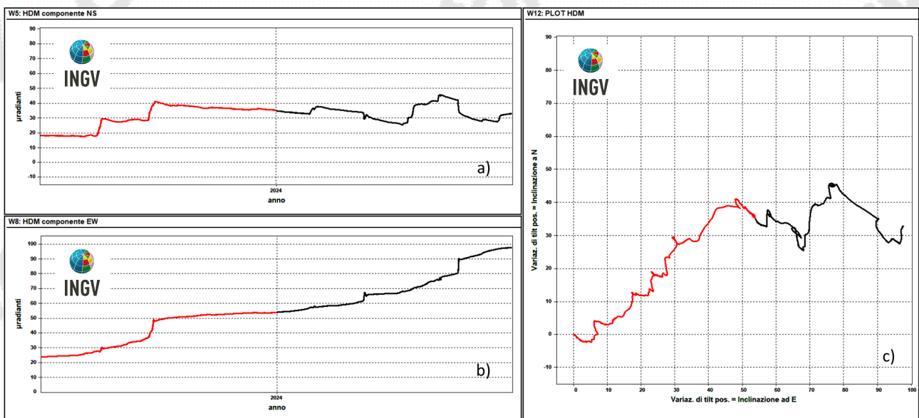
Figura 2.2.3 – Serie temporali e plot del tilt della stazione HDM della rete dei Campi Flegrei registrati negli ultimi 12 mesi ((luglio 2023 - giugno 2024).
