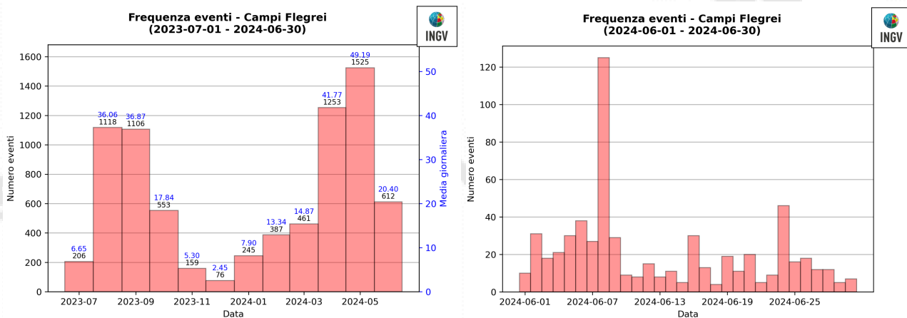
Figura 1.2 - A sinistra numero di eventi registrati ai Campi Flegrei nel corso degli ultimi 12 mesi (in totale 7701), mentre a destra quelli avvenuti nell'ultimo mese (in totale 612).
