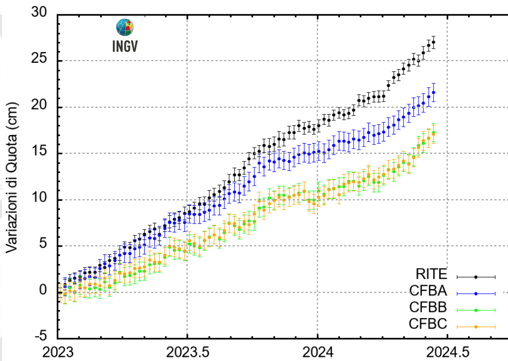
Figura 2.1.6 – Serie temporali delle variazioni settimanali in quota delle stazioni GNSS dell'infrastruttura marina MEDUSA nell'intervallo gennaio 2023 - giugno 2024, confrontate con quella della stazione RITE.
