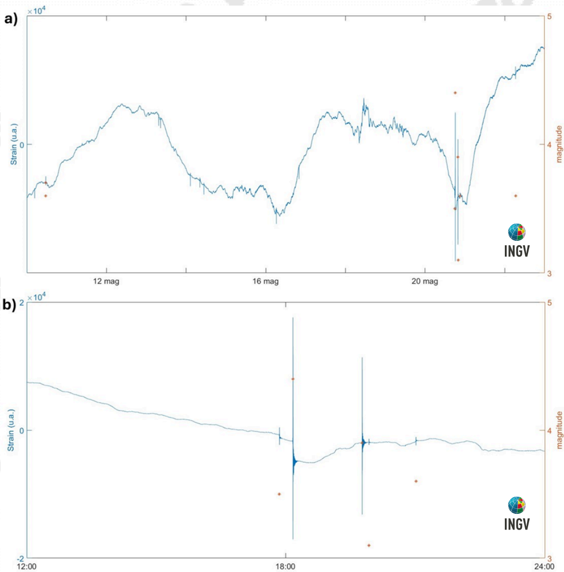
Figura 2.5.4 - a) Confronto tra la variazione di strain registrata alla stazione MRUS, e l'accadimento di eventi con magnitudo superiore a 3 nei giorni precedenti e successivi allo sciame del 20 maggio 2024. b) Variazione dello strain in concomitanza dello sciame del 20 maggio. Si registra una variazione cosismica dello strain per l'evento di magnitudo 4.4.
