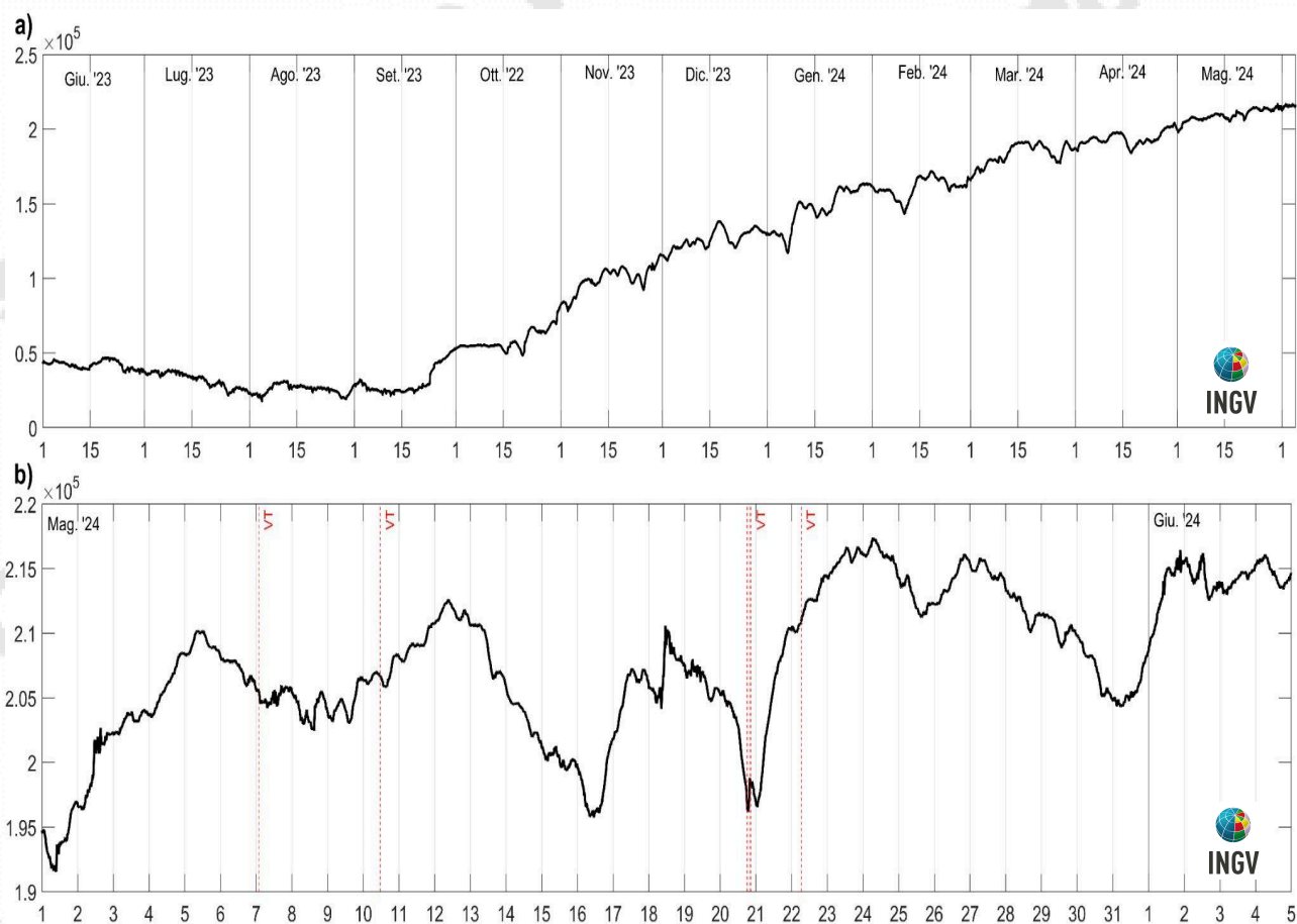
Figura 2.5.2 - a) Strain registrato nell'ultimo anno, dalle 00:00 UTC del 1/6/2023 alle 24:00 UTC del giorno 4/6/2024. b) Strain registrato nell'ultimo mese, dalle 00:00 UTC del giorno 1/5/2024 alle 24:00 UTC del giorno 4/5/2024. Le linee verticali rosse segnalano l'accadimento di terremoti (VT) di magnitudo durata maggiore di 3.
