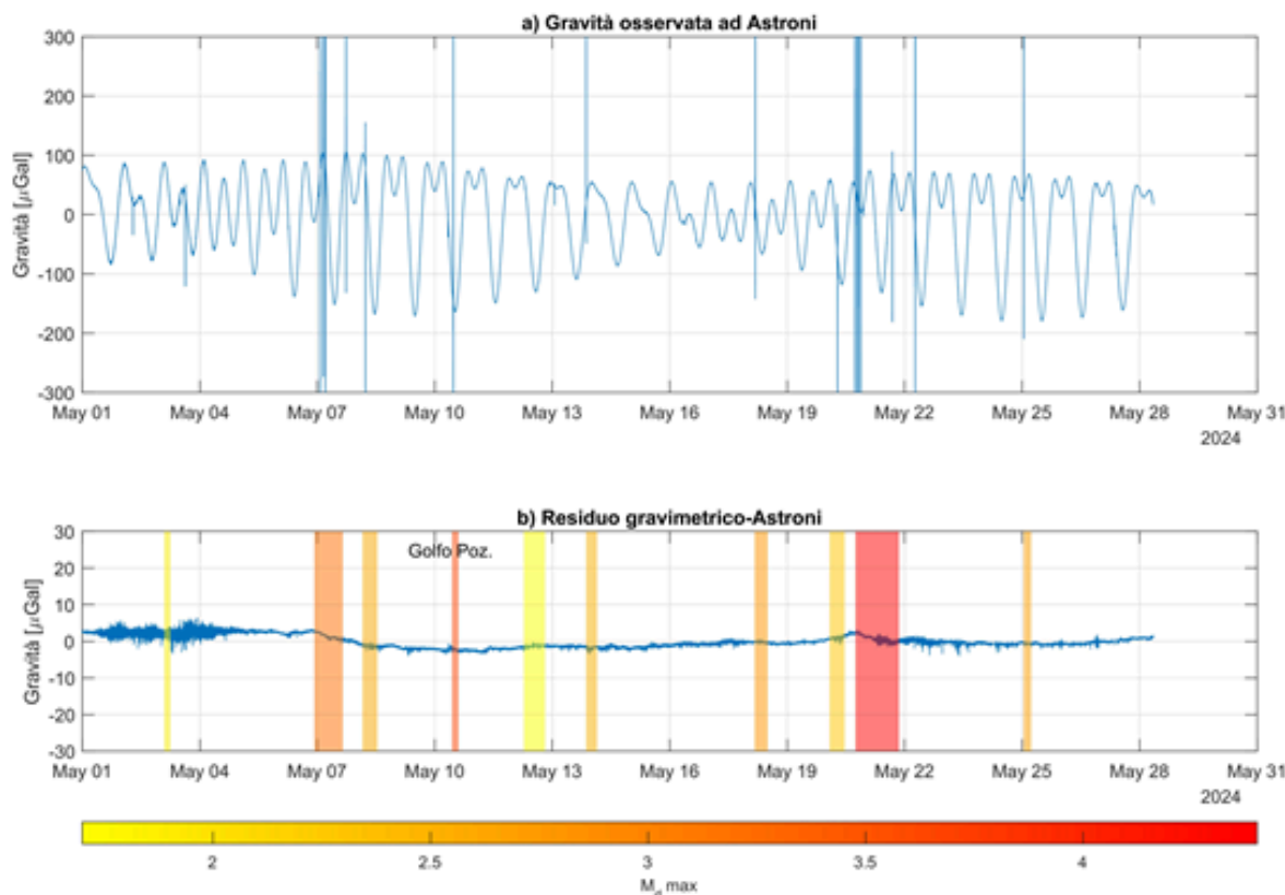
Figura 2.4.3 a: serie temporale (risoluzione temporale 1 minuto) raw registrata dal gPhone. Si osserva il contributo dominante delle maree. b: serie residua di gravità dove le bande verticali colorate individuano inizio e fine degli sciame. Il colore è proporzionale alla magnitudo massima dello sciame. Golfo Poz. indica uno sciame avvenuto a mare i rimanenti sono localizzati prevalentemente nell'area compresa tra Pozzuoli, Solfatara-Pisciarelli e Accademia.
