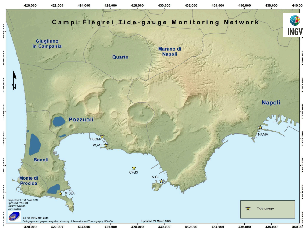
Figura 2.3.1 - Rete Mareografica dei Campi Flegrei.
