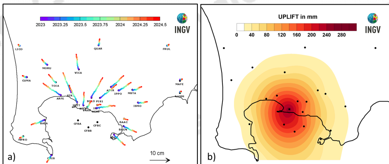
Figura 2.1.5 - Mappa degli spostamenti GNSS orizzontali (a) e verticali (b) registrati nell'area flegrea da gennaio 2023 a maggio 2024.
