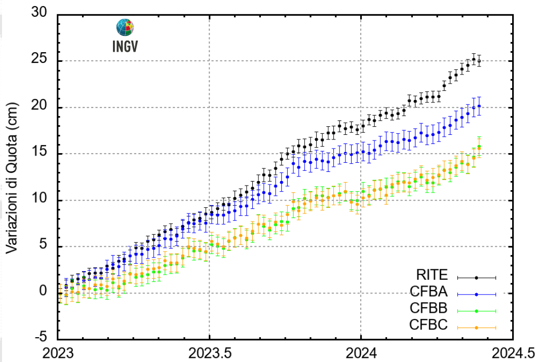
Figura 2.1.6 – Serie temporali delle variazioni settimanali in quota delle stazioni GNSS dell'infrastruttura marina MEDUSA nell'intervallo gennaio 2023 - maggio 2024, confrontate con quella della stazione RITE.
