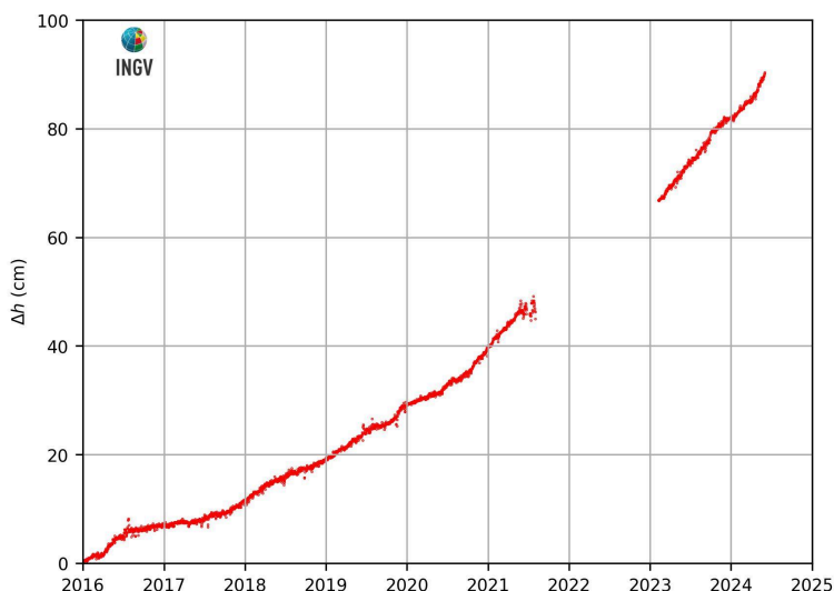
Figura 2.3.2 – Movimenti verticali del suolo, nel periodo gennaio 2016 – maggio 2024, ottenuti dall'analisi dei dati acquisiti dalla stazione mareografica di Pozzuoli Porto (POPT), area centrale della caldera Flegrea. Le variazioni, riportate in cm, rappresentano le medie giornaliere e sono riferite alla stazione mareografica di Napoli, molo San Vincenzo (NAMI).
