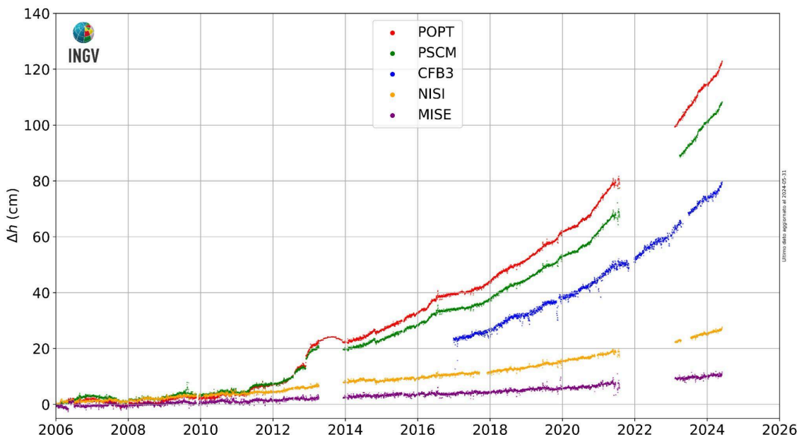
Figura 2.3.4 - Movimenti verticali del suolo nel periodo gennaio 2006 – maggio 2024, ottenuti dall'analisi dei dati acquisiti da tutte le stazioni mareografiche dell'area della caldera Flegrea. Le variazioni, riportate in cm, rappresentano le medie giornaliere e sono tutte riferite alla stazione mareografica di Napoli, molo San Vincenzo (NAMM).
