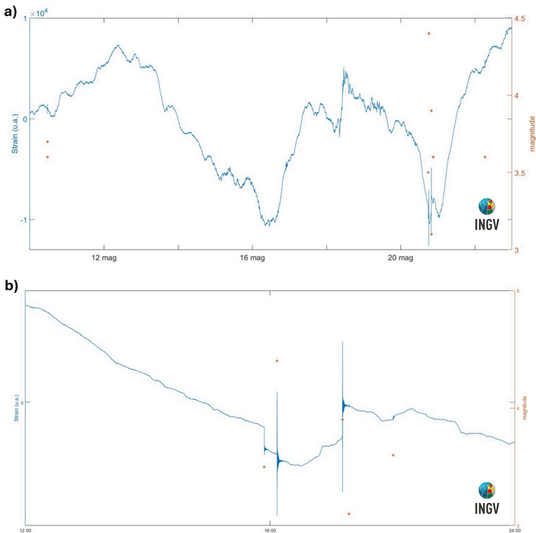
Figura 2.5.3 - a) Confronto tra la variazione di strain registrata alla stazione QUAR, e l'accadimento di eventi con magnitudo superiore a 3 nei giorni precedenti e successivi allo sciame del 20 maggio 2024. b) Variazione dello strain in concomitanza dello sciame del 20 maggio. Si registra una variazione cosismica dello strain per gli eventi di magnitudo 4.4, 3.9 e 3.5.
