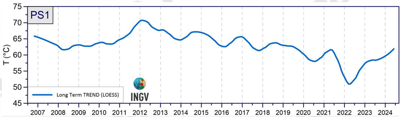
Figura 3.1.4 - Stazione PS1: Trend a lungo termine dei valori di temperatura massima rilevati nelle immagini IR ottenute mediante applicazione di fitting LOESS di 2° alle temperature massime destagionalizzate con algoritmo STL.
