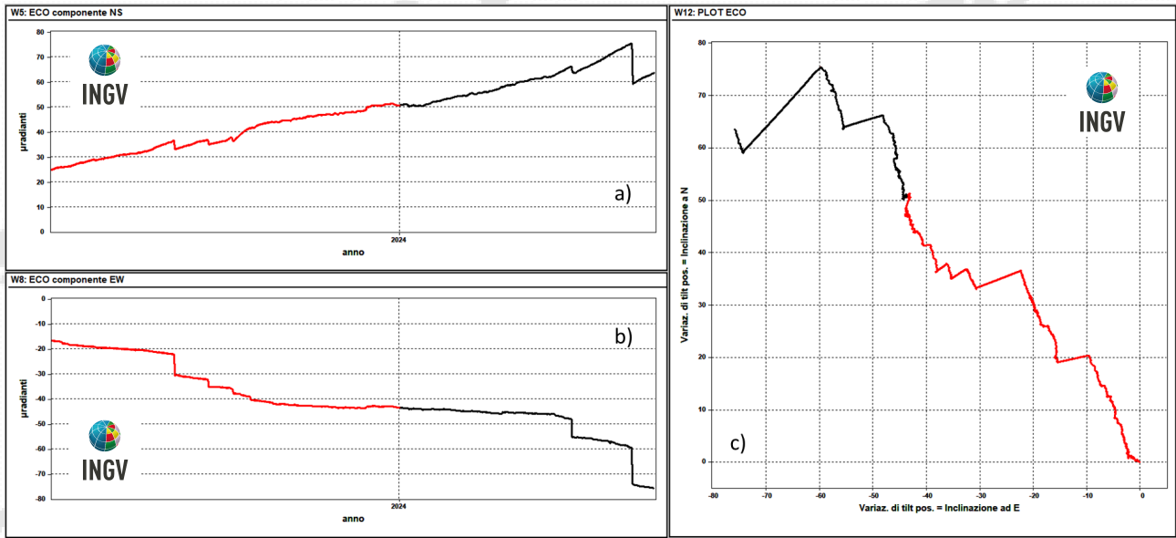
Figura 2.2.2 – Serie temporali e plot del tilt della stazione ECO della rete dei Campi Flegrei registrati negli ultimi 12 mesi (giugno 2023 - maggio 2024).
