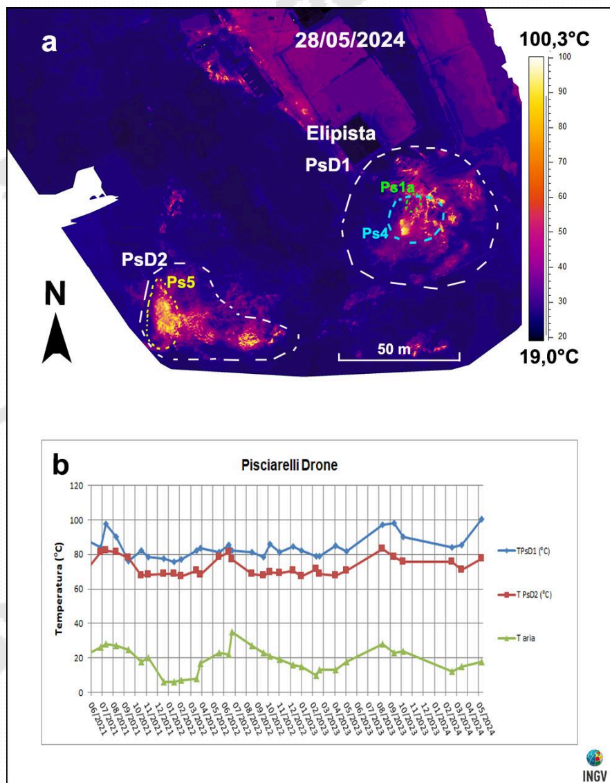
Figura 3.2.2 – Fotocomposizione di immagini termiche rilevate da drone nel mese di aprile 2023 (a) e valori massimi di temperatura (T) delle aree a maggiore anomalia termica (PsD1 e PsD2) confrontati con la temperatura dell'aria (Taria) misurata nel momento del rilievo termico da giugno 2021 a maggio 2024 (b).
