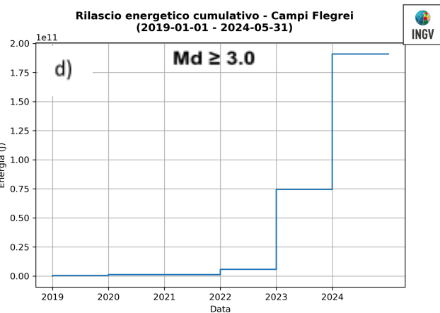
Figura 1.10 - Localizzazioni e andamento dei principali parametri sismologici dei terremoti con Md \geq 3.0 a partire dal 2019: a) frequenza di accadimento; b) profondità ipocentrali; c) magnitudo; d) energia cumulativa.
