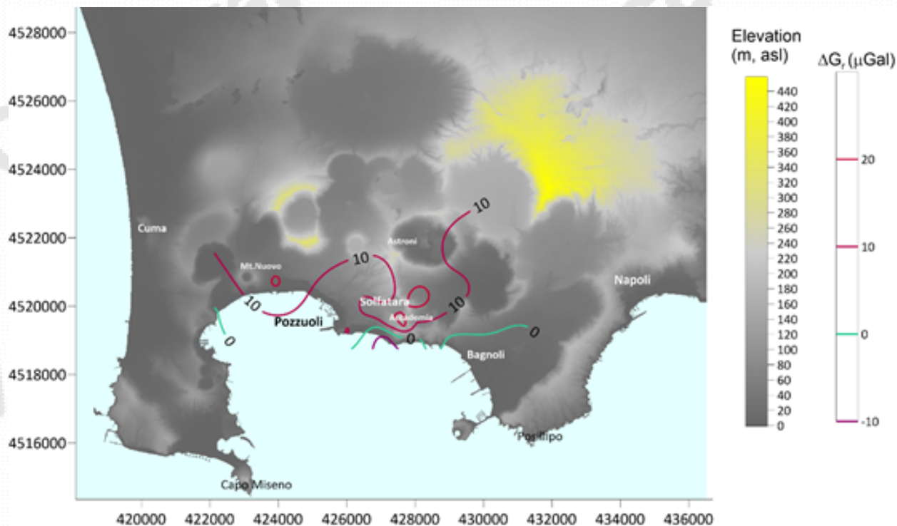
Figura 2.4.2. Mappa dei residui \Delta g_r ottenuti dopo aver eliminato l'effetto di variazione di g dovuto al sollevamento della caldera misurato tra maggio e febbraio 2024, considerando un FAG = -289 \text{ mGal/m} (Berrino et al., 1992); equidistanza 10 \mu\text{Gal} . L'errore totale sulla rete per la campagna di maggio 2024 è pari a \pm 6 \mu\text{Gal}
