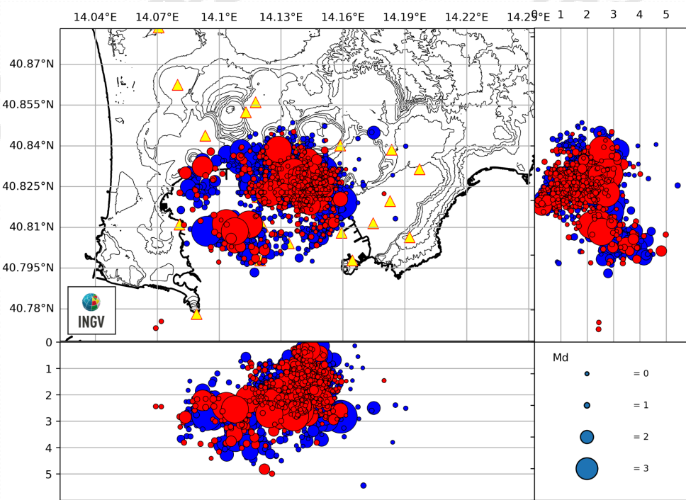
Figura 1.4 - Localizzazioni ipocentrali ai Campi Flegrei nel corso degli ultimi 12 mesi (in blu) e dell'ultimo mese (in rosso). La dimensione dei simboli è proporzionale alla magnitudo, come indicato nel riquadro in basso a destra.
