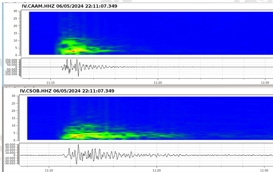
Figura 1.2 - Spettrogramma dell'evento del 06/05/2024 alle 22:11 UTC alle stazioni CAAM e CSOB
