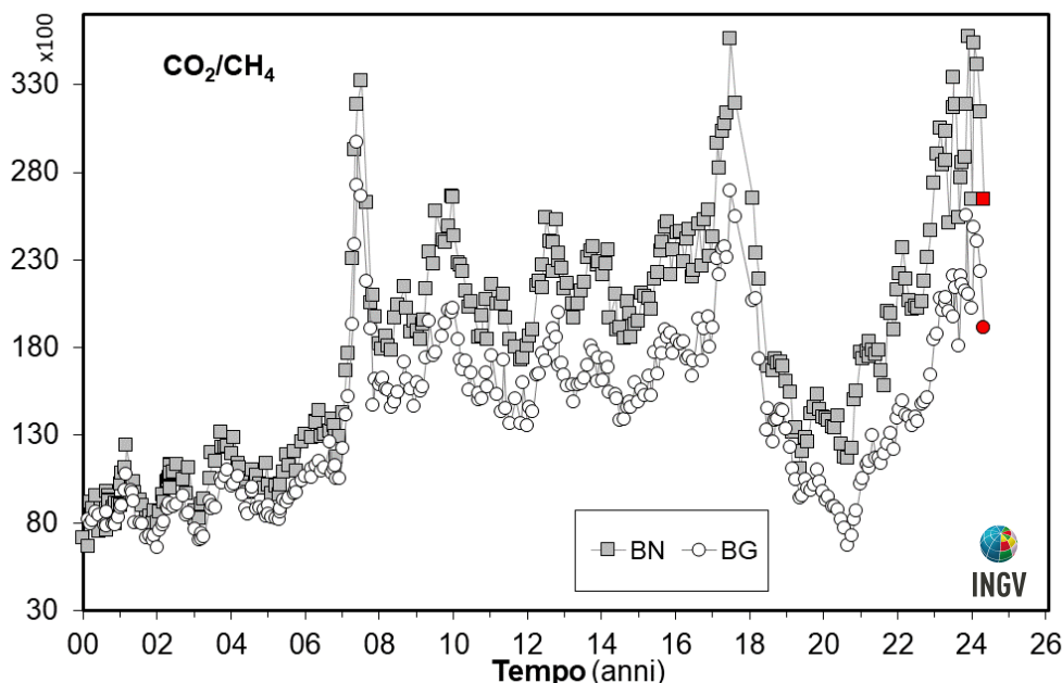
Figura 4.5 – Variazioni del rapporto CO_2/CH_4 per le fumarole BG e BN a partire dal 2000. I picchi nel rapporto, registrati in superficie con circa un anno di ritardo, evidenziano episodi di degassamento magmatico avvenuti ai Campi Flegrei (Chiodini et al., 2012). Con il simbolo rosso sono evidenziati i campioni di maggio 2024.
