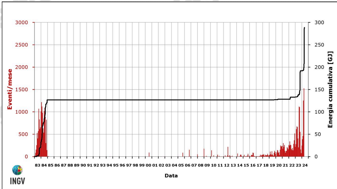
Figura 1.11 – Frequenza di accadimento dei terremoti registrati ai Campi Flegrei dal 1983. La linea nera rappresenta l'energia cumulativa.
