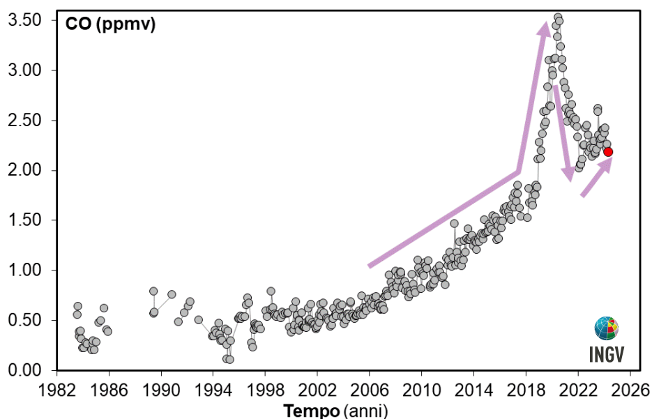
Figura 4.3 – Variazioni della concentrazione di monossido di carbonio (CO) misurato alla fumarola BG a partire dal 1983. Con il simbolo rosso è evidenziato il campione di maggio 2024. In generale alti contenuti di CO caratterizzano sistemi vulcanici a elevata temperatura, mentre fumarole alimentate da sistemi idrotermali mostrano concentrazioni più basse, in tali sistemi un aumento delle concentrazioni di CO può riflettere un incremento delle condizioni di pressione e temperatura.
