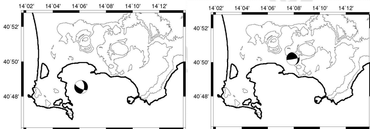
Figura 1.8a - Localizzazione e meccanismo focale dell'evento del 10/05/2024 alle 11:25 UTC Md 3.6 ( \pm 0.3 ) (a sinistra) e del 20/05/2024 alle 17:51 UTC Md 3.5 ( \pm 0.3 ) (a destra)
