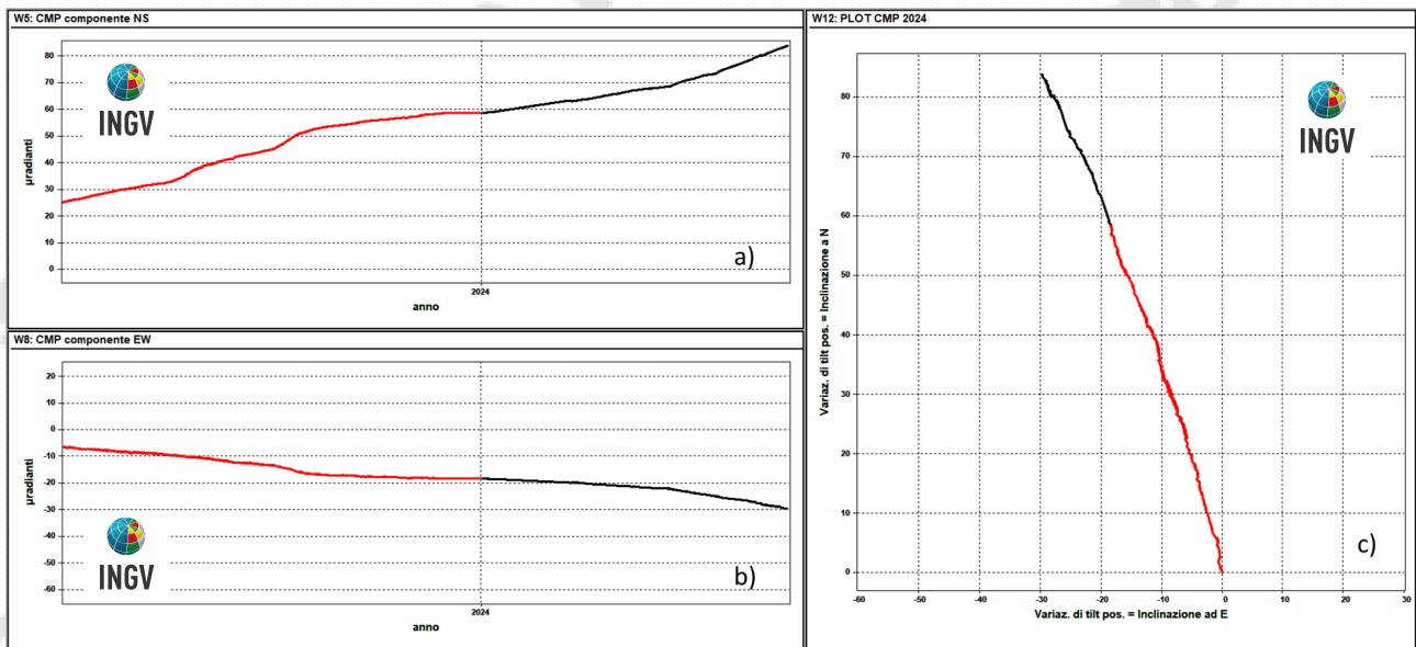
Figura 2.2.3 – Serie temporali e plot del tilt della stazione CMP della rete dei Campi Flegrei registrati negli ultimi 12 mesi (giugno 2023 - maggio 2024).
