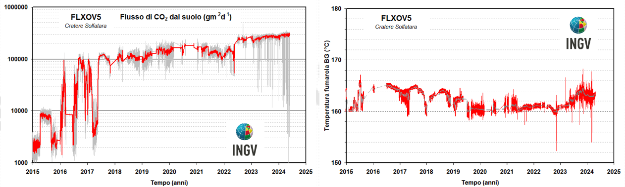
Figura 4.11 – Valori del flusso di CO 2 dal suolo e della temperatura della fumarola BG misurati dalla stazione FLXOV5 installata nel cratere della Solfatara, a pochi metri dalla fumarola principale BG. I valori di flusso di CO 2 dal suolo mostrano, in generale, un significativo incremento a partire dal 2016 (la linea rossa si riferisce alle medie giornaliere).
