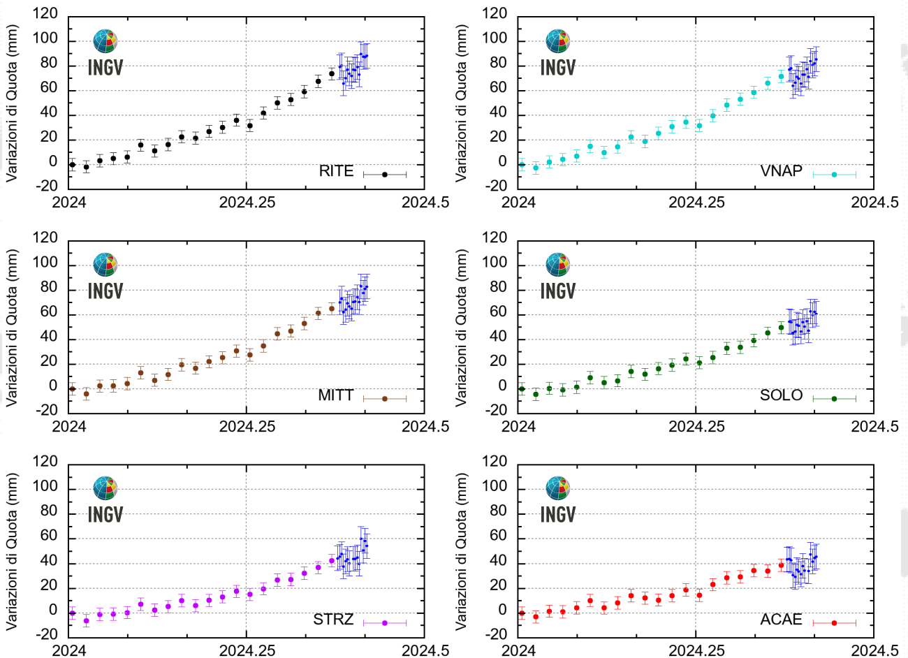
Figura 2.1.3 - Serie temporali delle variazioni in quota delle stazioni di RITE (Pozzuoli - Rione Terra), VNAP (Pozzuoli - Via Napoli), MITT (Pozzuoli - Porto), SOLO (Solfatara), STRZ (Pozzuoli - Cimitero) e ACAE (Accademia Aeronautica) dal 01/01/2024 al 02/06/2024. Elaborazione dati in modalità Precise Point Positioning con software PRIDE PPP-AR.
