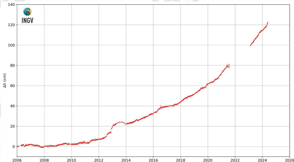
Figura 2.3.3 - Movimenti verticali del suolo nel periodo gennaio 2006 – maggio 2024, ottenuti dall'analisi dei dati acquisiti dalla stazione mareografica di Pozzuoli Porto (POPT) (area centrale della caldera Flegrea). Le variazioni, riportate in cm, rappresentano le medie giornaliere e sono riferite alla stazione mareografica di Napoli, molo San Vincenzo (NAMM).
