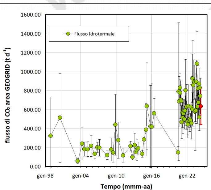
Figura 5.1.2 - Cronogramma dell'output di CO 2 diffuso dal suolo stimato per l'area di interesse. Le misure eseguite ad agosto 2020 hanno mostrato un valore tra i più bassi misurati, mentre quelle successive mostrano un aumento dei valori, con ~650 tonnellate di CO 2 al giorno per le misure di maggio 2024 (simbolo rosso). Le barre verticali rappresentano l'intervallo di confidenza del 95%.
