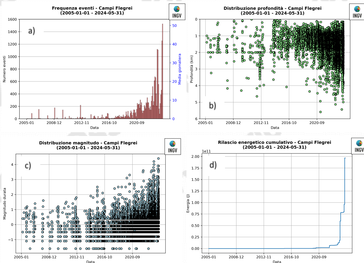
Figura 1.9 - Andamento dei principali parametri sismologici a partire dal 2005: a) frequenza di accadimento; b) profondità ipocentrali; c) magnitudo; d) energia cumulativa.
