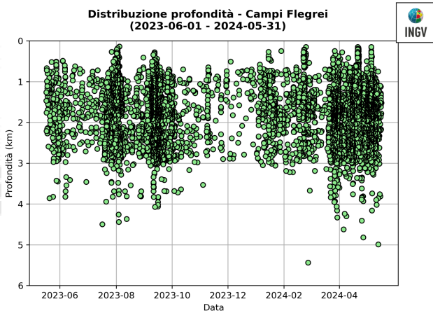
Figura 1.5 - Profondità ipocentrali degli eventi registrati ai Campi Flegrei nel corso degli ultimi 12 mesi (a sinistra) e dell'ultimo mese (a destra).
