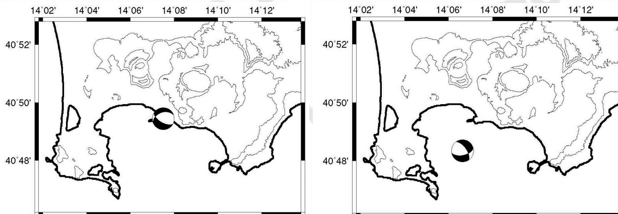
Figura 1.8c - Localizzazione e meccanismo focale dell'evento del 20/05/2024 alle 21:00 UTC Md 3.6 ( \pm 0.3 ) (a sinistra) e del 22/05/2024 alle 06:28 UTC Md 3.6 ( \pm 0.3 ) (a destra)
