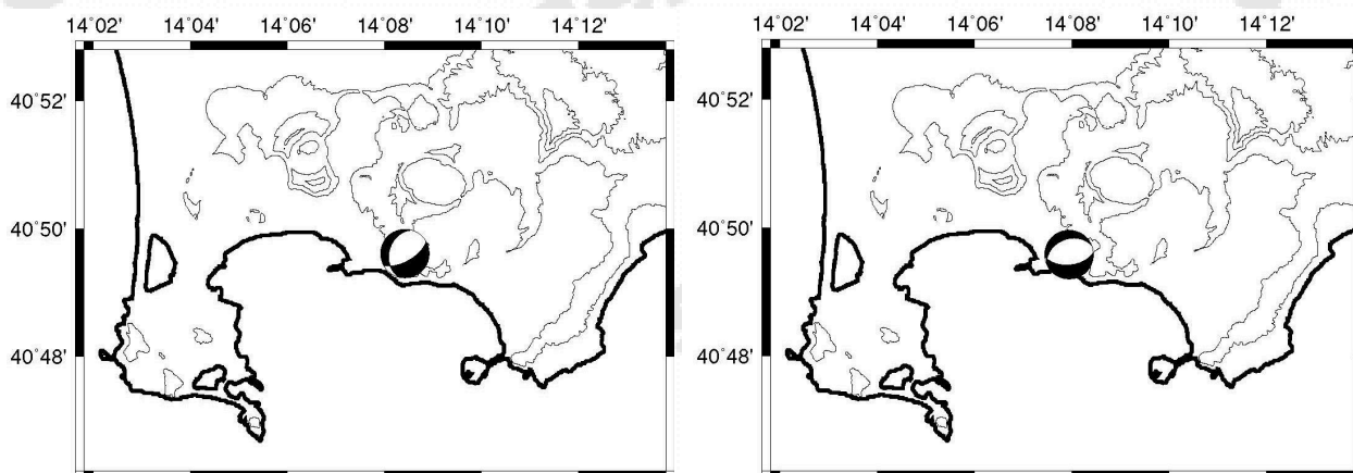
Figura 1.8b - Localizzazione e meccanismo focale dell'evento del 20/05/2024 alle 18:10 UTC Md 4.4 ( \pm 0.3 ) (a sinistra) e del 20/05/2024 alle 19:46 UTC Md 3.9 ( \pm 0.3 ) (a destra)
