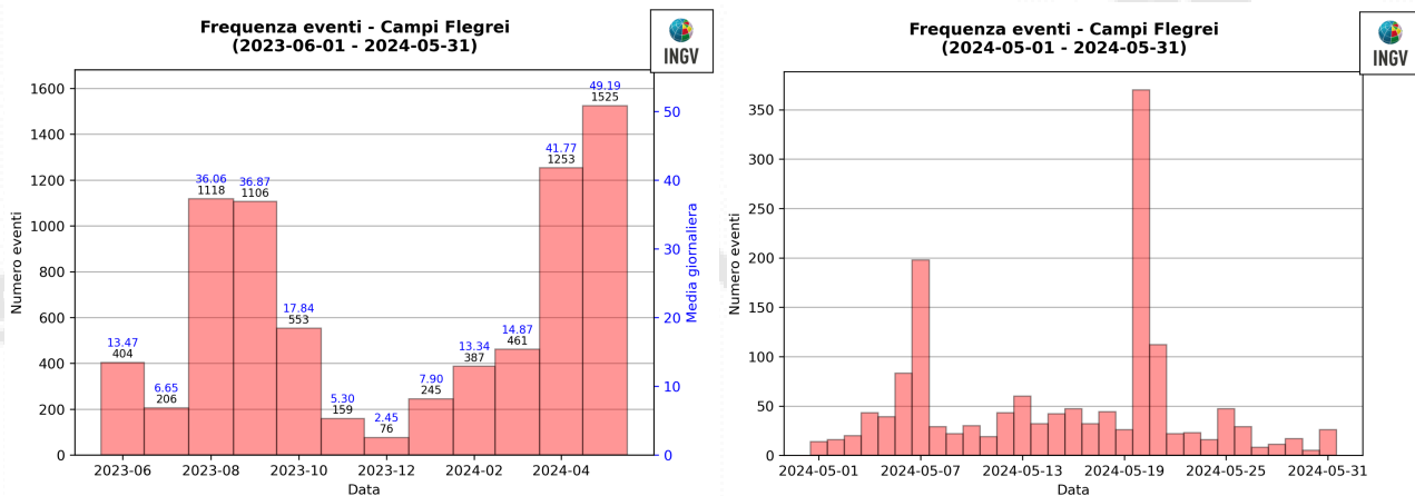
Figura 1.3 - A sinistra numero di eventi registrati ai Campi Flegrei nel corso degli ultimi 12 mesi (in totale 7493), mentre a destra quelli avvenuti nell'ultimo mese (in totale 1525).
