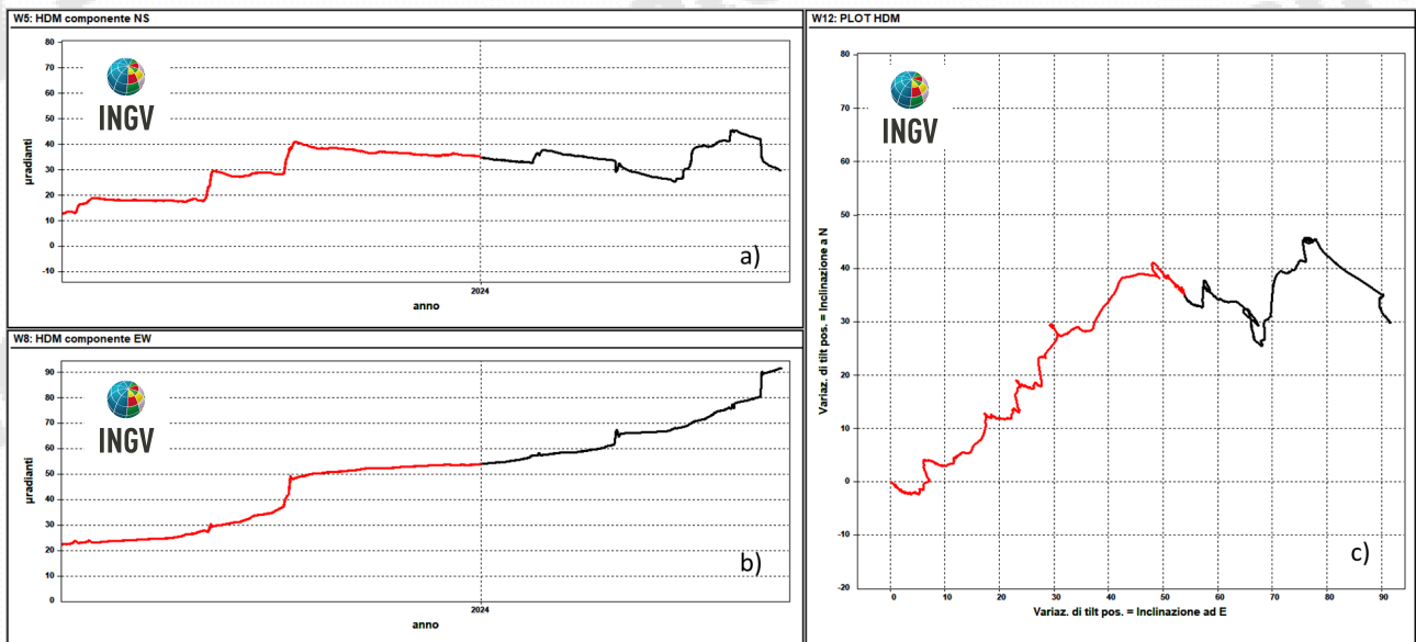
Figura 2.2.3 – Serie temporali e plot del tilt della stazione HDM della rete dei Campi Flegrei registrati negli ultimi 12 mesi (giugno 2023 - maggio 2024).
