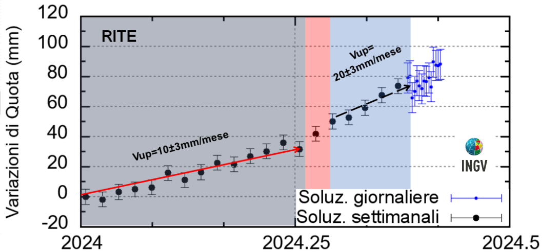
Figura 2.1.2 - Serie temporale delle variazioni in quota della stazione GNSS di RITE dal 01/01/2024 al 02/06/2024. Elaborazione dati in modalità Precise Point Positioning con software PRIDE PPP-AR.
