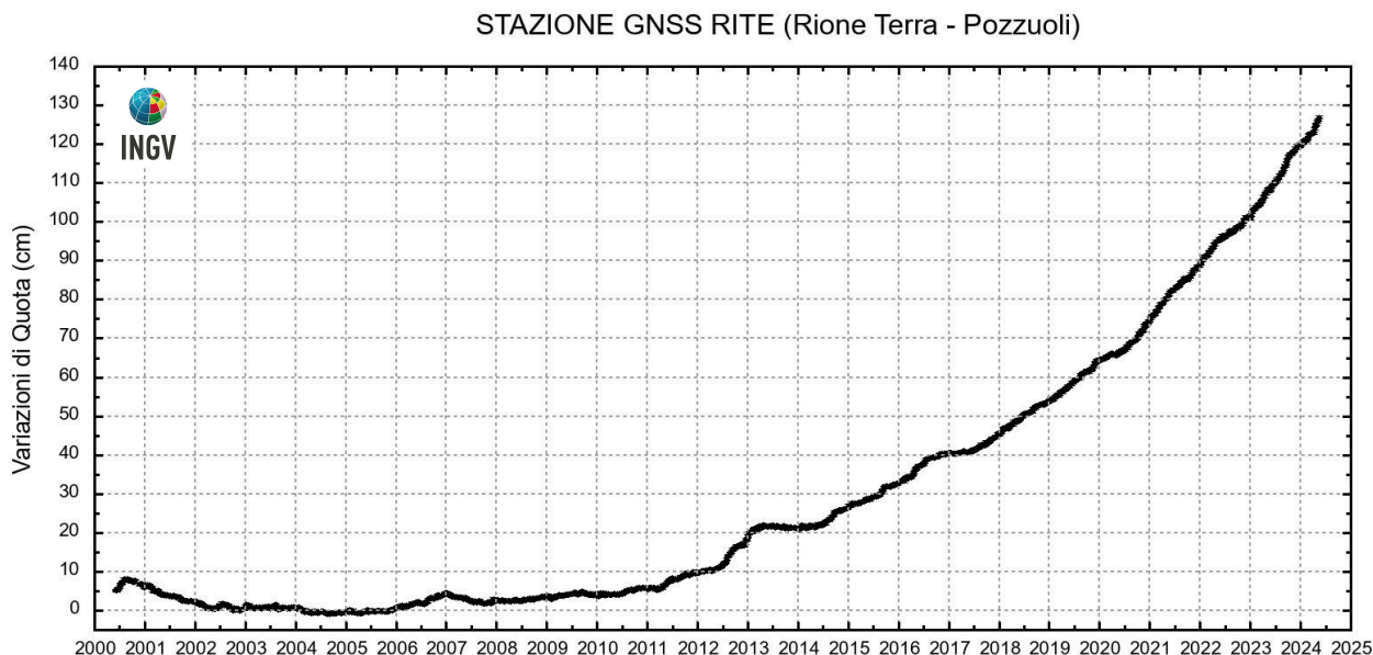
Figura 2.1.4 - Serie temporale delle variazioni settimanali in quota della stazione di RITE (Pozzuoli – Rione Terra) dal 2000 a maggio 2024.
