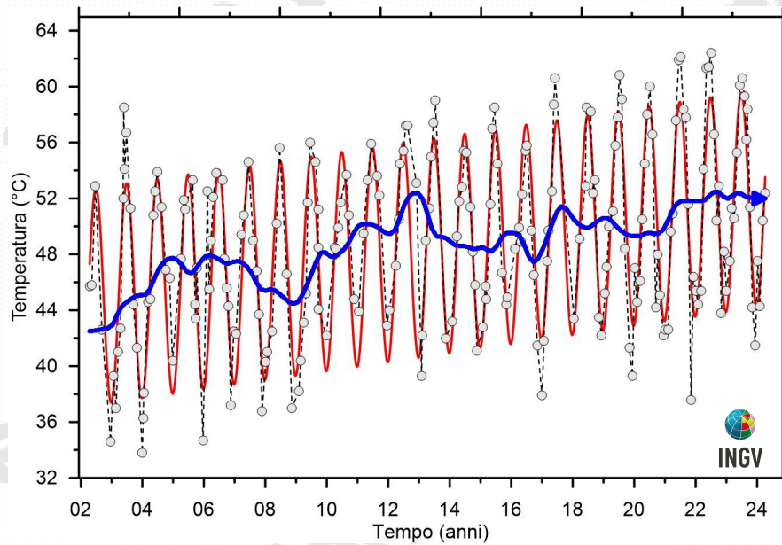
Figura 4.7 – Cronogramma della media delle temperature del suolo (a 10 cm di profondità) misurate su 61 punti fissi nell'area craterica della Solfatara. Va evidenziato l'aumento del valore medio nel periodo 2002-2024 di oltre 8 °C. Il trend depurato dalla componente stagionale mediante l'utilizzo dell'algoritmo di destagionalizzazione STL (Seasonal-Trend decomposition based on Loess, Cleveland et al., 1990), è riportato con la linea blu.
