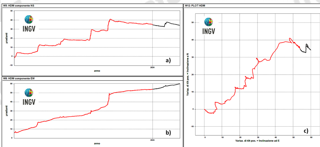
Figura 2.2.3 – Serie temporali e plot del tilt della stazione HDM della rete dei Campi Flegrei registrati negli ultimi 12 mesi (dal 1 marzo 2023 al 29 febbraio 2024).
