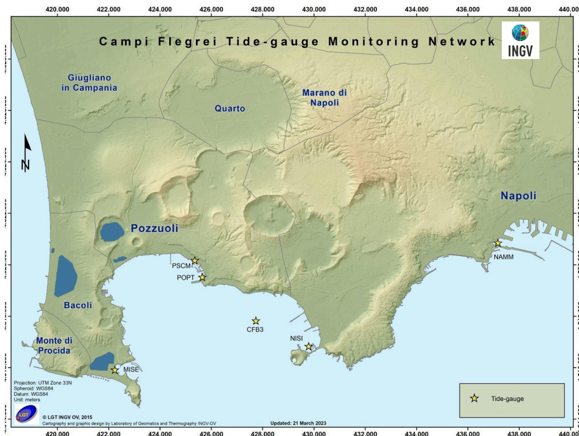
Figura 2.3.1 - Rete Mareografica dei Campi Flegrei.
