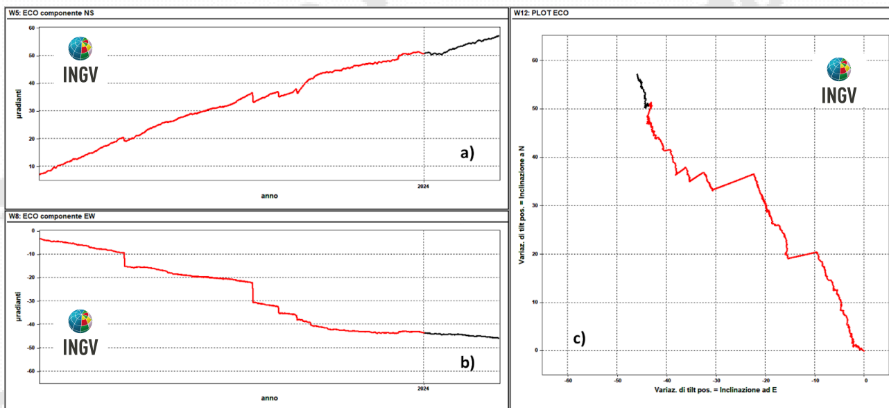
Figura 2.2.2 – Serie temporali e plot del tilt della stazione ECO della rete dei Campi Flegrei registrati negli ultimi 12 mesi (dal 1 marzo 2023 al 29 febbraio 2024).
