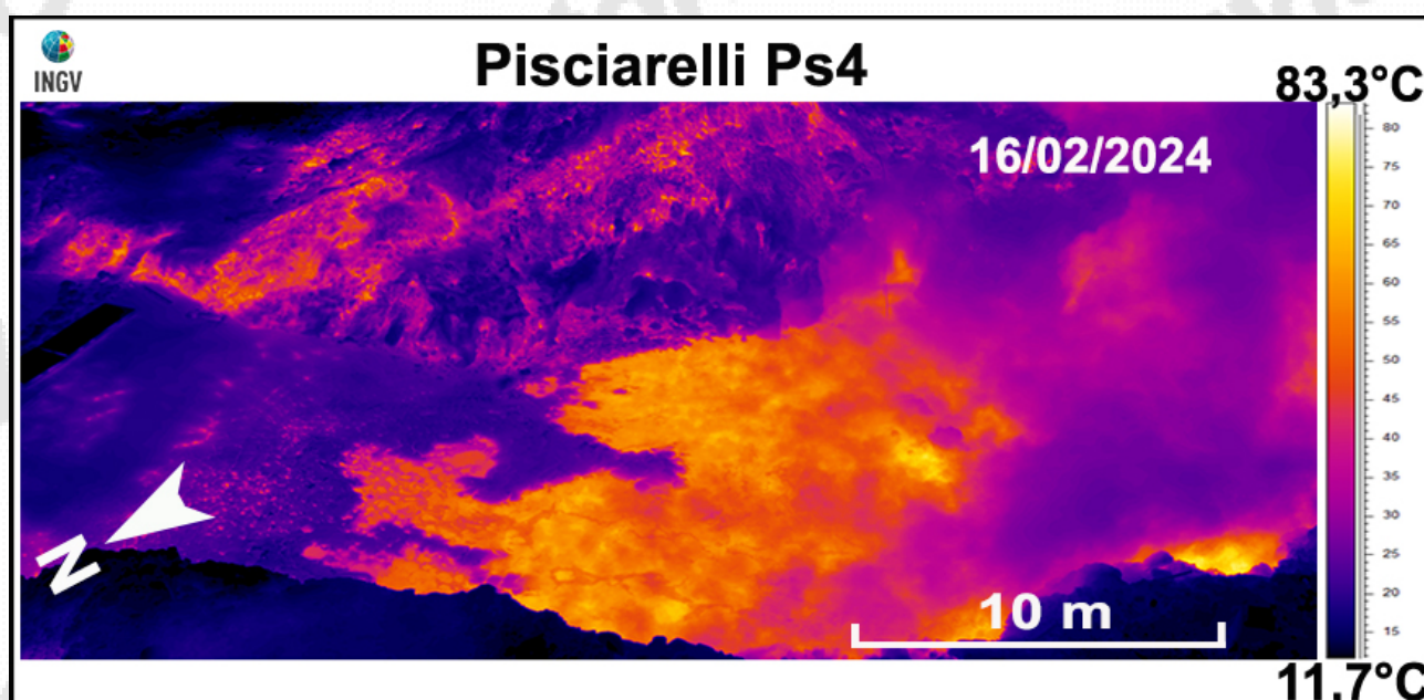
Figura 3.2.2 – Immagine termica, rilevata nel mese di febbraio 2024, dell'area denominata Ps4 (Fig.3.2.1b).
