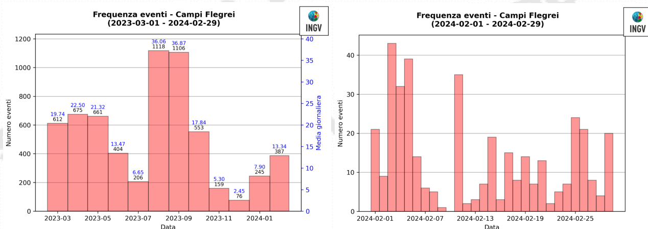
Figura 1.2 - A sinistra numero di eventi registrati ai Campi Flegrei nel corso degli ultimi 12 mesi (in totale 6202), mentre a destra quelli avvenuti nell'ultimo mese (in totale 387).
