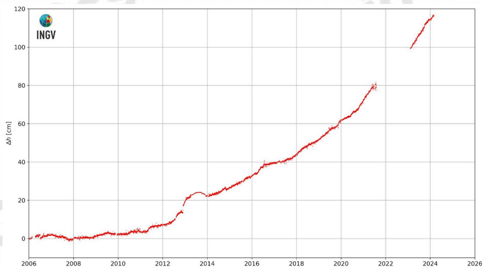
Figura 2.3.3 - Movimenti verticali del suolo nel periodo gennaio 2006 – febbraio 2024, ottenuti dall'analisi dei dati acquisiti dalla stazione mareografica di Pozzuoli Porto (POPT) (area centrale della caldera Flegrea). Le variazioni, riportate in cm, rappresentano le medie giornaliere e sono riferite alla stazione mareografica di Napoli, molo San Vincenzo (NAMM).
