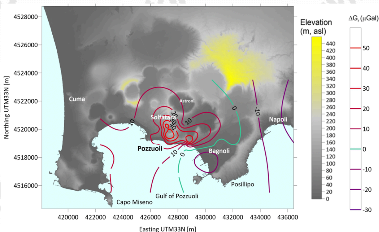
Figura 2.4.2 - Mappa dei residui ( \Delta g_r ) ottenuti dopo aver eliminato l'effetto di variazione di g dovuto al sollevamento della caldera misurato tra ottobre 2023 e febbraio 2024, considerando un FAG = -289 \mu\text{Gal/m} (Berrino et al., 1992); equidistanza 10 \mu\text{Gal} .
