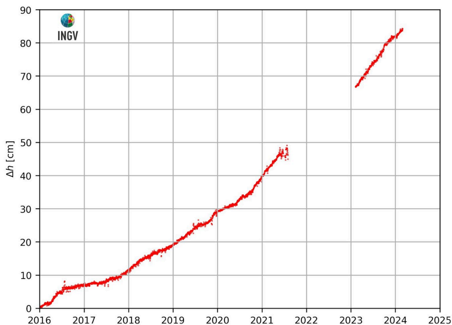
Figura 2.3.2 – Movimenti verticali del suolo, nel periodo gennaio 2016 – febbraio 2024, ottenuti dall'analisi dei dati acquisiti dalla stazione mareografica di Pozzuoli Porto (POPT), area centrale della caldera Flegrea. Le variazioni, riportate in cm, rappresentano le medie giornaliere e sono riferite alla stazione mareografica di Napoli, molo San Vincenzo (NAMM).
