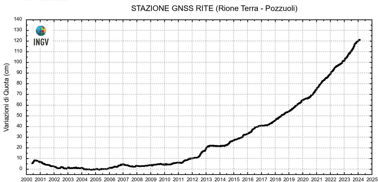
Figura 2.1.3 - Serie temporale delle variazioni settimanali in quota della stazione di RITE (Pozzuoli – Rione Terra) dal 2000 a febbraio 2024.
