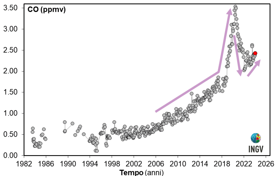
Figura 4.3 – Variazioni della concentrazione di monossido di carbonio (CO) misurato alla fumarola BG a partire dal 1983. Con il simbolo rosso è evidenziato il campione di febbraio 2024. In generale alti contenuti di CO caratterizzano sistemi vulcanici a elevata temperatura, mentre fumarole alimentate da sistemi idrotermali mostrano concentrazioni più basse, in tali sistemi un aumento delle concentrazioni di CO può riflettere un incremento delle condizioni di pressione e temperatura.
