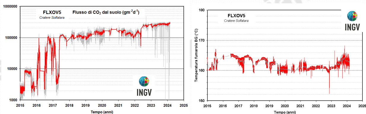
Figura 4.11 – Valori del flusso di \text{CO}_2 dal suolo e della temperatura della fumarola BG misurati dalla stazione FLXOV5 installata nel cratere della Solfatara, a pochi metri dalla fumarola principale BG. I valori di flusso di \text{CO}_2 dal suolo mostrano, in generale, un significativo incremento a partire dal 2016 (la linea rossa si riferisce alle medie giornaliere).
