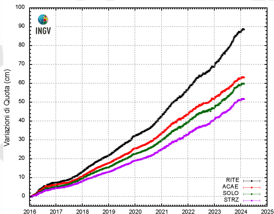
Figura 2.1.4 - Serie temporale delle variazioni settimanali in quota della stazione di RITE (Pozzuoli - Rione Terra), ACAE (Accademia Aeronautica), SOLO (Solfatara) e STRZ (Pozzuoli - Cimitero) da gennaio 2016 a febbraio 2024.
