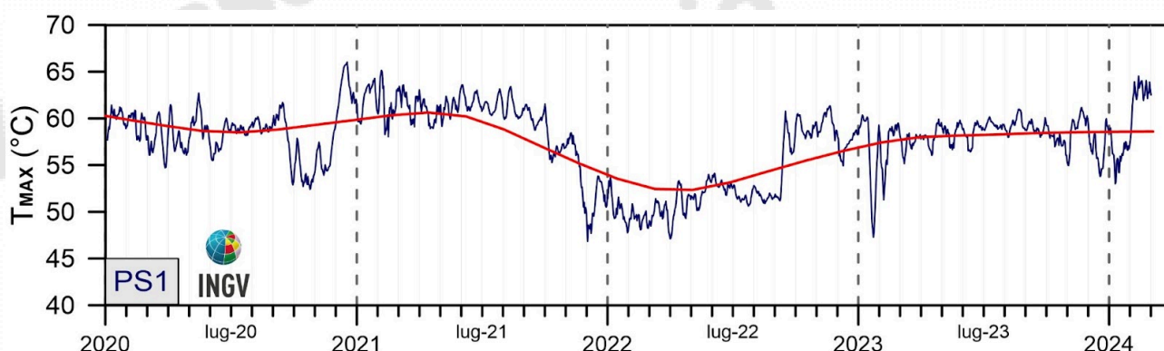
Figura 3.1.3 - Stazione PS1. Serie temporali dei valori di temperatura massima giornaliera rilevata nelle immagini IR destagionalizzate mediante applicazione dell'algoritmo STL [medie settimanali (blu); trend a lungo termine (rosso)].
