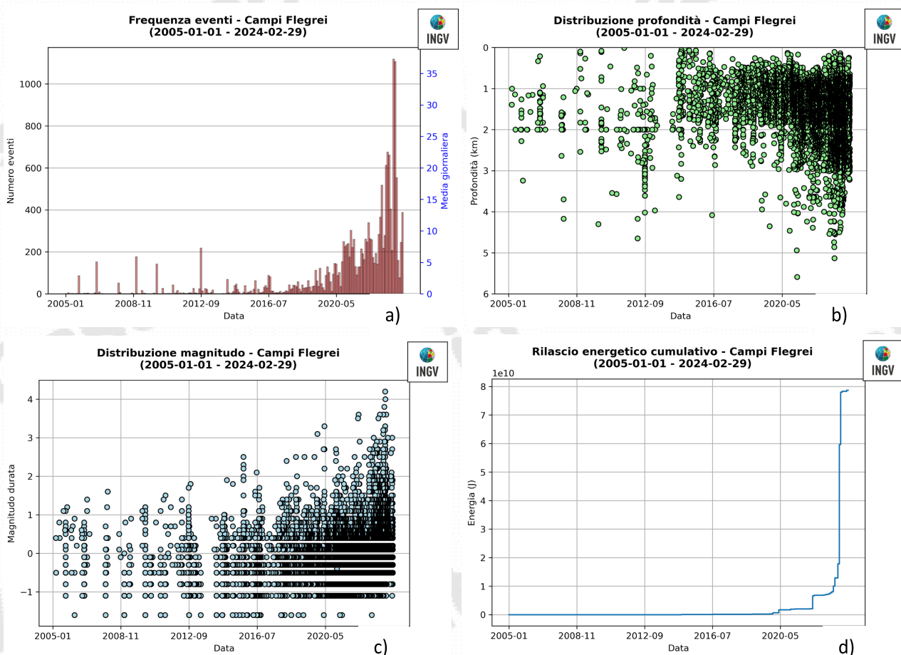
Figura 1.8 - Andamento dei principali parametri sismologici a partire dal 2005: a) frequenza di accadimento; b) profondità ipocentrali; c) magnitudo; d) energia cumulativa.
