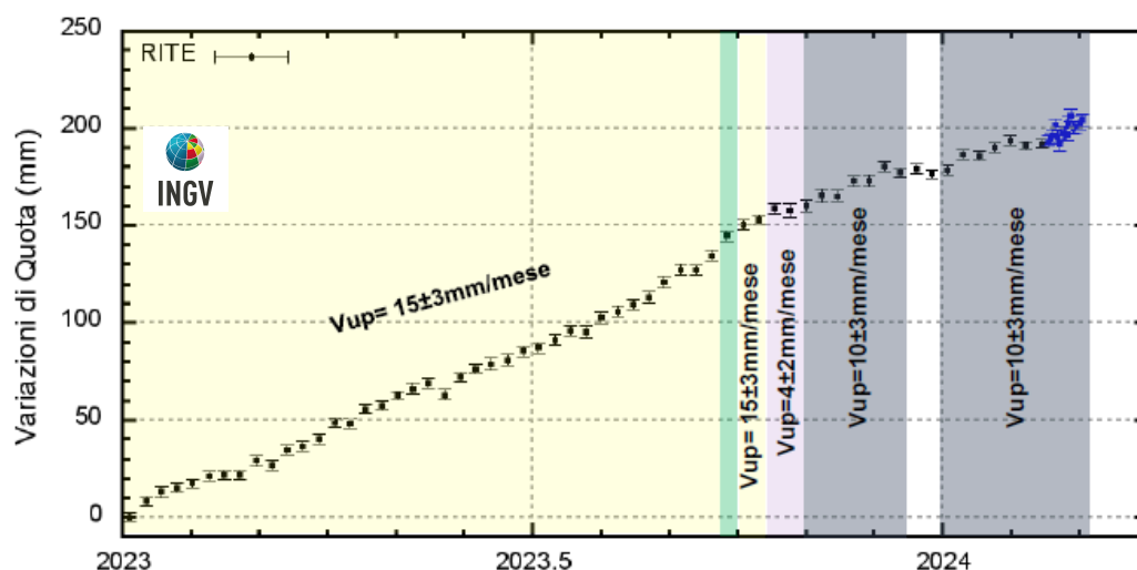
Figura 2.1.2 - Serie temporale delle variazioni in quota della stazione GNSS di RITE dal 01/01/2023 al 03/03/2024
