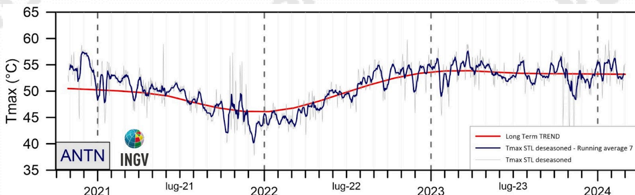
Figura 5.2.2 - Stazione ANTN. Serie temporale dei valori di temperatura massima giornaliera rilevata nelle immagini IR destagionalizzate mediante applicazione dell'algoritmo STL [medie settimanali (blu); trend a lungo termine (rosso)].
