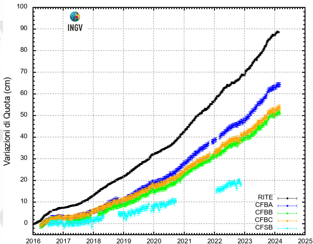
Figura 2.1.6 – Serie temporali delle variazioni settimanali in quota delle stazioni GNSS dell'infrastruttura marina sistema MEDUSA nell'intervallo aprile 2016-febbraio 2024, confrontate con quella della stazione RITE.
