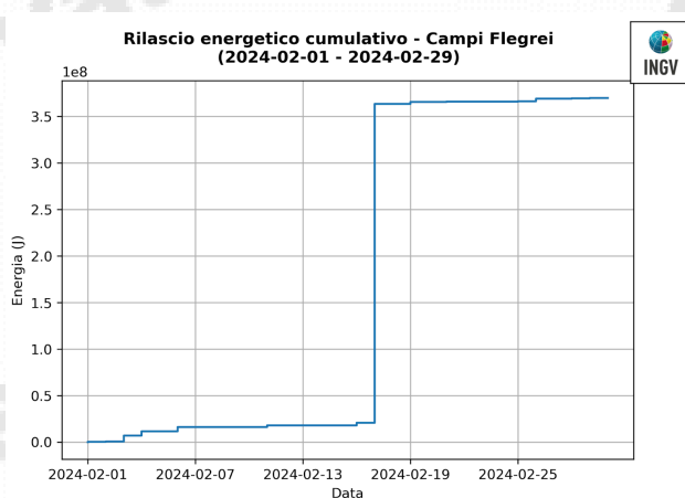
Figura 1.6 - Rilascio cumulativo di energia sismica ai Campi Flegrei nel corso degli ultimi 12 mesi (a sinistra) e dell'ultimo mese (a destra).
