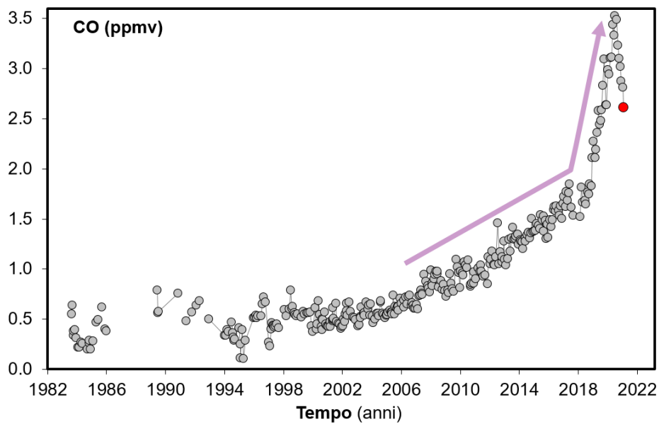
Figura 4.3 – Variazioni della concentrazione di monossido di carbonio (CO) misurato alla fumarola BG a partire dal 1983. Con il simbolo rosso è evidenziato il campione di febbraio 2021. In generale alti contenuti di CO caratterizzano sistemi vulcanici ad elevata temperatura mentre fumarole alimentate da sistemi idrotermali mostrano concentrazioni più basse, in tali sistemi un aumento delle concentrazioni di CO può riflettere un incremento delle condizioni di pressione e temperatura.
