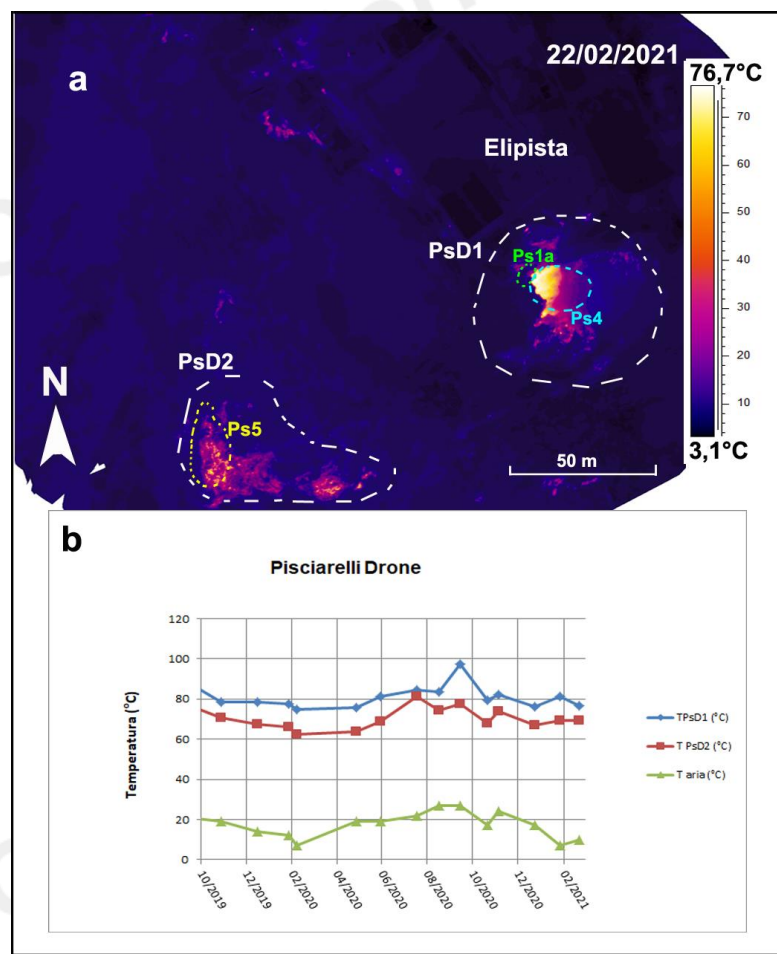
Figura 3.2.2 – Fotocomposizione di immagini termiche rilevate da drone nel mese di febbraio 2021 (a) e valori massimi di temperatura (T) delle aree a maggiore anomalia termica (PsD1 e PsD2) confrontati con la temperatura dell'aria misurata nel momento del rilievo termico da ottobre 2019 a febbraio 2021 (b).
