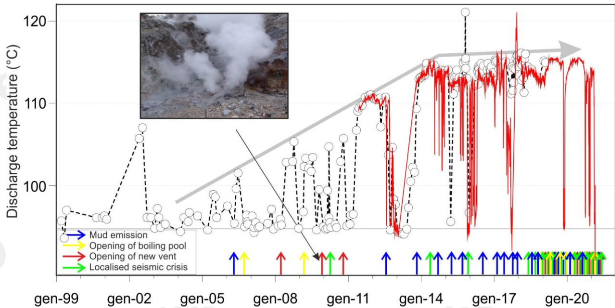
Figura 4.12 - Cronogramma delle temperature (°C) della fumarola di Pisciarelli e dei maggiori eventi occorsi legati all'aumento dell'attività idrotermale (i cerchi si riferiscono a misure discrete riferite al punto di maggior flusso dei gas, la linea rossa si riferisce alle medie giornaliere delle misure in continuo della stazione FLXOV8). La temperatura di ~95°C rappresenta la temperatura di ebollizione per i fluidi fumarolici di Pisciarelli. Nella foto è riportata la nuova vigorosa fumarola sorta il 20 dicembre 2009.
