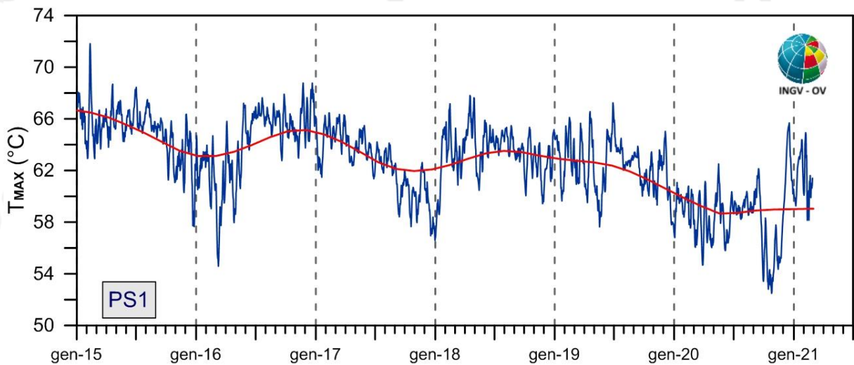
Figura 3.1.3 - Stazione PS1. Serie temporali dei valori di temperatura massima giornaliera rilevata nelle immagini IR destagionalizzate mediante applicazione dell' algoritmo STL [medie settimanali (blu); trend a lungo termine (rosso)].
