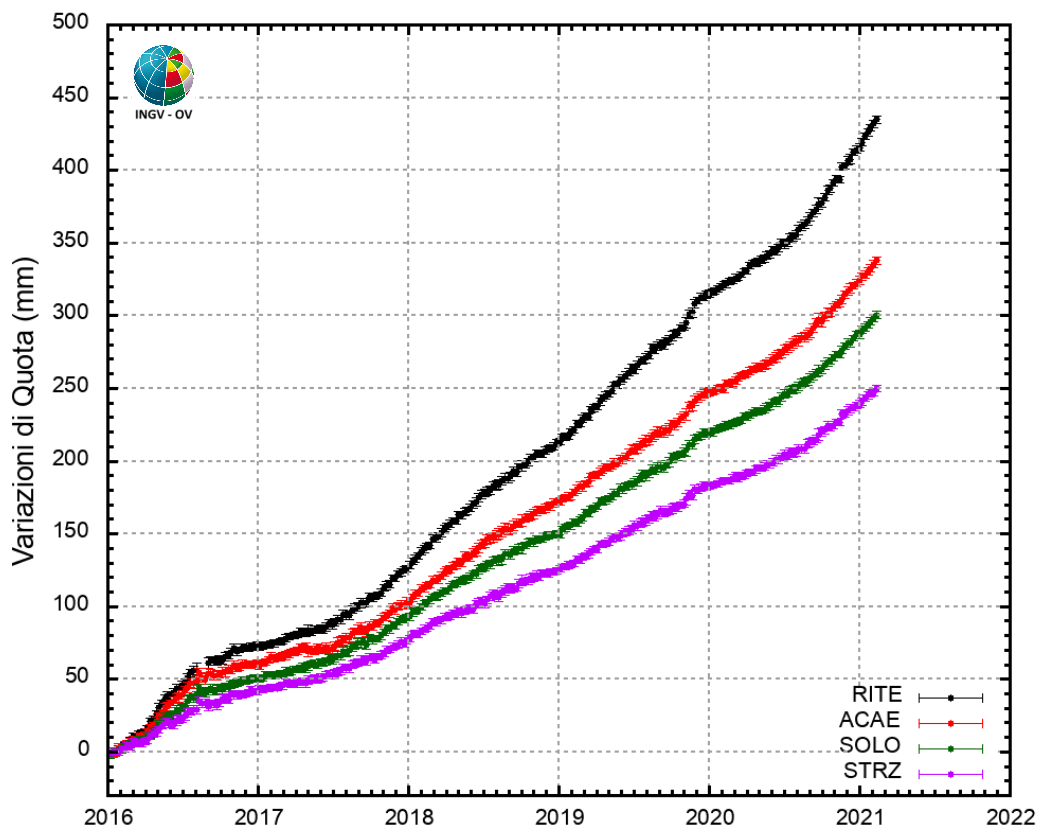
Figura 2.1.3 - Serie temporale delle variazioni in quota della stazione di RITE (Pozzuoli - Rione Terra), ACAE (Accademia Aeronautica), SOLO (Solfatara) e STRZ (Pozzuoli - Cimitero) da gennaio 2016 a febbraio 2021.
