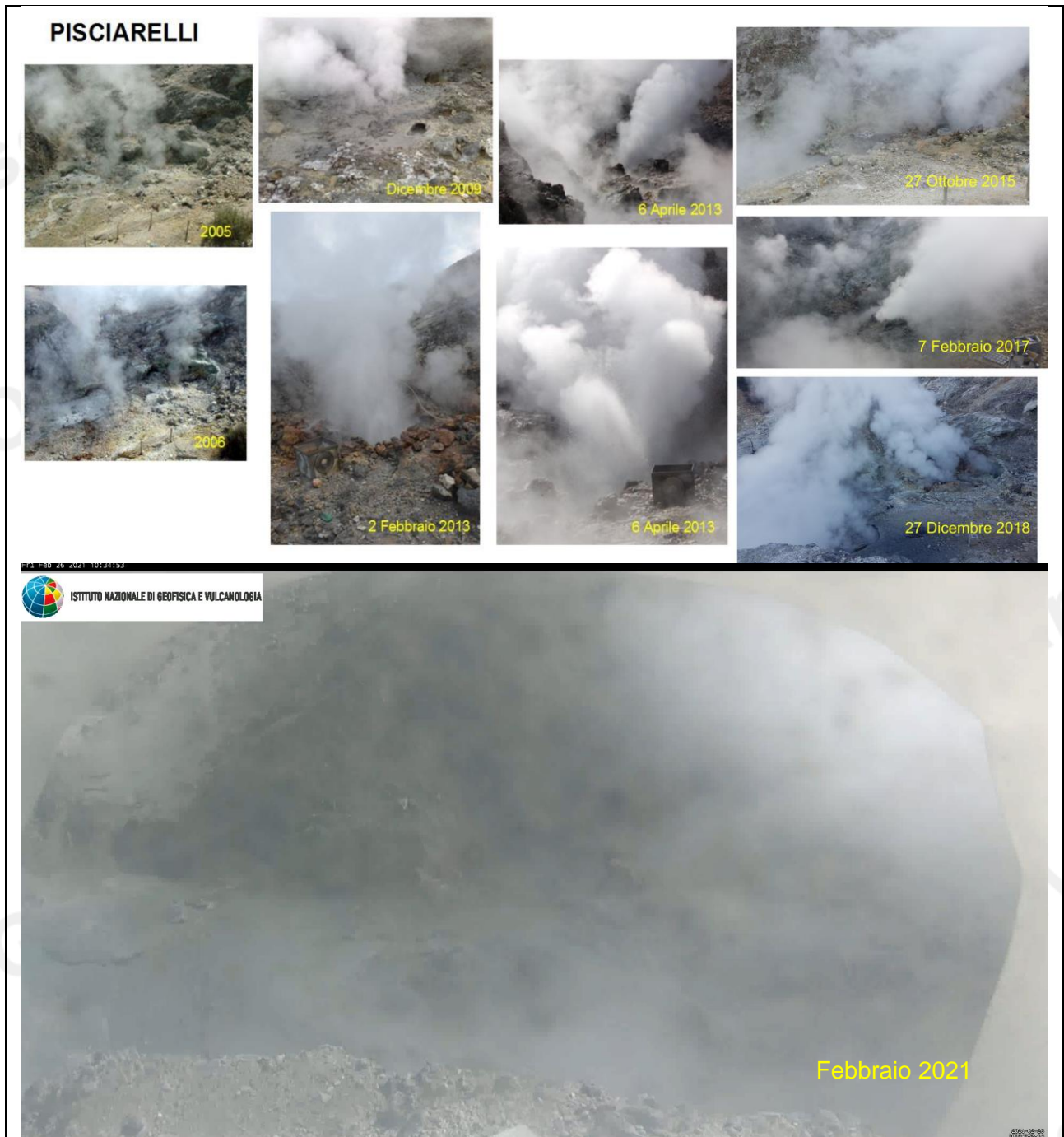
Figura 4.11 - Variazioni macroscopiche dell'area di emissione di Pisciarelli dal 2005.
