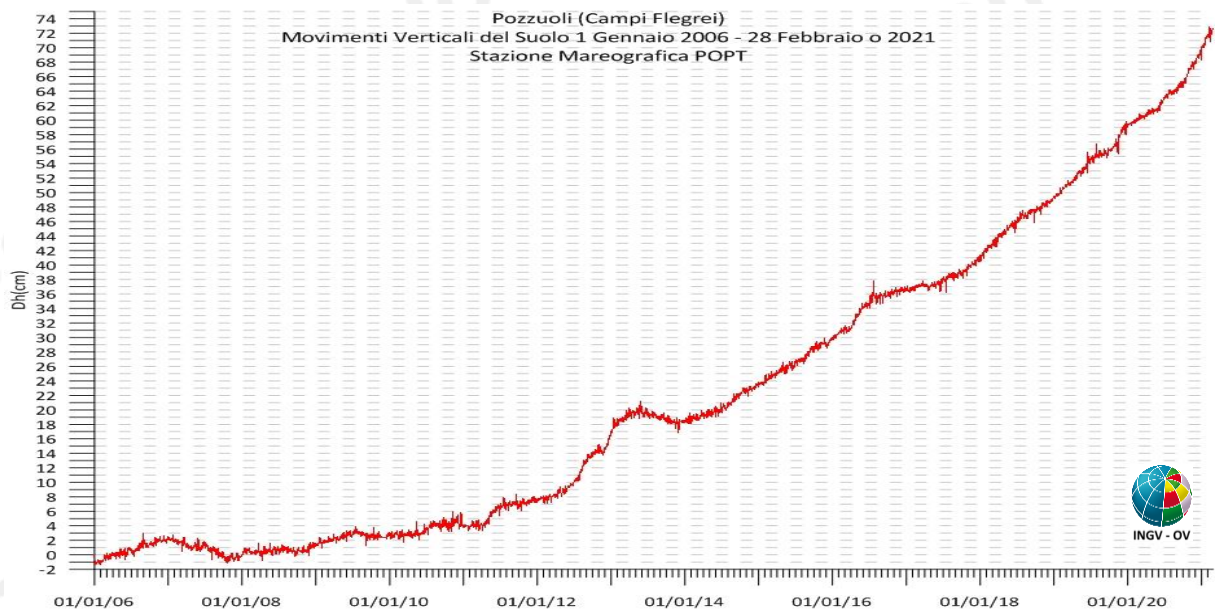
Figura 2.3.3 - Movimenti verticali del suolo, nel periodo gennaio 2006 – febbraio 2021, ottenuti dall'analisi dei dati acquisiti dal sensore digitale alla stazione mareografica di Pozzuoli Porto (POPT) (area centrale della caldera flegrea). Le variazioni riportate rappresentano le medie giornaliere e sono riferite alla stazione di Napoli molo S.Vincenzo (NAMM).
