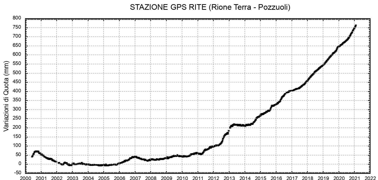
Figura 2.1.2 - Serie temporale delle variazioni settimanali in quota della stazione di RITE (Pozzuoli – Rione Terra) dal 2000 a febbraio 2021.
