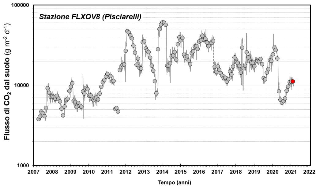
Figura 4.14 - Medie giornaliere (linea) e medie mensili (cerchi) dei flussi di \text{CO}_2 misurati dalla stazione automatica a Pisciarelli. E' da evidenziare il continuo trend d'aumento nel tempo a partire dal 2007 del flusso \text{CO}_2 . La media dei flussi relativa al mese di febbraio 2021 è riportata con il simbolo rosso. Il flusso di \text{CO}_2 dal suolo misurato dalla stazione dal mese di aprile 2020 ha mostrato una diminuzione dei valori. Tale condizione, già verificatasi in passato, potrebbe essere legata a variazioni locali del sito di emissione dove è installata la stazione.
