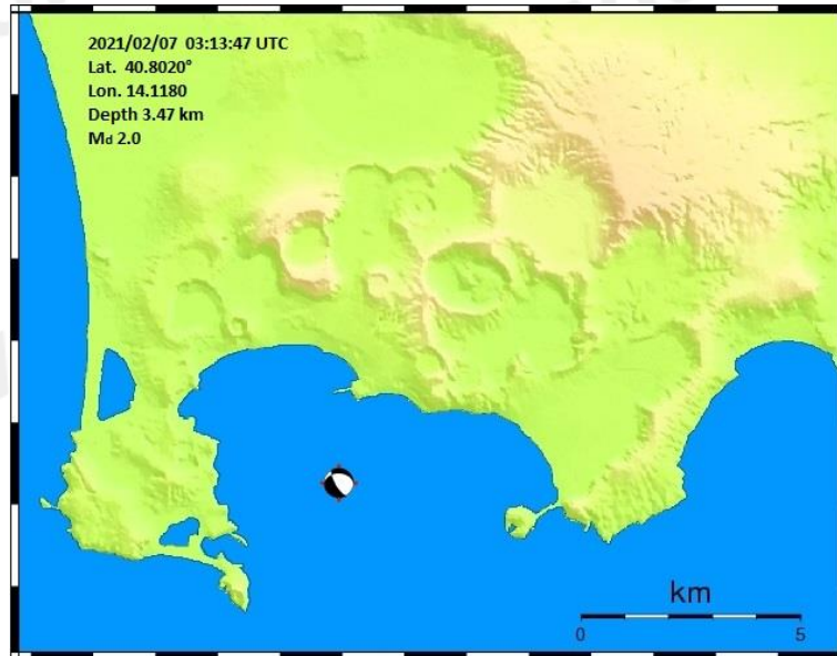
Figura 1.7 – Localizzazione e meccanismo focale dell'evento del 07/02/2021 alle 03:13 UTC.
