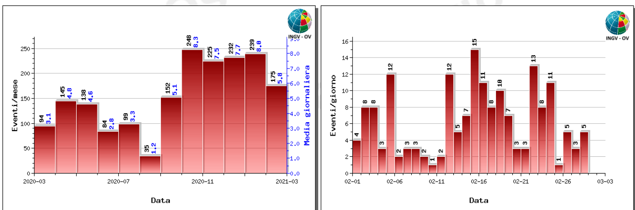
Figura 1.2 - A sinistra numero di eventi registrati ai Campi Flegrei nel corso degli ultimi 12 mesi (in totale 1866), mentre a destra quelli avvenuti nell'ultimo mese (in totale 175).
