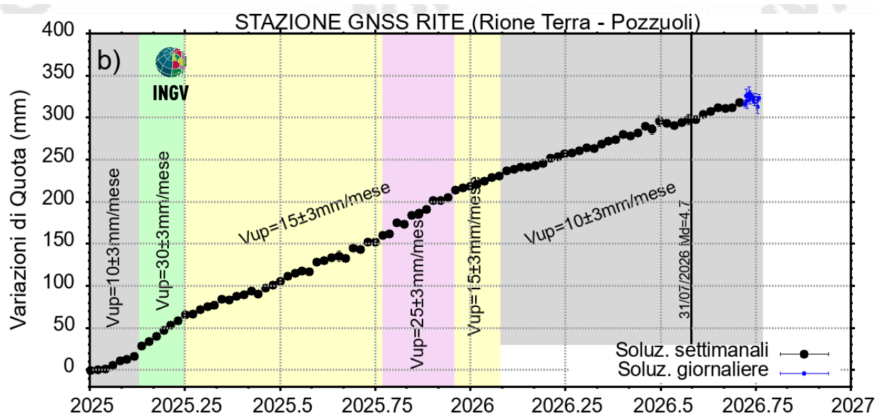
Figura 4.2 – Serie temporale delle variazioni in quota della stazione GNSS di RITE dal 01/01/2025 al 04/10/2026, con (a) e senza (b) la discontinuità cosismica del 31/07. Elaborazione dati in modalità differenziale singola baseline con software GNSS Spider.
