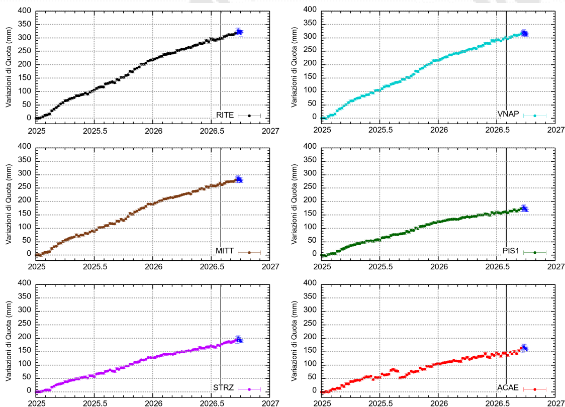
Figura 4.4 - Serie temporali delle variazioni in quota delle stazioni di RITE (Pozzuoli - Rione Terra), VNAP (Pozzuoli - Via Napoli), MITT (Pozzuoli - Porto), PIS1 (Pisciarelli), STRZ (Pozzuoli - Cimitero) e ACAE (Accademia Aeronautica) dal 01/01/2025 al 04/10/2026, con le discontinuità cosimiche corrette. Elaborazione dati in modalità differenziale singola baseline con software GNSS Spider. La linea nera verticale indica la data del 31 luglio.
