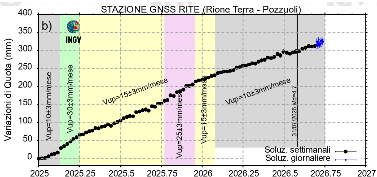
Figura 4.2 – Serie temporale delle variazioni in quota della stazione GNSS di RITE dal 01/01/2025 al 27/09/2026, con (a) e senza (b) la discontinuità cosismica del 31/07. Elaborazione dati in modalità differenziale singola baseline con software GNSS Spider.
