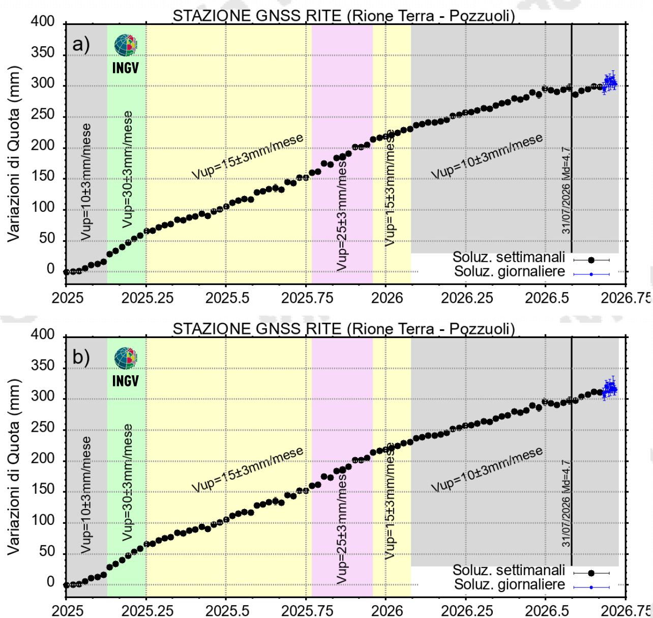
Figura 4.2 – Serie temporale delle variazioni in quota della stazione GNSS di RITE dal 01/01/2025 al 20/09/2026, con (a) e senza (b) la discontinuità cosismica del 31/07. Elaborazione dati in modalità differenziale singola baseline con software GNSS Spider.
