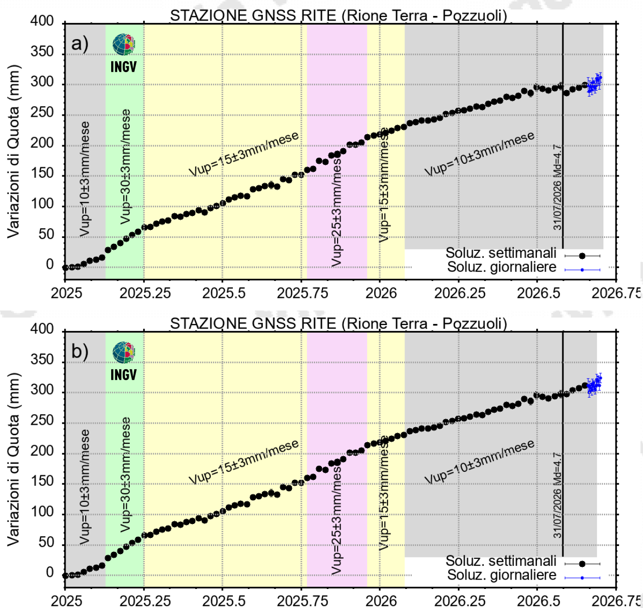
Figura 4.2 – Serie temporale delle variazioni in quota della stazione GNSS di RITE dal 01/01/2025 al 13/09/2026, con (a) e senza (b) la discontinuità cosismica del 31/07. Elaborazione dati in modalità differenziale singola baseline con software GNSS Spider.
