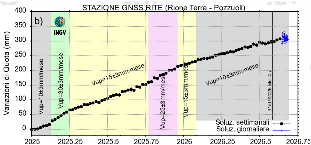
Figura 4.2 – Serie temporale delle variazioni in quota della stazione GNSS di RITE dal 01/01/2025 al 07/09/2026, con (a) e senza (b) la discontinuità cosismica del 31/07. Elaborazione dati in modalità differenziale singola baseline con software GNSS Spider.
