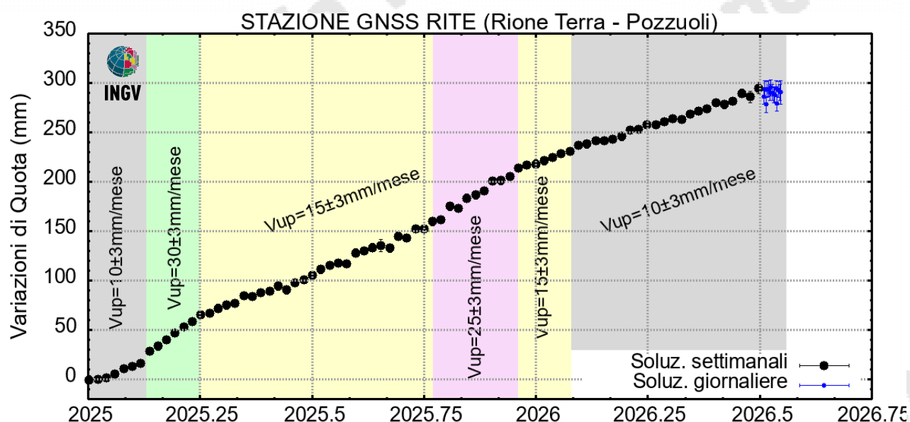
Figura 4.2 – Serie temporale delle variazioni in quota della stazione GNSS di RITE dal 01/01/2025 al 19/07/2026. Elaborazione dati in modalità differenziale singola baseline con software GNSS Spider.
