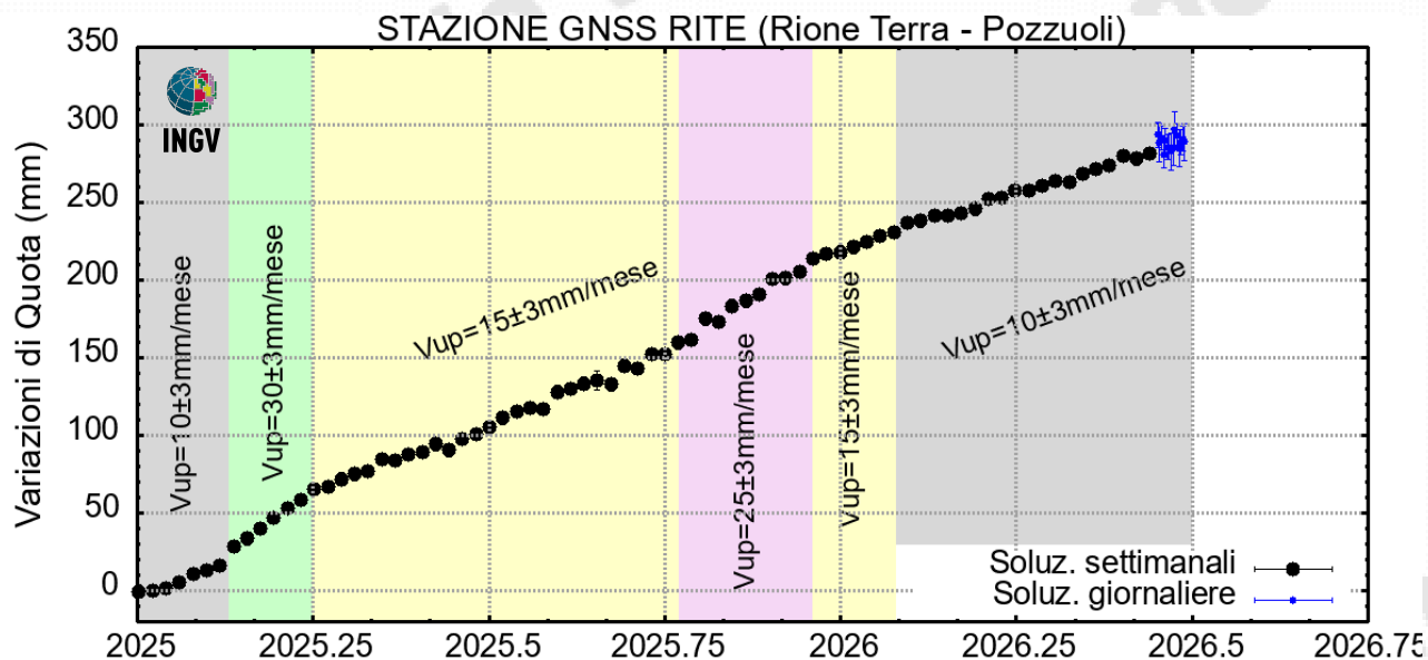
Figura 4.2 – Serie temporale delle variazioni in quota della stazione GNSS di RITE dal 01/01/2025 al 28/06/2026. Elaborazione dati in modalità differenziale singola baseline con software GNSS Spider.
