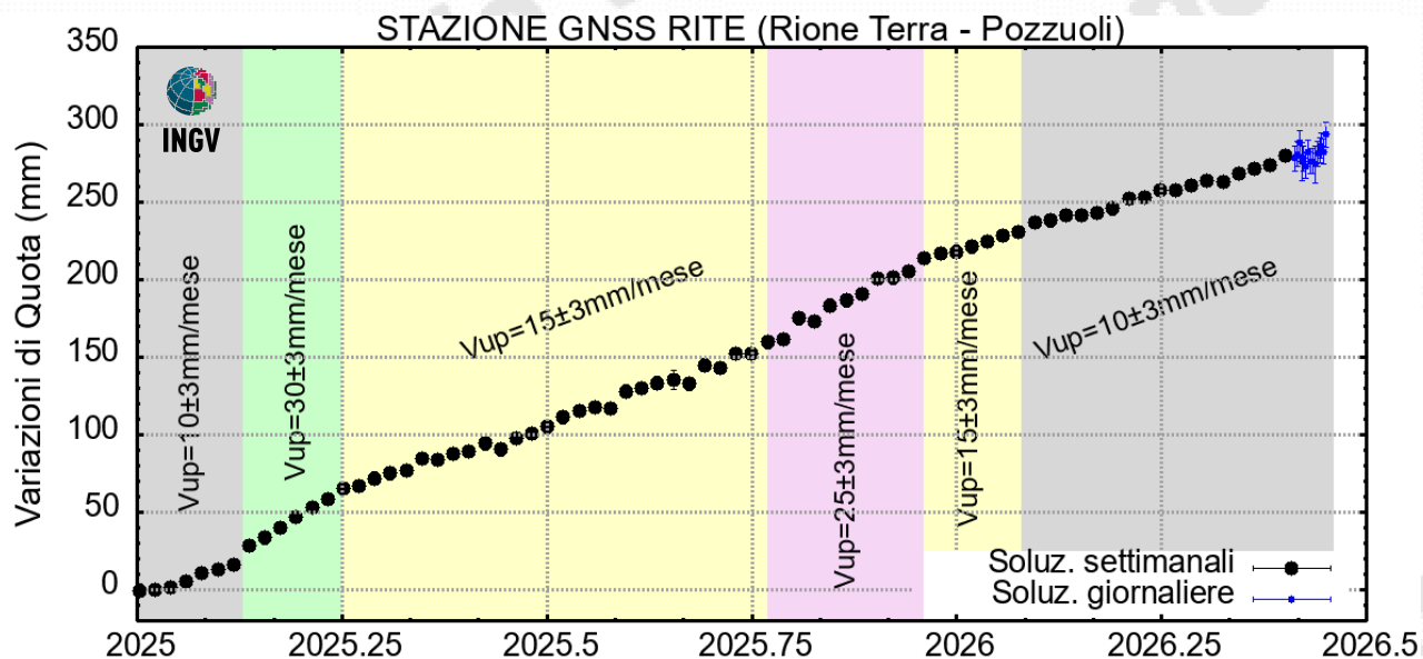
Figura 4.2 – Serie temporale delle variazioni in quota della stazione GNSS di RITE dal 01/01/2025 al 14/06/2026. Elaborazione dati in modalità differenziale singola baseline con software GNSS Spider.
