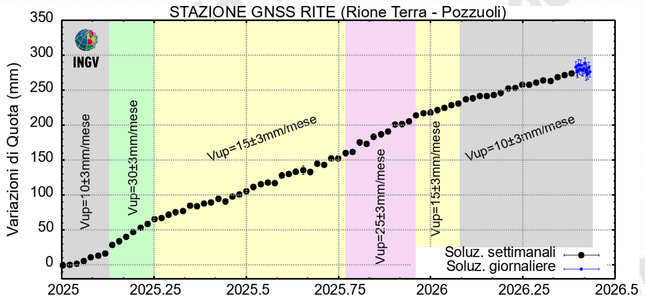
Figura 4.2 – Serie temporale delle variazioni in quota della stazione GNSS di RITE dal 01/01/2025 al 07/06/2026. Elaborazione dati in modalità differenziale singola baseline con software GNSS Spider.
