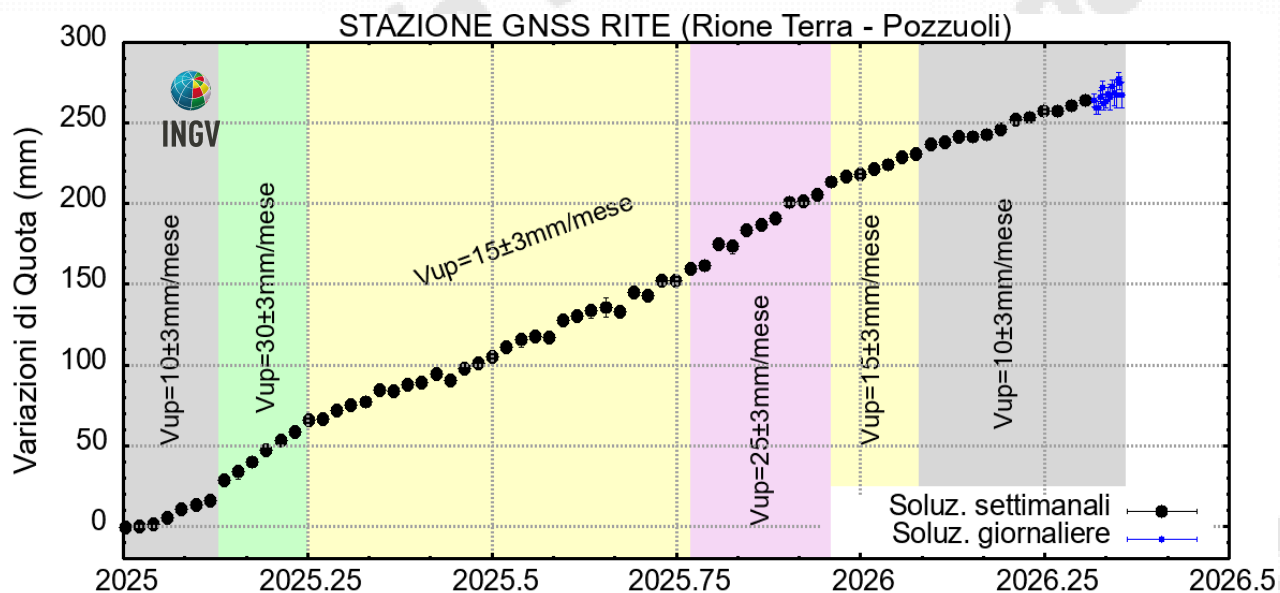
Figura 4.2 – Serie temporale delle variazioni in quota della stazione GNSS di RITE dal 01/01/2025 al 10/05/2026. Elaborazione dati in modalità differenziale singola baseline con software GNSS Spider.
