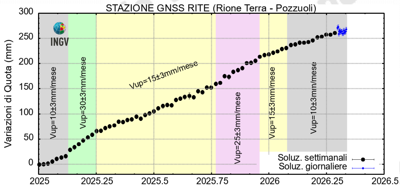
Figura 4.2 – Serie temporale delle variazioni in quota della stazione GNSS di RITE dal 01/01/2025 al 03/05/2026. Elaborazione dati in modalità differenziale singola baseline con software GNSS Spider.
