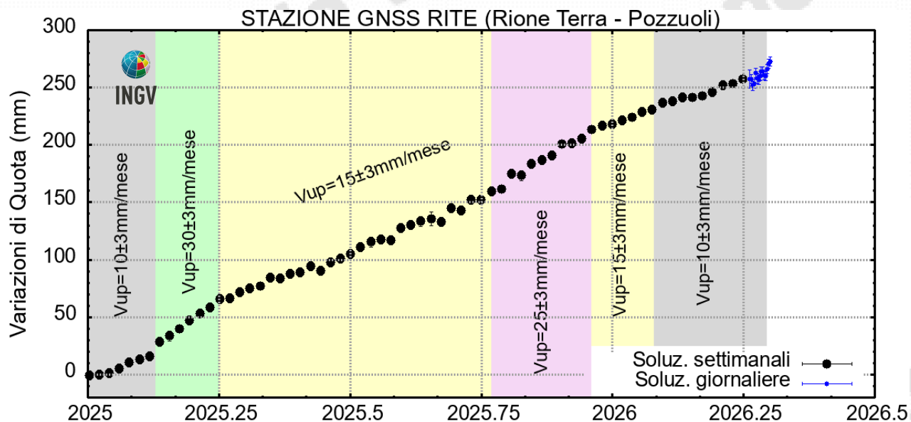
Figura 4.2 – Serie temporale delle variazioni in quota della stazione GNSS di RITE dal 01/01/2025 al 20/04/2026. Elaborazione dati in modalità differenziale singola baseline con software GNSS Spider.
