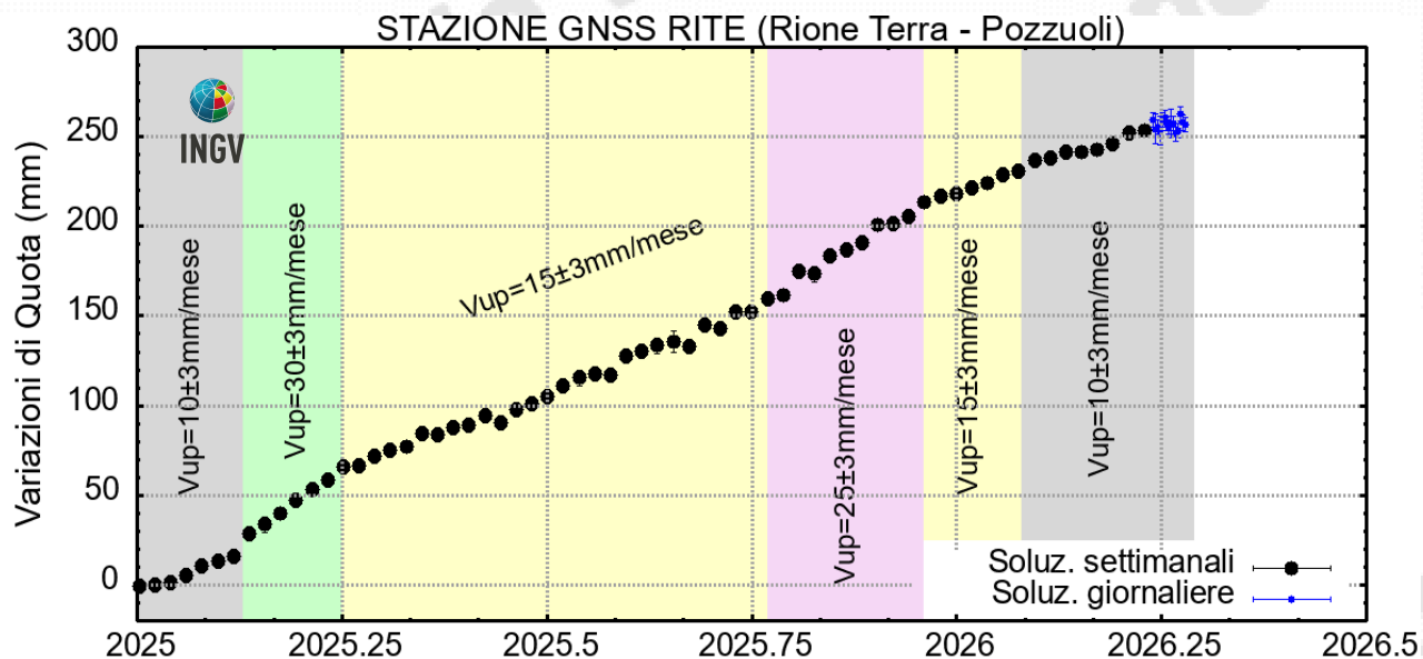
Figura 4.2 – Serie temporale delle variazioni in quota della stazione GNSS di RITE dal 01/01/2025 al 12/04/2026. Elaborazione dati in modalità differenziale singola baseline con software GNSS Spider.
