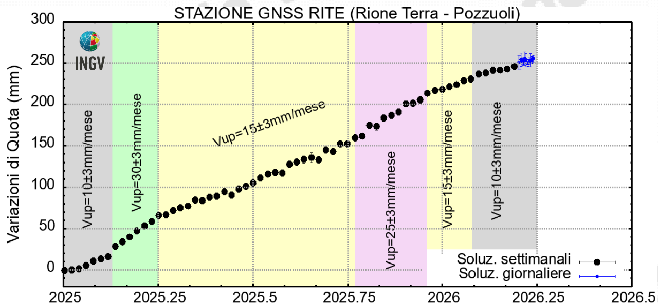
Figura 4.2 – Serie temporale delle variazioni in quota della stazione GNSS di RITE dal 01/01/2025 al 29/03/2026. Elaborazione dati in modalità differenziale singola baseline con software GNSS Spider.
