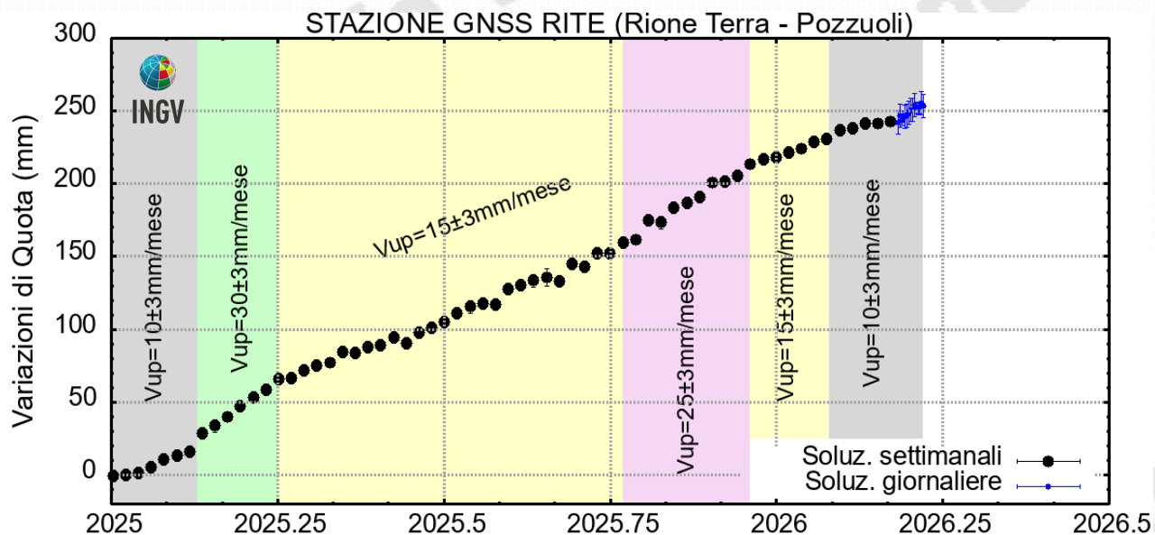
Figura 4.2 – Serie temporale delle variazioni in quota della stazione GNSS di RITE dal 01/01/2025 al 22/03/2026. Elaborazione dati in modalità differenziale singola baseline con software GNSS Spider.
