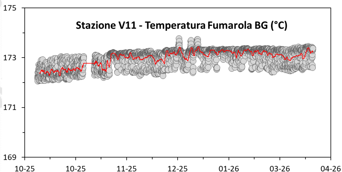
Figura 5.3 Valori della temperatura della fumarola BG misurati dalla stazione V11 installata nel cratere della Solfatara a pochi metri dalla fumarola principale BG.
