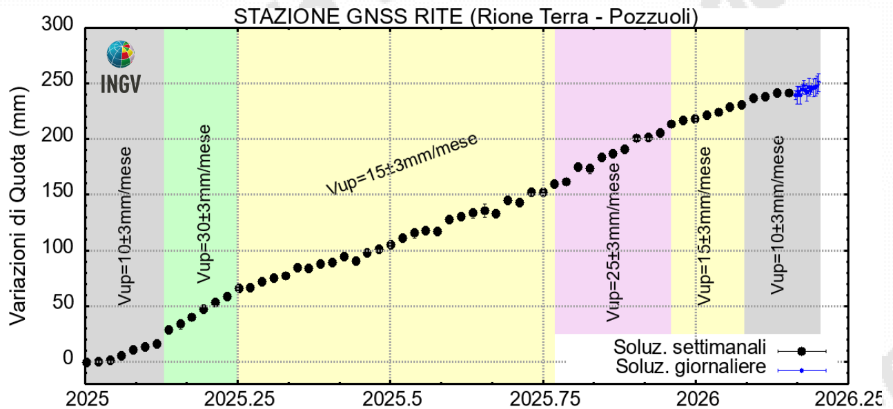
Figura 4.2 – Serie temporale delle variazioni in quota della stazione GNSS di RITE dal 01/01/2025 al 15/03/2026. Elaborazione dati in modalità differenziale singola baseline con software GNSS Spider.
