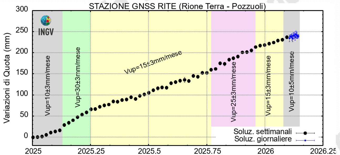
Figura 4.2 – Serie temporale delle variazioni in quota della stazione GNSS di RITE dal 01/01/2025 al 22/02/2026. Elaborazione dati in modalità differenziale singola baseline con software GNSS Spider.
