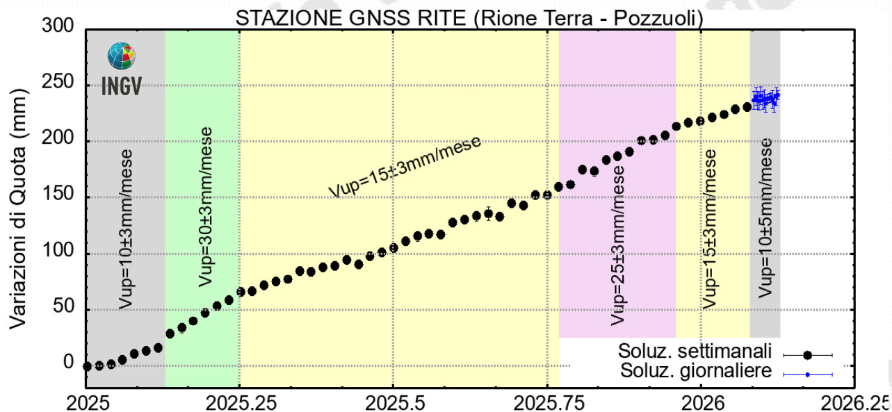
Figura 4.2 – Serie temporale delle variazioni in quota della stazione GNSS di RITE dal 01/01/2025 al 15/02/2026. Elaborazione dati in modalità differenziale singola baseline con software GNSS Spider.
