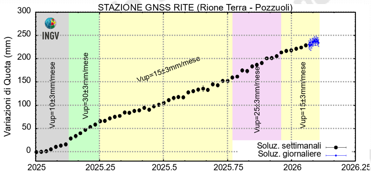
Figura 4.2 – Serie temporale delle variazioni in quota della stazione GNSS di RITE dal 01/01/2025 al 08/02/2026. Elaborazione dati in modalità differenziale singola baseline con software GNSS Spider.
