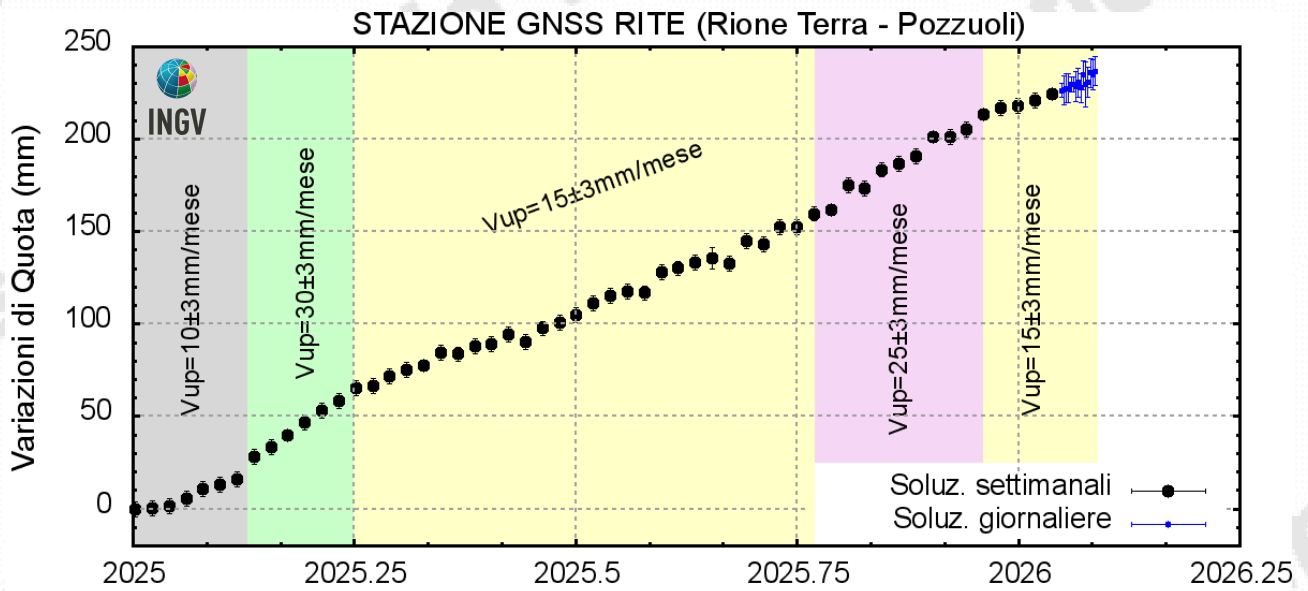
Figura 4.2 – Serie temporale delle variazioni in quota della stazione GNSS di RITE dal 01/01/2025 al 01/02/2026. Elaborazione dati in modalità differenziale singola baseline con software GNSS Spider.
