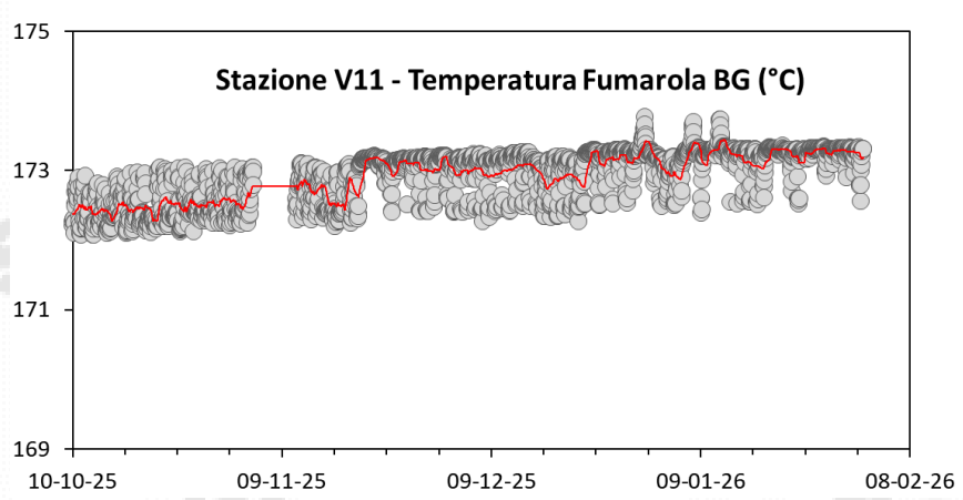
Figura 5.3 Valori della temperatura della fumarola BG misurati dalla stazione FLXOV5 (in alto) e dalla stazione V11 (in basso) installate nel cratere della Solfatara a pochi metri dalla fumarola principale BG. Si noti il trend di aumento degli ultimi anni misurato dalla stazione FLXOV5.
